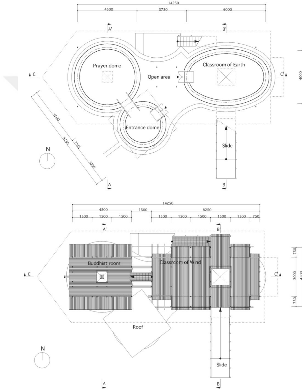
Şekil 5.3. Shangkhabori Köy Okulu zemin kat ve vaziyet planı;
