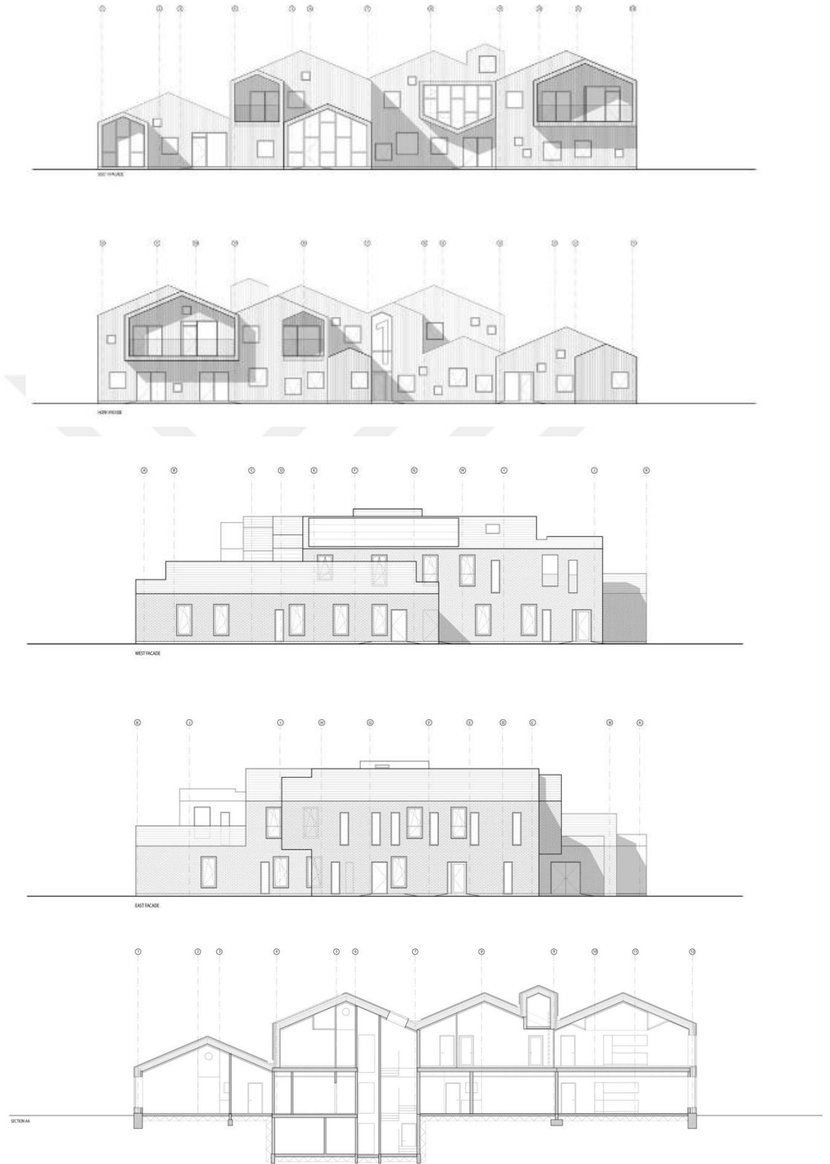
Şekil 5.5. Kerteminde Bakım Evi görünüşleri ve kesiti; https://www.arquine.com/casa-del-futuro-para-ninos/ ; erişim tarihi: Kasım 2018
