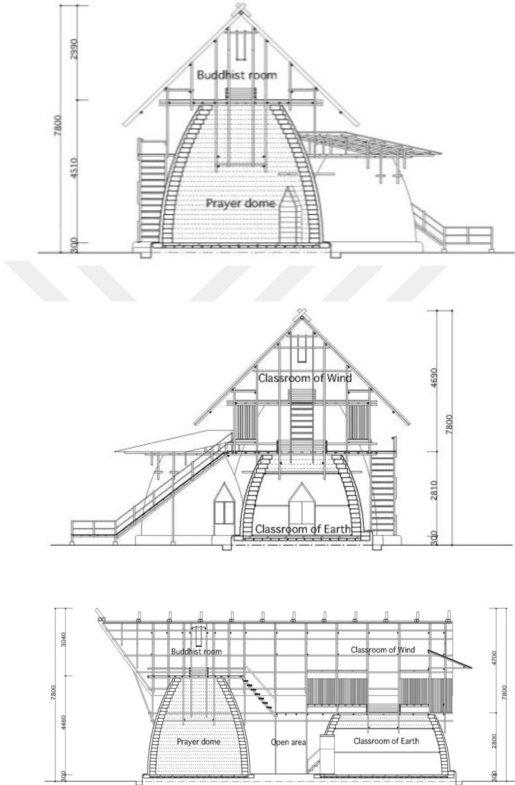
Şekil 5.4. Shangkhaburi Köy Okulu kesitleri;
