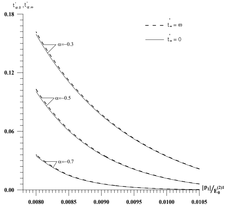
Şekil 2.12 E_0^{(2)1}/E^{(1)1} = 0,05 , \alpha = -0,5 , \pi h/\ell_1 = 0,15 durumunda \omega reolojik parametresinin farklı değerleri için kritik zaman ( t'_{\text{cr},0} , t'_{\text{cr},\infty} ) ile |p_1|/E_0^{(2)1} ilişkisi
