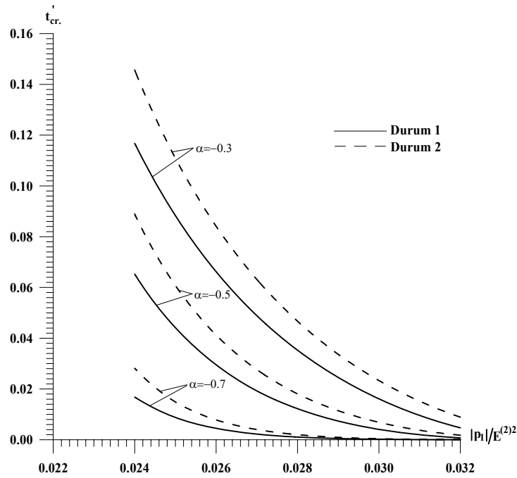
Şekil 2.22 h = h_1^{(1)} + h_1^{(2)} + h_2^{(1)} , h_1^{(1)} = h_1^{(2)} = h_2^{(1)} , \alpha = -0,5 , \pi h/\ell_1 = 0,75 durumunda \omega reolojik parametresinin farklı değerleri için kritik zaman ( t'_{cr.} ) ile |p_1|/E^{(2)2} ilişkisi.
