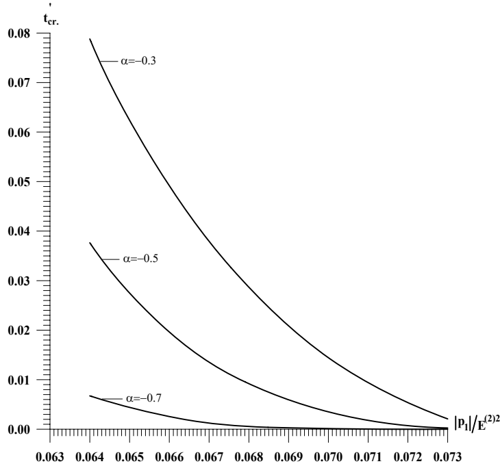
Şekil 2.18 h_1^{(1)} = 0,5 * h , h_1^{(2)} = 0,5 * h , \alpha = -0,5 , \pi h / \ell_1 = 1,25 durumunda \omega reolojik parametresinin farklı değerleri için kritik zaman ( t'_{cr} ) ile |p_1|/E^{(2)2} ilişkisi
