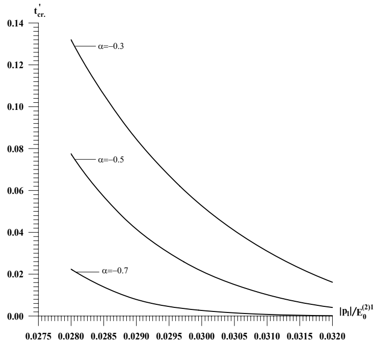
Şekil 2.26 \kappa=1 , E_0^{(2)1}/E^{(1)1}=0,05 , \alpha=-0,5 , \pi h_1^{(1)}/\ell_1=0,200 durumunda \omega reolojik parametresinin farklı değerleri için kritik zaman ( t'_{cr.} ) ile |p_1|/E_0^{(2)1} ilişkisi
