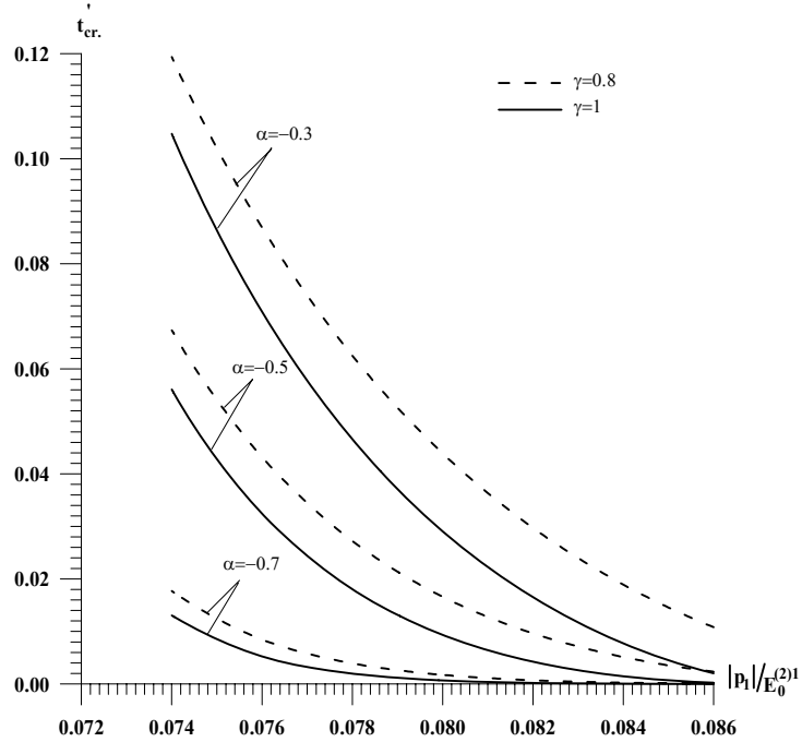
Şekil 3.36 \kappa=1 , p_3=p_1 , \gamma=0,8 , \gamma=1 , E_0^{(2)1}/E^{(1)1}=0,05 , \omega=1 , \pi h_1^{(1)}/\ell_1=0,150 durumunda \alpha reolojik parametresinin farklı değerleri için kritik zaman ( t'_{cr.} ) ile |p_1|/E_0^{(2)1} ilişkisi
