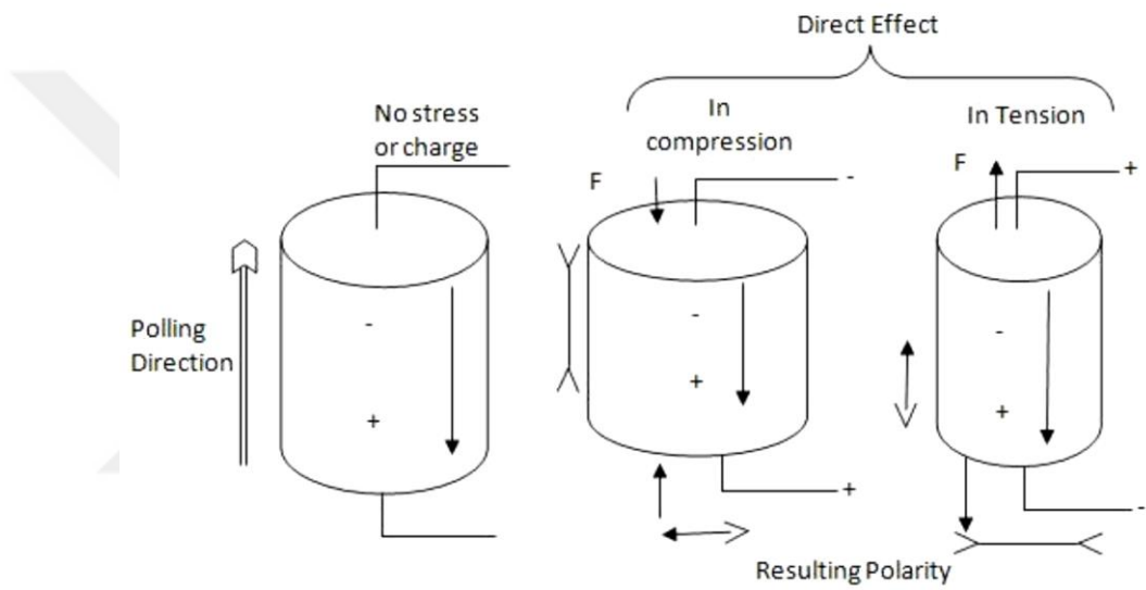
Şekil 3.7. Direkt piezoelektrik etki [77]
