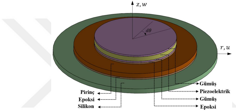
Şekil 3.2. Polar koordinat sistemine sahip 7 katmanlı dairesele aktüatörün yapısı
