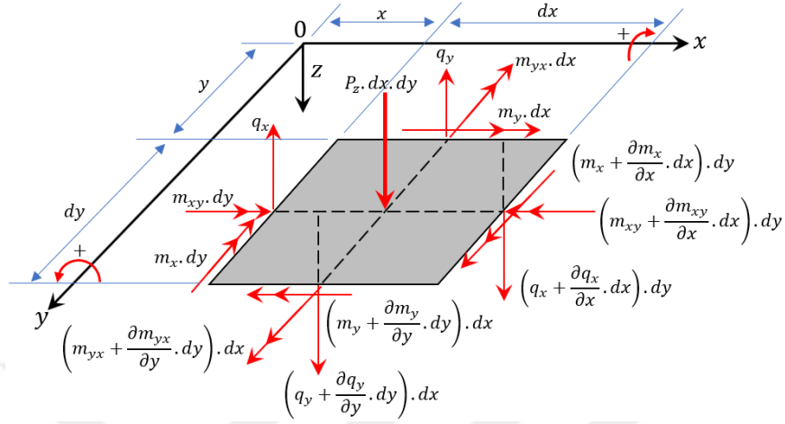
Şekil 2.7. Tarafsız düzlem üzerindeki kuvvet ve moment dengesi
