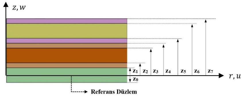
Şekil 3.5. Analitik modellemede kullanılan aktüatörün katmanlarının referans düzleme göre olan mesafeleri
