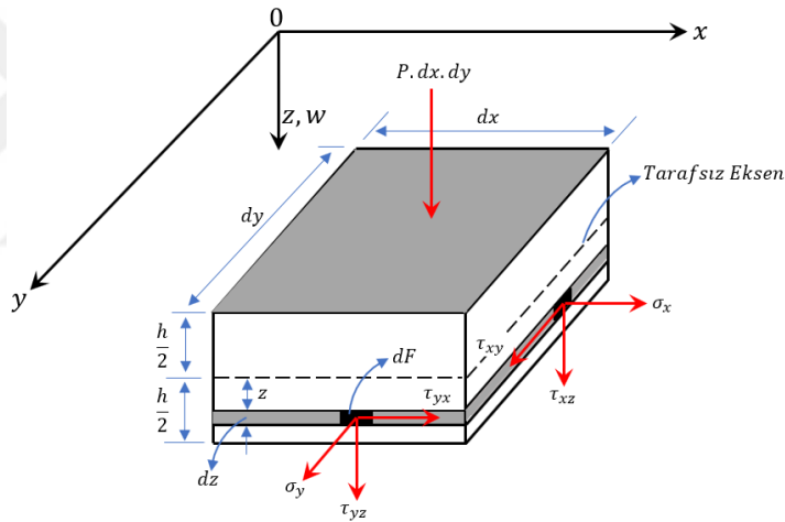
Şekil 2.5. Plâgın birim elemanı üzerindeki gerilmeler
