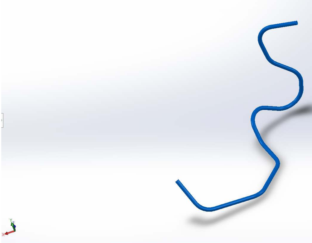
Şekil 3.6. Yakıt borusu üç boyutlu modeli-2
