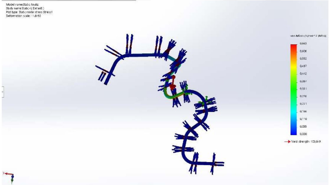
Şekil 4.10. Gerilme analiz sonuçları-4
