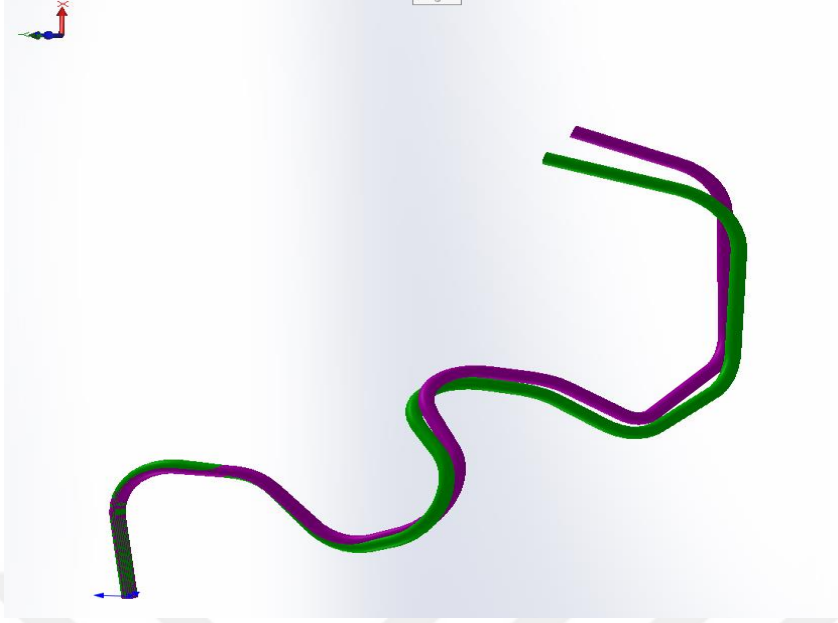
Şekil 4.3. Analiz sonucuna göre elde edilen datanın fırın prosesi sonrası taranan data ile çakıştırılması-2
