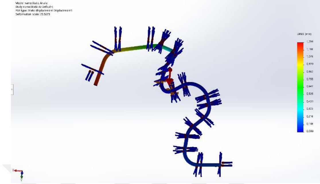
Şekil 4.9. Yer değıştirme analiz sonuçları-3
