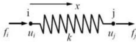
Şekil 3.4. Doğrusal yayın serbest cisim diyagramı (Tursun 2019)
