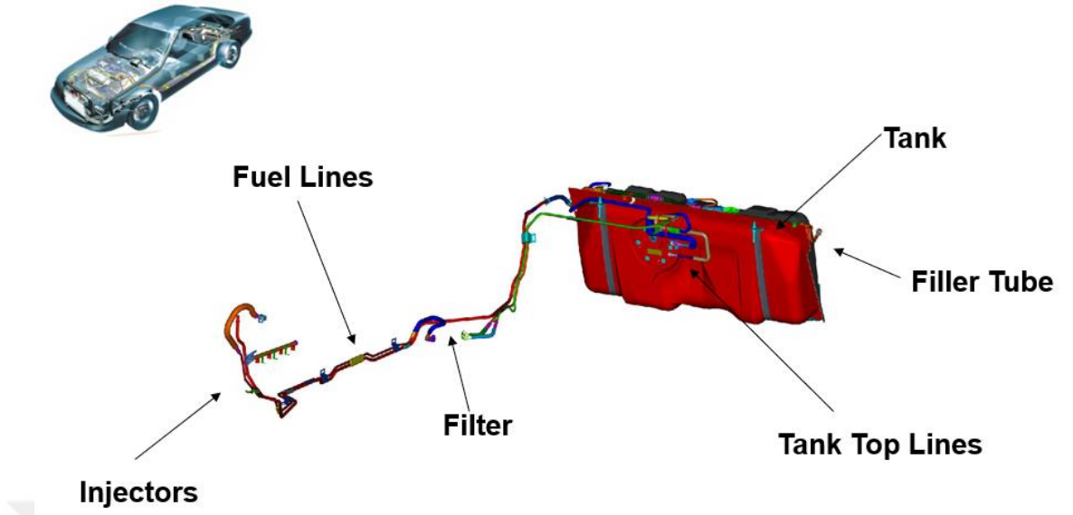
Şekil 2.2. Araç yakıt sistemi şeması-2
