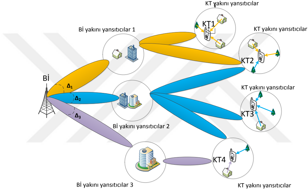
Şekil 2-6 Yoğun MIMO Kanalındaki Bireysel ve Ortak Seyreklik Gösterimi
