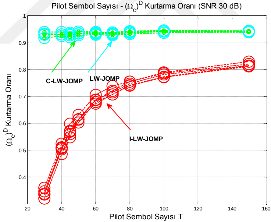
Şekil 6-25 Aşağı Yönlü ve Yukarı Yönlü Kanal Merkez Frekans Farkına Bağlı Pilot Sembol Sayısına Karşılık (\Omega_c)^D Kurtarma Oranının Değişimi - SNR = 30\text{ dB}
