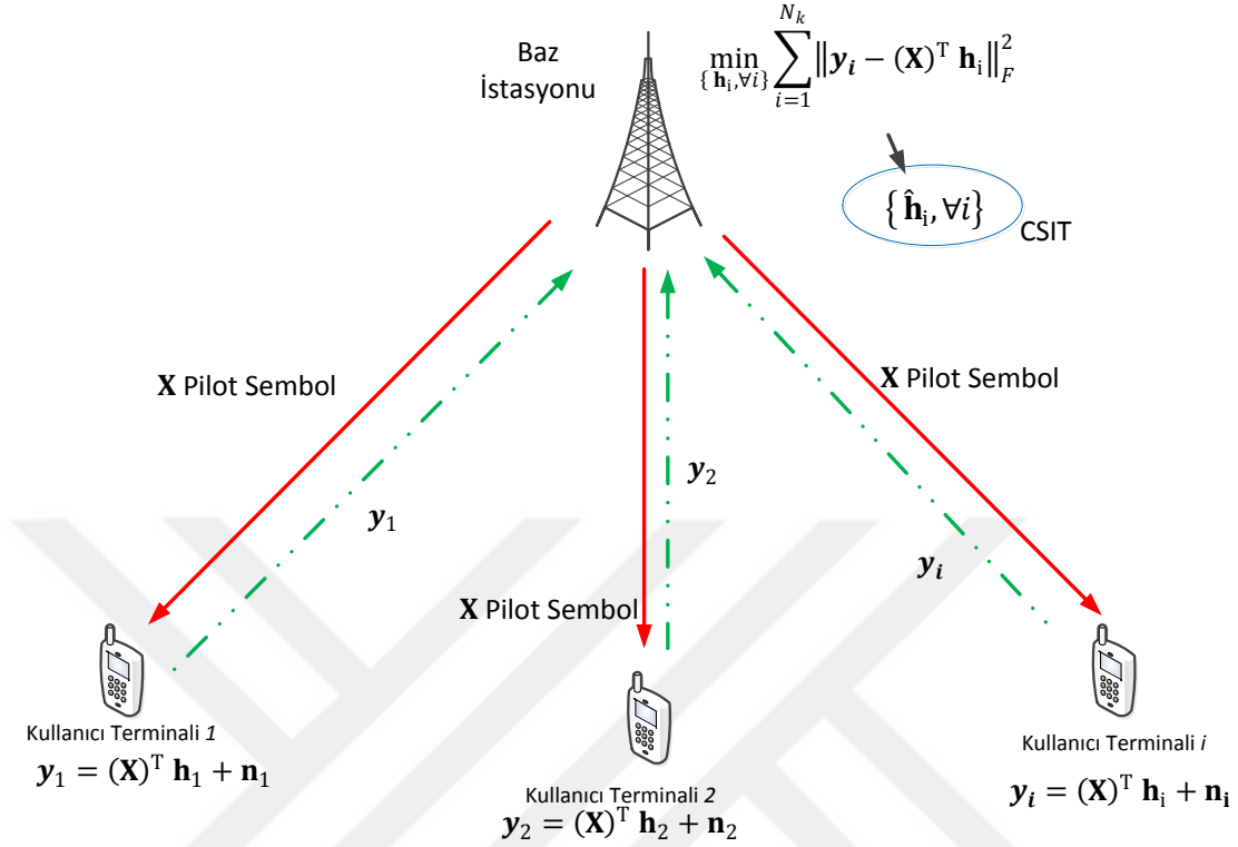
Şekil 4-4 Dağıtık Şıkıştırılmış Algılama Aşağı Yönlü Kanal Durum Bilgisi Kestirimi
