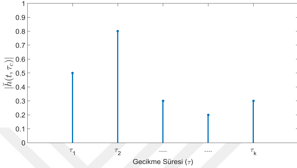
Şekil 4-2 Kanal Vektörü Gecikme Yayılmı
