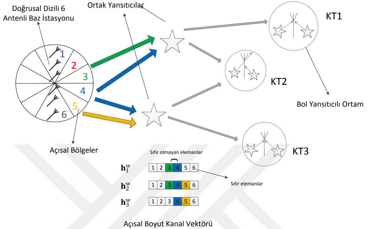
Şekil 4-3 Baz İstasyonu ve Yansıtıcıların Açısal Boyut ile İlişkisi Yoğun MIMO kanalına ait seyreklik Eşitlik (3.1)'e benzer olarak
