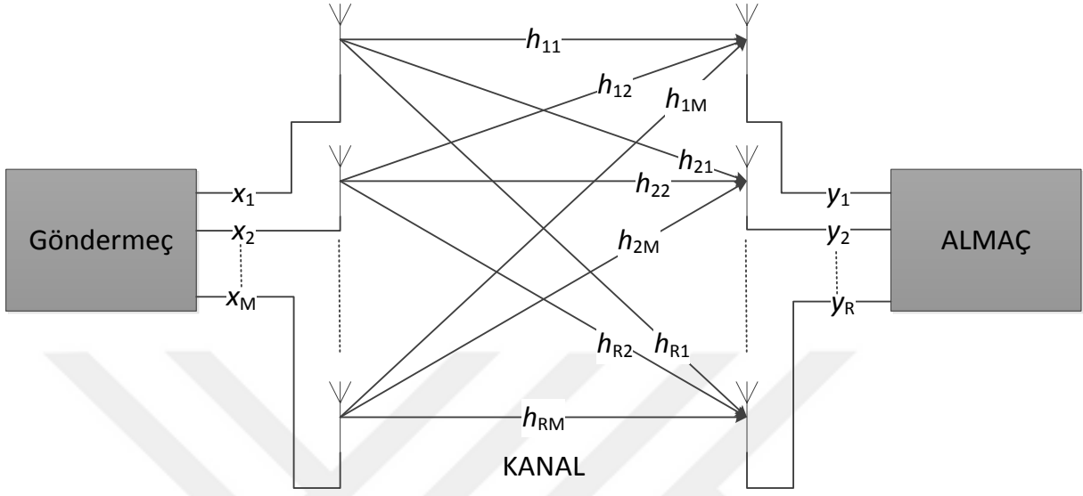
Şekil 2-1 Çok Girişli Çok Çıkışlı Haberleşme Sistemi
