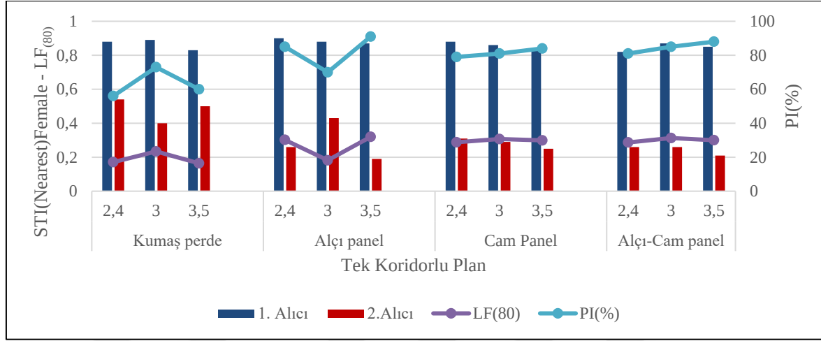
Şekil 6.26. Senaryo 4- Tek koridorlu plan STI(nearest)Female – LF_{(80)} - PI(%) grafiği
