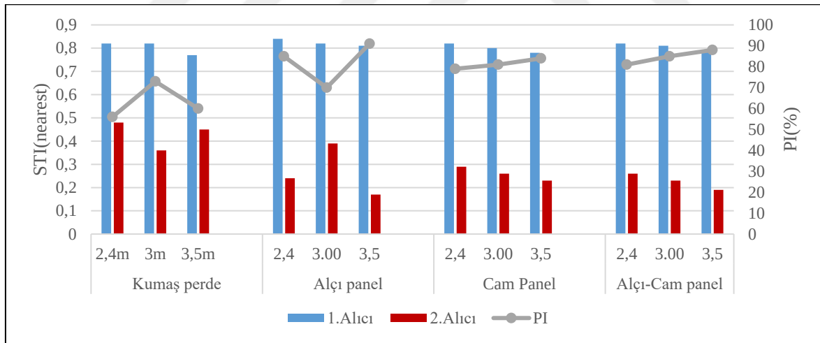
Şekil 6.9. Senaryo 3 - Tek koridorlu plan STI-PI(%) grafiği
