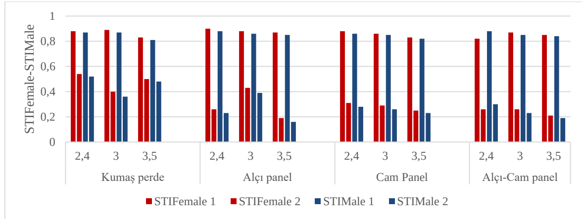
Şekil 6.28. Senaryo 4 - Tek Koridorlu Plan STIFemale-STI Male grafiği
