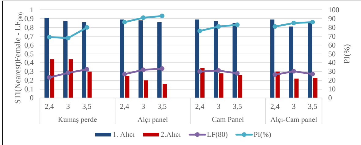
Şekil 6.32. Senaryo 4 - Çift koridorlu plan STI(Nearest) female-PI(%) grafiği
