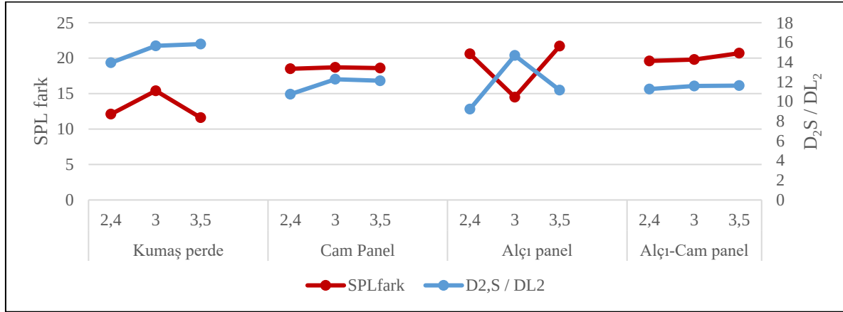
Şekil 6.12. Senaryo 3 - Tek koridorlu plan D_2S / DL_2 - SPLfark grafiği
