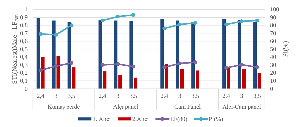
Şekil 6.33. Senaryo 4 - Çift koridorlu plan STI(Nearest) Male - PI(%) grafiği
