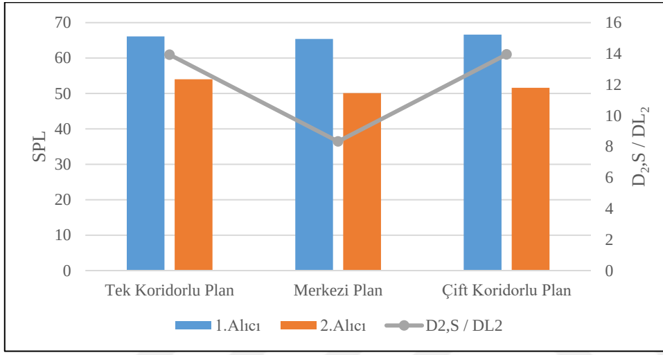
Şekil 6.1. Senaryo 1 - Plan tiplerine göre SPL - D_{2,S} / DL_2 grafiği
