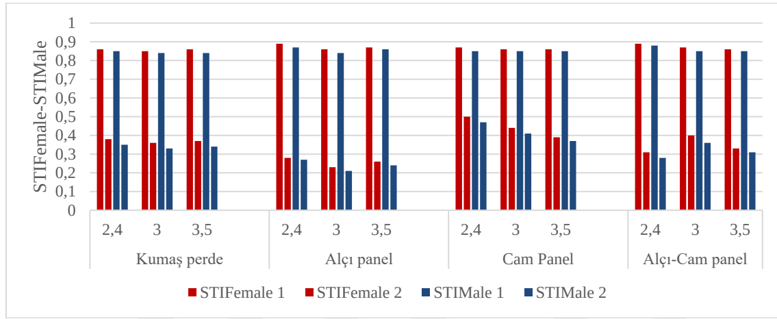
Şekil 6.31. Senaryo 4- Merkezi plan STI Female-STI Male-PI(%) grafiği
