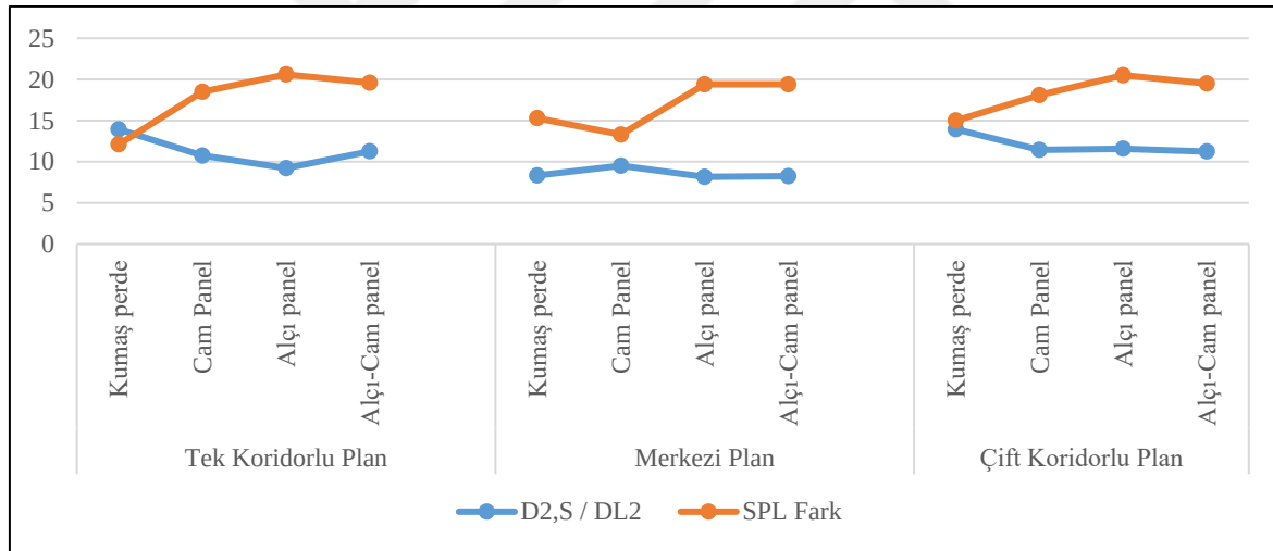
Şekil 6.5. Senaryo 2 - Plan tipleri ve bölme panellere göre D 2 S / DL 2 -SPL fark grafiği
