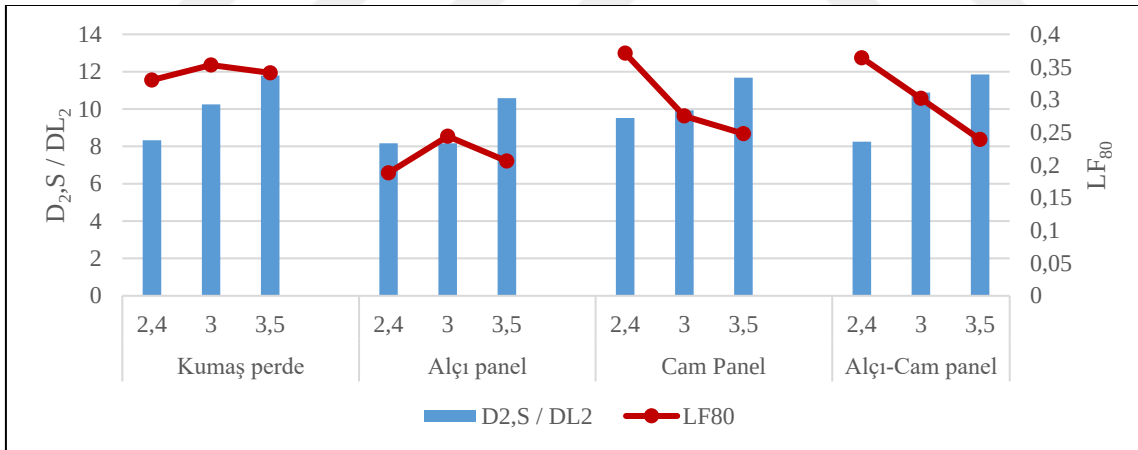
Şekil 6.15. Senaryo 3 - Merkezi plan D_{2,S} / DL_2 - LF_{80} grafiği
