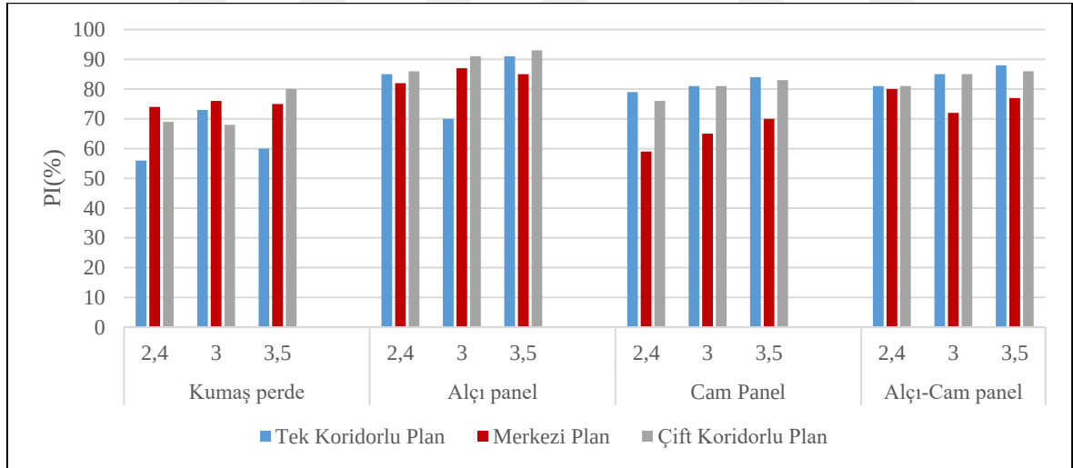
Şekil 6.24. Senaryo 3- Plan tiplerine göre PI(%) grafiği
