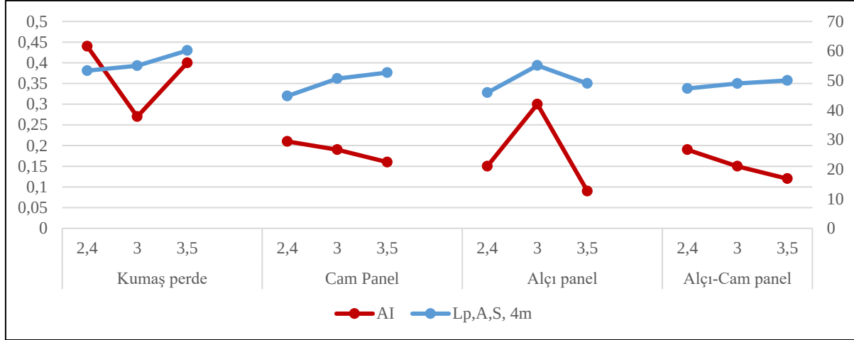
Şekil 6.13. Senaryo 3 - Tek koridorlu plan L_{p,A,S,4m} - AI grafiği
