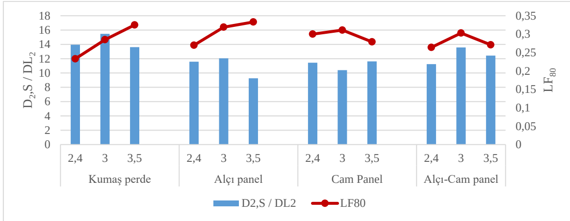
Şekil 6.21. Senaryo 3 - Çift koridorlu plan D 2,S /DL 2 - LF 80 grafiği
