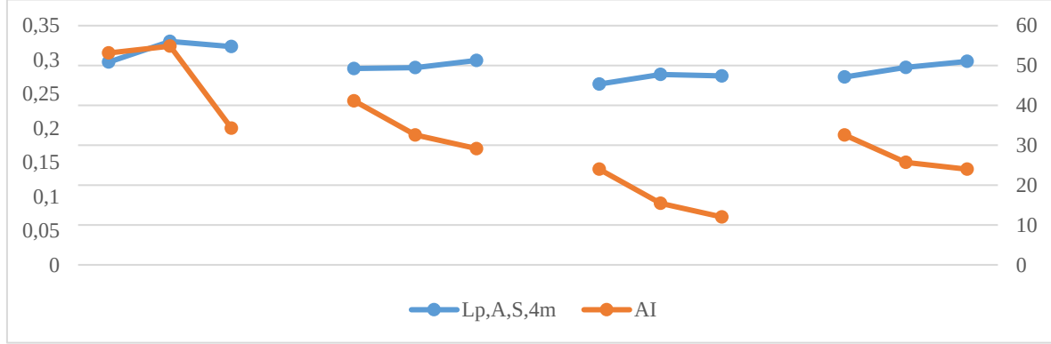
Şekil 6.23. Senaryo 3 - Çift koridorlu plan L_{p, A,S,4m} - AI grafiği
