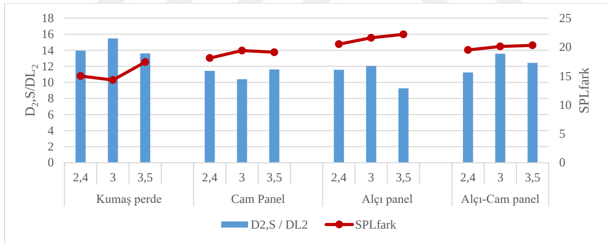
Şekil 6.22. Senaryo 3 - Çift koridorlu plan D 2,S /DL 2 - SPLfark grafiği
