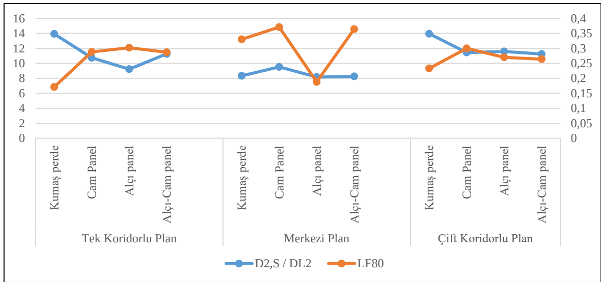
Şekil 6.6. Senaryo 2 - Plan tipleri ve bölme panellere göre D 2 S / DL 2 –LF 80 grafiği
