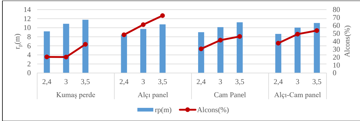
Şekil 6.20. Senaryo 3 - Çift koridorlu plan r_p -Alcons grafiği
