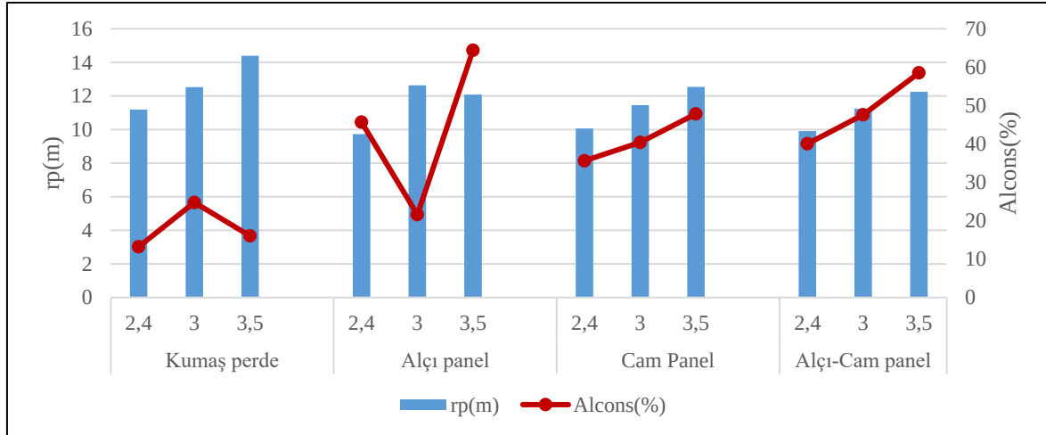
Şekil 6.10. Senaryo 3 - Tek koridorlu plan r_p -Alcons grafiği
