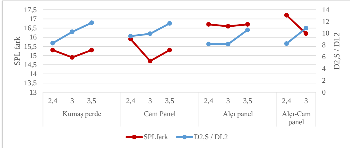
Şekil 6.16. Senaryo 3 - Merkezi plan D_{2,S} / DL_2 -SPLfark grafiği
