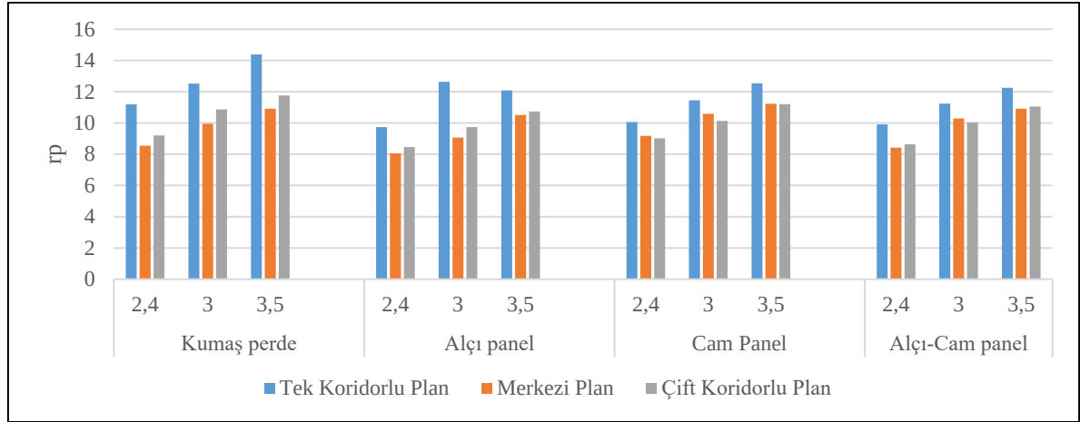
Şekil 6.25. Senaryo 3- Plan tiplerine göre r_p grafiği
