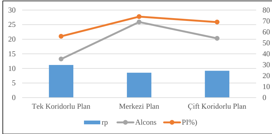
Şekil 6.3. Senaryo 1 - Plan tiplerine göre r_p(m) - PI(%)-Alcons) grafiği
