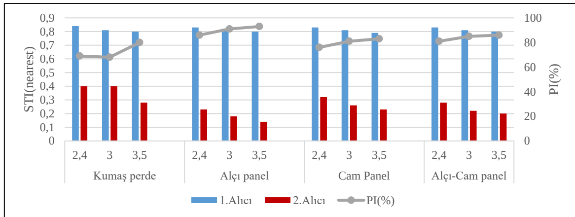
Şekil 6.19. Senaryo 3 - Çift koridorlu plan STI(nearest)-PI(%) grafiği
