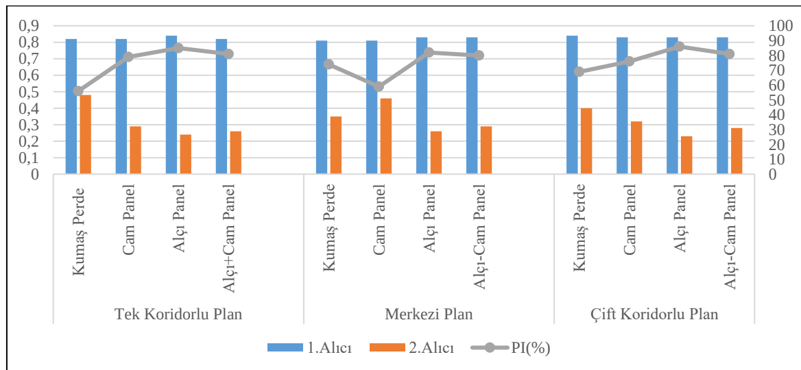
Şekil 6.4. Senaryo 2 - Plan tipleri ve bölme panellere göre STI - PI grafiği
