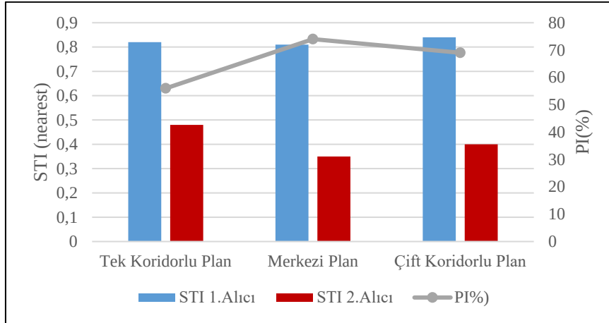
Şekil 6.2. Senaryo 1 - Plan tiplerine göre STI (nearest)-PI grafiği
