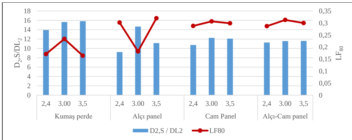
Şekil 6.11. Senaryo 3 - Tek koridorlu plan D_{2,S} / DL_2 - LF_{80} grafiği
