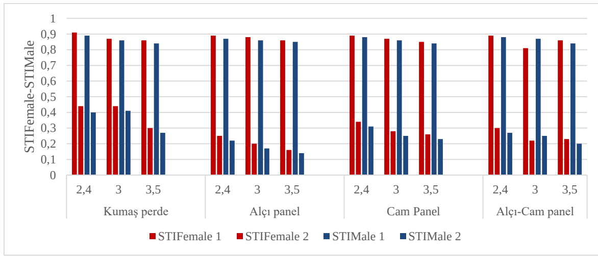
Şekil 6.34. Senaryo 4 - Çift Koridorlu Plan STI Female-STI Male grafiği
