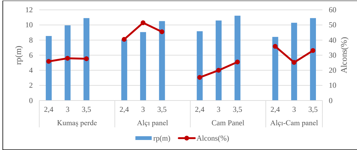
Şekil 6.18. Senaryo 3 - Merkezi plan r p -Alcons grafiği
