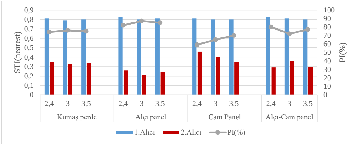
Şekil 6.14. Senaryo 3 - Merkezi plan STI(nearest)-PI(%) grafiği
