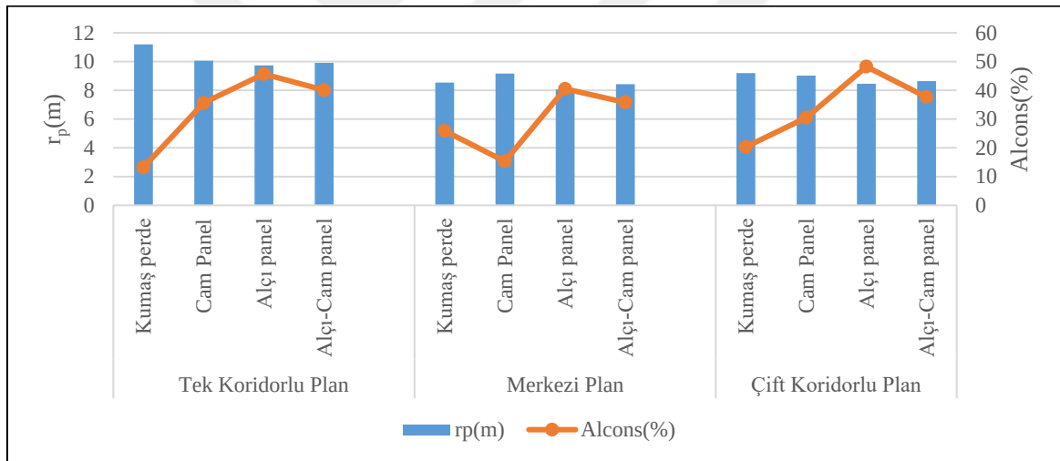
Şekil 6.8. Senaryo 2 - Plan tipleri ve bölme elemanlarına göre r_p(m) -Alcons(%) grafiği
