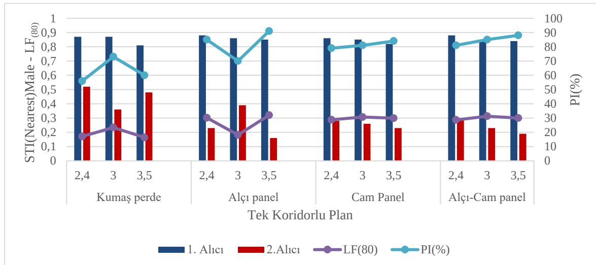
Şekil 6.27. Senaryo 4- Tek koridorlu plan STI(nearest)Male – LF_{(80)} – PI(%) grafiği
