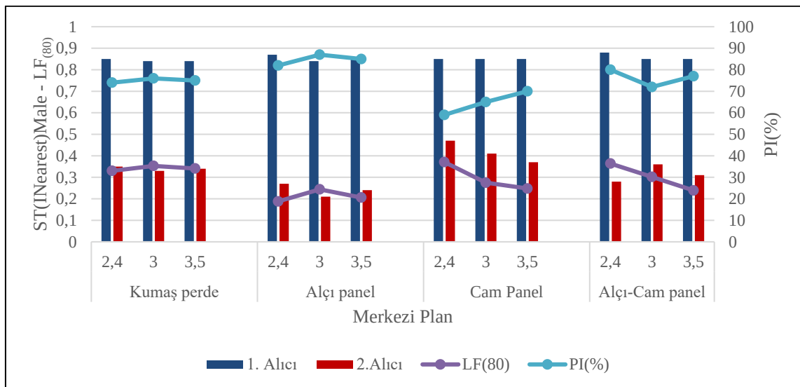
Şekil 6.30. Senaryo 4- Merkezi plan STI Male – LF (80) grafiği
