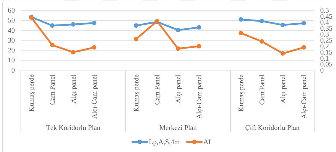
Şekil 6.7. Senaryo 2 - Plan tipleri ve bölme panellere göre L_{p,A,S,4m} - AI grafiği
