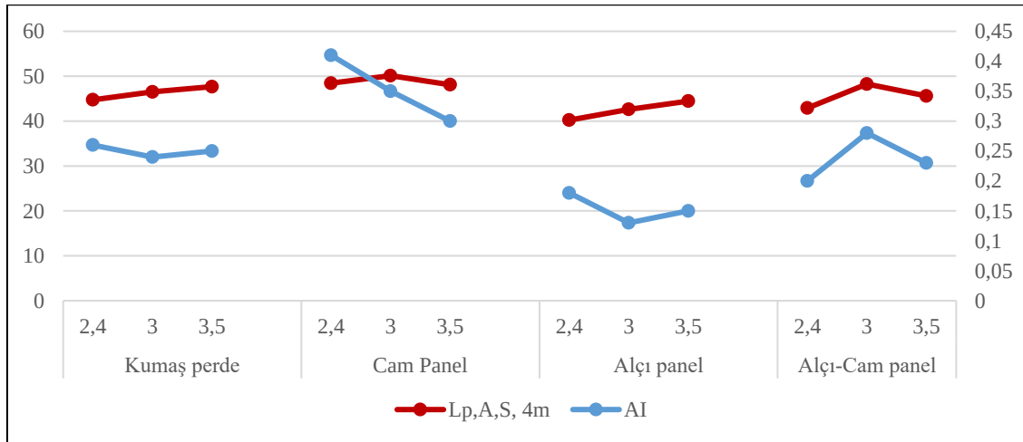
Şekil 6.17. Senaryo 3 - Merkezi plan L_{p,A,S,4m} – AI grafiği
