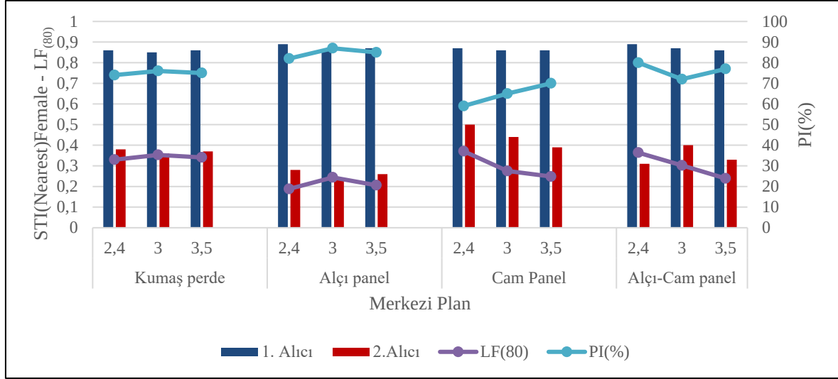
Şekil 6.29. Senaryo 4- Merkezi plan STI(Nearest) Female – LF (80) – PI grafiği
