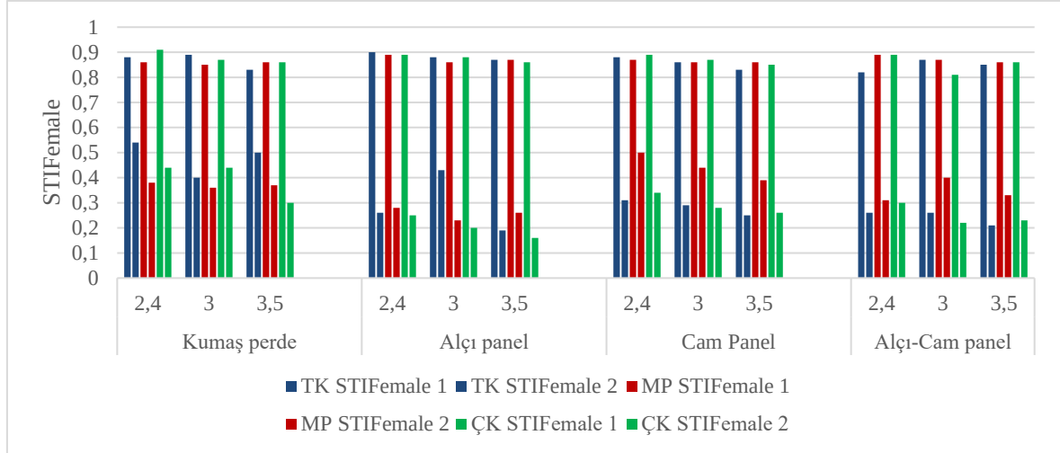
Şekil 6.35. Senaryo 4 - STIFemale grafiği
