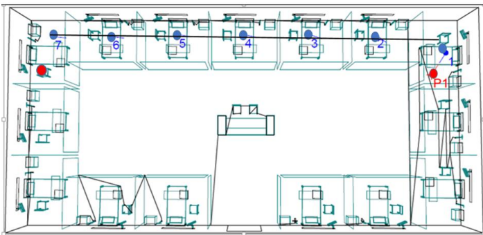
Şekil 5.3. Merkezi plan tipinde kaynak-alıcı noktaları
