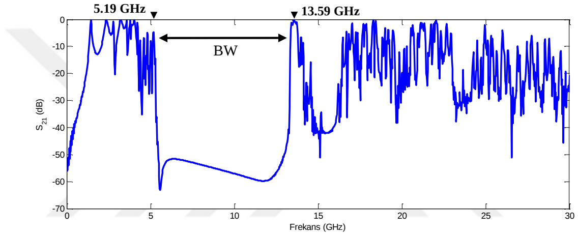
Şekil 4.3. Sadece dairesel kesitli pin dizisi içeren PMC yüzeyin frekansa bağlı iletim parametre değerleri
