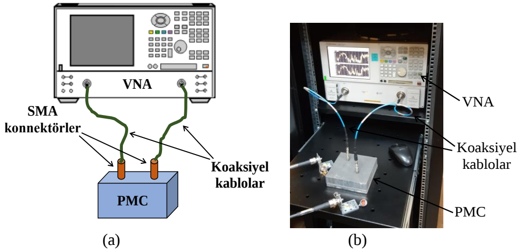
Şekil 4.13. Dairesel ve kare kesitli pin dizisi içeren multi-bant PMC yapının (a) elektriksel test düzeneğinin şematik gösterimi, ve (b) elektriksel test anını gösteren görsel
