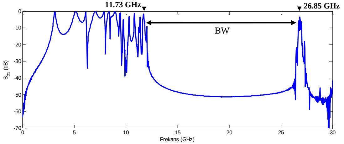
Şekil 4.5. Sadece kare kesitli pin dizileri içeren PMC yapının frekansa bađlı iletim parametre değeri
