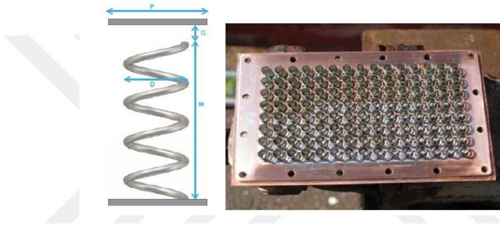
Şekil 3.4. Düşük frekanslar için çözüm ve üretilen prototipi [33]
