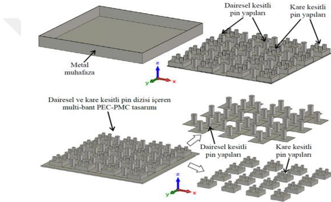
Şekil 4.6. Dairesel ve kare kesitli pin dizileri içeren multi-bant PMC yapı (üstte) pin yapıları, (altta) genel görünüş
