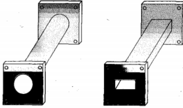
Şekil 2.1. Dairesel ve dikdörtgen yapıları dalga kılavuzları [3]
