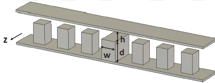
Şekil 2.10. Sonsuz z düzlemi boyunca dağılım merkezi sırt olan bir pim dizisi diyagramı [25]
