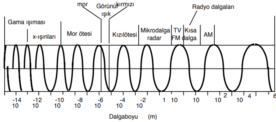
Şekil 1.1. Elektromanyetik spektrum [13]
