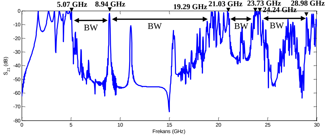
Şekil 4.7. Dairesel ve kare kesitli pin dizileri içeren multi-bant PMC yapının frekansa bağlı iletim parametre değerleri
