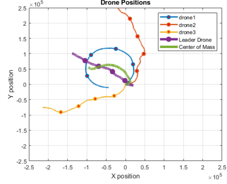
(d) 200 km communication range.
