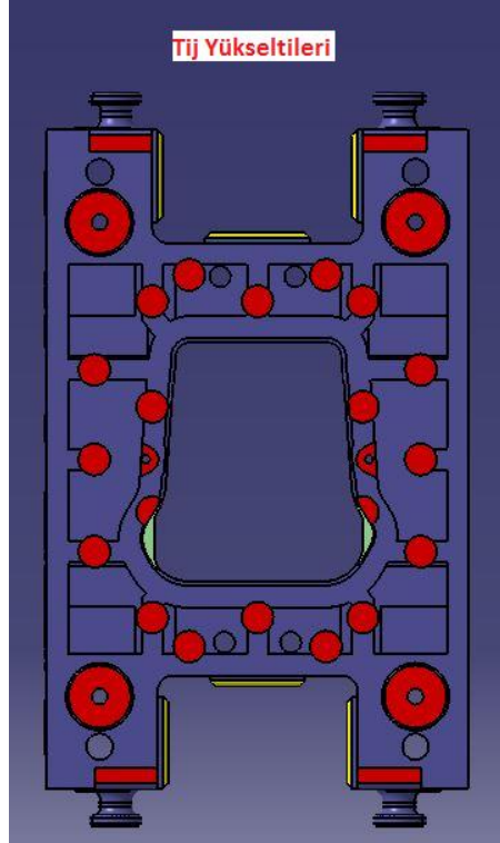
Şekil 78: Pot Çemberindeki Tij Eklmeleri
