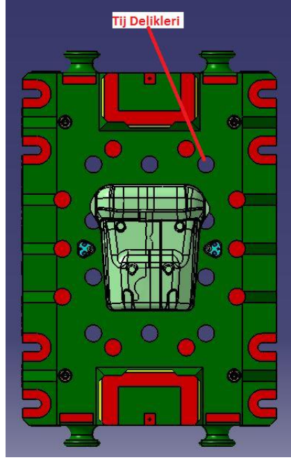
Şekil 77: Alt Dökümde ki Tij Delikleri
