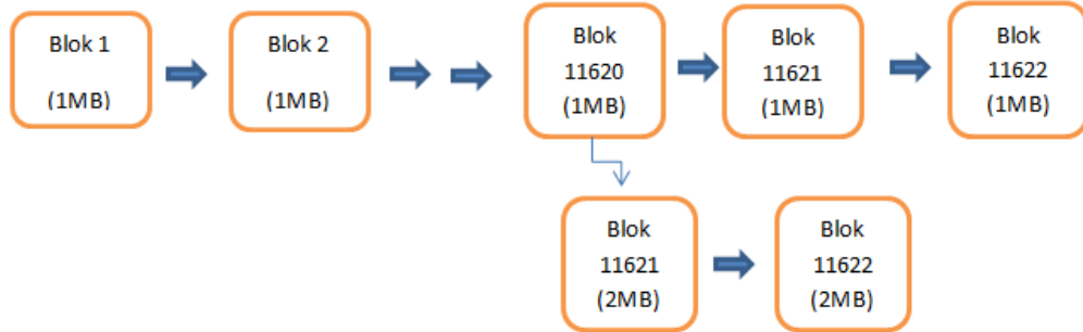
Şekil 7: Mecburi Çatallanma
