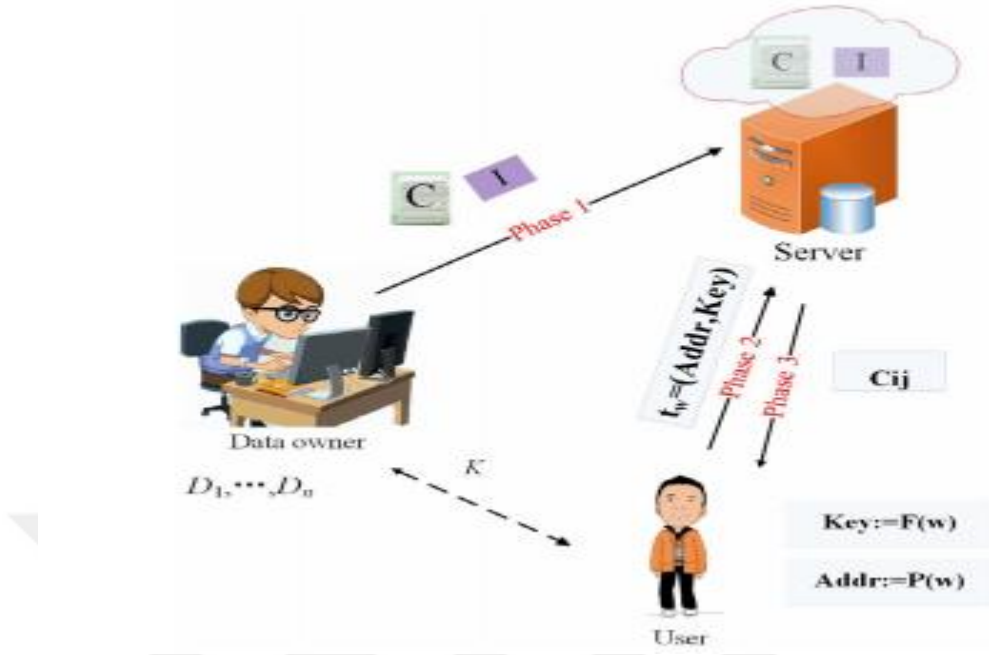
Şekil 3: Simetrik Şifreleme
