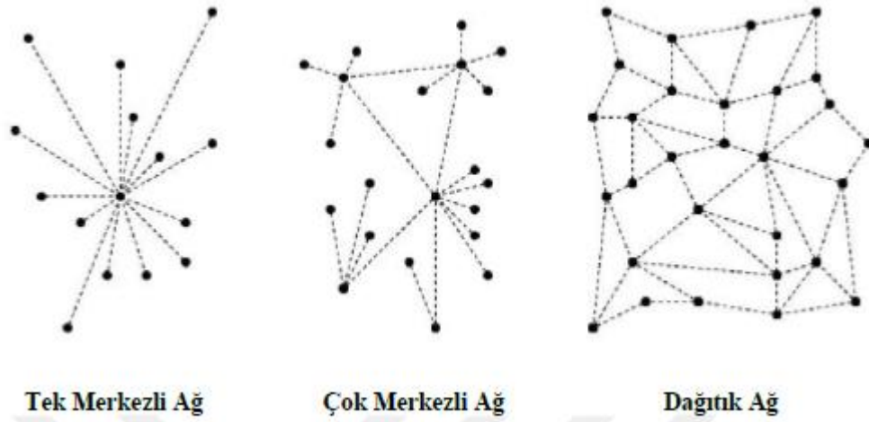
Şekil 1: Blokzincir Yapısı
