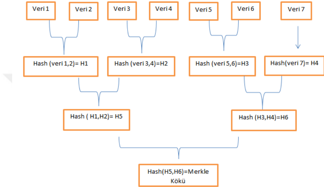
Şekil 5: Merkle Kökü
