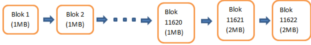
Şekil 6: Gönüllü Çatallanma
