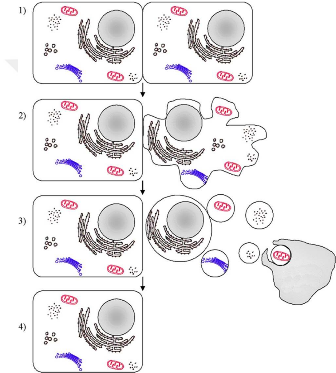
Şekil 6. Apoptozun evreleri 54
