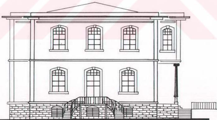
Şekil 47. Orduevi Misafirhanesi Yan Görünüş (Orduevi Misafirhanesi Arşivi)
