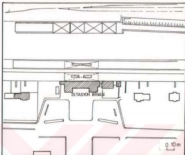
Şekil 26. İstasyon Binası Vaziyet Planı (TCDD Arşivi)
