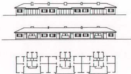
Şekil 71. "C" Tipi Ev Siluetleri
