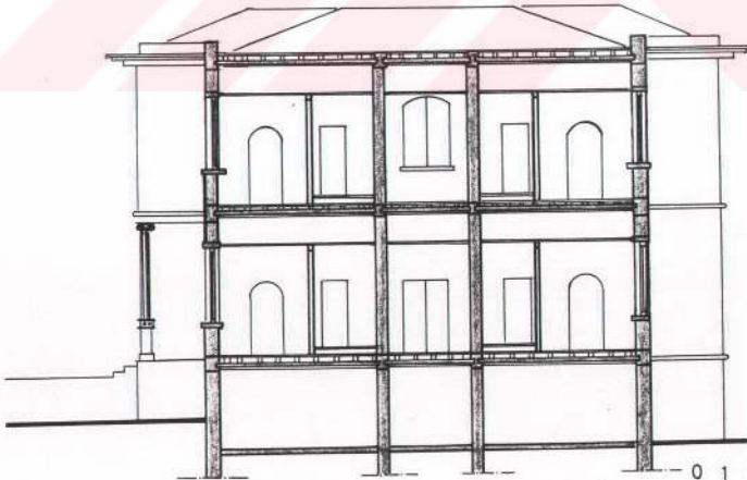
Şekil 45. Orduevi Misafirhanesi Enine Kesit
