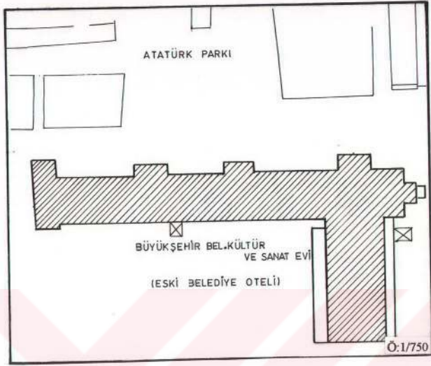
Şekil 75. Adana Eski Belediye Otelı Vaziyet Planı (Şeyhan Belediyesi)
