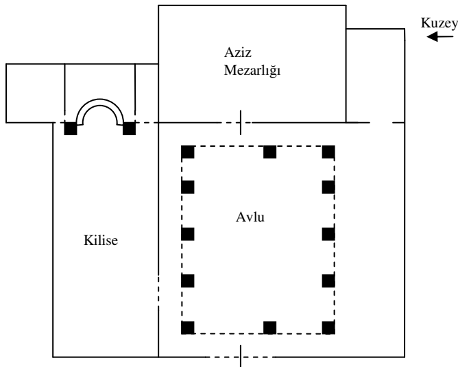
Şekil 3.44 Mor Evgin Manastırı Planı
