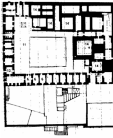
Şekil 3.5 Deyrul Zafaran Manastırı Ara Kat Planı
