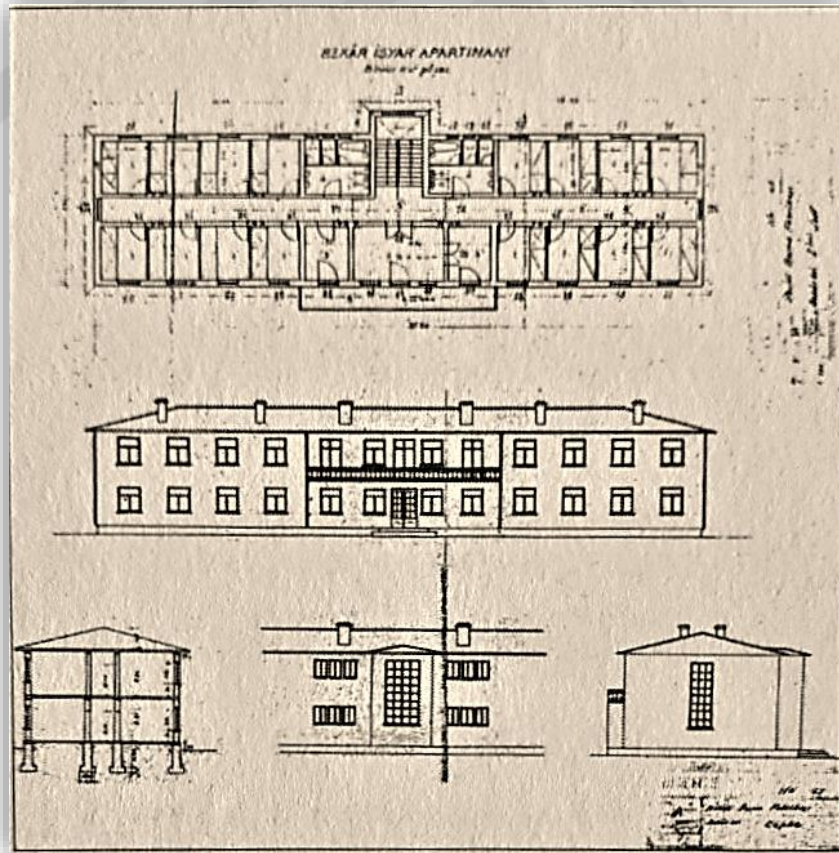
Şekil 3.11. Nazilli Basma Fabrikası Bekâr Memur Apartmanı Planı (20.01.1937)
