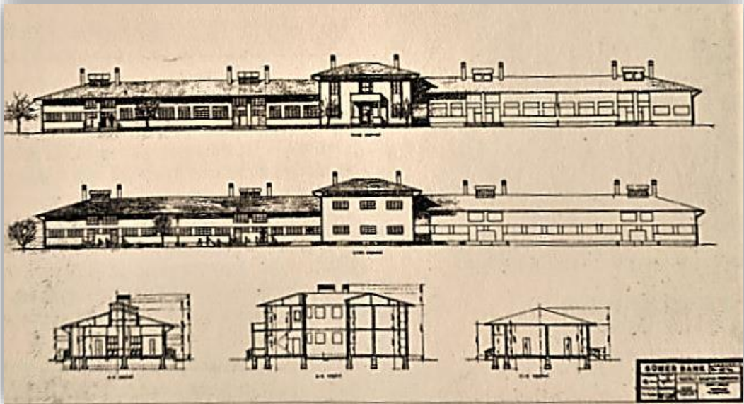
Şekil 3.9. Nazilli Basma Fabrikası İşçi Pavyonu Tadilat Projesi (4.12.1940)
