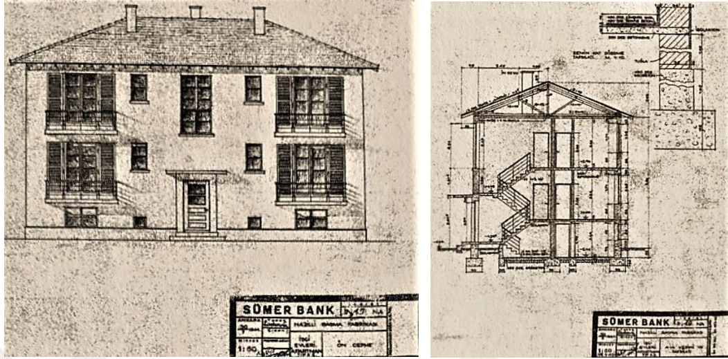
Şekil 3.10. Nazilli Basma Fabrikası İşçi Evleri, A2 Apartman Tipi (30.07.1941)
