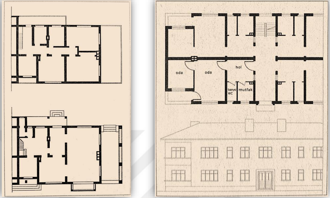
Şekil 3.8. Nazilli Basma Fabrikası Evli Memur Apartmanları (İç Apartmanlar) ve U Tipi Evli Memur Apartmanları
