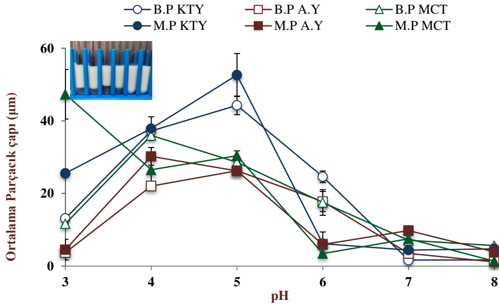
Şekil 5.11: pH değişiminin farklı emülgatörler (B.P ve M.P) ve farklı yağlar (KTY, A.Y ve MCT) ile stabilize edilen geleneksel emülsiyonlarda ortalama partikül çapı üzerindeki etkisi.
