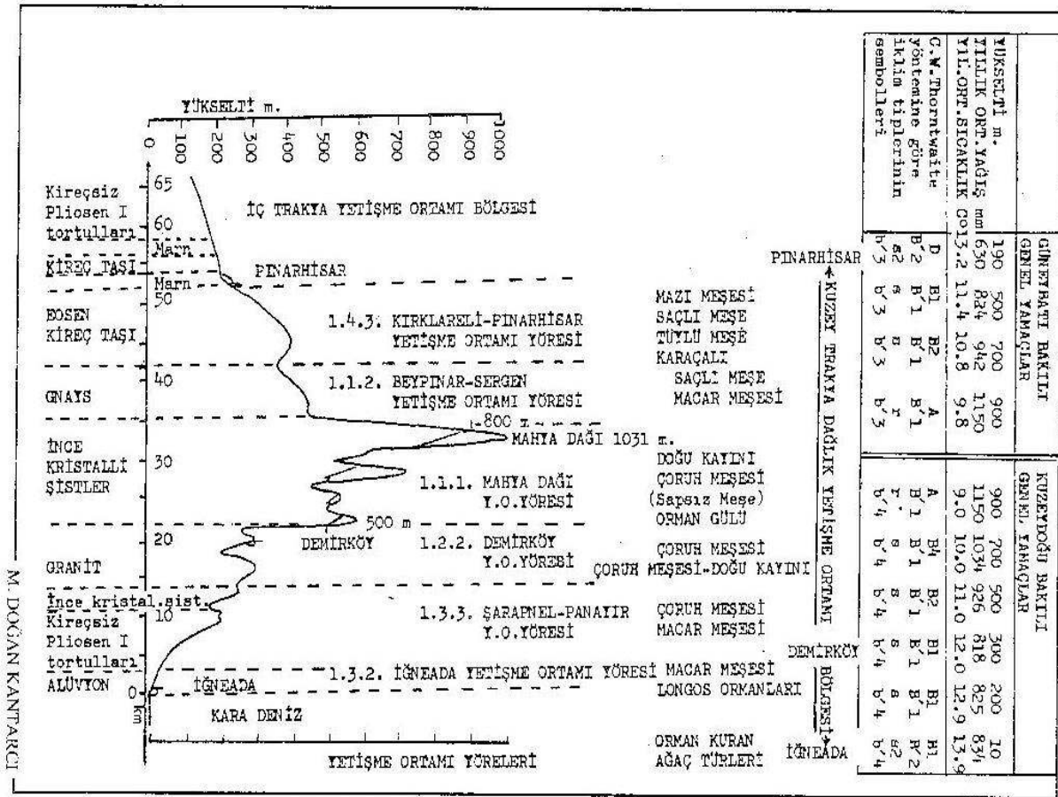
Şekil 4.9 Kuzey Trakya Dağlık yetişme ortamı bölgesinde Pınarhisar-Mahya dağı-İğneada kesitinde anakayalar, yeryüzü şekli, iklim orman kuran ağaç ve çalı türlerinin bulunuşu ve yetişme ortamı yöreleri arasındaki ilişki (Kantarıcı, 2005a).
