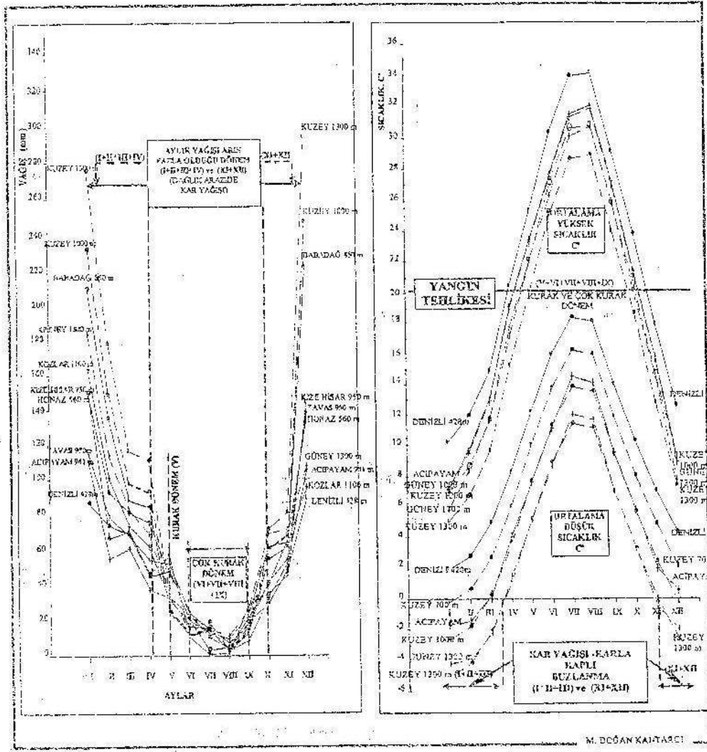
Şekil 4.12 Denizli, Kızılcabölük, Acıpayam arasındaki dağlık arazide ortalama yağış ile ortalama yüksek ve ortalama düşük sıcaklıkların aylık değişimi (Kantarci, 2005a).
