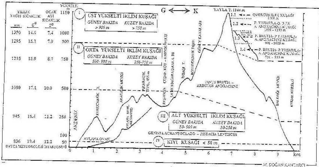
Şekil 4.13 Reşadiye (Datça) Yarımadasında yükselti-iklim kuşakları (Kantarcı, 1990)
