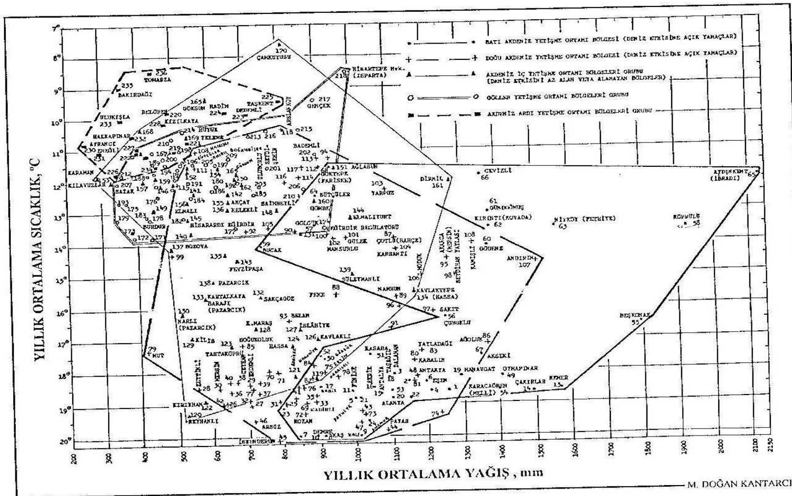
Şekil 4.17 Akdeniz Bölgesi'ndeki Yetiştirme Ortamı BölgeleriGruplarında yıllık ortalama yağış ve sıcaklık ilişkileri (Kantarıcı, 2005a).
