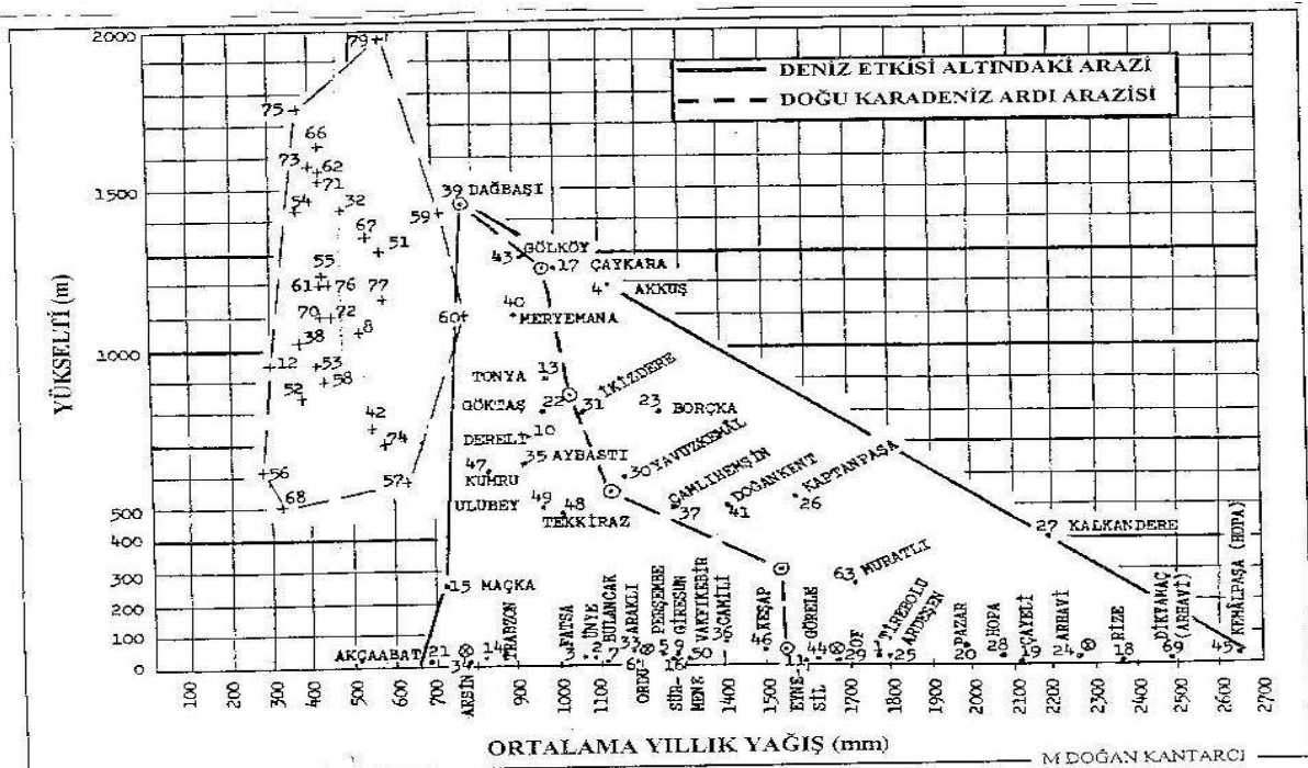
Şekil 4.24 Doğu Karadeniz Bölümünde ortalama yıllık yağış ve sıcaklığın yükseltiye göre değişimi (Kantarcı, 2005a).
