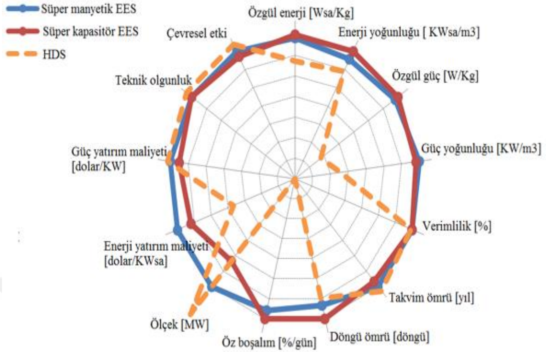
Şekil 2.30. Tablo 2.11.'deki normalleştirilmiş ve logaritmik olarak çizilmiş ortalama verileri kullanarak elektrik enerji depolama sistemlerinin karşılaştırılması. Kesikli çizgi olarak gösterilen HDS, diğer tüm elektrik enerji depolama teknolojileri için karşılaştırma temeli olarak kullanılmıştır. (yeniden düzenlenmiştir (Sabihuddin ve ark., 2014).)
