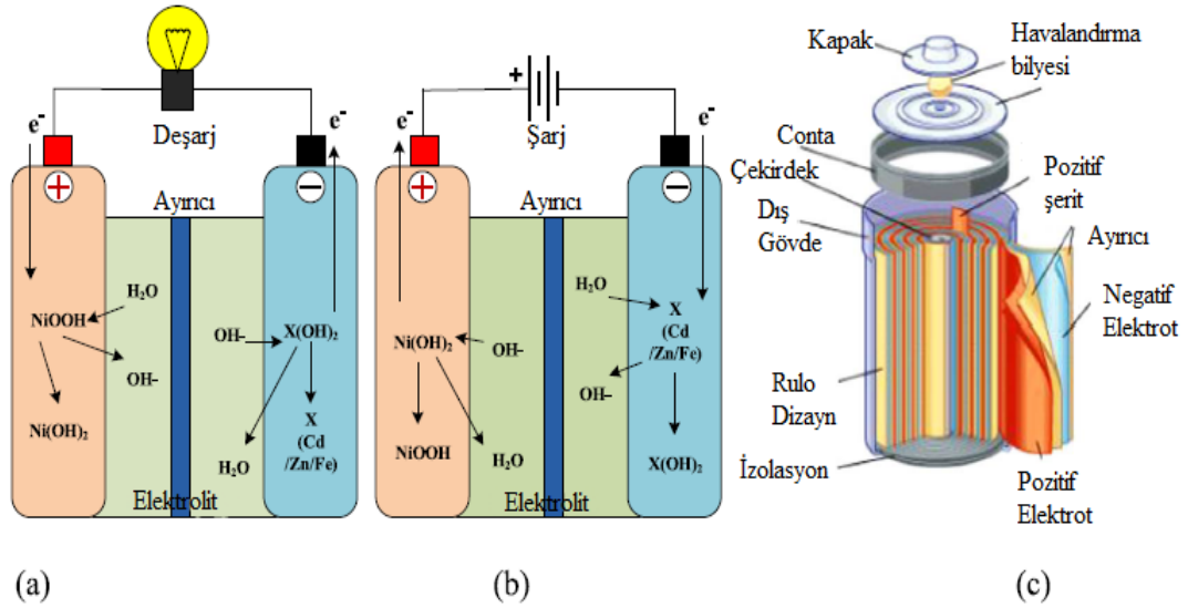
Şekil 2.20. Basit bir Nikel bazlı enerji depolama sistemi hücresinin kimyasal yapısı: a) Şarj esnasında b) Deşarj esnasında ve c) Nikel nazlı pil prototipi (yeniden düzenlenmiştir (Chau ve ark., 1999, Storage, 2011, Hannan ve ark., 2017).)
