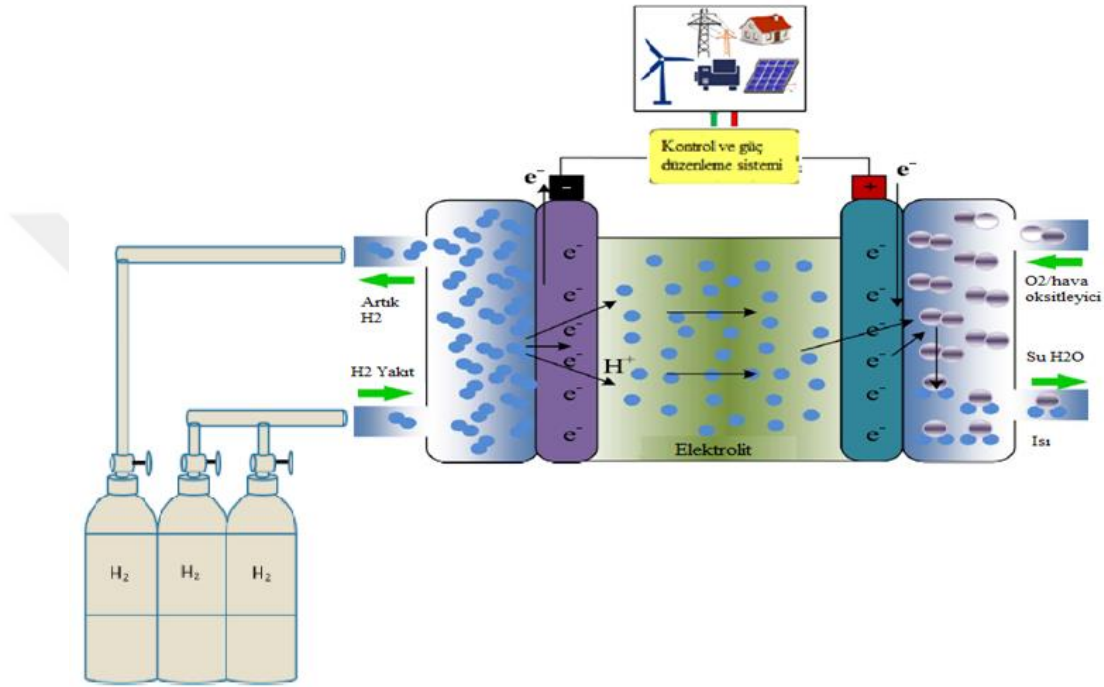
Şekil 2.29. PDMYP enerji destekleme sistemi şeması (yeniden düzenlenmiştir (Nikolaidis ve Poullikkas, 2017, Olabi ve ark., 2020).)
