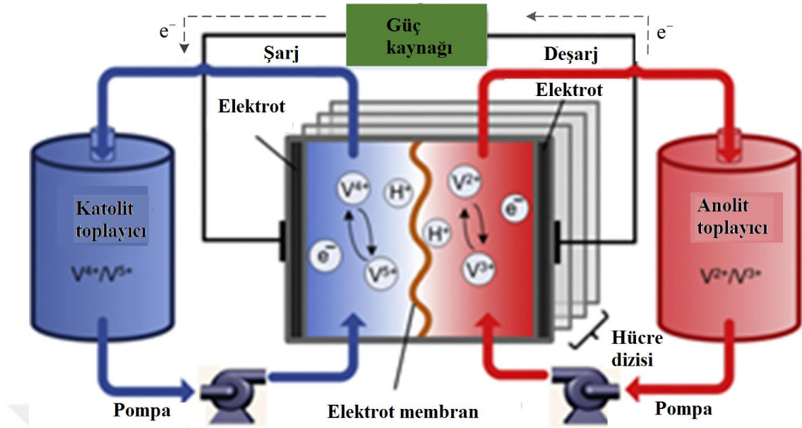
Şekil 2.15. Vanadyum redoks akış pilleri depolama sistemi genel şeması (yeniden düzenlenmiştir (Kaldellis ve Zafirakis, 2007).)
