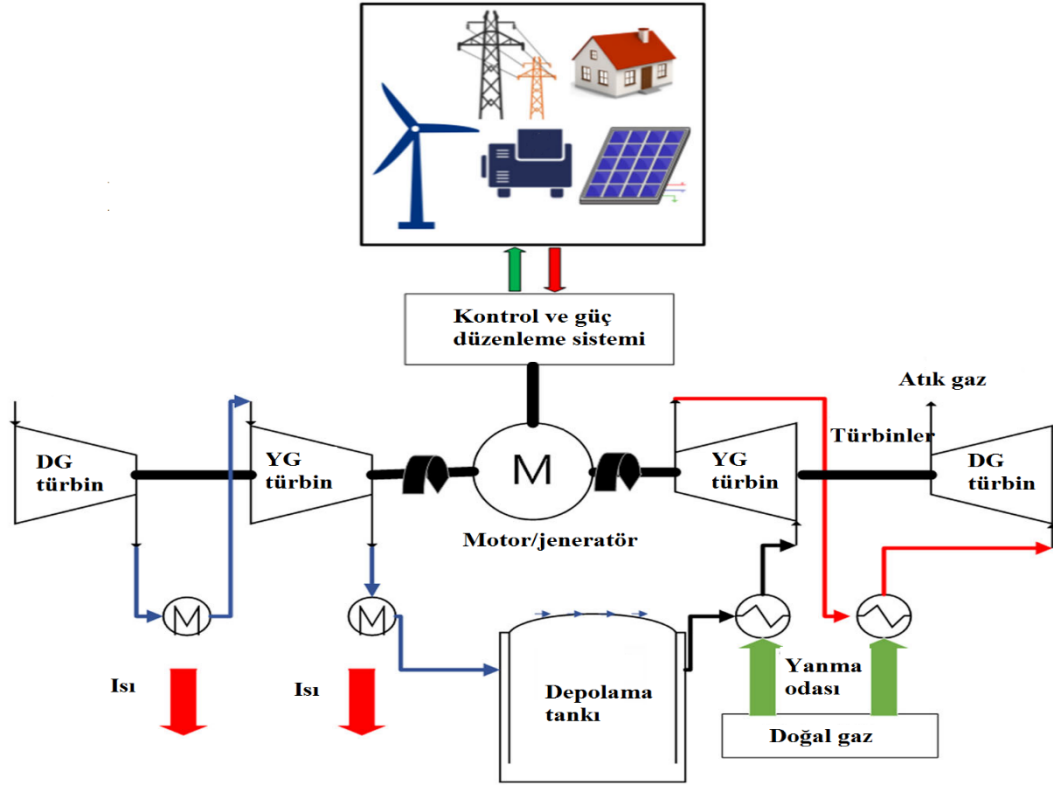
Şekil 2.10. Sıkıştırılmış hava enerji depolama sistemi akış şeması (yeniden düzenlenmiştir (Krishan ve Suhag, 2019).)
