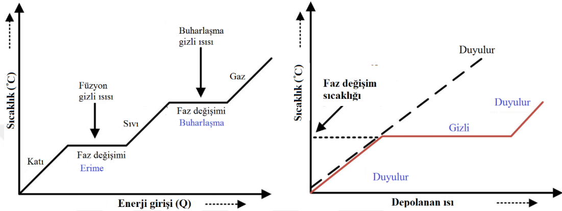
Şekil 2.37. PCM'ler için sıcaklıkla- enerji girişi (solda) ve gizli ve duyulur ısı depolama miktarının sıcaklıkla değişimi (sağda) (yeniden düzenlenmiştir (Mehling ve Cabeza, 2008, Gil ve ark., 2010).)
