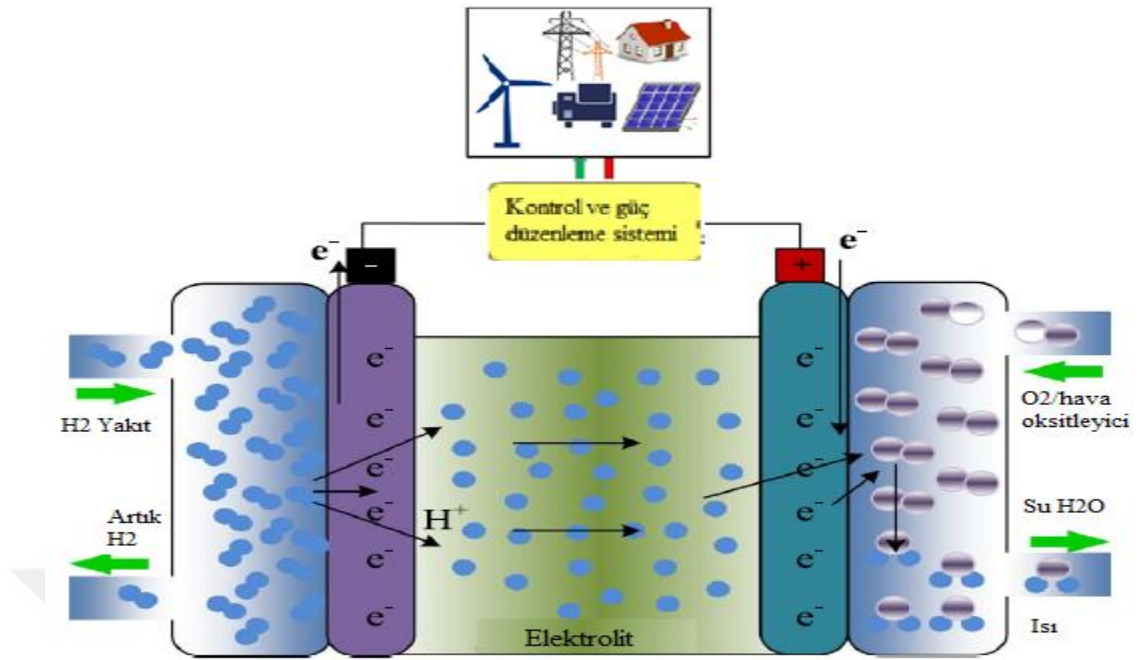
Şekil 2.27. Yakıt pili enerji depolama sisteminin kimyasal tepkimeleri ve yapısı (yeniden düzenlenmiştir (Chau ve ark., 1999, Ibrahim ve ark., 2008, Rashid, 2011, Hannan ve ark., 2017).)
