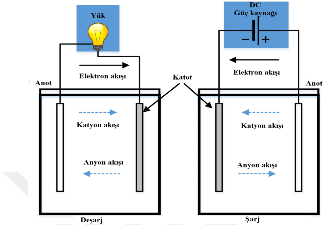
Şekil 2.12. Temel bir elektrokimyasal enerji depolama sisteminin çalışma prensibi (yeniden düzenlenmiştir (Khan ve ark., 2019).)
