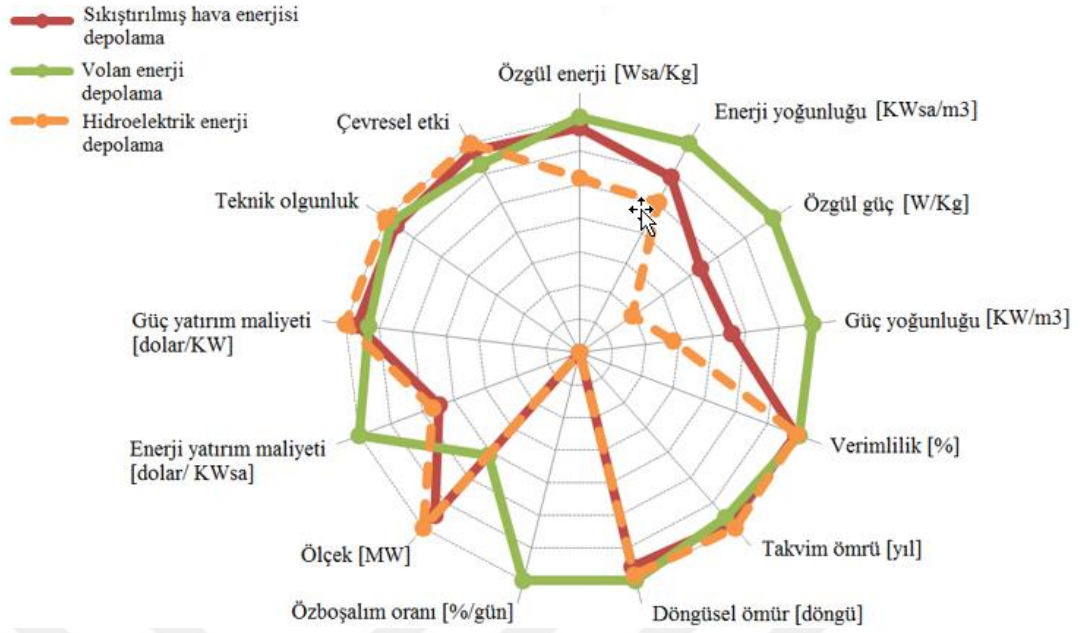
Şekil 2.6. Tablo 2.1.'deki normalleştirilmiş ve logaritmik olarak çizilmiş ortalama verileri kullanarak mekanik enerji depolama sistemlerinin karşılaştırılması. Kesikli çizgi olarak gösterilen HDS, diğer tüm mekanik enerji depolama teknolojileri için karşılaştırma temeli olarak kullanılmıştır (yeniden düzenlenmiştir (Sabihuddin ve ark., 2014) ).
