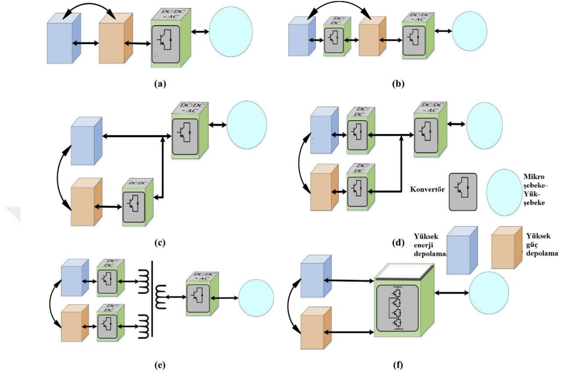
Şekil 2.44. HSS topoloji sınıflandırması (a) pasif topoloji ve (b) yarı-aktif topoloji (c) seri aktif topoloji (d) paralel aktif topoloji (e) izole aktif topoloji (f) çoklu topoloji (yeniden düzenlenmiştir (Hajiaghahi ve ark., 2019).)
