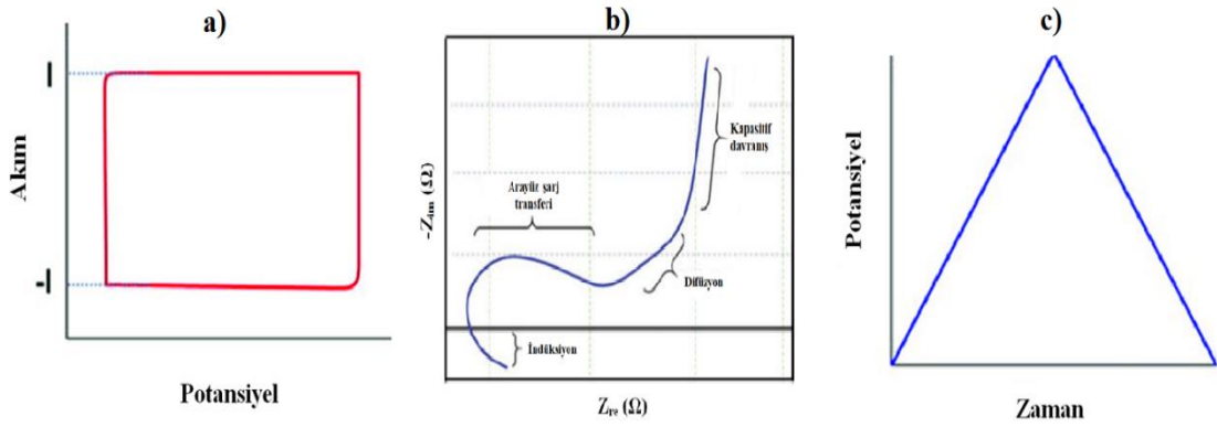
Şekil 2.32. Süper kapasitöre air elektrokimyasal performans eğrileri a) İdeal bir süperkapasitör CV eğrisi b) Şematik EIS eğrisi çizimi ((Bolat Maden, 2020)'ten uyarlanmıştır.) ((Azman ve ark., 2018)'ten uyarlanmıştır.) c) İdeal bir süperkapasitör GCD eğrisi ((Azman ve ark., 2018)'ten uyarlanmıştır.)
