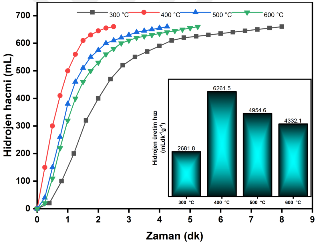
Şekil 3.13. Farklı yanma sıcaklıkları için HPR'nin zamanın bir fonksiyonu olarak değişimi (Reaksiyon Koşulları: %2,5 \text{NaBH}_4 , katalizör = 0,1 g, T = 30 °C, V_{\text{metanol}} = 10 mL).
