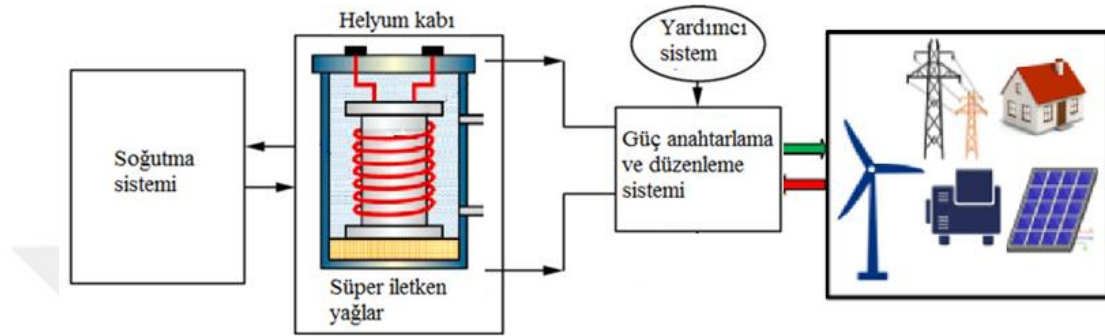
Şekil 2.33. Basit bir süper iletken manyetik enerji depolama sistemi şeması (yeniden düzenlenmiştir (Chen ve ark., 2009).)
