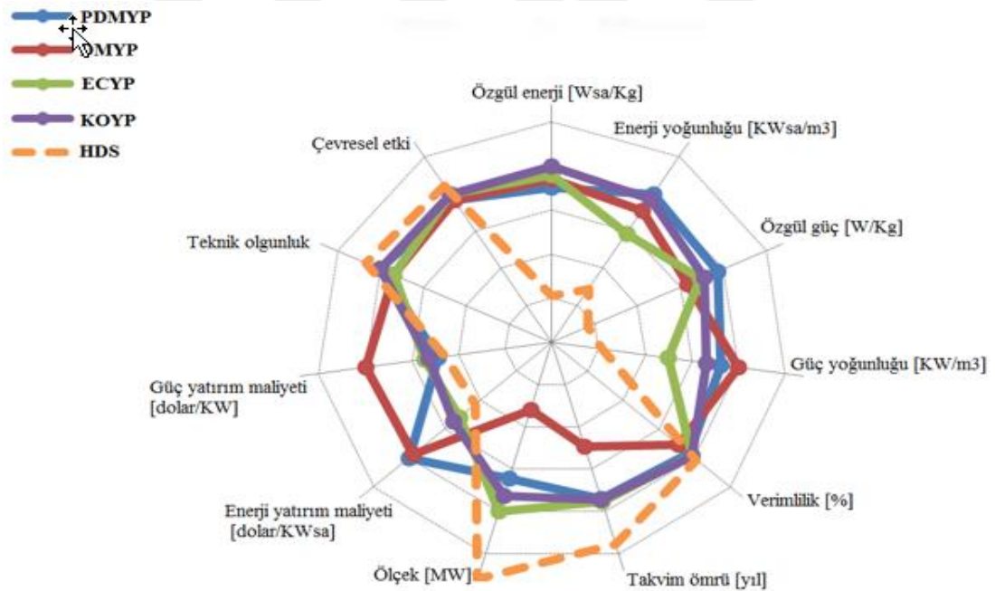
Şekil 2.26. Tablo 2.10.'daki normleştirilmiş ve logaritmik olarak çizilmiş ortalama verileri kullanarak YP pillerdeki kimyasal enerji depolama sistemlerinin karşılaştırılması. Kesikli çizgi olarak gösterilen HDS, diğer tüm yakıt pilleri enerji depolama teknolojileri için karşılaştırma temeli olarak kullanılmıştır. (yeniden düzenlenmiştir (Sabihuddin ve ark., 2014).)
