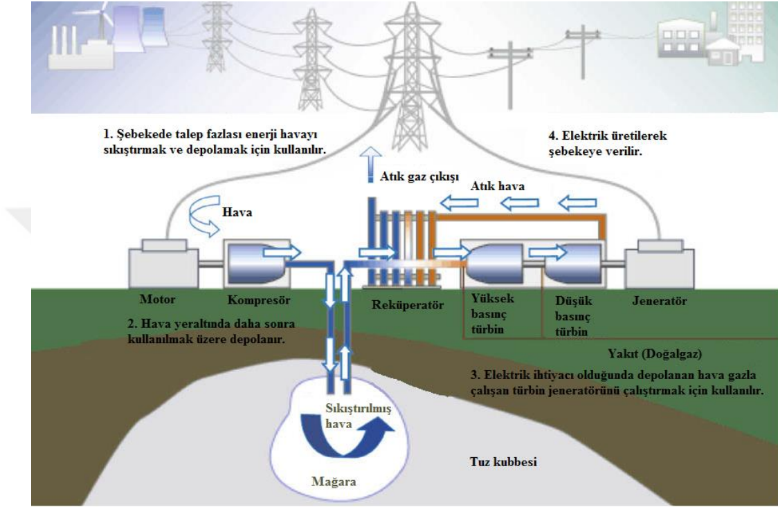
Şekil 2.9. Sıkıştırılmış hava enerji depolama sistemi (yeniden düzenlenmiştir (Mcdowall, 2004).)
