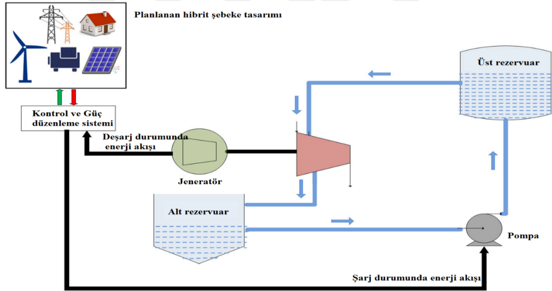
Şekil 2.8. Kapalı döngü HDS genel akış şeması (yeniden düzenlenmiştir (Krishan ve Suhag, 2019).)
