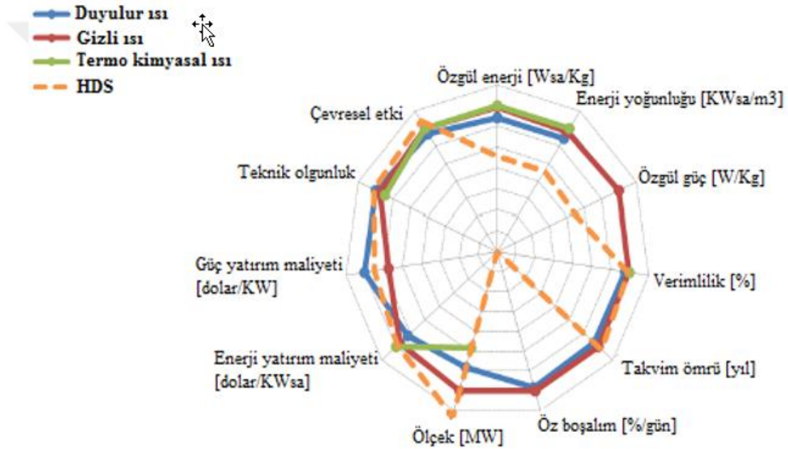
Şekil 2.36. Tablo 2.15.'deki normalleştirilmiş ve logaritmik olarak çizilmiş ortalama verileri kullanarak TEDS'lerin karşılaştırılması. Kesikli çizgi olarak gösterilen HDS, diğer tüm elektrik enerji depolama teknolojileri için karşılaştırma temeli olarak kullanılmıştır (yeniden düzenlenmiştir (Sabihuddin ve ark., 2015)).
