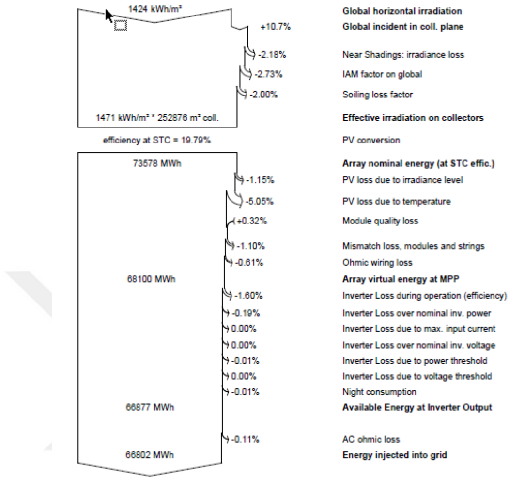
Şekil 4.8. Hidro-solar GES'e ait benzetim sonucunda elde edilen enerji akış ve kayıp diyagramı.
