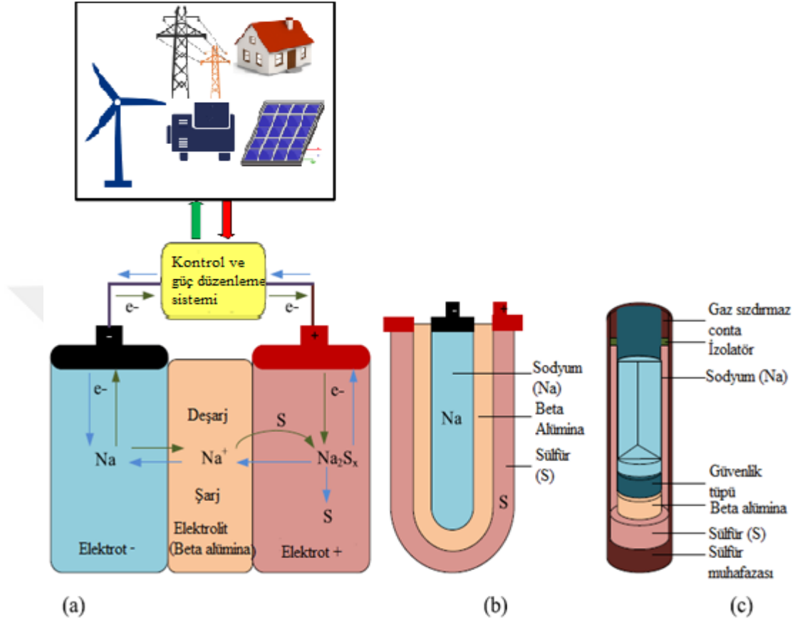
Şekil 2.23. Basit bir Sodyum sülfür enerji depolama sistemi hücresinin kimyasal yapısı a) Şarj/deşarj esnasında b) Na-S teknoloji depolama sisteminin boru tipi tasarımı c) Na-S enerji depolama sistemi prototipi (yeniden düzenlenmiştir (Storage, 2011, Vazquez ve ark., 2010, Chen ve ark., 2009, Hannan ve ark., 2017, Akhil ve ark., 2013)
