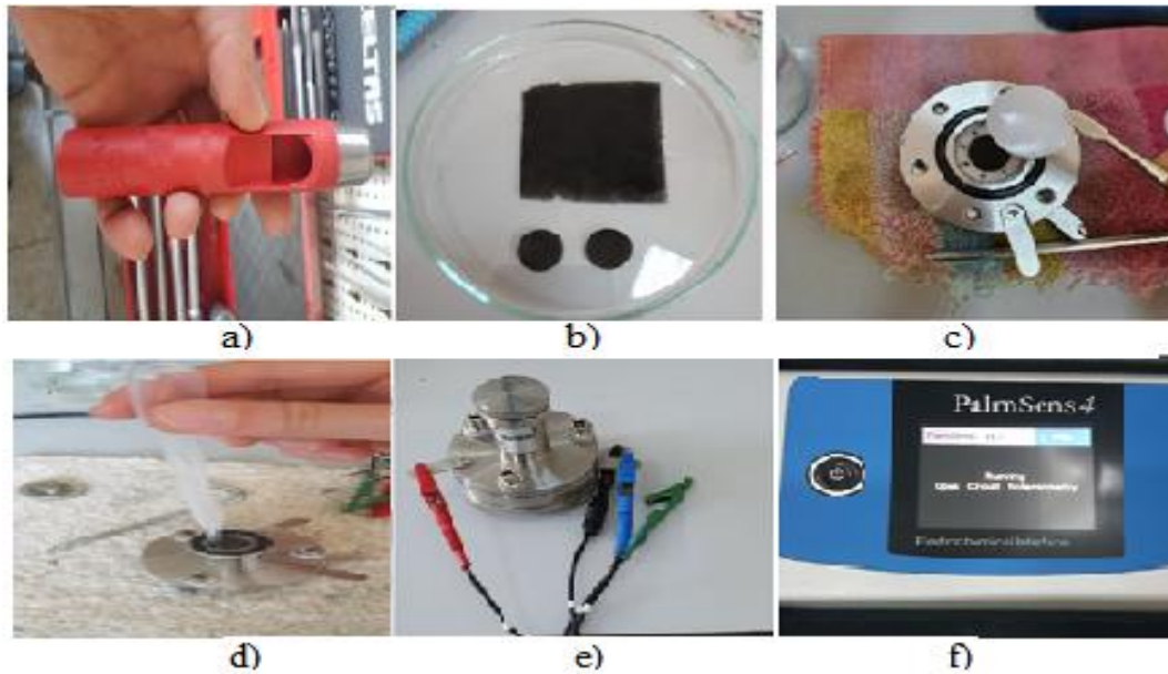
Şekil 3.6. a,b) Elektrotların oluşturulması, c) Elektrotların test hücreğine yerleştirilmesi, d) Elektrotlara elektrolit sıvısı uygulanması, d) Alüminyum kapasitör test hücresi bağlantıları, e) Test hücresi yazılım ara yüzü.
