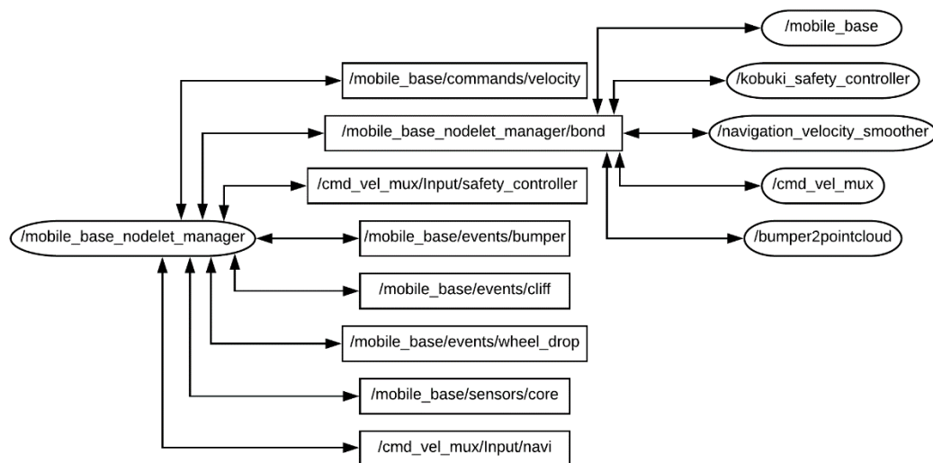
Şekil 4.7. Navigasyon esnasında kullanılan düğümler ve aralarındaki ilişki
