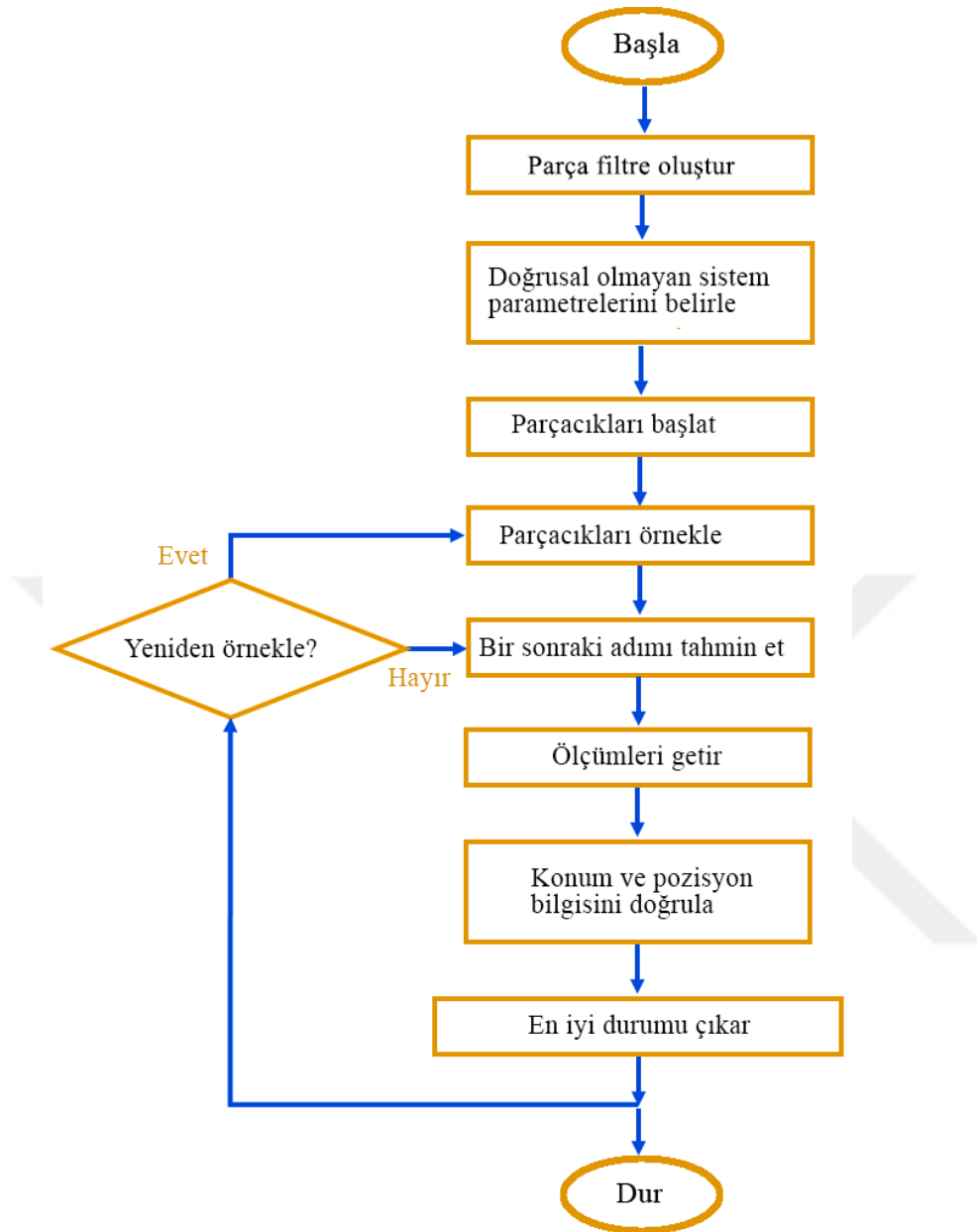
Şekil 3.5. Parçacık filtresi akış diyagramı
