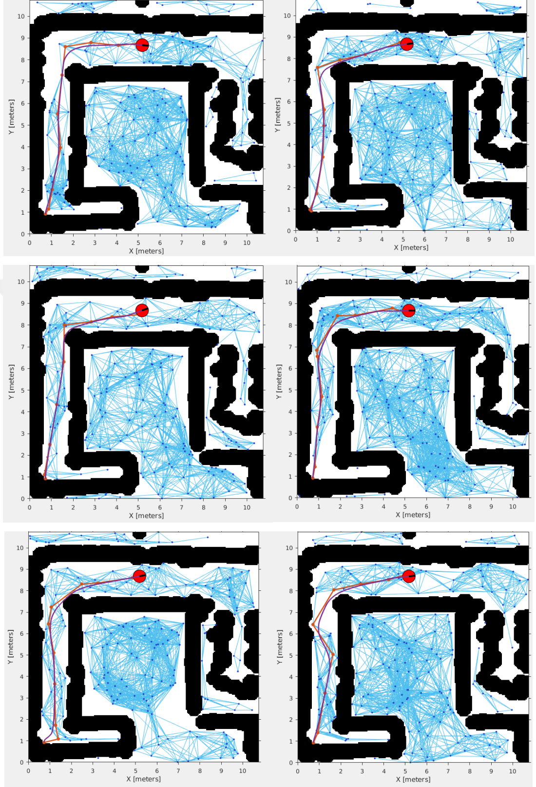
Şekil 5.19. PRM testlerine ait 6 ayrı deney sonucu
