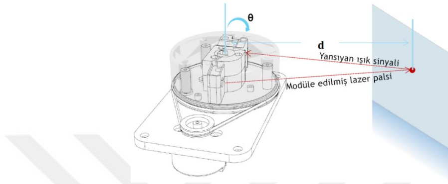
Şekil 3.3. SLAM için kullanılan 2D LIDAR [41]
