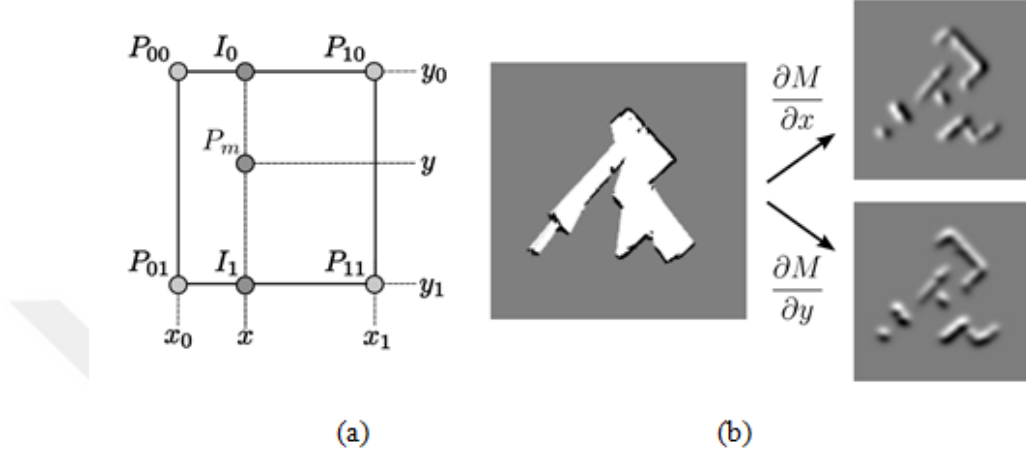
Şekil 3.4. (a) Doluluk kafesi haritasının bi-lineer filtrelenmesi. ( P_m noktası enterpolasyonlu olan noktadır) (b) Doluluk kafesi ile haritalama ve mekansal türevleri [43]
