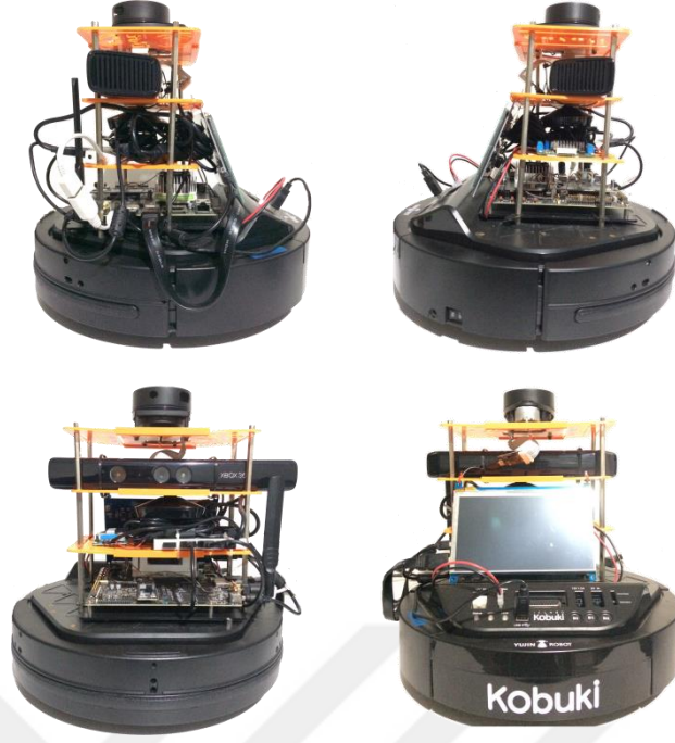
Şekil 5.1. Mobil robotun sağ, sol, ön ve arka görüşleri
