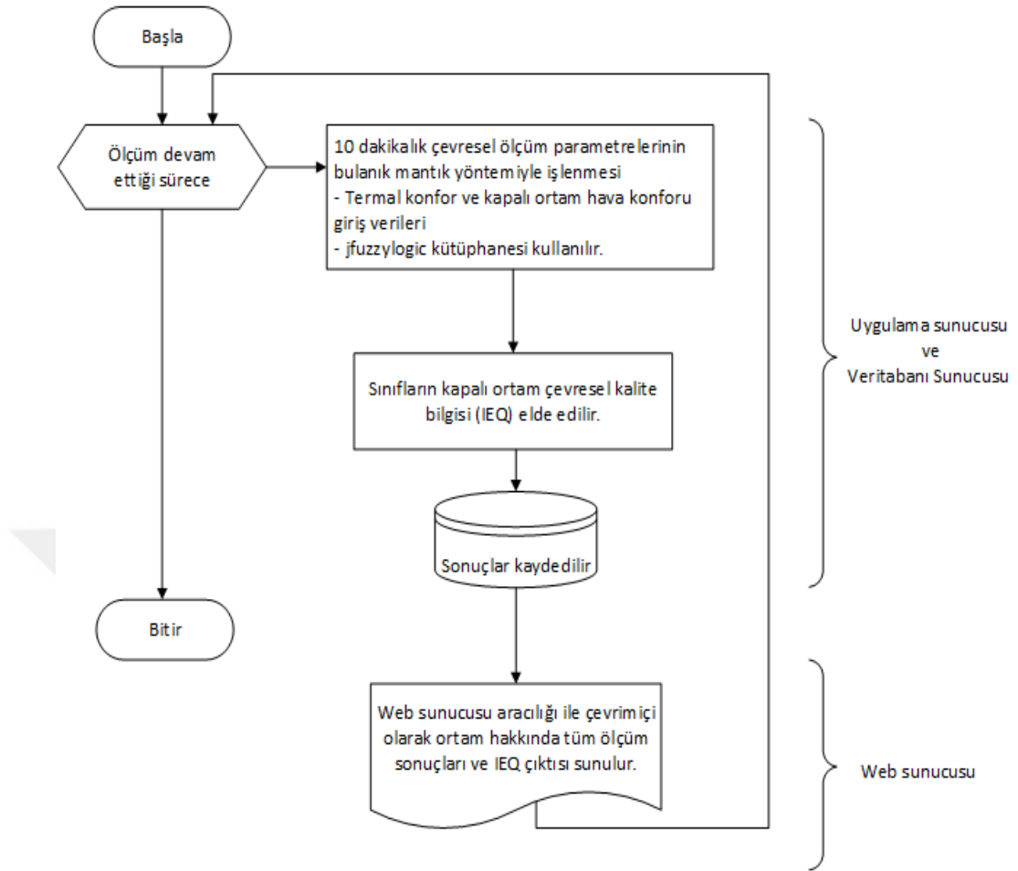
Şekil 3.19. Sistemin işleyişi akış diyagramı (Veri işleme ve ölçüm sisteminin çıktısı)
