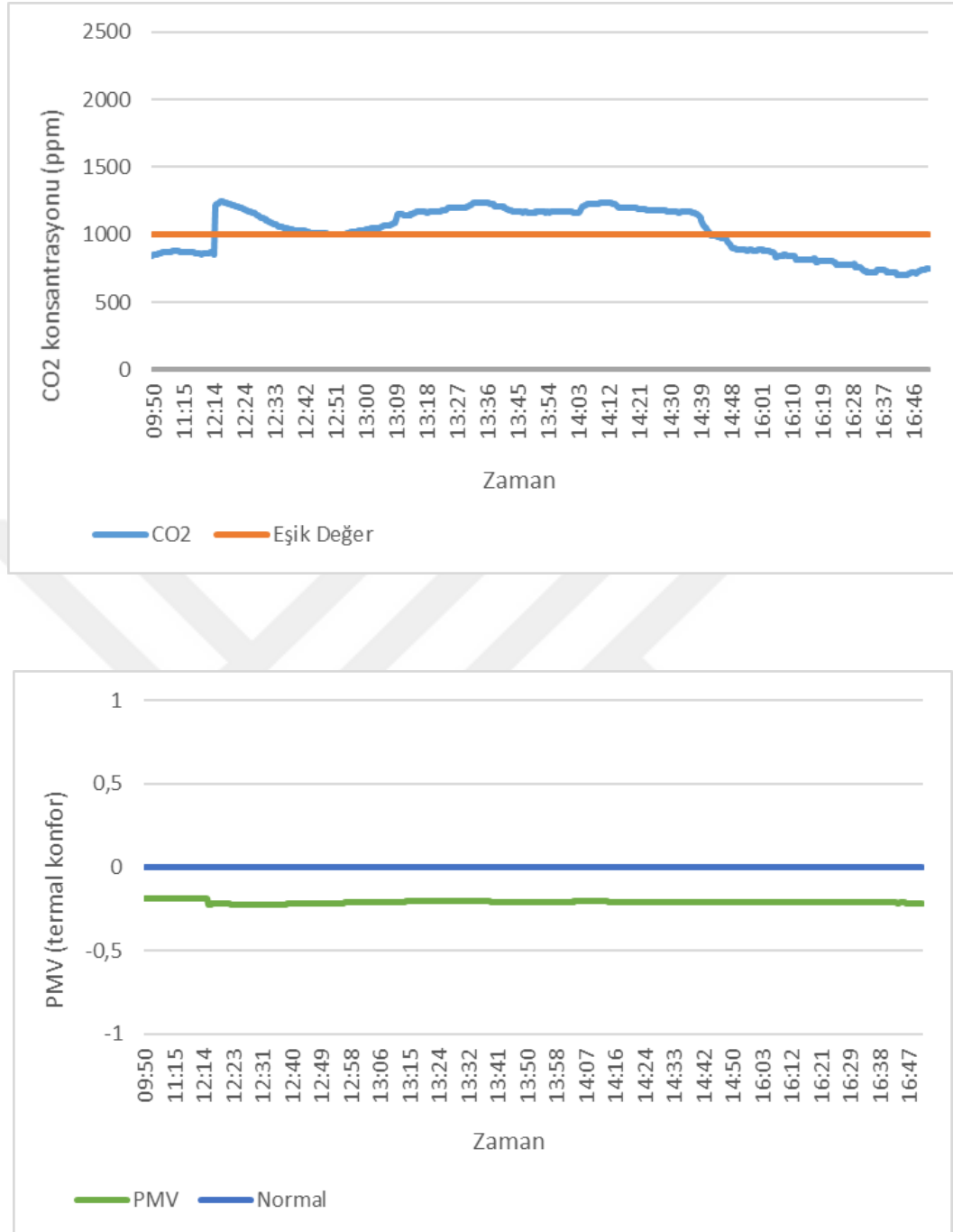
Şekil 4.4. C1105 nolu sınıfa ait bir günlük ölçüm verileri (zamana bağlı CO 2 konsantrasyonu (ppm) ve PMV (termal konfor))
