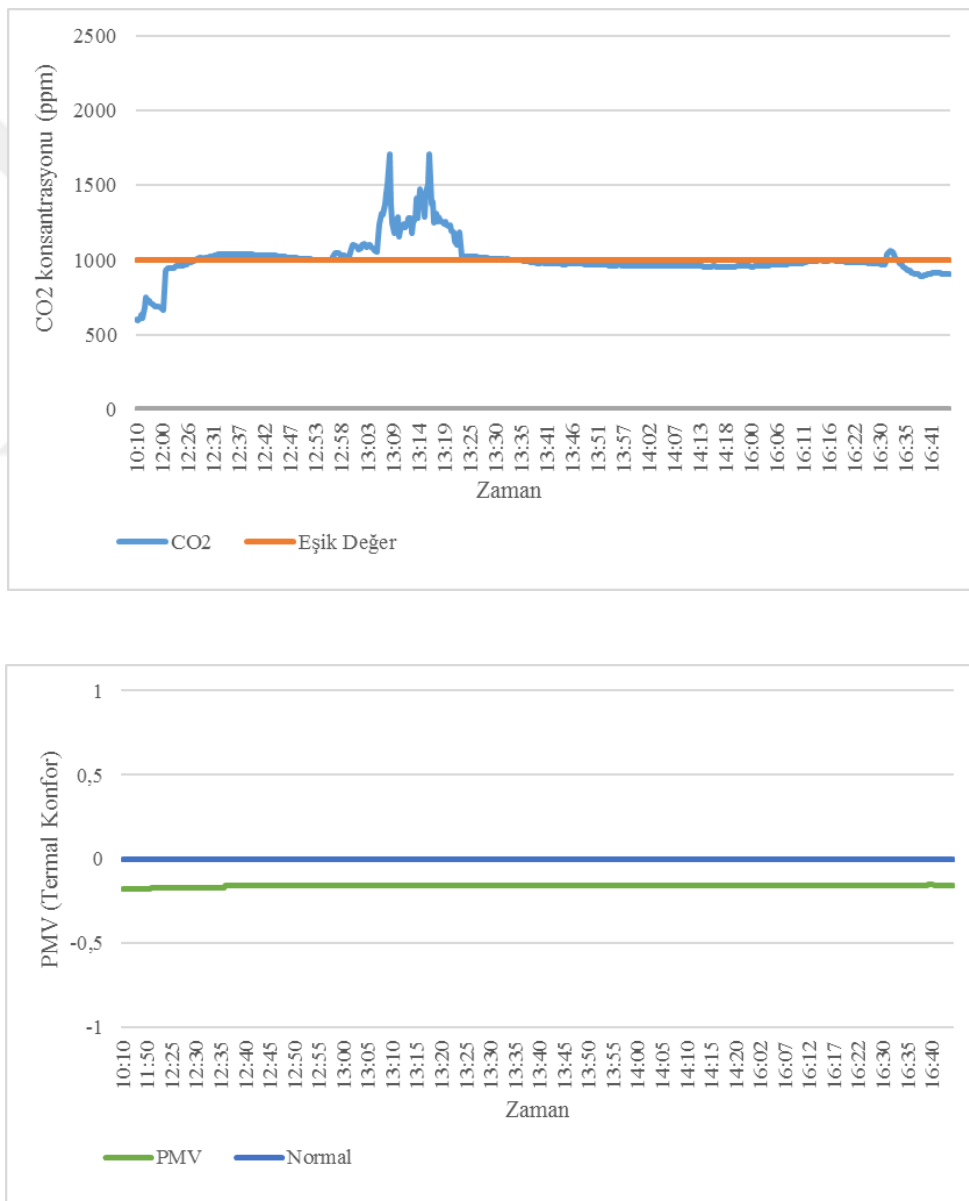
Şekil 4.3. C1104 nolu sınıfa ait bir günlük ölçüm verileri (zamana bağlı CO 2 konsantrasyonu (ppm) ve PMV (termal konfor))
