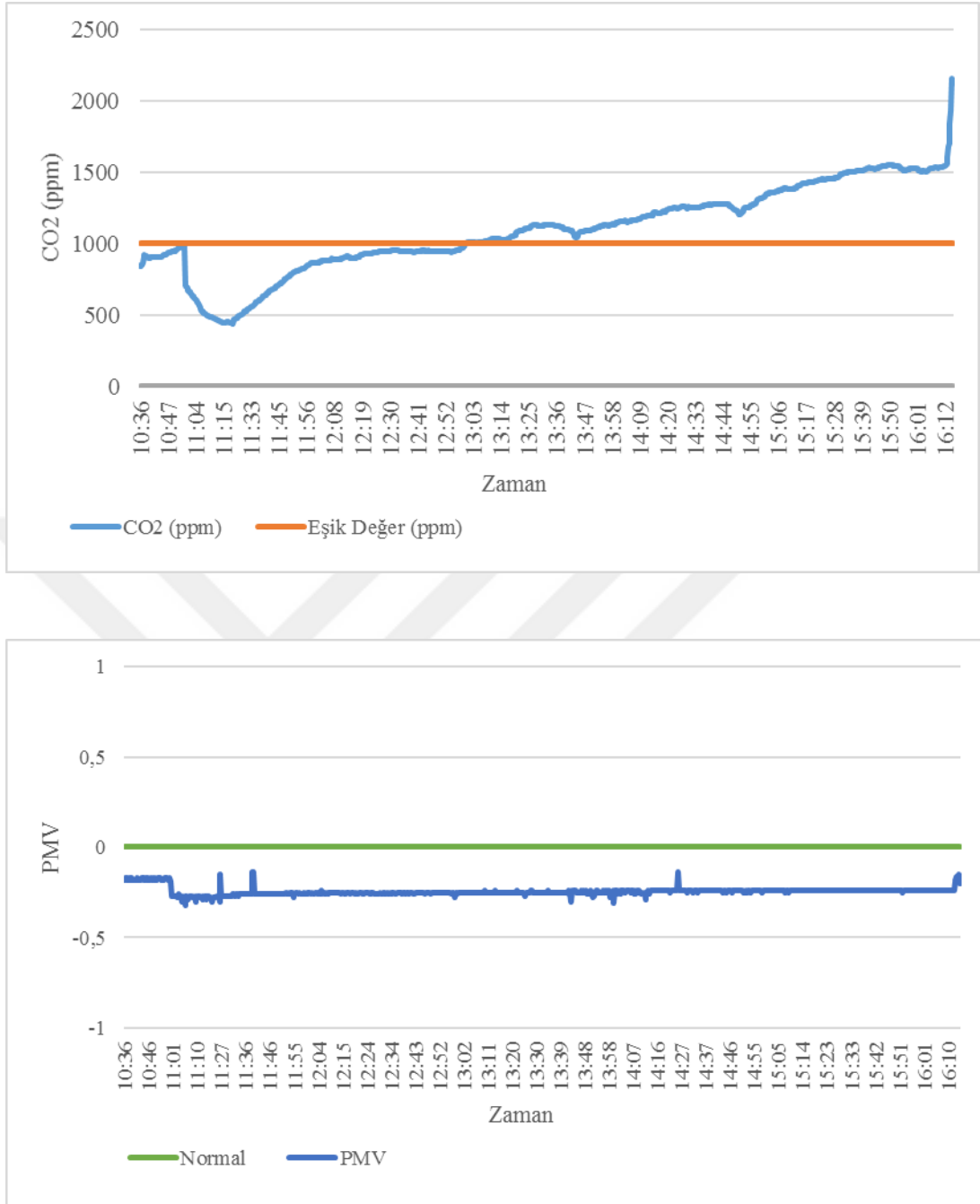
Şekil 4.5. C1106 nolu sınıfa ait bir günlük ölçüm verileri (zamana bağlı CO 2 konsantrasyonu (ppm) ve PMV (termal konfor))
