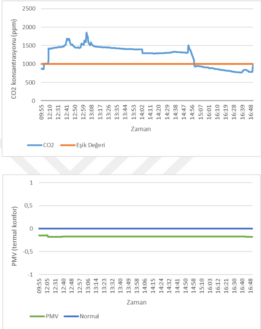
Şekil 4.6. C1107 nolu sınıfa ait bir günlük ölçüm verileri (zamana bağlı CO 2 konsantrasyonu (ppm) ve PMV (termal konfor))
