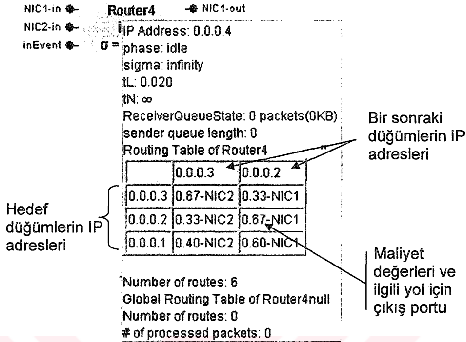
Şekil 5.9 Bir yönlendirme tablosunun DEVJAVA altında ekran görüntüsü.
