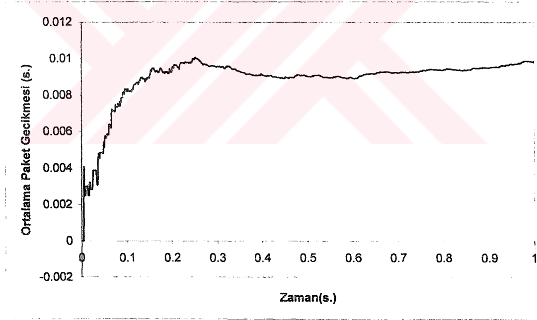
Şekil 6.5 Ortalama paket gecikmesi
