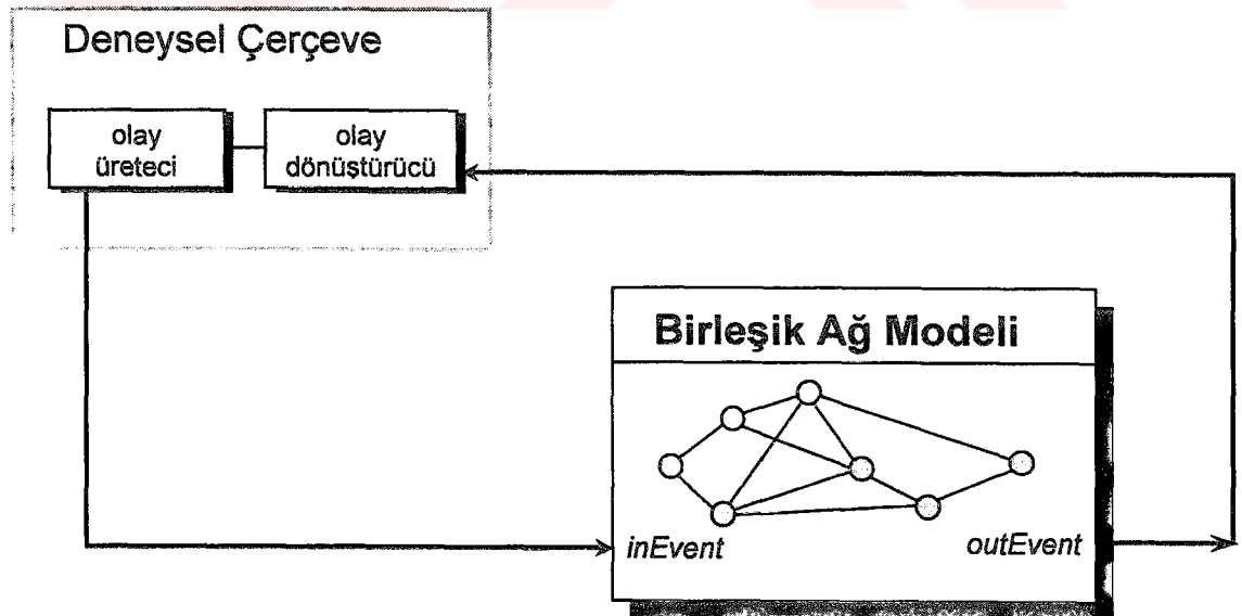
Şekil 5.10 Deneysel çerçeve.
