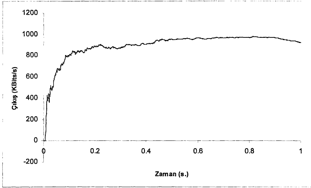
Şekil 6.4 Ağ içerisinde oluşan trafik çıkışı
