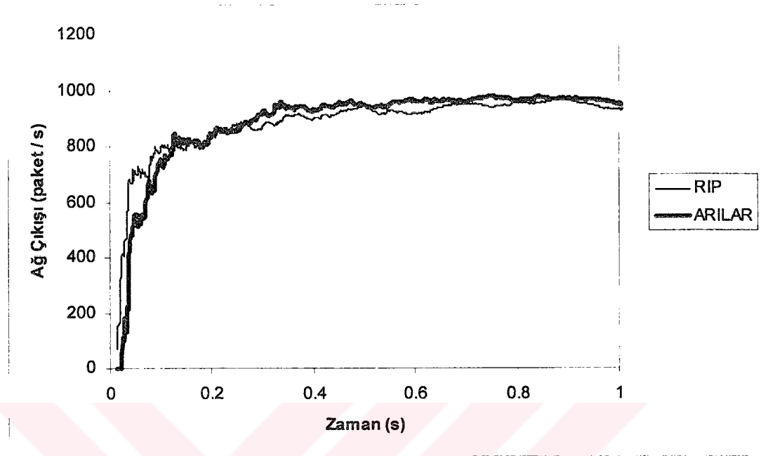
Şekil 6.9 RIP ve Arılarla gerçekleştirilen algoritmalarının ağ çıkış değerlerinin karşılaştırılması.
