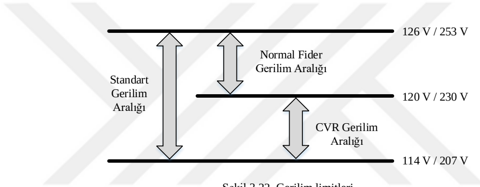
Şekil 3.22. Gerilim limitleri
