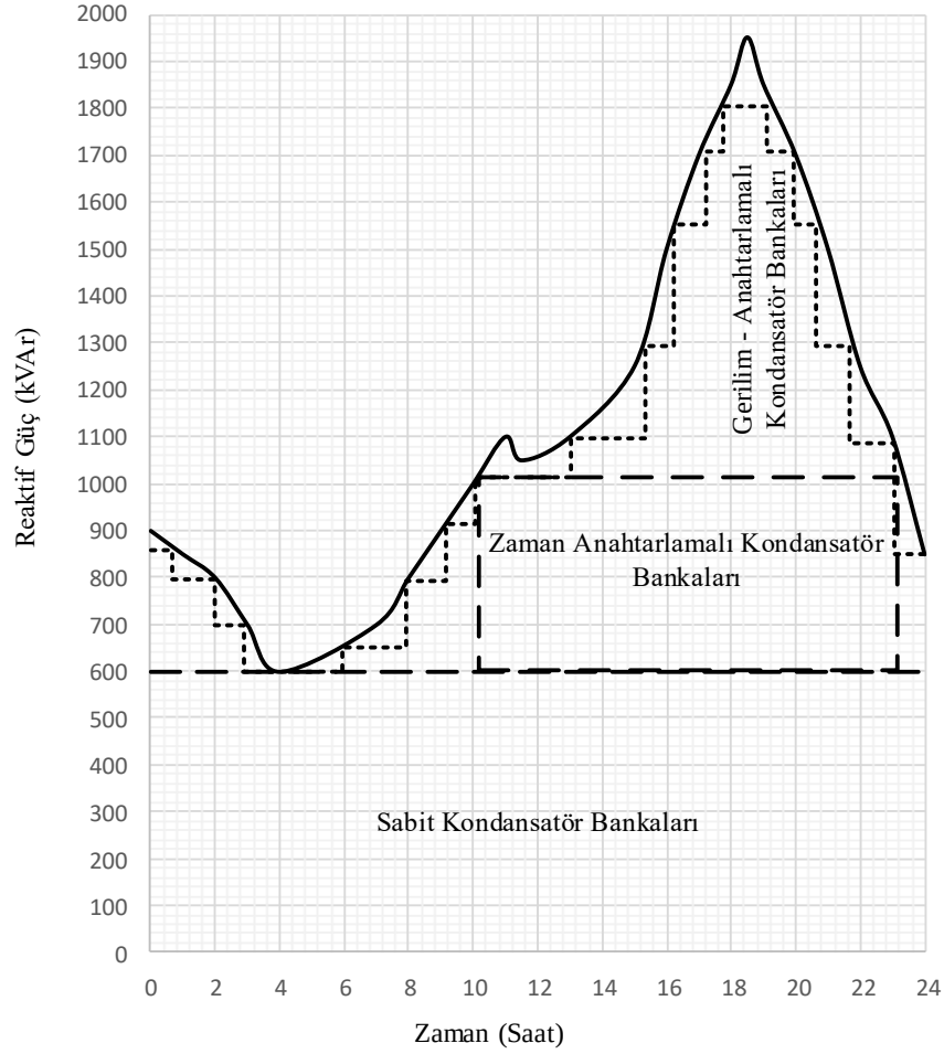
Şekil 3.16. Anahtarlama kondansatör kontrolü [88].
