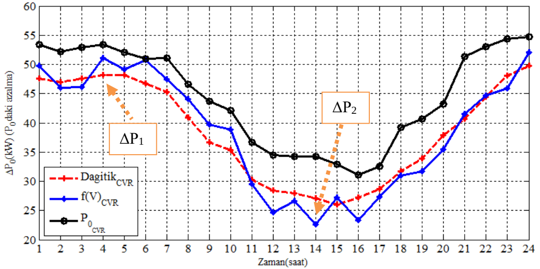
Şekil 6.36. Tüm CVR durumlarının geleneksel duruma göre oluşan dağıtım trafo merkezinden çekilen güçteki ( P_0 ) azalma (PV'siz sistem)
