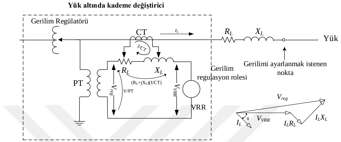
Şekil 3.10. Gerilim Düşüm Kompanzatör (LDC) devresi [81].
