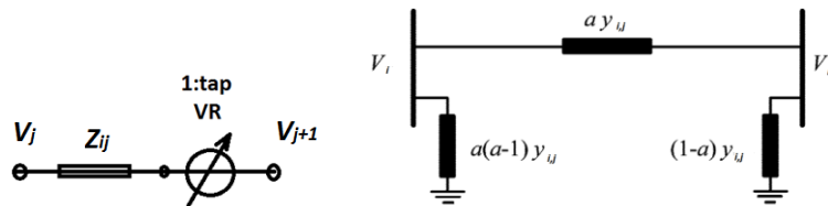
Şekil 3.11. VR tek hat şeması ve pi eş değer devresi [89].
