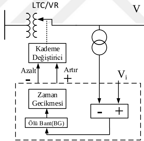
Şekil 3.9. VR kontrol algoritması ve şeması
