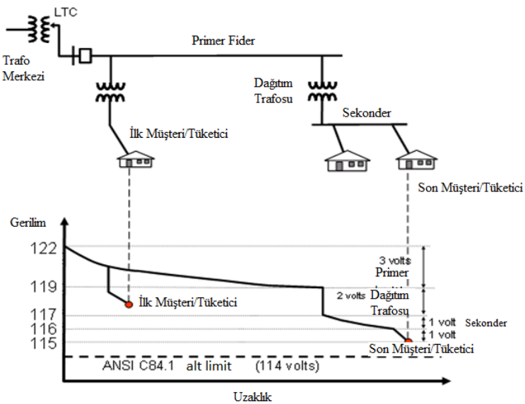
Şekil 3.1. Dağıtım şebekesinde gerilim limitleri [82].
