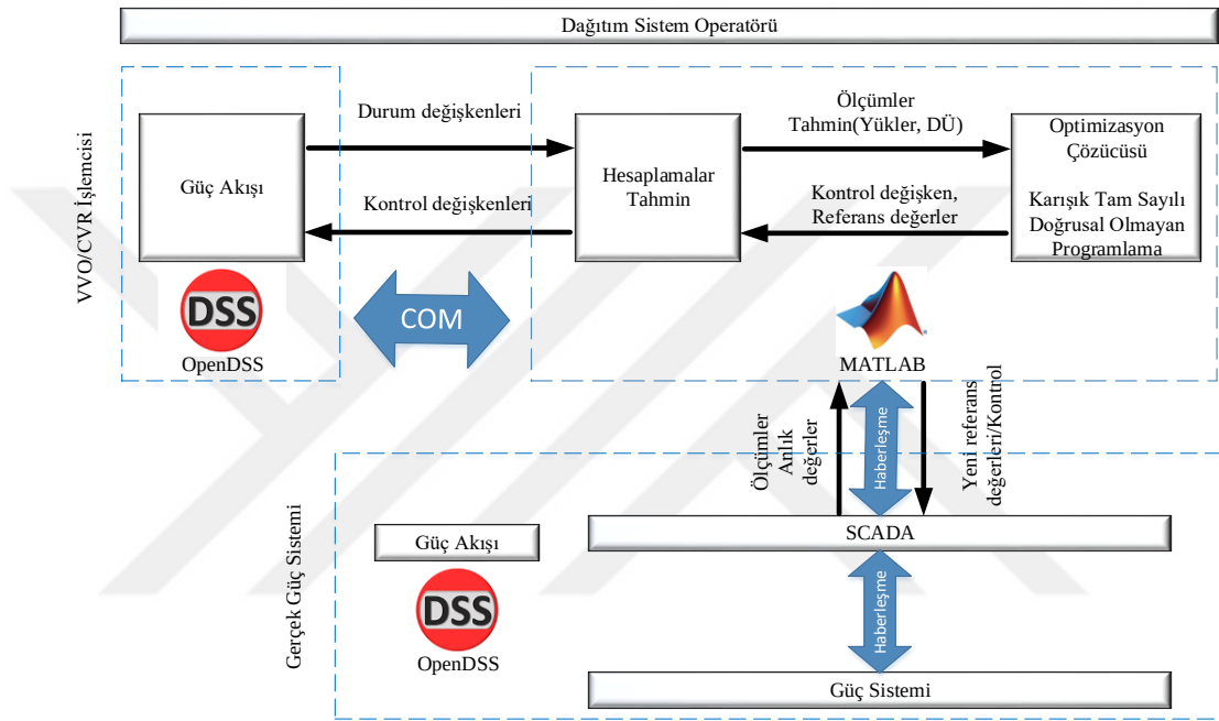
Şekil 6.15. OpenDSS ve MATLAB ile algoritmanın benzetimi
