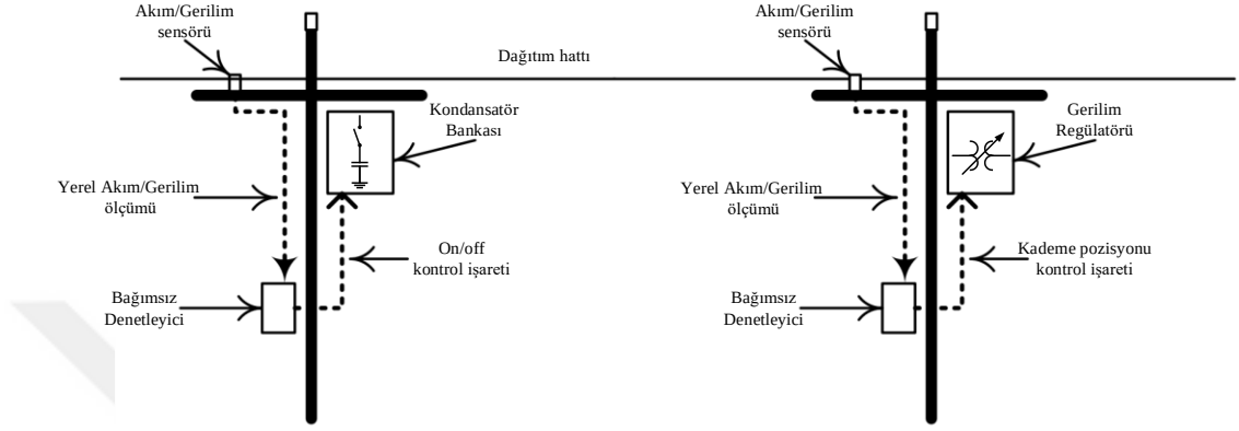
Şekil 3.25. Bağımsız Volt/VAr denetleyici yaklaşımı [9].
