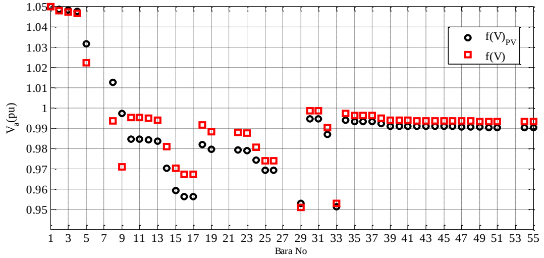
Şekil 6.39. PV içeren ve içermeyen modifiye edilmiş IEEE 34 baralı test sistemine merkezi/birleşik f(V) amaçlı VVO/CVR uygulanması durumunda a fazı bara gerilimleri (Saat 13.00)
