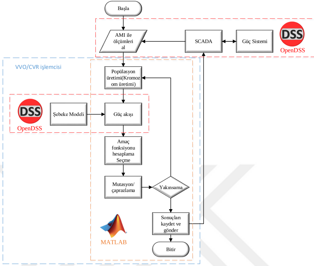
Şekil 6.17. Önerilen VVO/CVR probleminin GA ile çözülmesi
