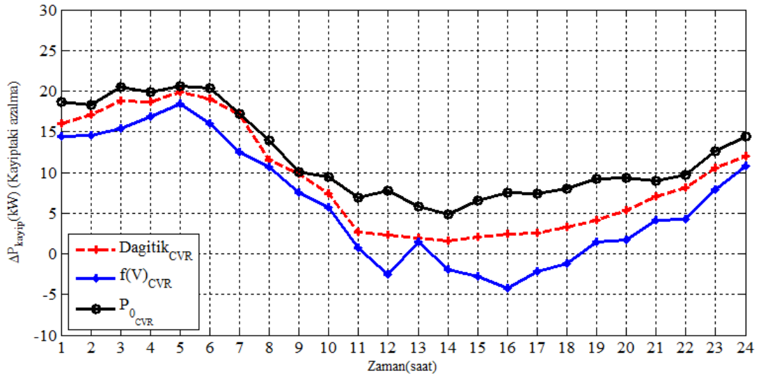
Şekil 6.37. Tümü CVR durumlarının geleneksel duruma göre oluşan kayıptaki azalma (PV'li sistem)
