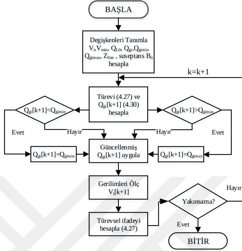
Şekil 4.1. Dağıtık reaktif güç kontrol tabanlı güç kaybı minimizasyonu
