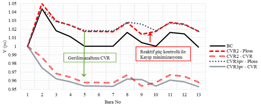
Şekil 6.7. Tüm baralardaki c fazının gerilimleri (Saat 18.00)
