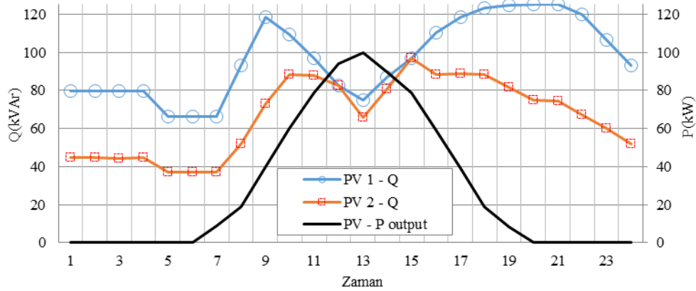
Şekil 6.9. CVR3pv durumu için PV eviricilerinin aktif ve reaktif güç çıkışı
