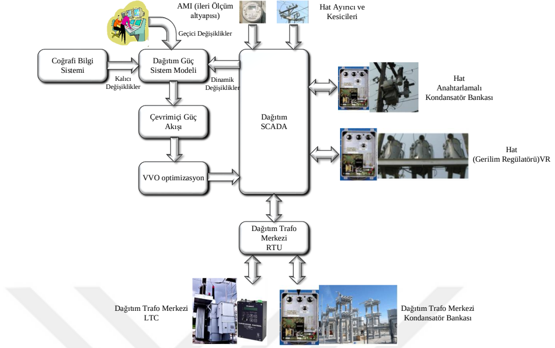
Şekil 3.27. Model odaklı VVO [9].
