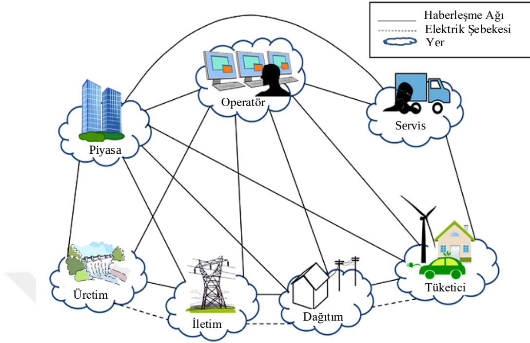
Şekil 2.1. NIST tarafından önerilen akıllı şebeke modeli [68].
