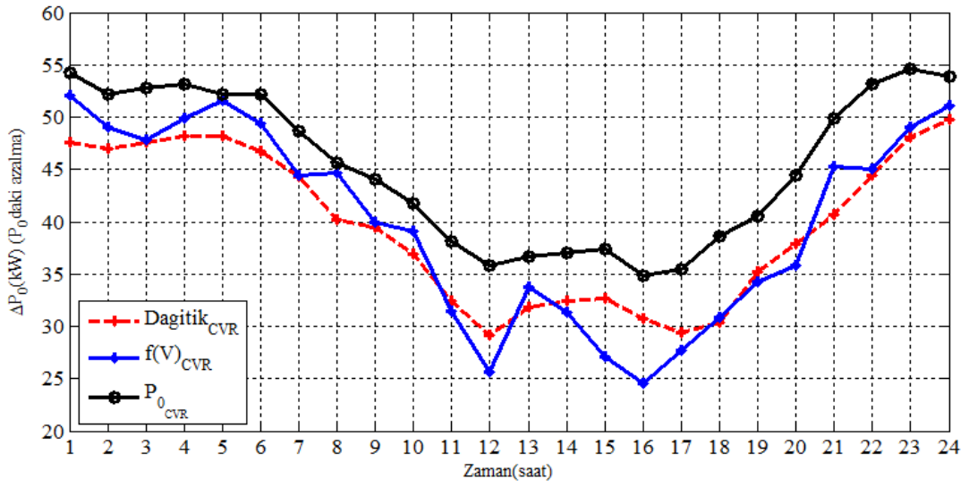
Şekil 6.35. Tüm CVR durumlarının geleneksel duruma göre oluşan dağıtım trafo merkezinden çekilen güçteki ( P_0 ) azalma (PV'li sistem)
