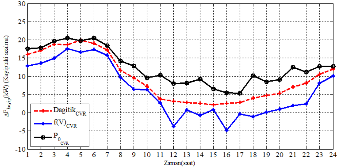
Şekil 6.38. Tümü CVR durumlarının geleneksel duruma göre oluşan kayıptaki azalma (PV'siz sistem)
