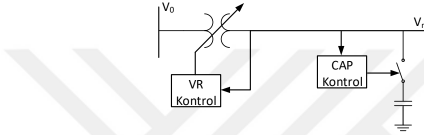
Şekil 3.3. Dağıtım fideri üzerinde kullanılan gerilim regülatörü ve kondansatör bankası
