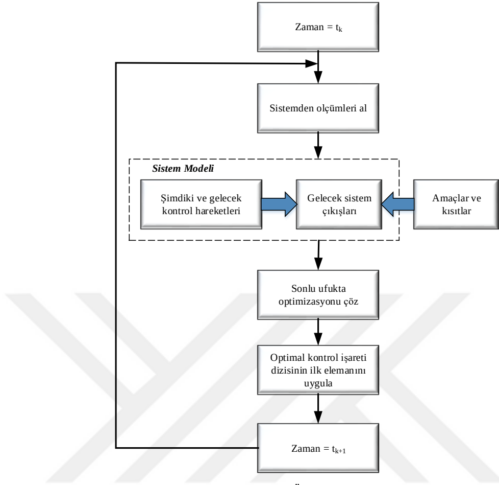
Şekil 5.3. MÖK algoritması
