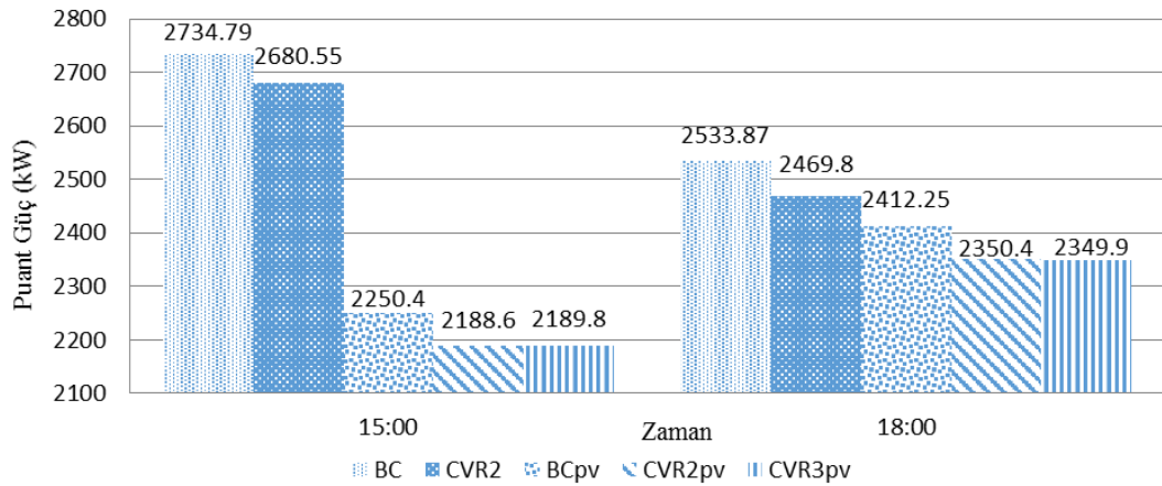
Şekil 6.5. Puant güç
