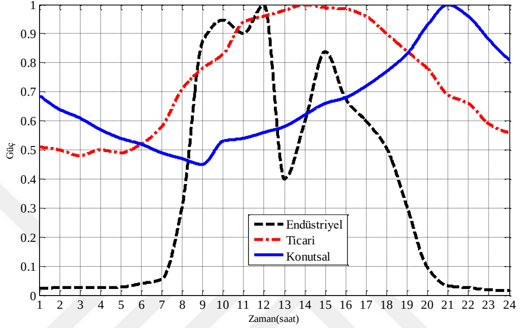
Şekil 6.2. Endüstriyel, ticari ve konutsal tüketiciye ait günlük yük eğrisi
