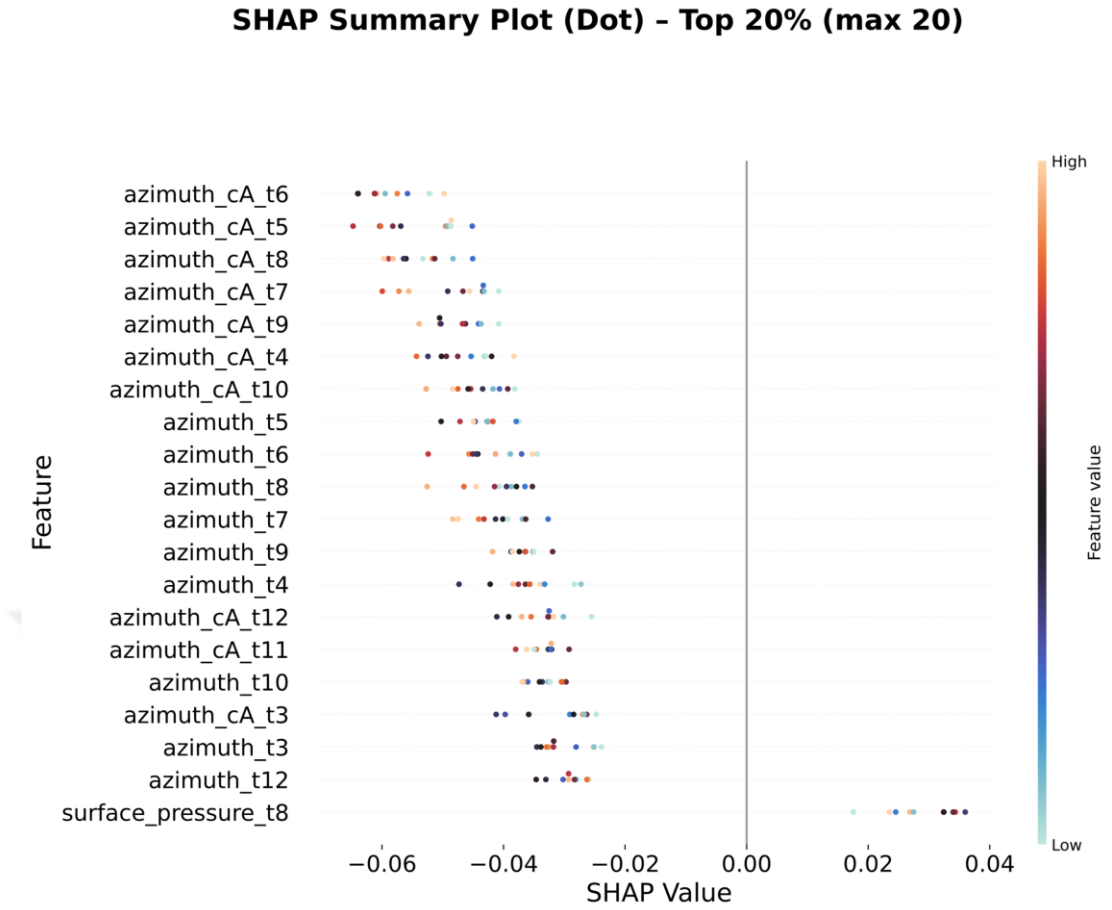
Şekil 4.8. SHAP tabanlı analizle belirlenen en etkili özniteliklerin görselleştirilmesi (En etkili yüksek %80'lik dilim)
