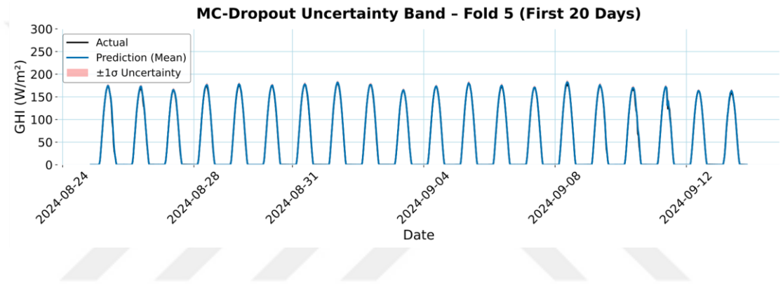
Şekil 4.6. MC Dropout ile elde edilen \pm 1\sigma belirsizlik bandı ve tahmin güvenilirliği
