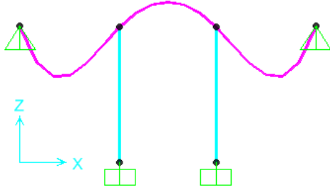
Şekil 4.100 Kirişte kaplama ve kar yükü altında şekil değiştirme.
