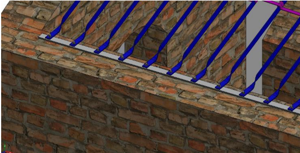
Şekil 4.123 14 numaralı yapıda merteklerin duvar üzerinde birleşim önerisi.
