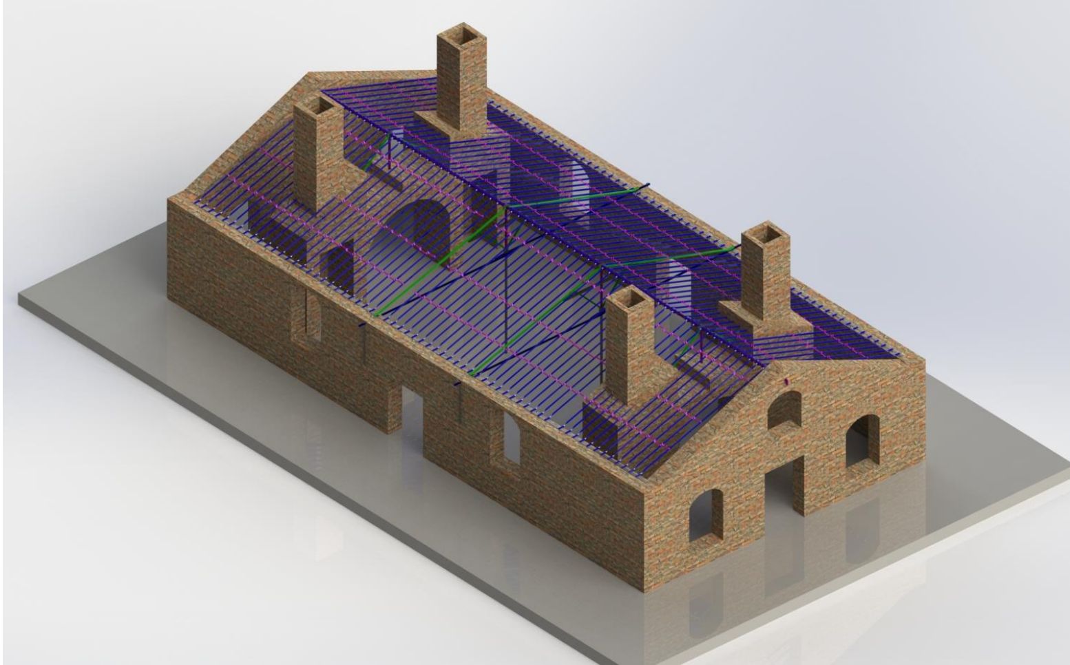
Şekil 4.83 14 numaralı yapı çatı str  kt  r  n  n restit  syon durum   nerisi.
