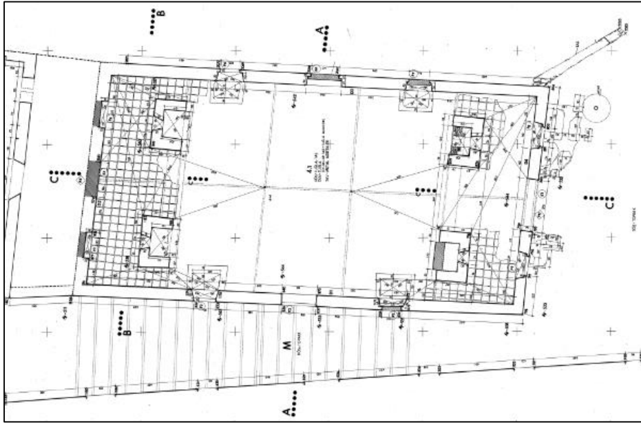
Őekil 4.3 14 numaralı yapının 1995 yılı plan rlvesi [36].
