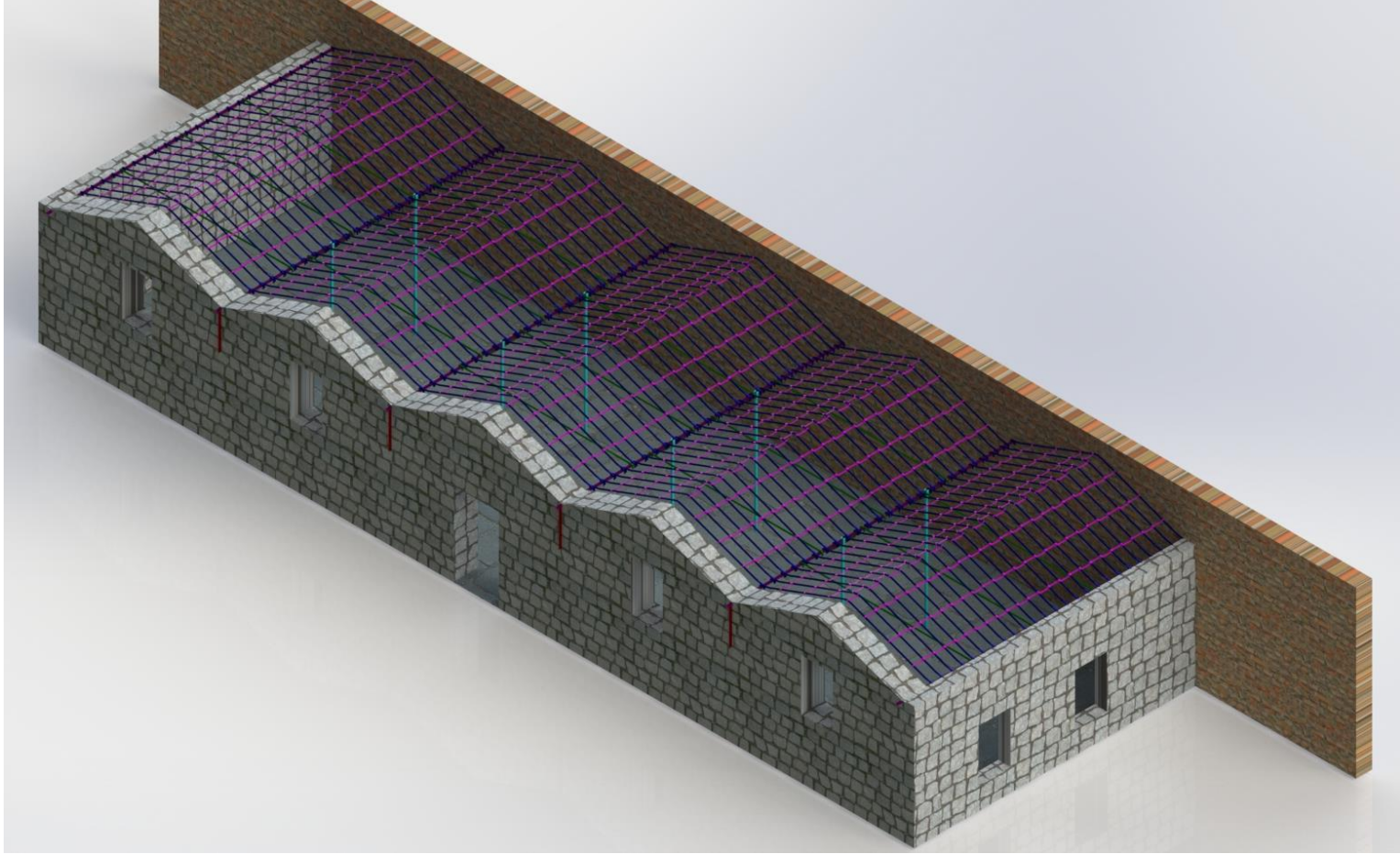
Şekil 4.80 15 numaralı yapı çatı strüktürünün restitüsyon durum önerisi (baca detayı gösterilmemiştir).
