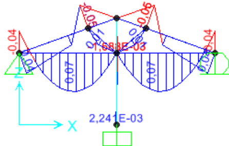
Şekil 4.115 Makasta yükleme altında moment diyagramı.
