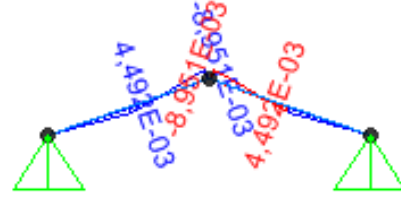
Şekil 4.90 Mertek öz ağırlıklar altında moment diyagramı.
