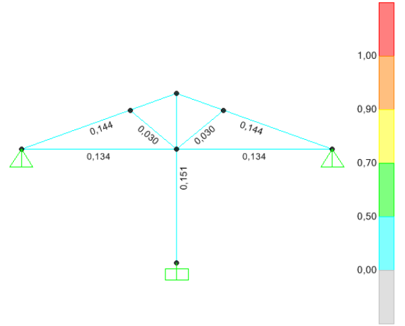
Şekil 4.122 Makasta öz ağırlıklar altında taşıma kapasitesi.
