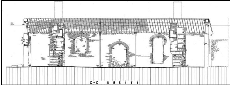
Şekil 4.5 14 numaralı yapının 1995 yılı kesit rölövesi [36].
