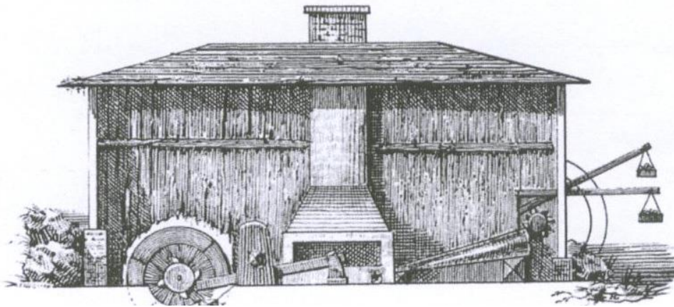
Şekil 2.7 Samakov dökümhanesinin kesitine ait gravür [5].
