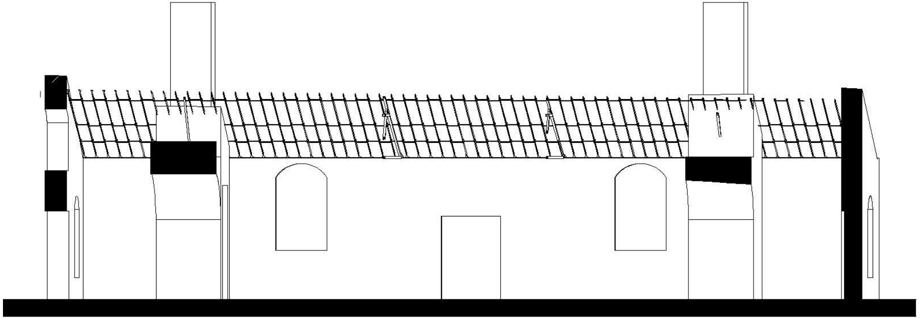
Şekil D. 2 14 numaralı yapının öneri çatı sistemi restitüsyon boy kesiti.
