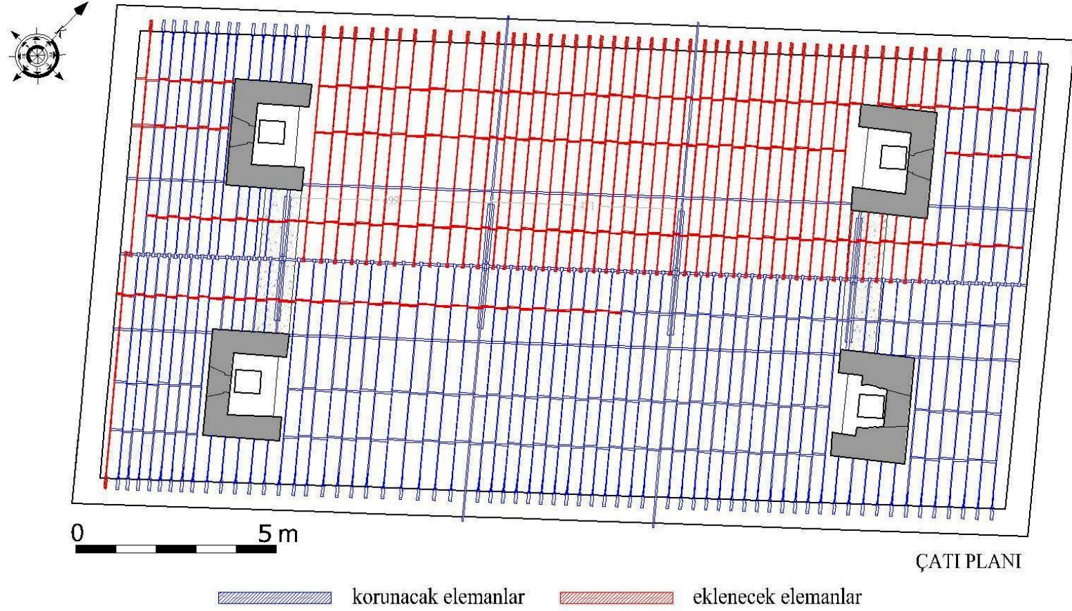
Şekil 4.125 14 numaralı yapıda korunacak ve tamamlanacak demir elemanlar.
