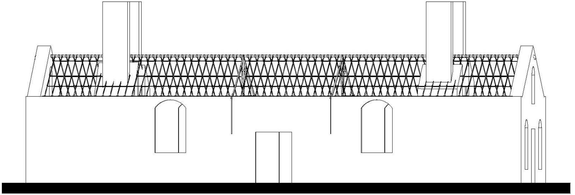
Şekil D. 3 14 numaralı yapının öneri çatı sistemi restitüsyon cephe görünüşü.
