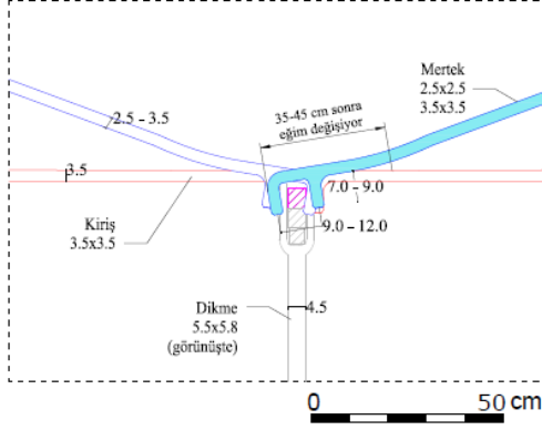
Şekil 4.40 15 numaralı yapı mertek birleşim detayı (B detayı).
