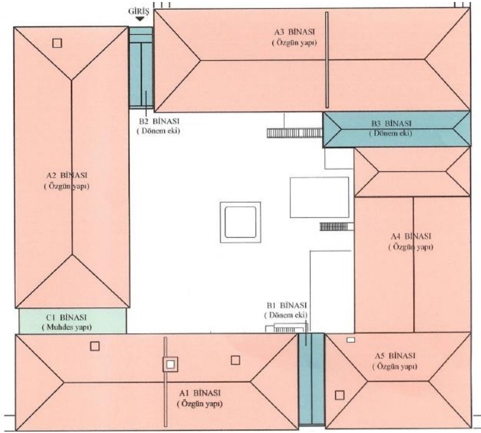
Şekil 3.19 Damga Matbaası binarının çatı planı [3].
