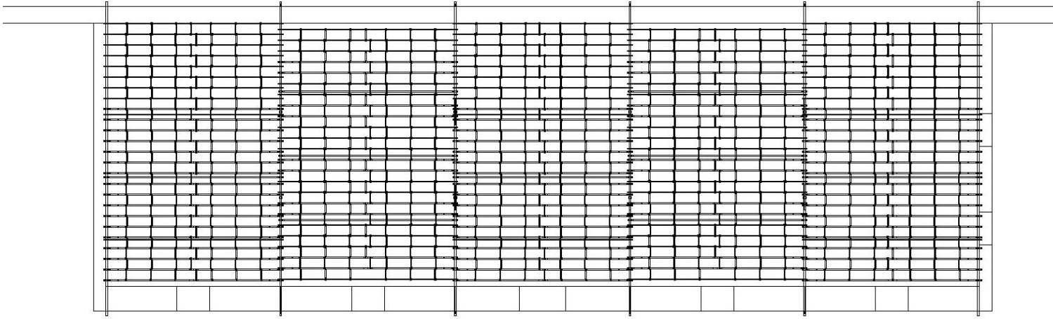
Şekil C. 1 15 numaralı yapının öneri çatı sistemi restitüsyon planı.
