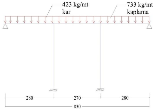
Şekil 4.97 15 numaralı yapı kirişi üzerinde yayılı yük.
