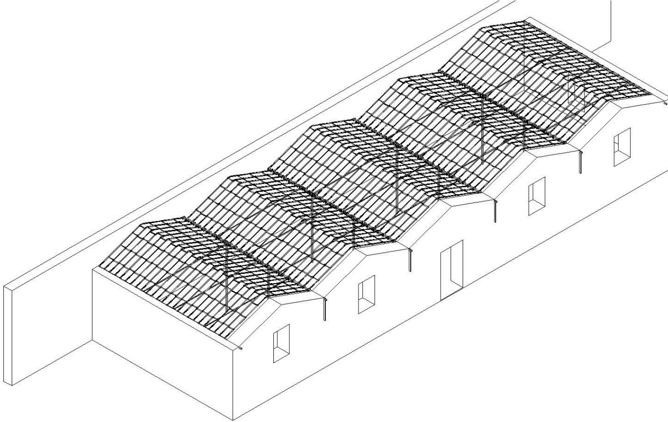
Şekil C. 3 15 numaralı yapının öneri çatı sistemi restitüsyon üç boyutlu görüntüsü.
