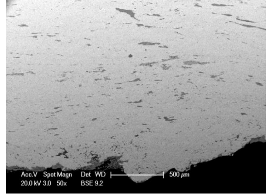
Şekil 4.71 14 numaralı yapıdan alınan örneğin elektron mikroskobu görüntüsü (x50).
