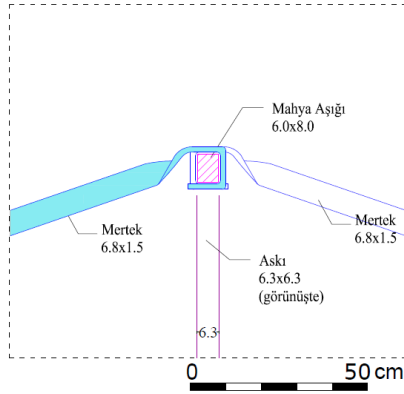
Şekil 4.60 14 numaralı yapı mahya birleşim detayı (G detayı).
