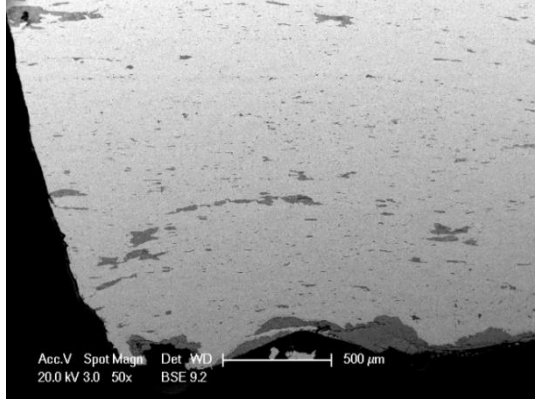
Şekil 4.70 14 numaralı yapıdan alınan örneğin elektron mikroskobu görüntüsü (x50).
