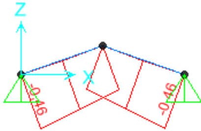
Şekil 4.91 Mertek kaplama ve kar yükü eksenel kuvvet diyagramı.
