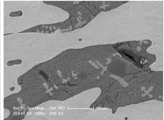
Şekil 4.73 14 numaralı yapıdan alınan örneğin elektron mikroskobu görüntüsü (x1000).
