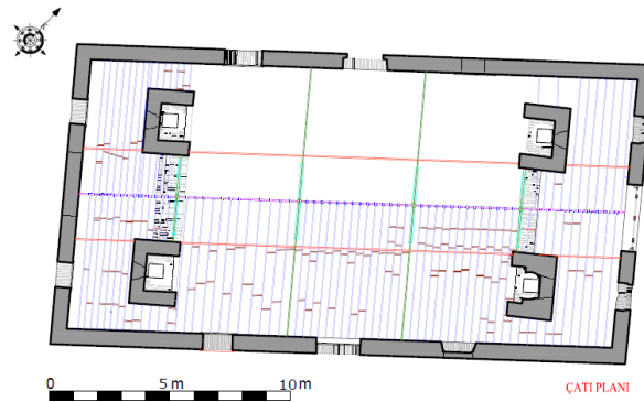
Şekil 4.34 14 numaralı yapı çatı karkas planı [26].
