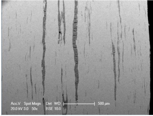
Şekil 4.66 15 numaralı yapıdan alınan örneğin elektron mikroskobu görüntüsü (x50).
