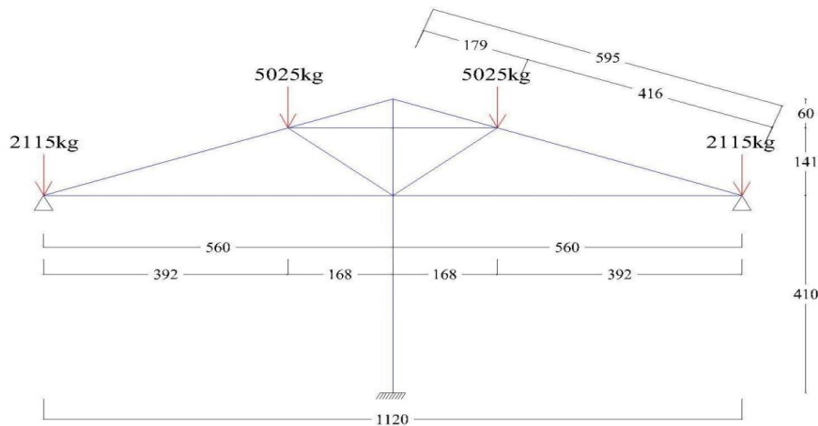
Şekil 4.112 14 numaralı yapının makas sistemi üzerine kaplama, kar ve merteklerden gelen yük.
