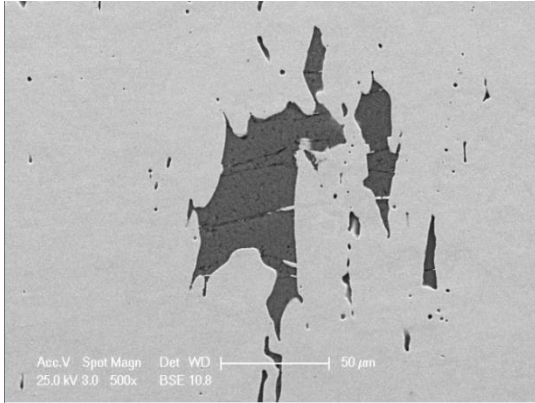
Şekil 4.68 15 numaralı yapıdan alınan örneğin elektron mikroskobu görüntüsü (x500).
