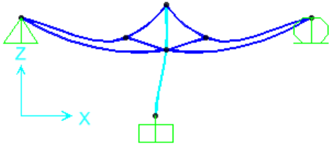
Şekil 4.113 Makasta yükleme altında şekil değiştirme.
