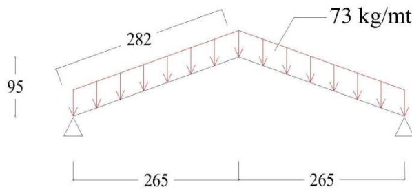
Şekil 4.84 15 numaralı yapı merteki üzerine etkiyen kaplama ve kar yükü.
