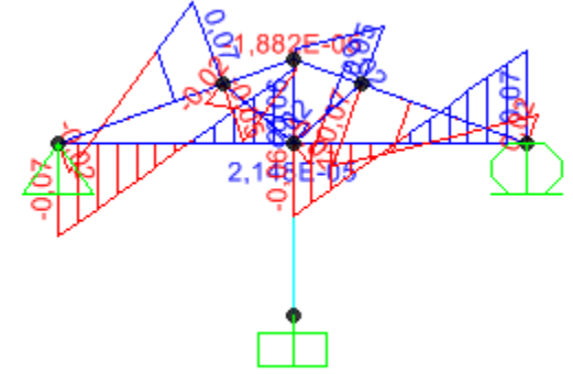
Şekil 4.120 Makasta öz ağırlıklar kesme kuvveti diyagramı.
