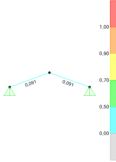
Şekil 4.96 Mertek öz ağırlıklar altında taşıma kapasitesi.
