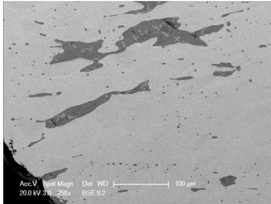
Şekil 4.72 14 numaralı yapıdan alınan örneğin elektron mikroskobu görüntüsü (x250).
