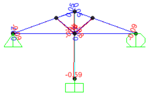
Şekil 4.118 Makasta öz ağırlıklar eksenel kuvvet diyagramı.
