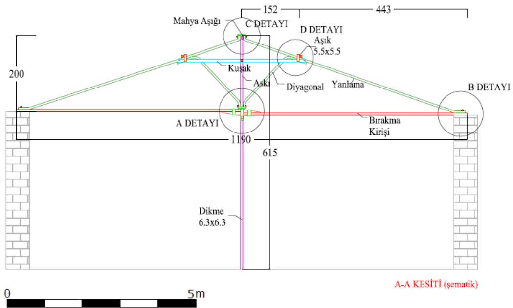
Şekil 4.47 14 numaralı yapıda çatı makasının detayları.
