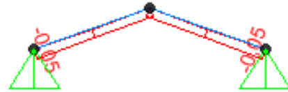
Şekil 4.92 Mertek öz ağırlıklar altında eksenel kuvvet diyagramı.
