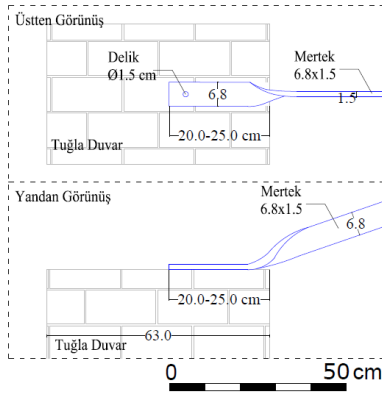
Şekil 4.56 14 numaralı yapı mertek bağlantı detayı (E detayı).
