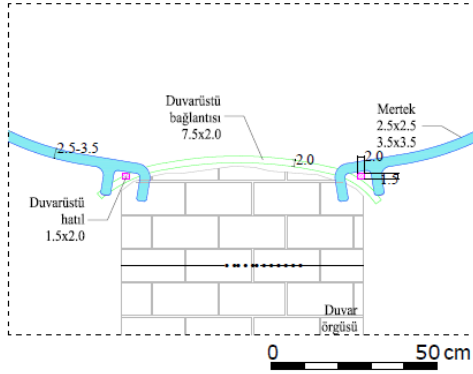
Şekil 4.44 15 numaralı yapı mertek bağlantı detayı (D detayı).
