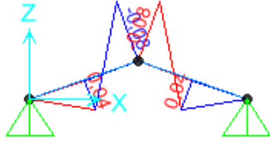
Şekil 4.89 Mertek kaplama ve kar yükü altında moment diyagramı.
