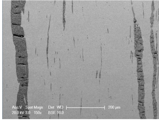
Şekil 4.67 15 numaralı yapıdan alınan örneğin elektron mikroskobu görüntüsü (x150).
