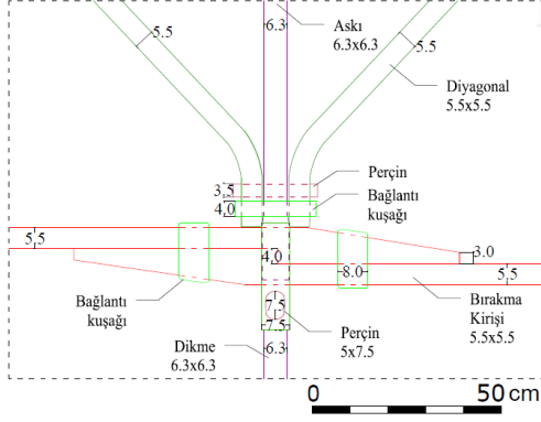
Şekil 4.48 14 numaralı yapı makası bağlantı detayı (A detayı).
