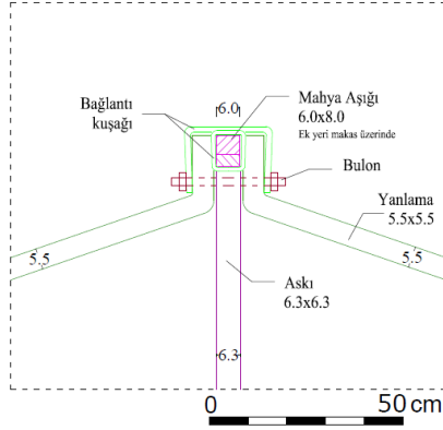
Şekil 4.52 14 numaralı mahya aşığı birleşim detayı (C detayı).
