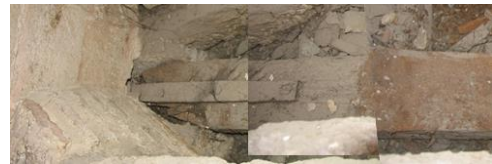
Şekil 2.12 Süleymaniye Camii ahşap hatılların demirli birleşimi.
