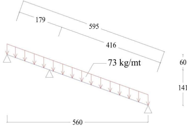
Şekil 4.110 14 numaralı yapı merteği üzerine etkiyen kaplama ve kar yükü.
