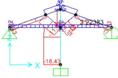
Şekil 4.117 Makasta yükleme altında eksenel kuvvet diyagramı.
