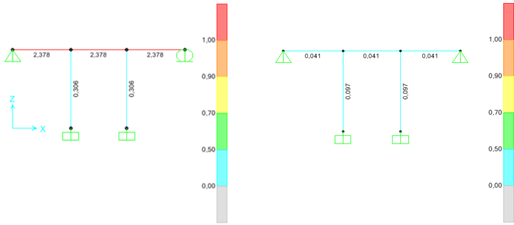
Şekil 4.108 Kirişte kaplama ve kar yükü altında taşıma kapasitesi.
