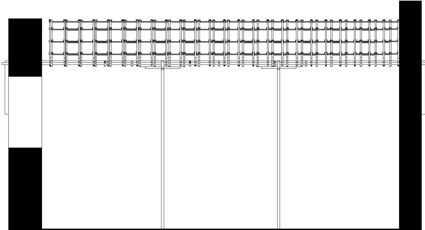
Şekil C. 4 15 numaralı yapının öneri çatı sistemi restitüsyon en kesiti.
