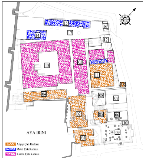
Şekil 3.27 Darphane-i Amire yapılarının mevcut üst örtü taşıyıcı sistem karkasının malzemesel analizi.
