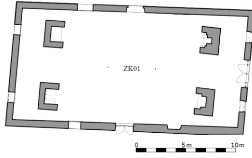
Şekil 4.16 14 numaralı yapının plan şeması [26].
