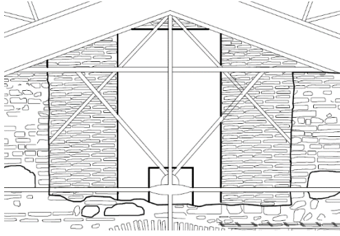
Şekil 4.11 14 nolu yapının 2010 yılı çiziminde detay [26].
