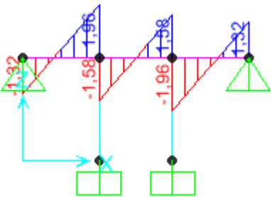
Şekil 4.106 Kirişte kaplama ve kar yükü kesme kuvveti diyagramı.
