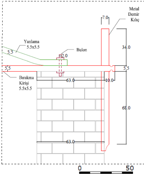
Şekil 4.50 14 numaralı yapı makası birleşim detayı (B detayı).
