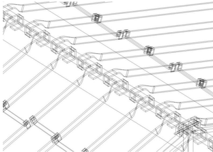
Şekil 4.62 14 numaralı yapıda merteklerin mahya aşığına bağlantısı.
