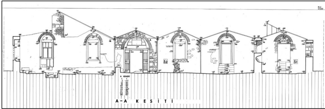
Şekil 4.6 15 numaralı yapının 1995 yılı kesit rölövesi [36].
