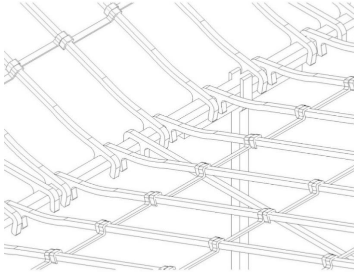
Şekil 4.46 15 numaralı yapıda mertek ve tali kirişlerin ana kirişler üzerinde bağlantısı.
