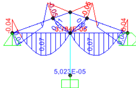
Şekil 4.116 Makasta öz ağırlıklar altında moment diyagramı.
