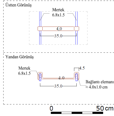
Şekil 4.58 14 numaralı yapı bağlantı elemanı detayı (F detayı).
