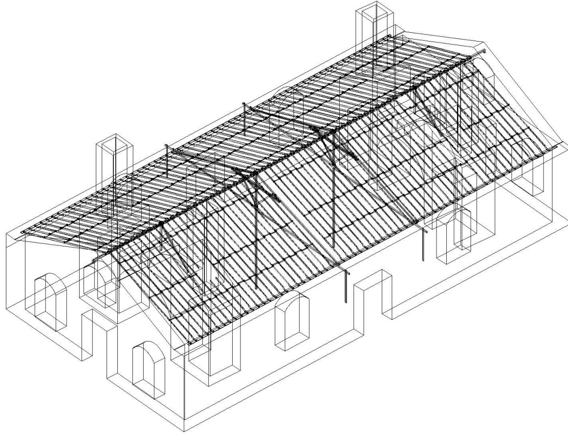
Şekil D. 4 14 numaralı yapının öneri çatı sistemi restitüsyon üç boyutlu görüntüsü.
