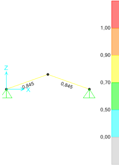
Şekil 4.95 Mertek kaplama ve kar yükü altında taşıma kapasitesi.
