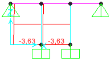
Şekil 4.104 Kirişte kaplama ve kar yükü eksenel kuvvet diyagramı.
