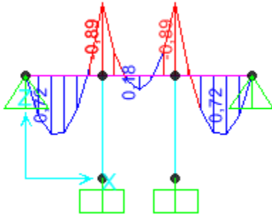
Şekil 4.102 Kirişte kaplama ve kar yükü altında moment diyagramı.
