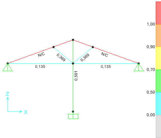
Şekil 4.121 Makasta yükleme altında taşıma kapasitesi.
