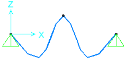
Şekil 4.87 Mertek kaplama ve kar yükü altında şekil değişimi.
