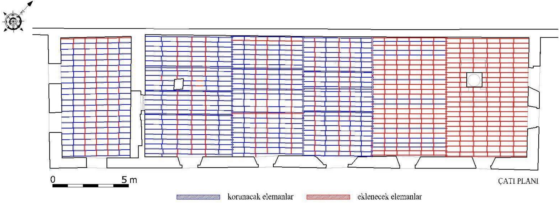
Şekil 4.124 15 numaralı yapıda korunacak ve tamamlanacak demir elemanlar.
