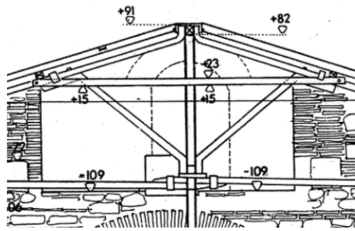
Şekil 4.12 14 nolu yapının 1995 yılı çiziminde detayı [36].
