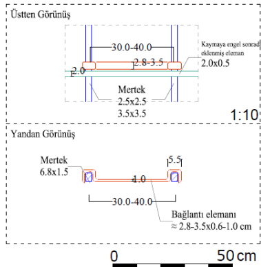
Şekil 4.42 15 numaralı yapı bağlantı elemanı detayı (C detayı).
