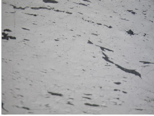
Şekil 4.77 14 numaralı yapı örneğinin optik mikroskopta görünen mikro yapısı.
