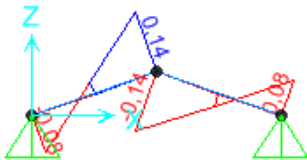
Şekil 4.93 Mertek kaplama ve kar yükü kesme kuvveti diyagramı.
