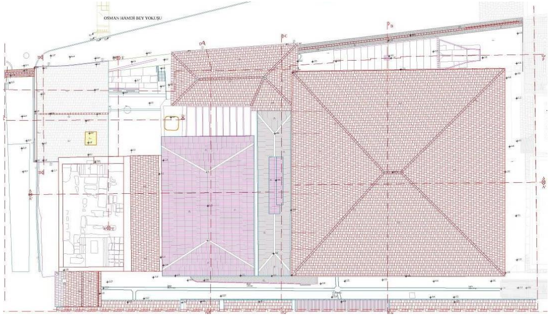
Şekil 3.18 11 ve 12 numaralı yapılar grubunun çatı örtüsü planı [26].
