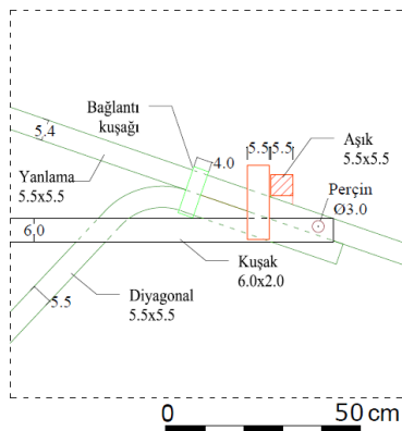
Şekil 4.54 14 numaralı yapı yanlama birleşim detayı (D detayı).
