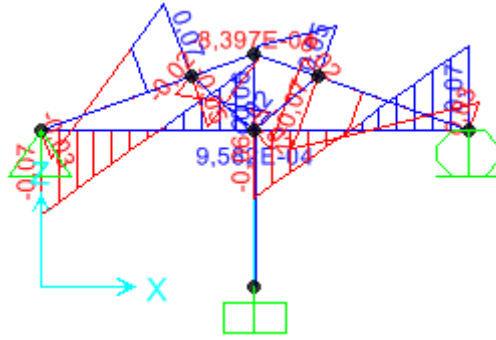
Şekil 4.119 Makasta yükleme altında kesme kuvveti diyagramı.
