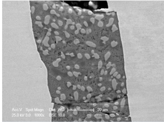
Şekil 4.69 15 numaralı yapıdan alınan örneğin elektron mikroskobu görüntüsü (x1000).
