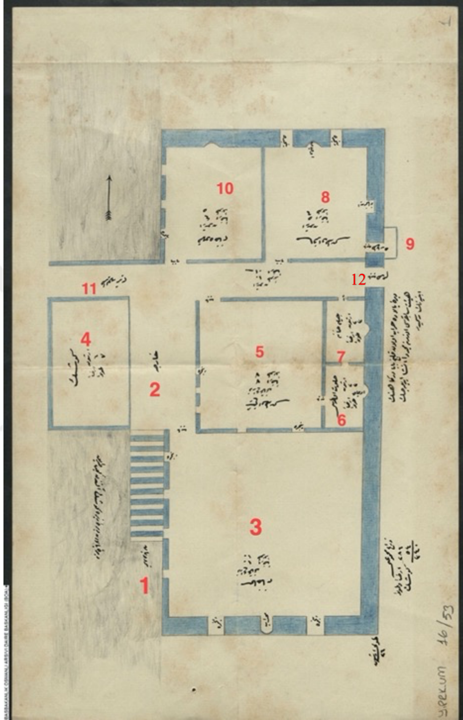
Şekil 18: Kılıç Baba Tekkesi Planı. 1- Merdiven 2- Hârici 3- Semahane 4- Köşk 5-Şeyh Odası 6-Halvet Odası 7- Çilehane 8-Misafir Odası 9- Bâb-ı tahare 10- Kahve Odası 11-Türbe-i Tarık 12- Bâb-ı harem. (BOA, Y.PRK.UM.16.53.1.)
