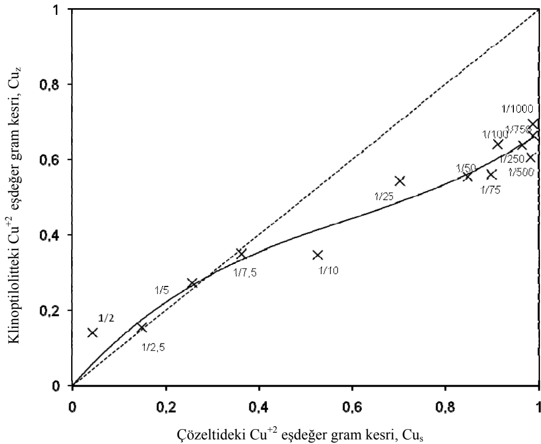
Şekil 6. 2. Farklı klinoptilolit (g)/çözelti(mL) oranlarında Na-klinoptilolit ile \text{Cu}^{+2} katyonunun değişim izotermi ( T=25^{\circ}\text{C} ve Toplam çözelti derişimi=0,1N)
