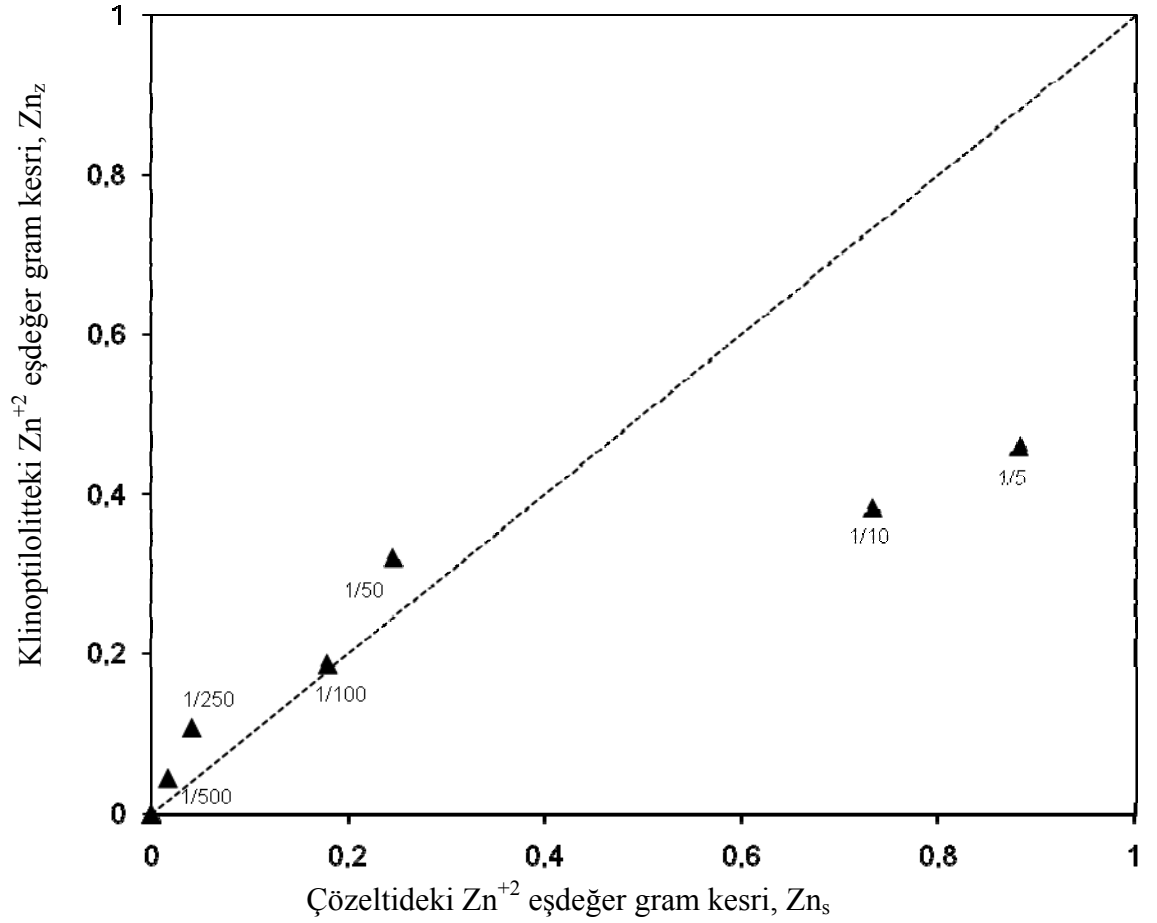
Şekil 8. 2. Farklı klinoptilolit (g)/çözelti(ml) oranlarında Zn-klinoptilolit Na katyonu için değişim izotermi ( T=25^{\circ}C ve Toplam çözelti derişimi=0,1N)
