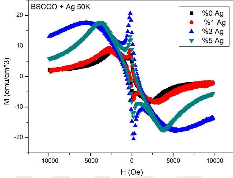
Şekil 4.49. %Ag katkılı \text{Bi}_2\text{Sr}_2\text{Ca}_{0.925}\text{Na}_{0.075}\text{Cu}_2\text{O}_y örneklerinin 50K'de M - H eğrileri
