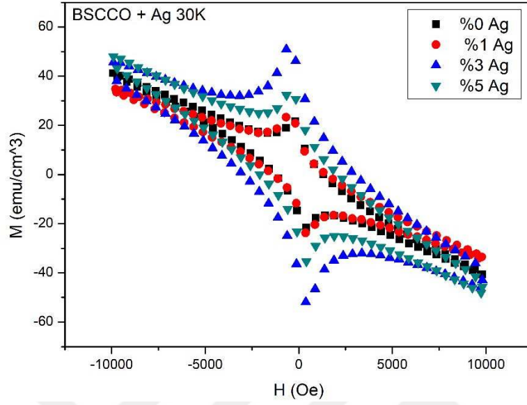
Şekil 4.47. %Ag katkılı \text{Bi}_2\text{Sr}_2\text{Ca}_{0.925}\text{Na}_{0.075}\text{Cu}_2\text{O}_y örneklerinin 30K'de M - H eğrileri
