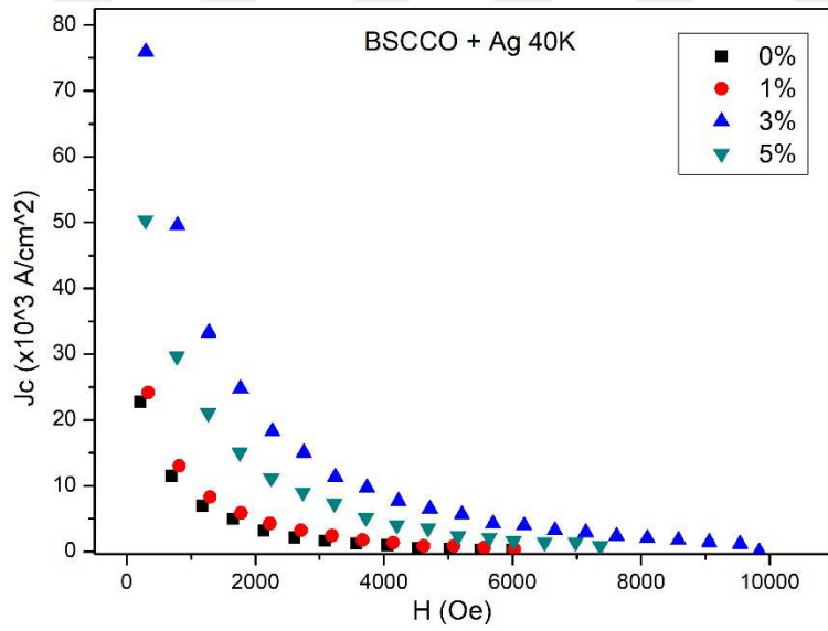
Şekil 4.57. %Ag katkılı \text{Bi}_2\text{Sr}_2\text{Ca}_{0.925}\text{Na}_{0.075}\text{Cu}_2\text{O}_y örneklerinin 40K'de kritik akım yoğunluğu grafiği
