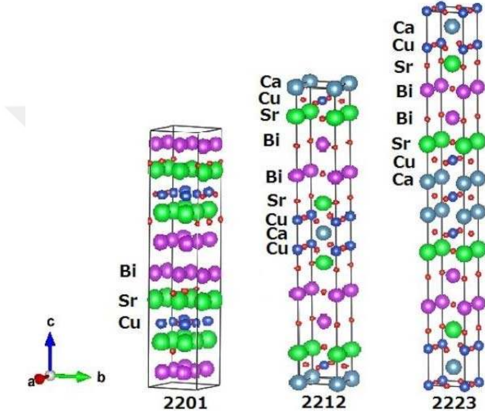
Şekil 1.6. Bi-2201, Bi-2212 ve Bi-2223 fazlarının kristal yapıları ( http://www.researchgate.net )
