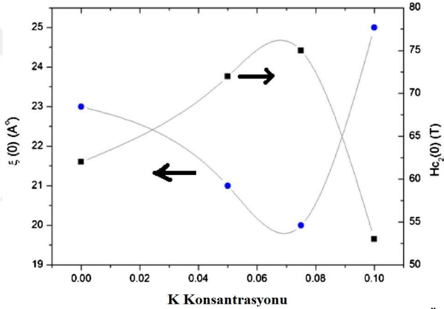
Şekil 2.8. H_{c2} ve \xi değerlerinin K konsantrasyonuna göre değişimleri (B. Özçelik, 2014)
