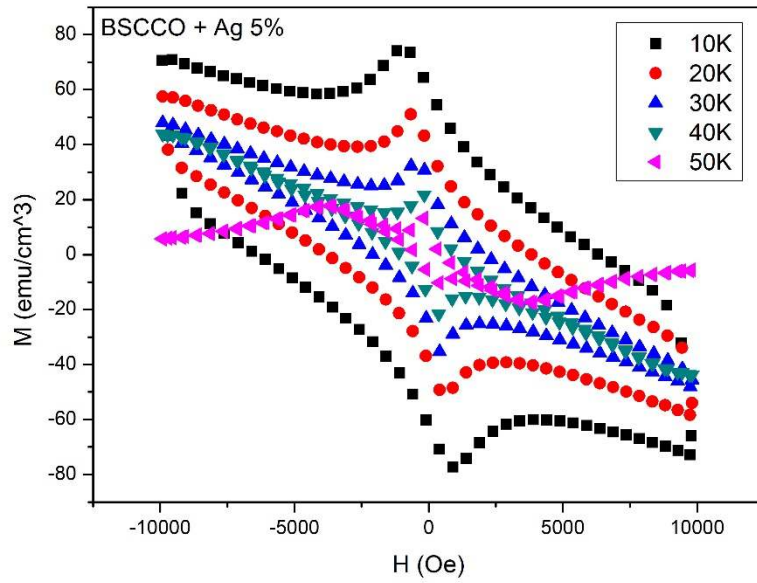
Şekil 4.44. %5 Ag katkılı \text{Bi}_2\text{Sr}_2\text{Ca}_{0.925}\text{Na}_{0.075}\text{Cu}_2\text{O}_y örneklerinin M - H eğrileri
