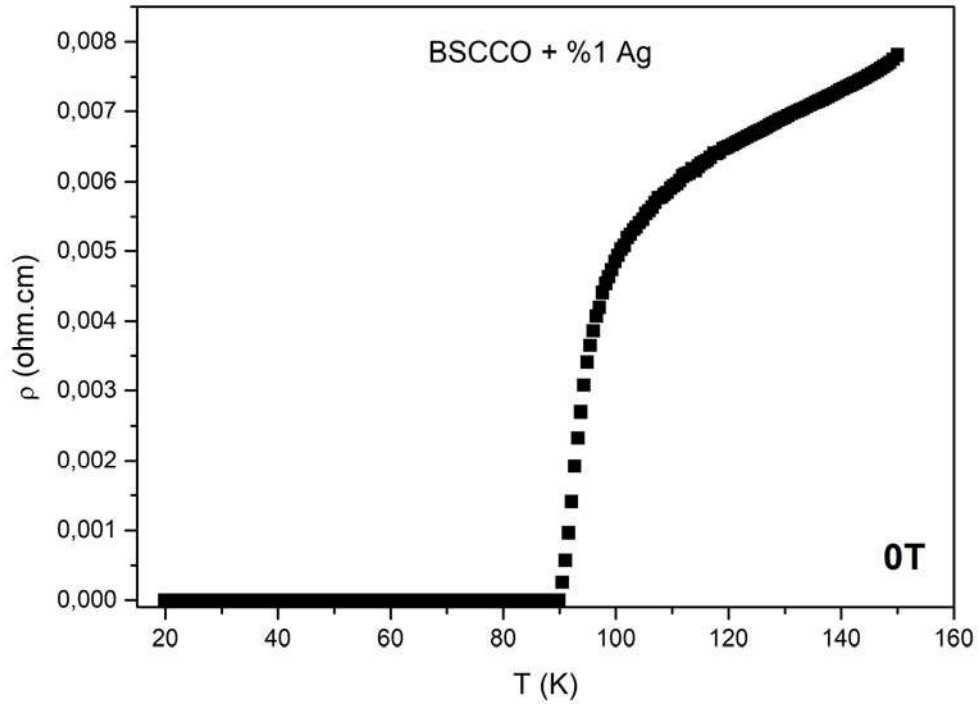
Şekil 4.12. %1 Ag katkılı \text{Bi}_2\text{Sr}_2\text{Ca}_{0.925}\text{Na}_{0.075}\text{Cu}_2\text{O}_y örneklerinin 0 T’da \rho - T grafiği
