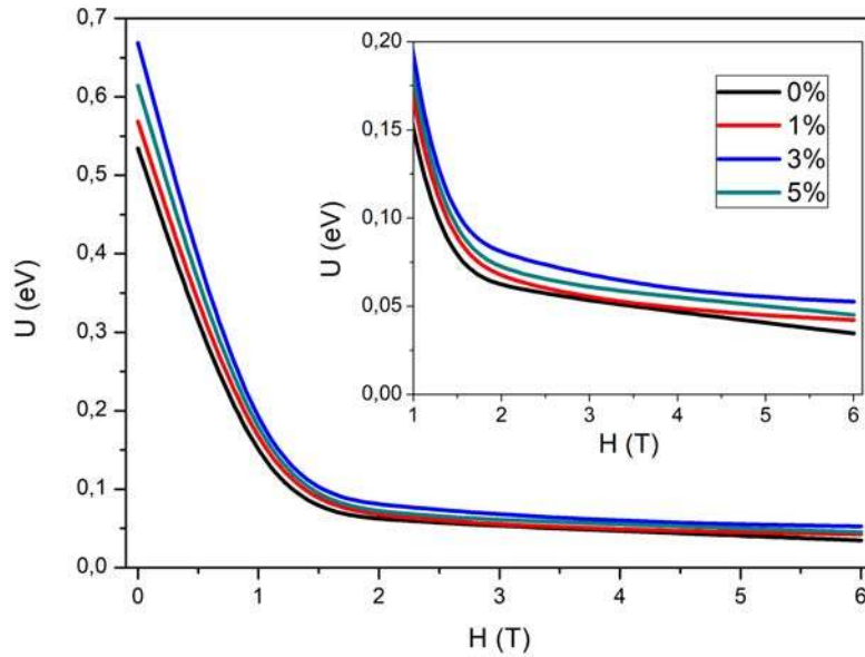
Şekil 4.39. %Ag katkılı \text{Bi}_2\text{Sr}_2\text{Ca}_{0.925}\text{Na}_{0.075}\text{Cu}_2\text{O}_y örneklerinin çivileme aktivasyon enerjileri
