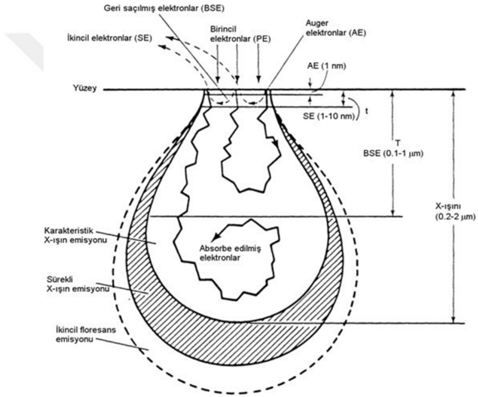
Şekil 3.3. Taramalı elektron mikroskobunda (SEM) elektronların malzeme ile etkileşimi ( https://www.metalurjik.net )
