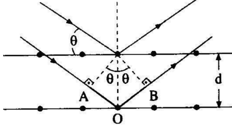
Şekil 3.2. Bragg kırınım yasası ( https://www.muhendisbeyinler.net/kristalografi-nedir )
