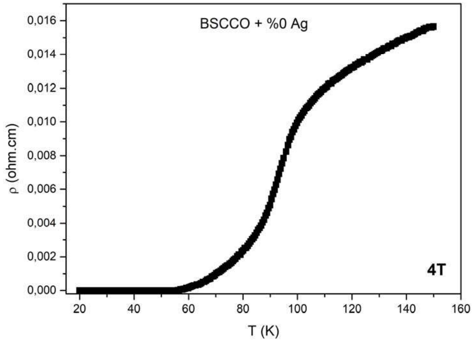
Şekil 4.9. %0 Ag katkılı \text{Bi}_2\text{Sr}_2\text{Ca}_{0.925}\text{Na}_{0.075}\text{Cu}_2\text{O}_y örneklerinin 4 T’da \rho - T grafiği
