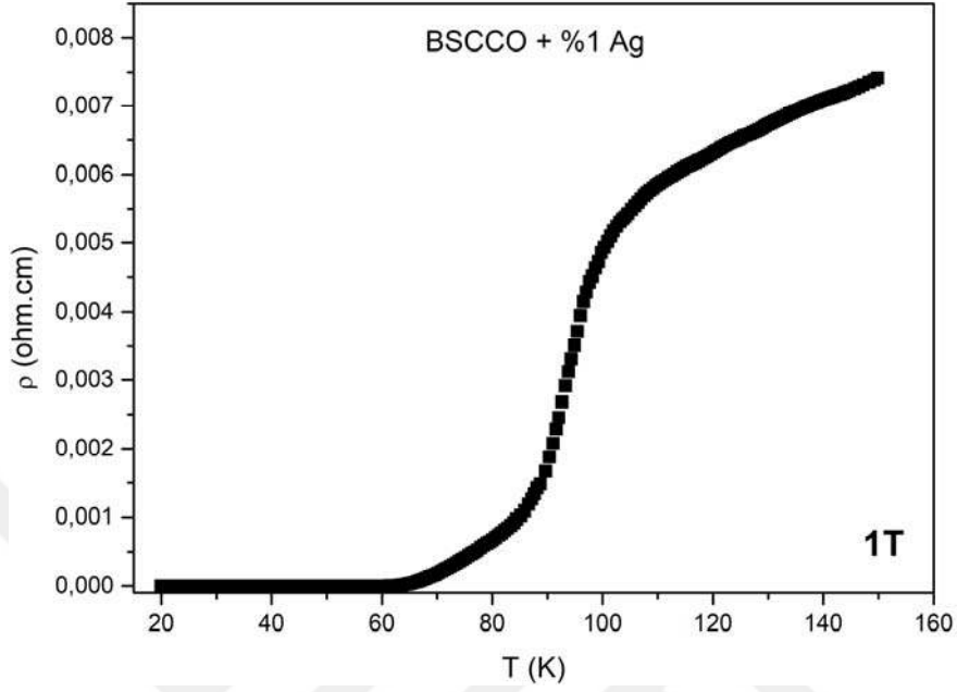
Şekil 4.13. %1 Ag katkılı \text{Bi}_2\text{Sr}_2\text{Ca}_{0.925}\text{Na}_{0.075}\text{Cu}_2\text{O}_y örneklerinin 1 T'da \rho - T grafiği
