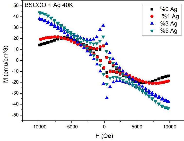
Şekil 4.48. %Ag katkılı \text{Bi}_2\text{Sr}_2\text{Ca}_{0.925}\text{Na}_{0.075}\text{Cu}_2\text{O}_y örneklerinin 40K’de M - H eğrileri
