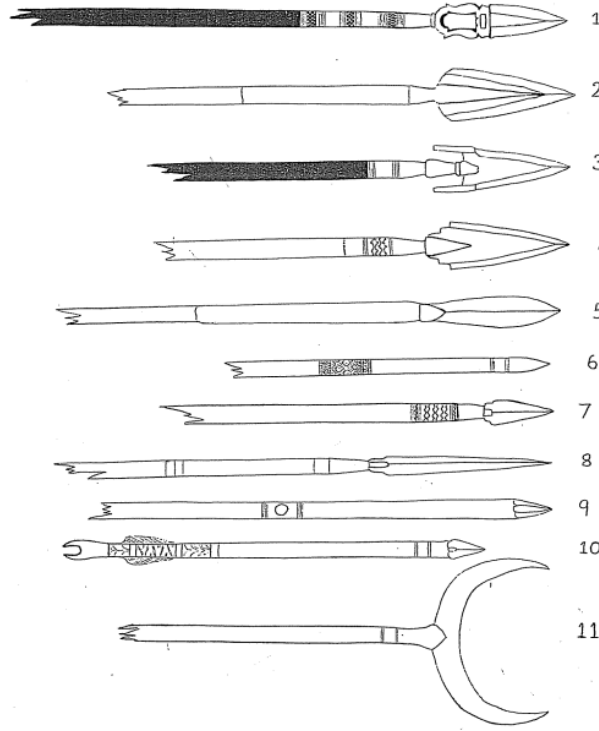
Şekil 3: Racastan ve Haydarâbâd Menşeiili Temren Örnekleri
