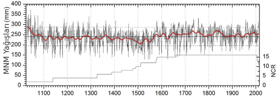
Şekil 1: Batı Himalayalar'ın ağaç halkası verileri ile oluşturulan boreal (MNM) bahar yağışı rekonstrüksiyonu (M. 1030-2011)
