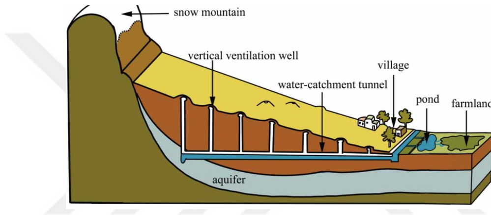
Şekil 2: Kâriz Uygulamalarının Şematik Diyagramı
