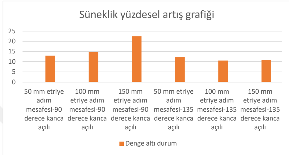
Şekil 6.15. Süneklikte yüzdesel artış grafiği
