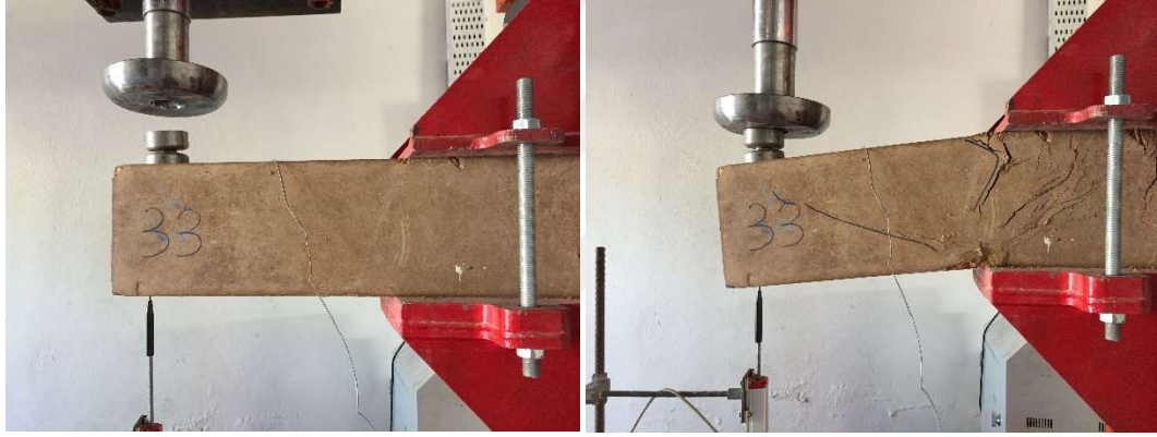
Şekil 5.2. 33 nolu seriye ait kiriş kırılma öncesi ve sonrası
