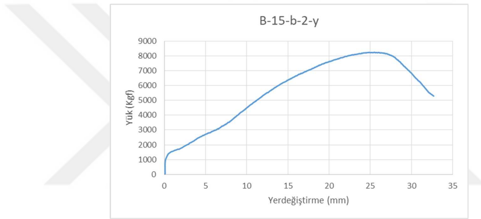
Şekil 5.29. B-15-b-2-y numunesi grafiği
