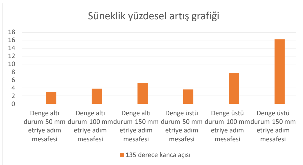
Şekil 6.7. Süneklikte yüzdesel artış grafiği
