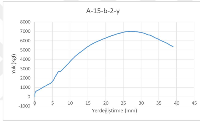
Şekil 5.23. A-15-b-2-y numunesi grafiği
