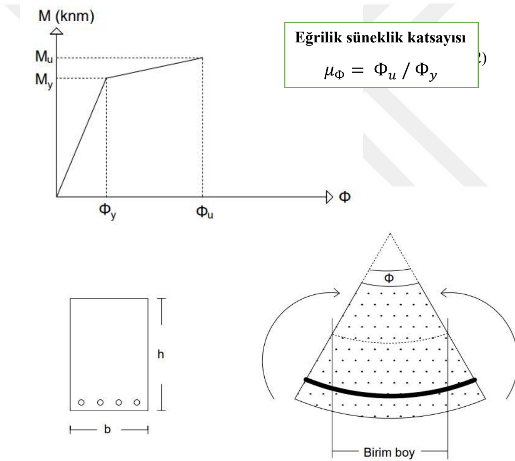
Şekil 3.11. Betonarme bir kirişin eğrilik sünekliği belirlenmesi
