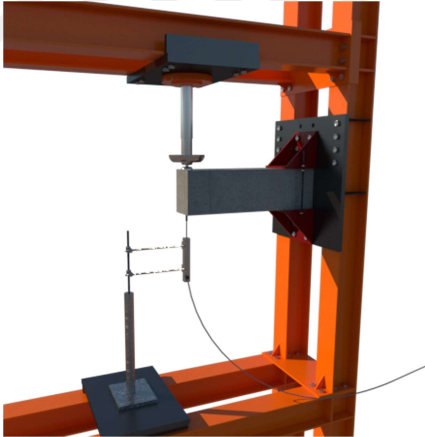
Şekil 4.20. Deney düzeneği
