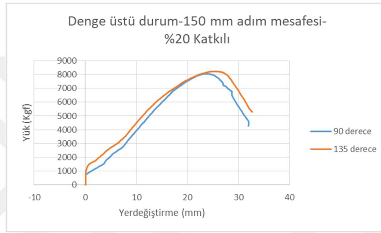
Şekil 6.14. Denge üstü durum-%20 Katkılı-150 mm Adım Mesafeli Numunelerin Karşılaştırmalı Grafiği
