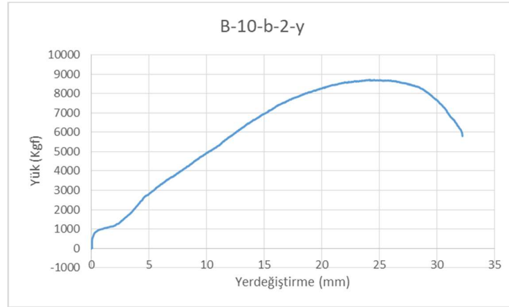
Şekil 5.27. B-10-b-2-y numunesi grafiği
