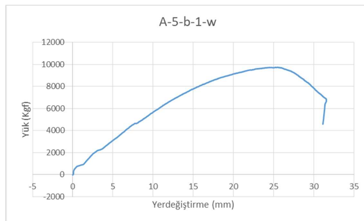
Şekil 5.7. A-5-b-1-w numunesi grafiği
