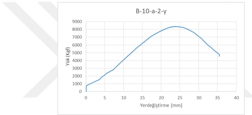
Şekil 5.26. B-10-a-2-y numunesi grafiği
