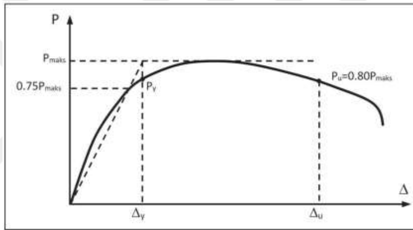
Şekil 3.10. Yük Yerdeğiřtirme Grafiğı [32]
