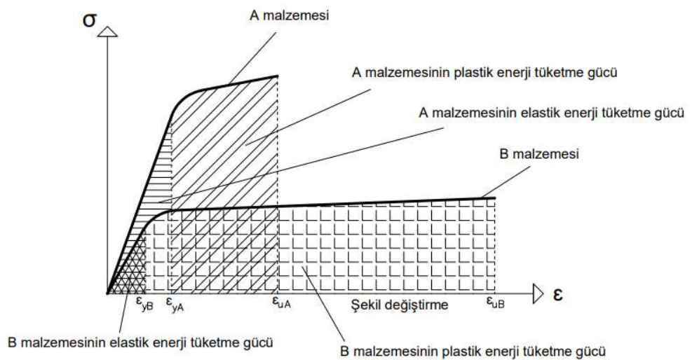
Şekil 3.9. Malzemelerin sünekliklerinin karşılaştırılması
