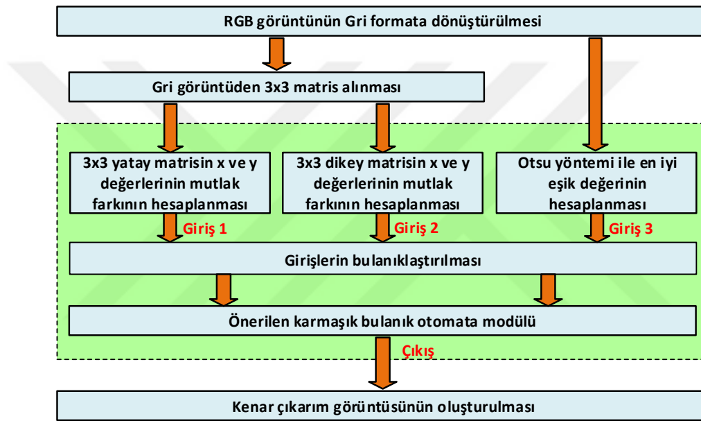
Şekil 3.20. Önerilen karmaşık bulanık otomata yönteminin akış şeması
