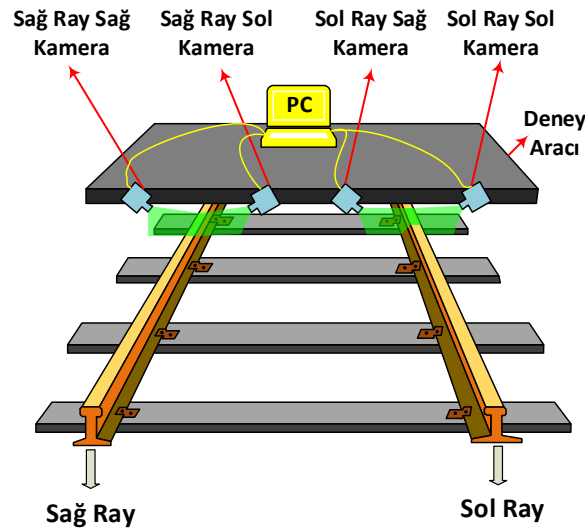
Şekil 4.19. Görüntü alımında kullanılan deneysel yapı
