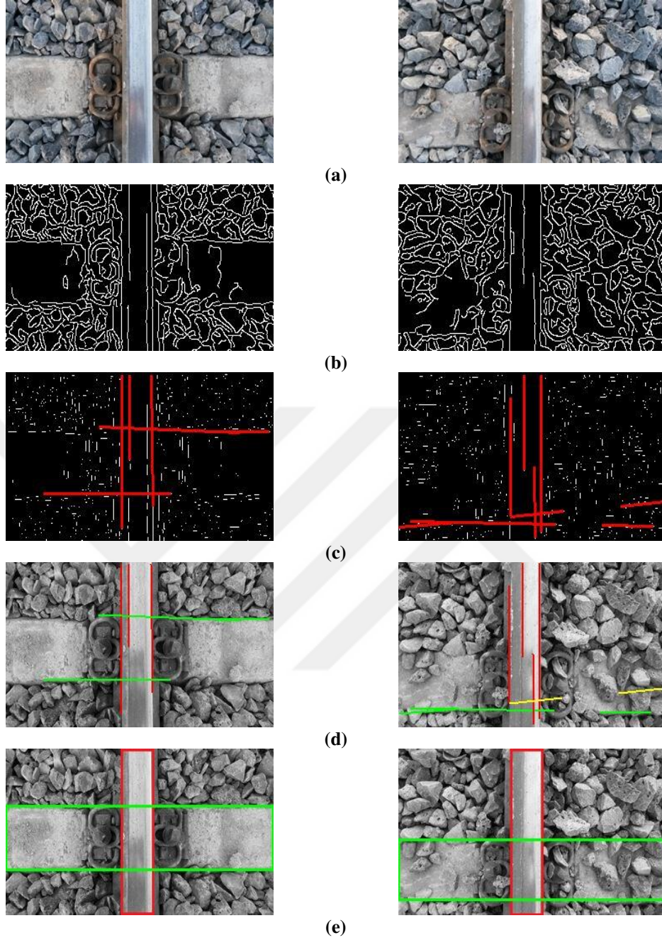
Şekil 4.12. Beton traverse ait bir demiryolundan alınan örnek görüntüler (a) Normal görüntü (b) Kenar çıkarım sonucunda elde edilen görüntü (c) Maske sonucunda Hough dönüşümü ile doğruların tespit edilmesi (d) Doğruların sınıflandırılması (e) Demiryolu bileşenlerinin tespit edilmesi
