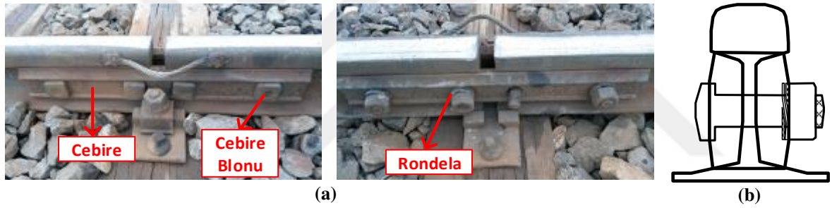
Şekil 2.6. Rayı raya bağlayan malzemeler (a) Örnek görüntü (b) Bağlantının farklı açıdan görünümü
