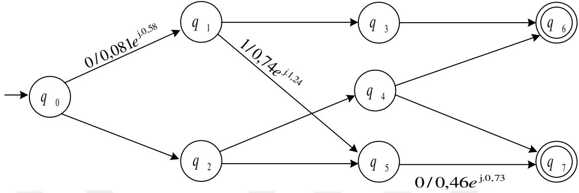
Şekil 3.22. Karmaşık bulanık otomata geçiş diyagramı
