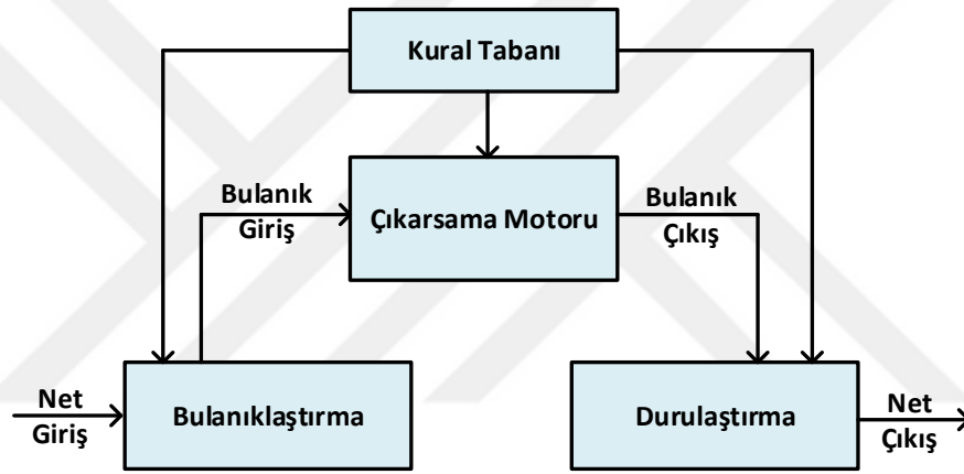
Şekil 3.4. Bulanık mantık yaklaşımının genel gösterimi
