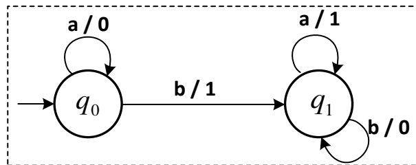
Şekil 3.1. Örnek bir sonlu durum makinesi için geçiş diyagramı
