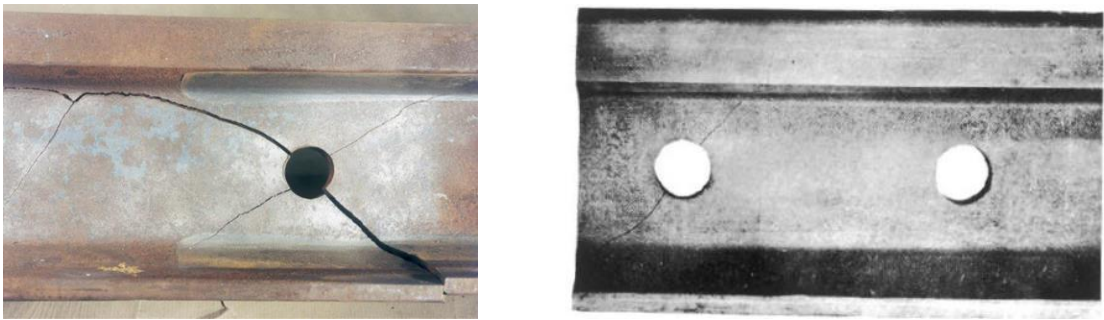
Şekil 2.25. Ray gövdesinde çapraz çatlak kusuru görüntüleri [124].
