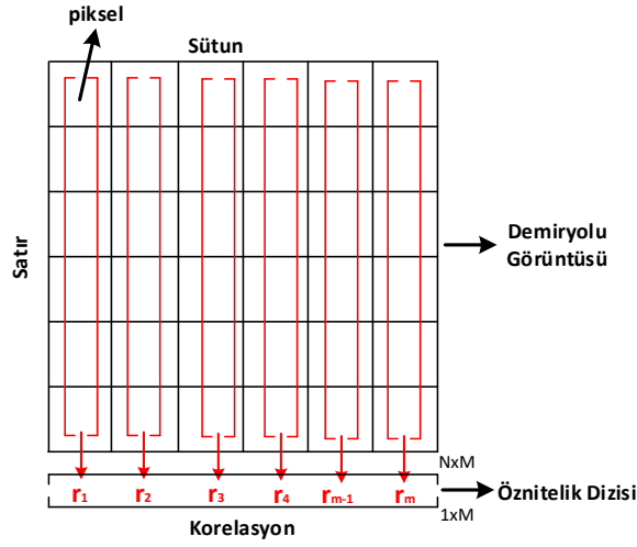
Şekil 5.3. Görüntüden oto korelasyon değeri hesaplanarak öznitelik dizisinin elde edilmesi
