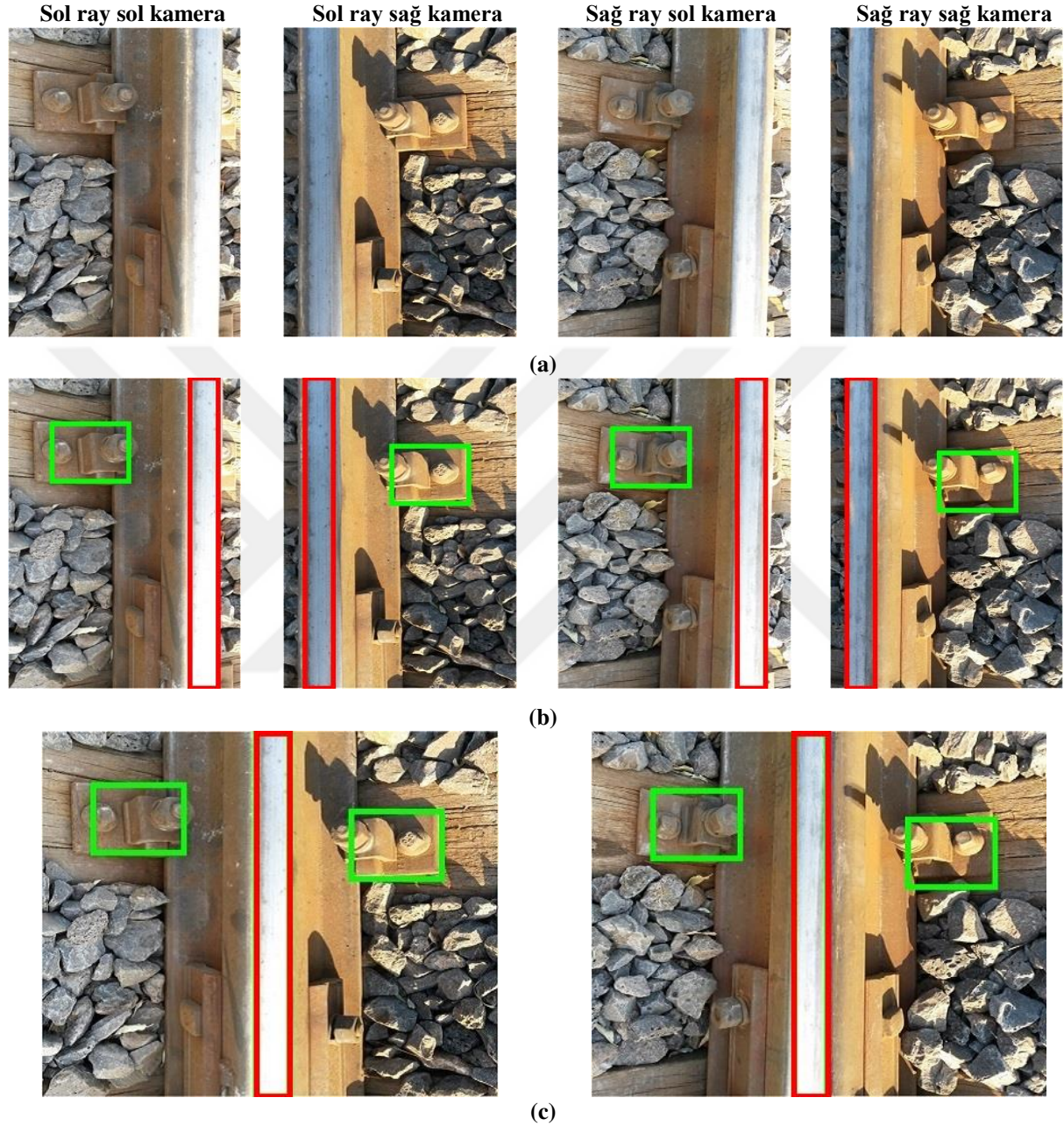
Şekil 4.20. Ahşap traverse sahip olan demiryolu hattından alınan görüntüler ve bu görüntülere önerilen yöntemin uygulanması (a) Dört kameradan alınan görüntüler (b) Görüntüler üzerinde ray yüzeyi ve demiryolu bileşenlerinin tespit edilmesi (c) Ray yüzeyleri dikkate alınarak görüntülerin birleştirilmesi
