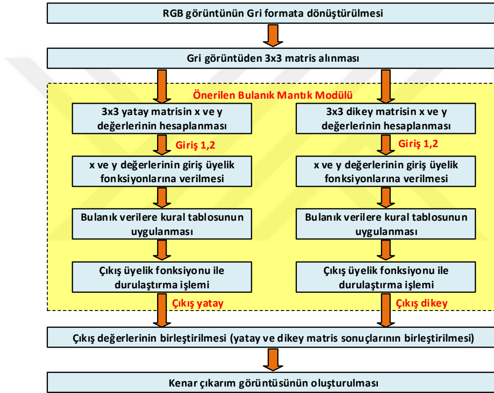
Şekil 3.5. Bulanık mantık tabanlı kenar çıkarım yöntemi
