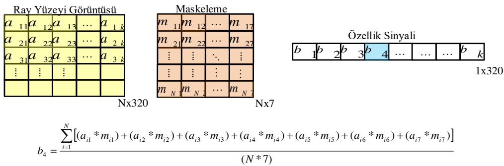
Şekil 6.17. Ray yüzey görüntüsünden özellik sinyalinin elde edilmesi
