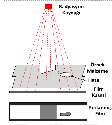
Şekil 2.30. Radyografi yönteminin temel yapısı [131]
