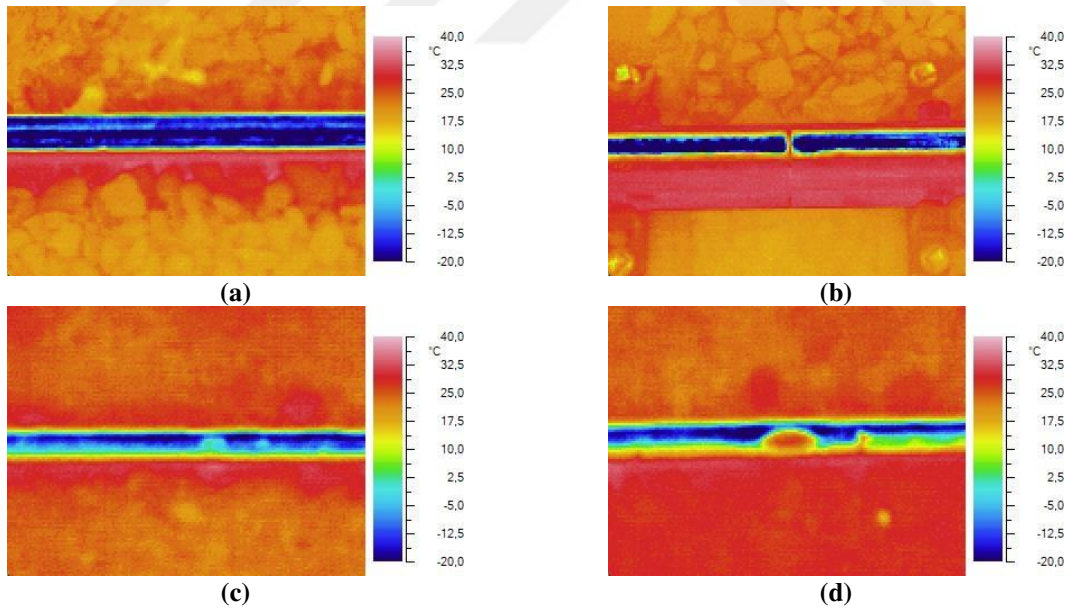
Şekil 6.22. Bu çalışmada kullanılan örnek termal görüntüler (a) Sağlam ray yüzeyi (b) Ray birleşme noktası (c) Arızalı ray yüzeyi (d) Arızalı ray yüzeyi
