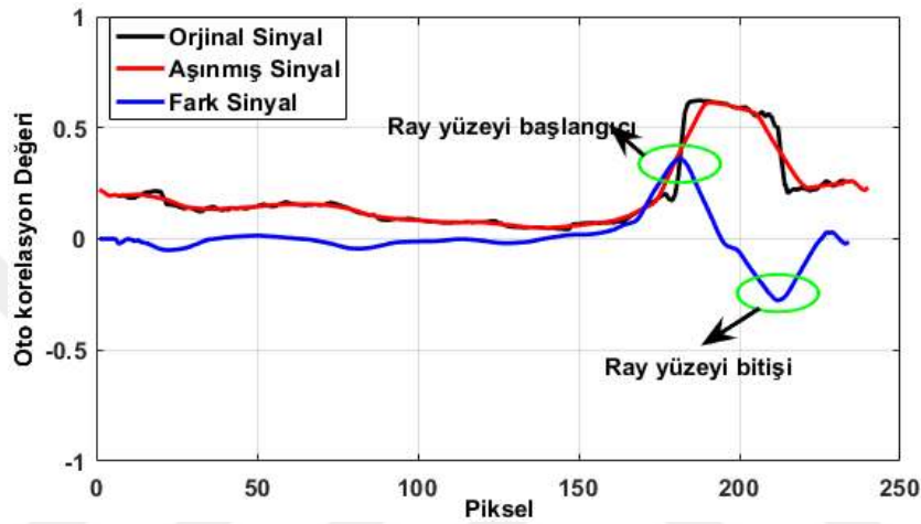
Şekil 5.4. Örnek bir görüntüden elde edilen sinyaller ve ray yüzeyinin tespit edilmesi
