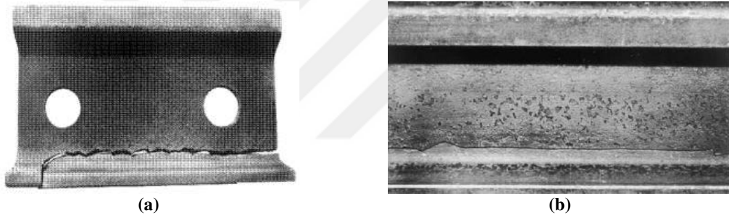
Şekil 2.22. Ray gövdesi ile tabanı arasındaki yatay çatlak görüntüsü [124] (a) UIC 1322 (b) UIC 2322.
