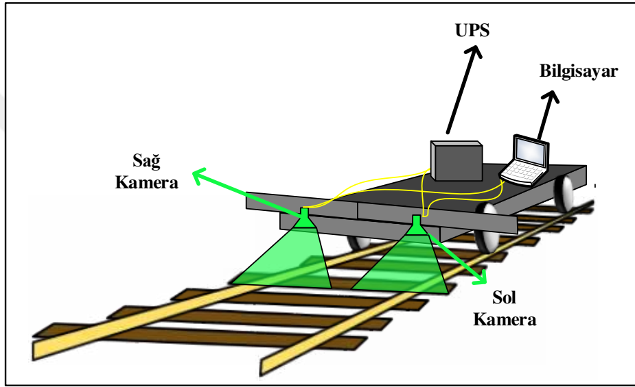
řekil 4.11. nerilen yntemde geliřtirilen deneysel dzenek
