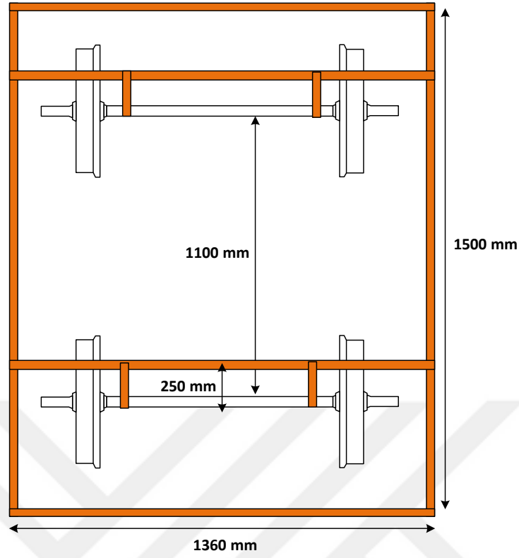
Şekil 4.1. Deney aracının bilgisayar ortamındaki çizimi
