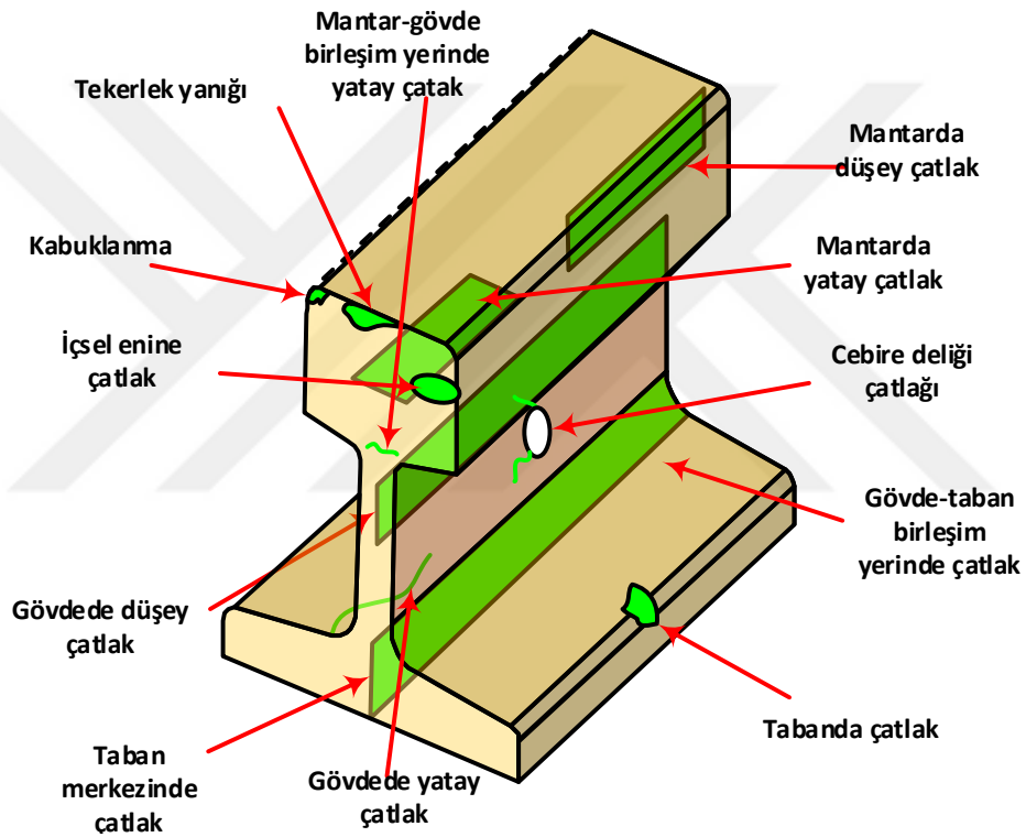
Şekil 2.8. Örnek bir ray üzerinde sıklıkla oluşan arızalar [117].
