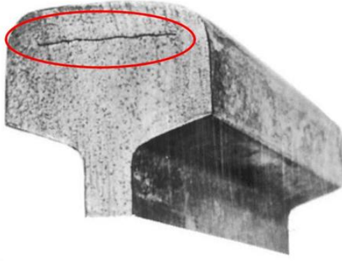
Şekil 2.10. Ray mantarında oluşan yatay çatlaklara ait örnek görüntü [124].
