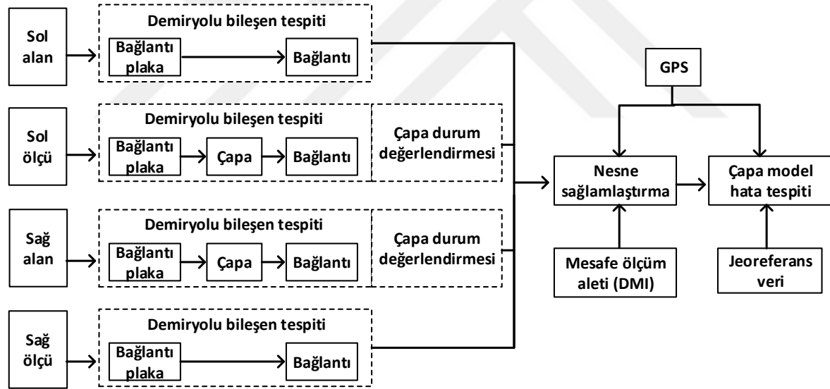
Şekil 1.4. Literatürde önerilen demiryolu denetim sisteminin genel mimarisi [33]
