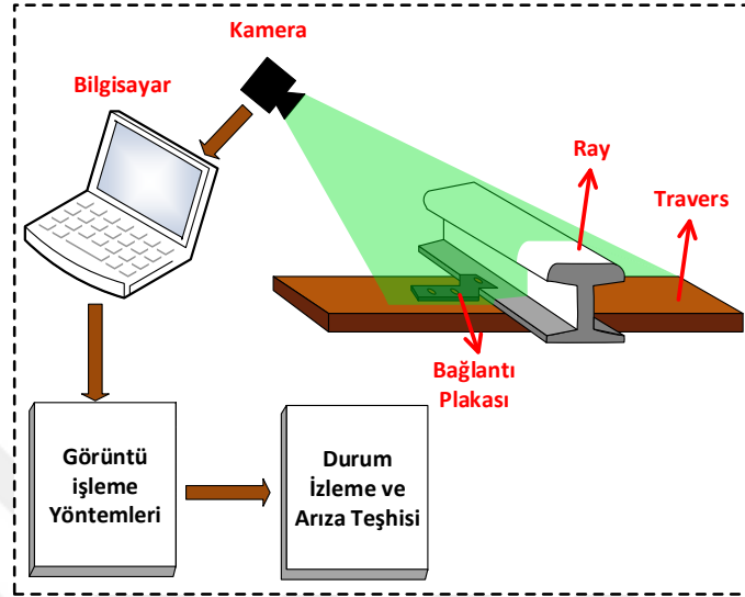
Şekil 1.1. Durum izleme ve arıza tespiti için kullanılan temassız yöntem
