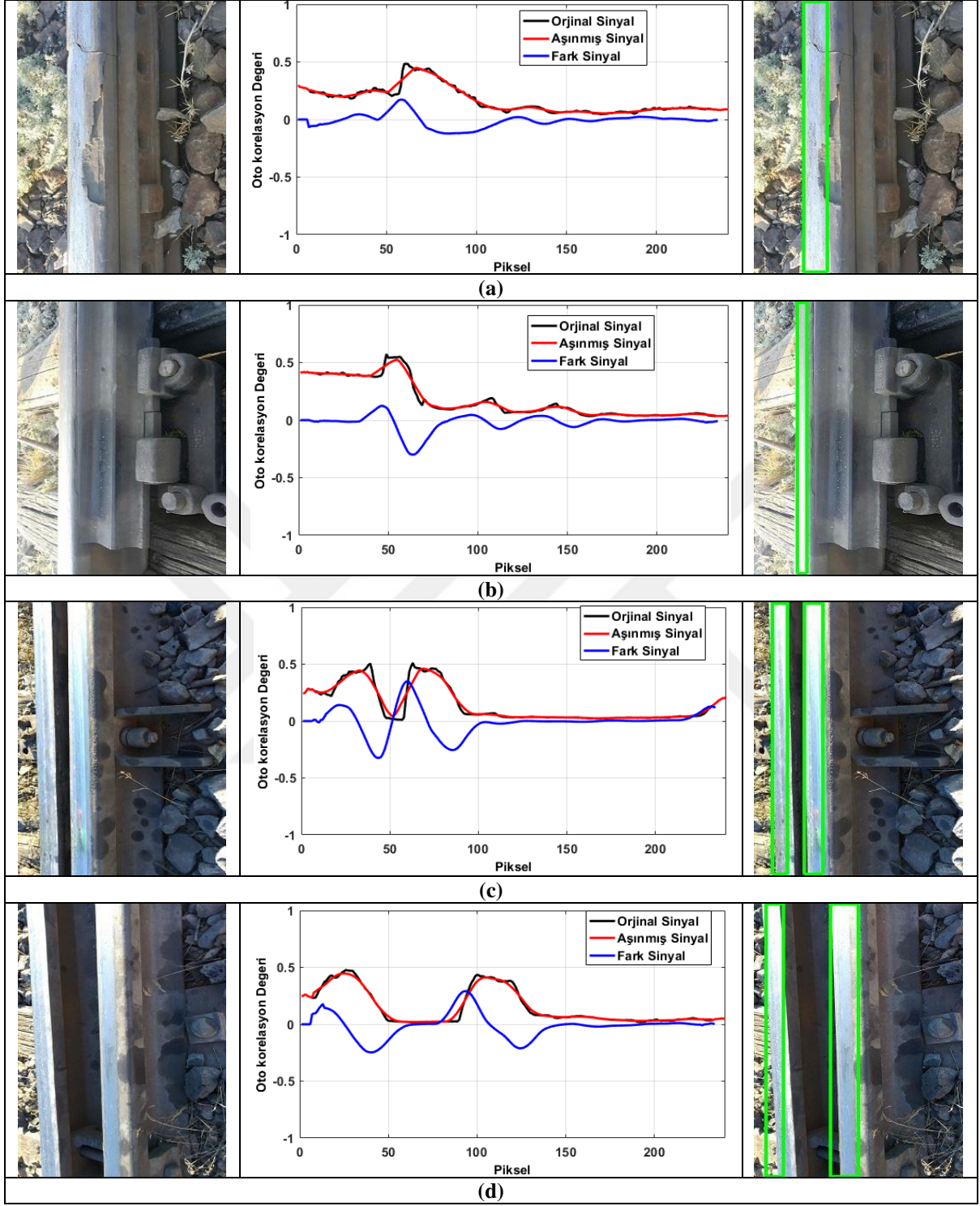
Şekil 5.6. Ahşap traverse sahip demiryolu hattında makas tespiti örneği (a) 1780. Çerçeve (b) 1900.Çerçeve (c) 2130. Çerçeve (d) 2300. Çerçeve
