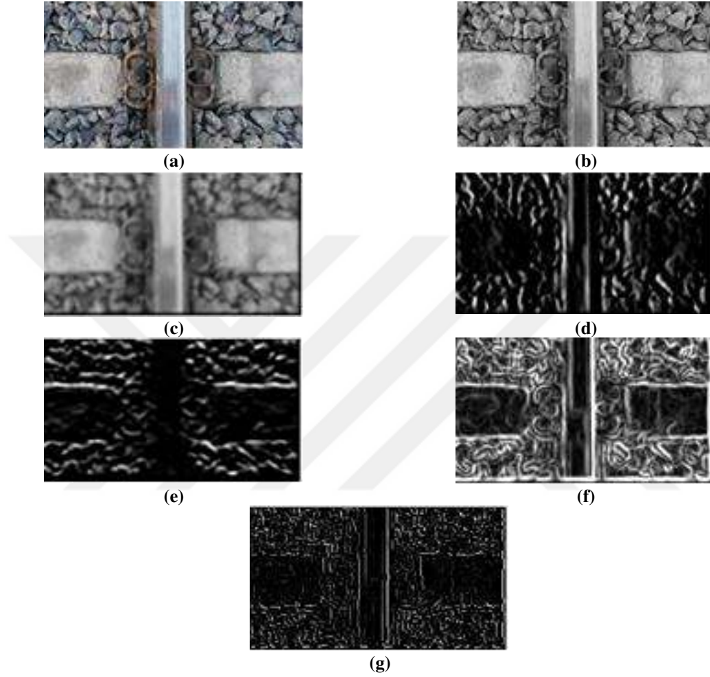
Şekil 4.8. Canny kenar çıkarım adımların örnek görüntüde uygulanması (a) Orijinal görüntü (b) Gri görüntü (c) Gaussian görüntü (d) X yönünde kenar çıkarımı (e) Y yönünde kenar çıkarımı (f) XY yönünde kenar çıkarımı (g) Özel açılara göre kenar çıkarım sonucu
