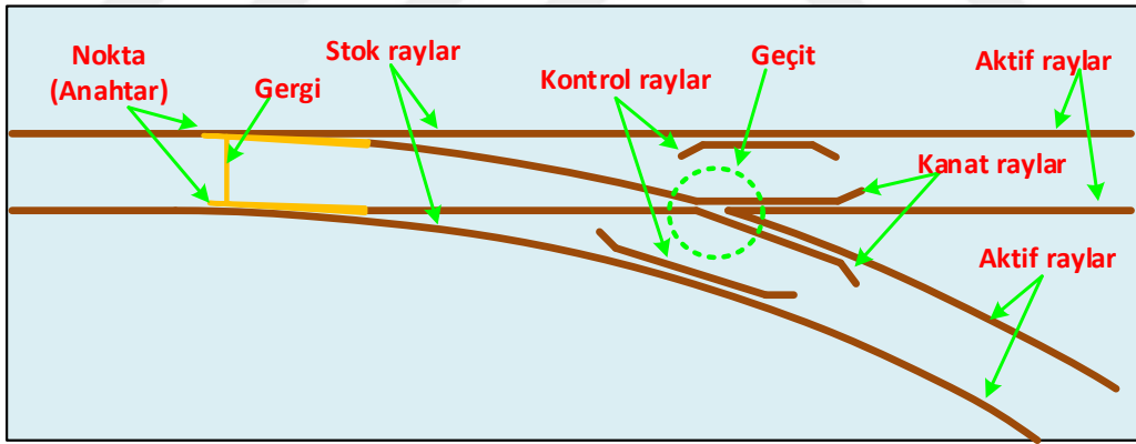
Şekil 2.5. Örnek bir makas geçiş sistemi ve bileşenleri
