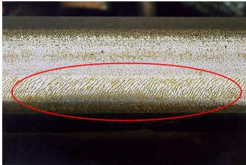
Şekil 2.18. Ray mantarının iç köşesinde oluşan kılcal çatlak görüntüsü [118].
