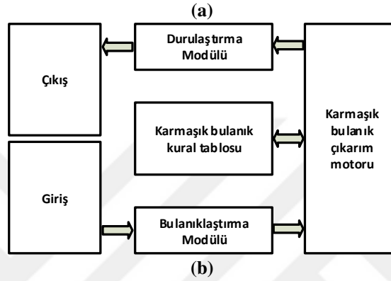
Şekil 3.15. Karmaşık bulanık kümesi ve mimarisi (a) Karmaşık bulanık kümeler (b) Karmaşık bulanık sistemin mimarisi [152].
