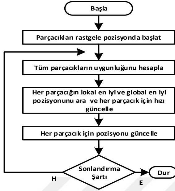
Şekil 4.17. PSO'nun akış diyagramı
