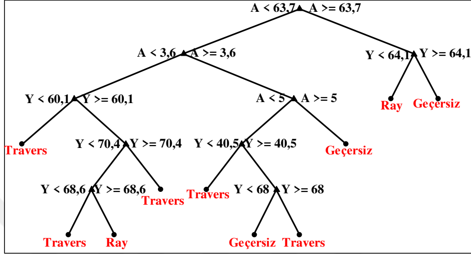
Şekil 4.10. Karar ağacı yapısı (A: Aç, Y: Yatay)
