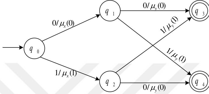
Şekil 3.12. Önerilen bulanık otomata yapısı
