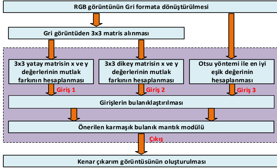
Şekil 3.16. Önerilen karmaşık bulanık mantık tabanlı yöntemin akış şeması
