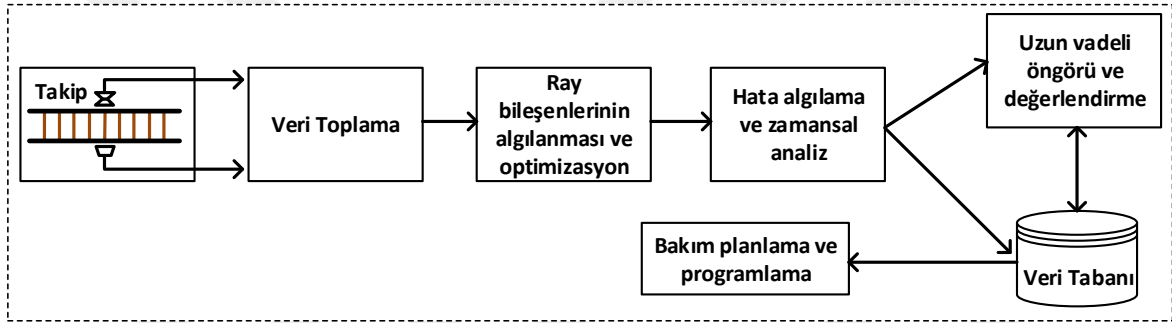
Şekil 1.7. Önerilen demiryolu denetim sisteminin genel mimarisi [37]
