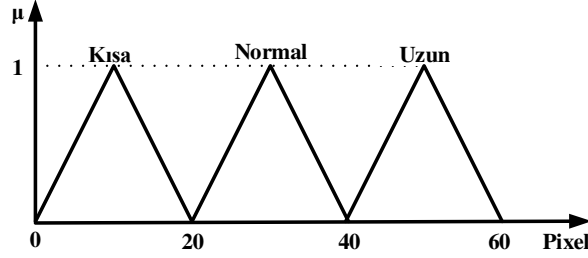
Şekil 6.12. İki ray arası mesafenin izlenmesi için önerilen çıkış üyelik fonksiyonu
