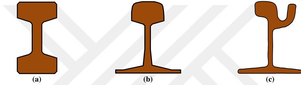
Şekil 2.2. Demiryolu rayları (a) Çift mantarlı ray (b) Tek mantarlı patenli ray (c) Oluklu patenli ray
