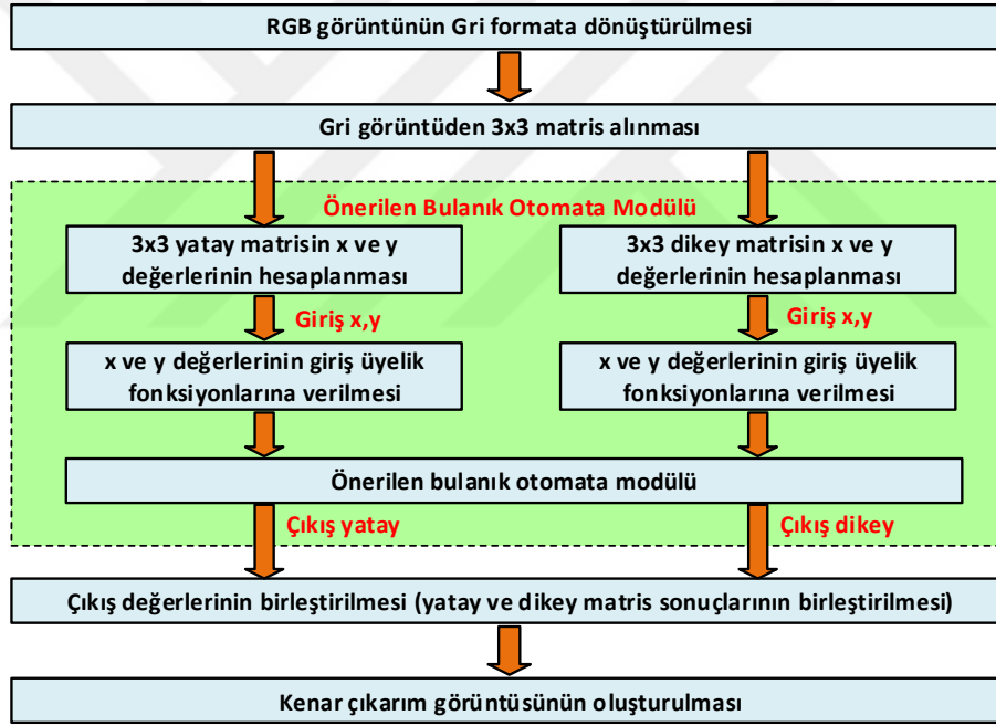
Şekil 3.11. Bulanık otomata tabanlı kenar çıkarım yöntemi
