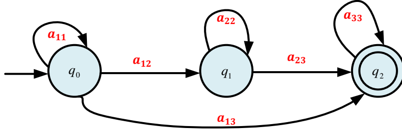
Şekil 3.10. Otomata ile ayrık bir olay sistemin modellenmesi
