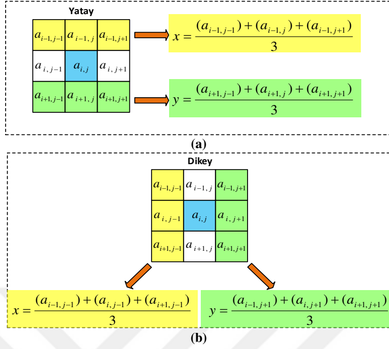
Şekil 3.6. Gri görüntüden alınan 3 \times 3 boyutundaki matrisler (a) Yatay hesaplama (b) Dikey hesaplama
