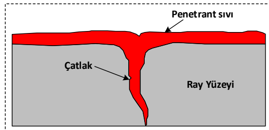
Şekil 2.31. Penetrant sıvısının uygulanması
