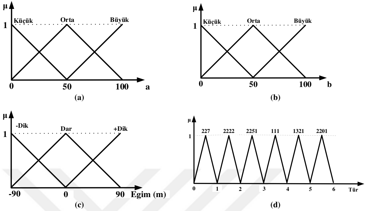
Şekil 5.13. Giriş ve çıkış üyelik fonksiyonları
