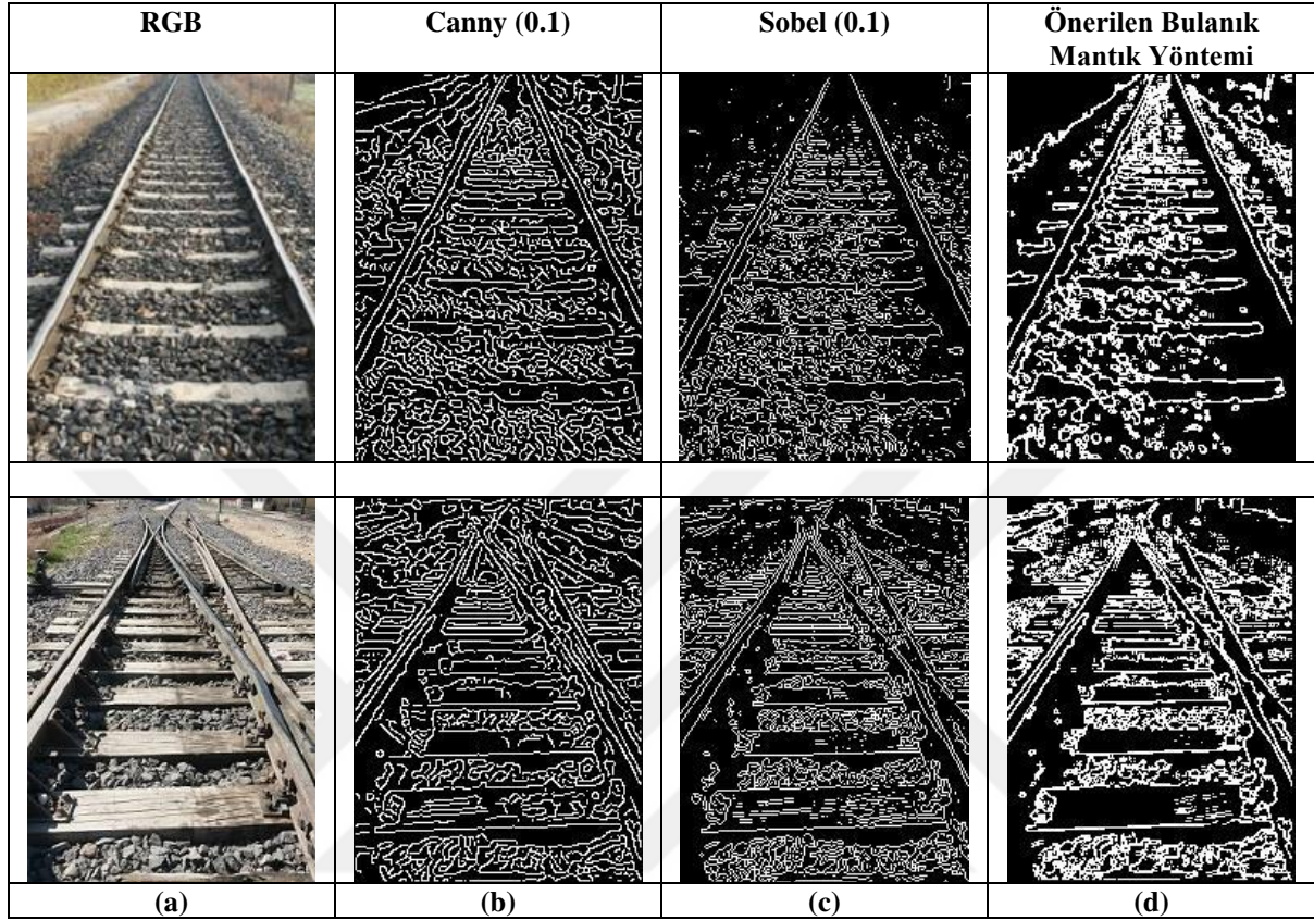
Şekil 3.8. Önerilen yöntem için kullanılan örnek görüntüler ve sonuçları (a) RGB görüntü (b) Canny kenar çıkarımı (0.1) (c) Sobel kenar çıkarımı (0.1) (d) Önerilen bulanık mantık tabanlı kenar çıkarımı
