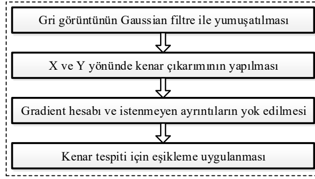
Şekil 4.7. Canny kenar çıkarım algoritmasının akış şeması [165].
