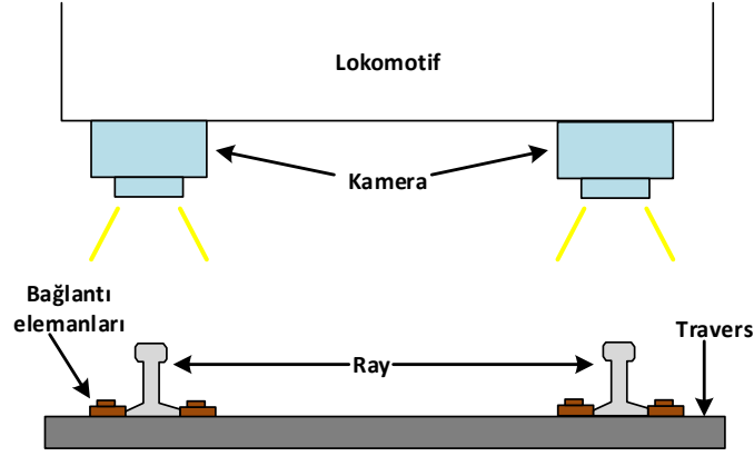
Şekil 1.5. Önerilen yöntemde kullanılan deneysel düzenek [34]
