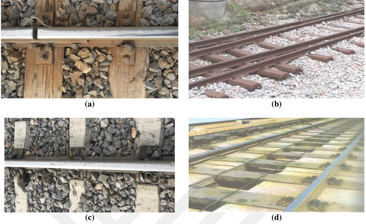
Şekil 2.3. Demiryolu travers türleri (a) Ahşap travers (b) Demir travers (c) Beton travers (d) Plastik travers
