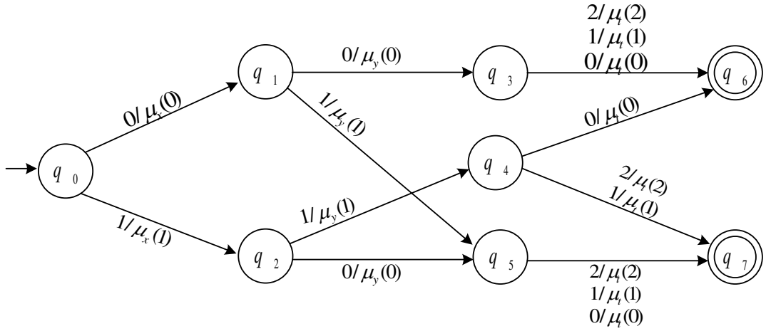
Şekil 3.21. Önerilen karmaşık bulanık otomata yapısı
