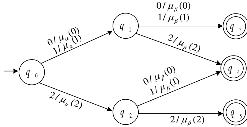
Şekil 6.21. Önerilen karmaşık bulanık otomata yapısı
