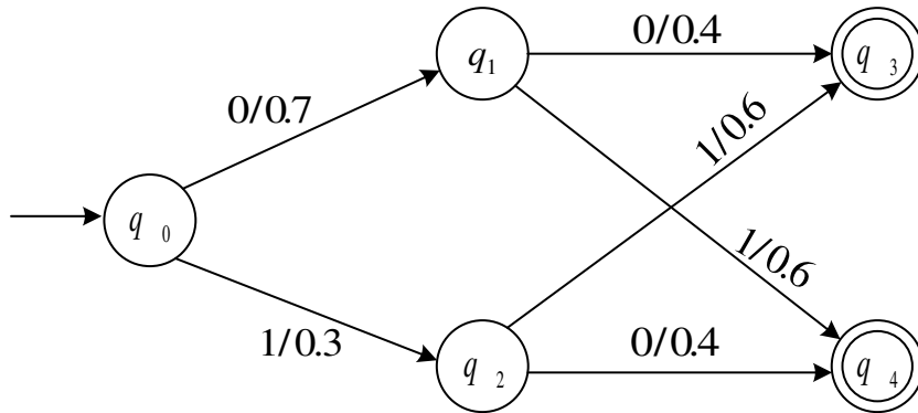
Şekil 3.13. Bulanık otomata geçiş diyagramı
