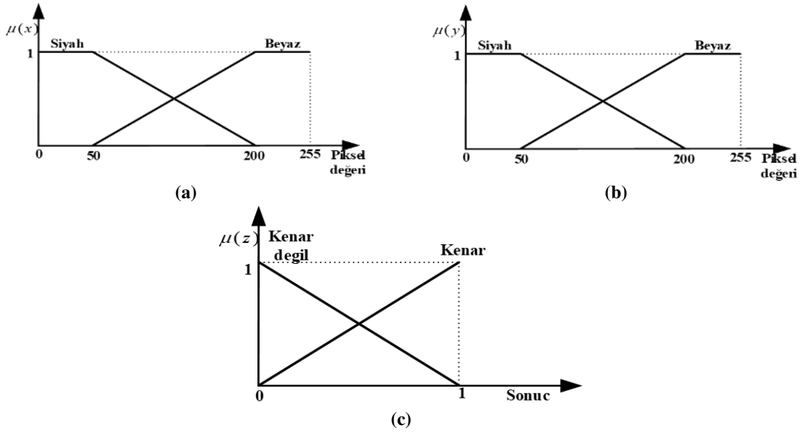
Şekil 3.7. Önerilen yöntemde kullanılan üyelik fonksiyonları (a) Giriş üyelik fonksiyonu (b) Giriş üyelik fonksiyonu (c) Çıkış üyelik fonksiyonu
