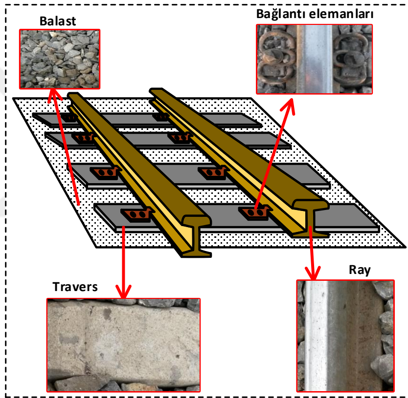
Şekil 2.1. Demiryolu hattının genel bileşenleri
