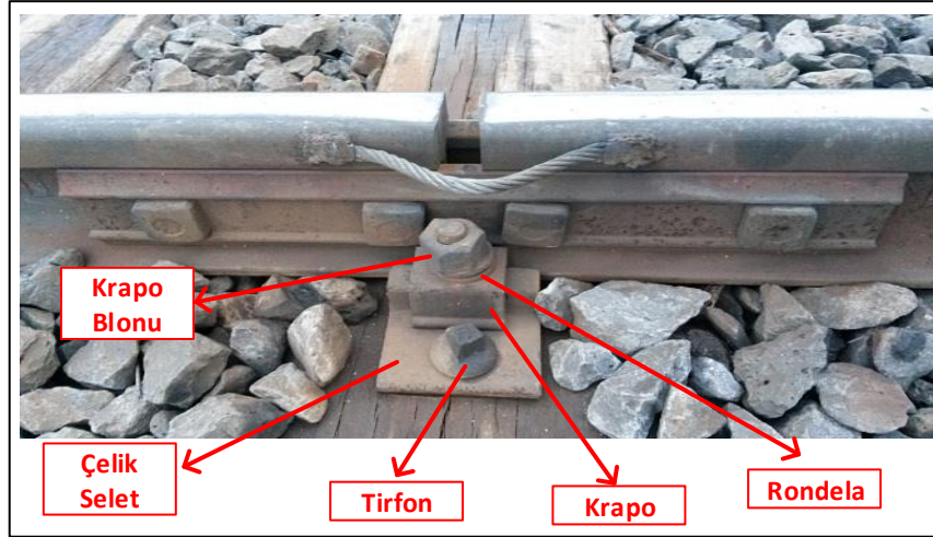
Şekil 2.7. Rayı traverse bağlayan bağlantı malzemeleri
