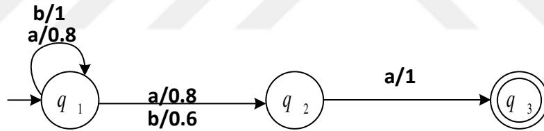
Şekil 3.9. Bulanık otomata için örnek geçiş diyagramı
