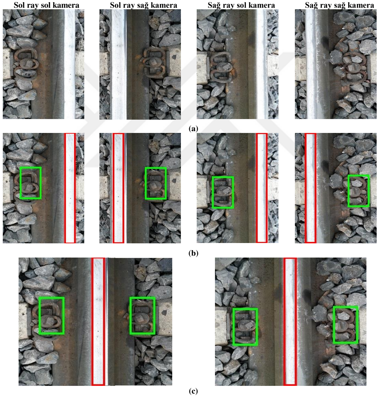
Şekil 4.21. Beton traverse sahip olan demiryolu hattından alınan görüntüler ve bu görüntülere önerilen yöntemin uygulanması (a) Dört kameradan alınan görüntüler (b) Görüntüler üzerinde ray yüzeyi
