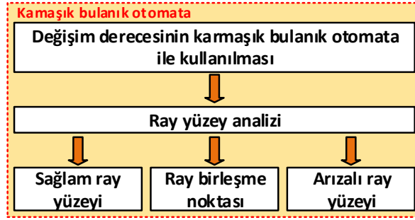
Şekil 6.19. Önerilen karmaşık bulanık otomata akış şeması
