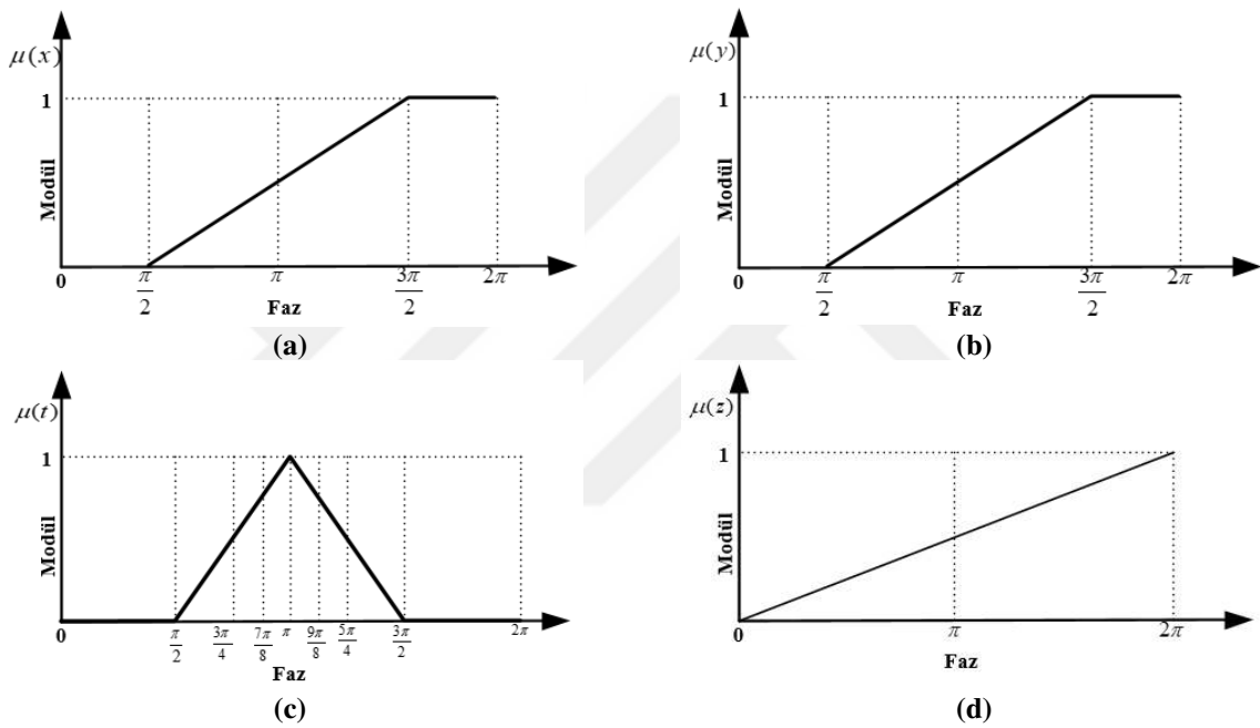
Şekil 3.18 Önerilen yöntemde kullanılan üyelik fonksiyonları (a) Giriş üyelik fonksiyonu (b) Giriş üyelik fonksiyonu (c) Giriş üyelik fonksiyonu (d) Çıkış üyelik fonksiyonu
