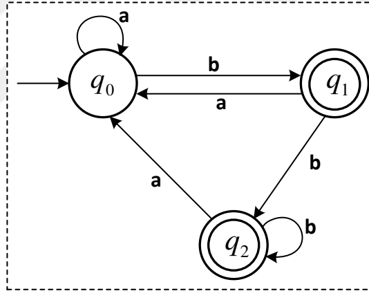
Şekil 3.2. Örnek bir sonlu durum otomatın geiş diyagramı
