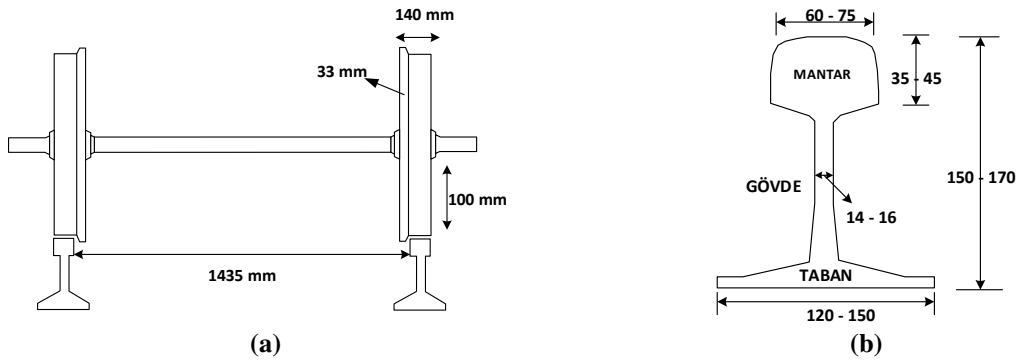
Şekil 4.2. Gerçek bir demiryolu tekerinin ve rayın ölçüleri (a) İki ray arası mesafe ve teker ölçüleri (b) Rayın ölçüleri
