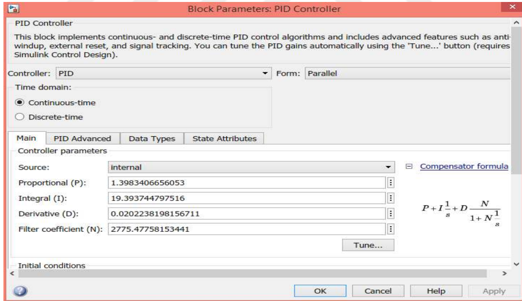
Şekil 5.20. PID parametre değerleri
