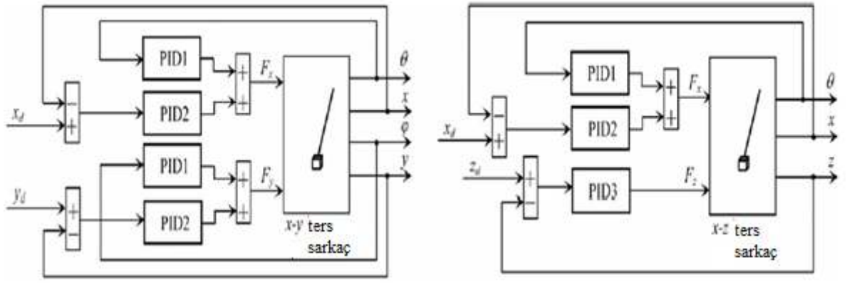
Şekil 2.13. İki ve üç kontrolörlü ters sarkaç tasarımı [22].
