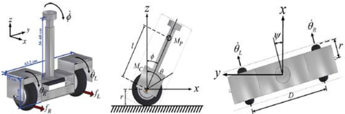
Şekil 2.14. İki tekerlekli bir ters sarkaç sistemi [23].
