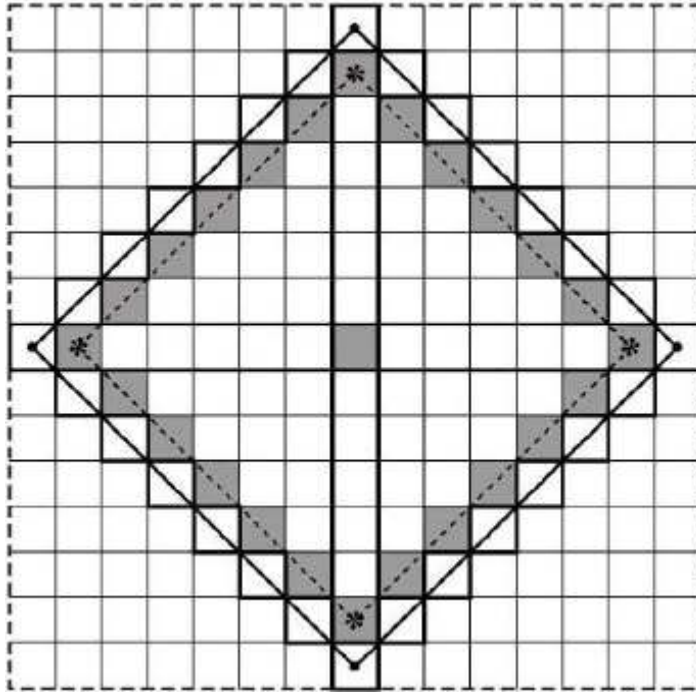
Şekil 2.4 M_{\mu} ve M_{\mu-2} İç Merdivenli Çerçeveler
