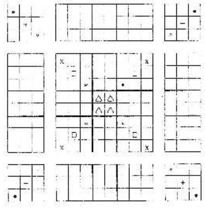
Şekil 2.3 Karenin Çerçevelerinin Sıralanması veya Derecelenmesi
