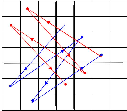
\alpha_5 ve \beta_5 Grafikleri
