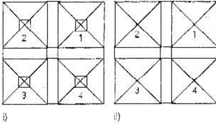
Şekil 3.5 Tek dereceden karenin özel bölgeleri
