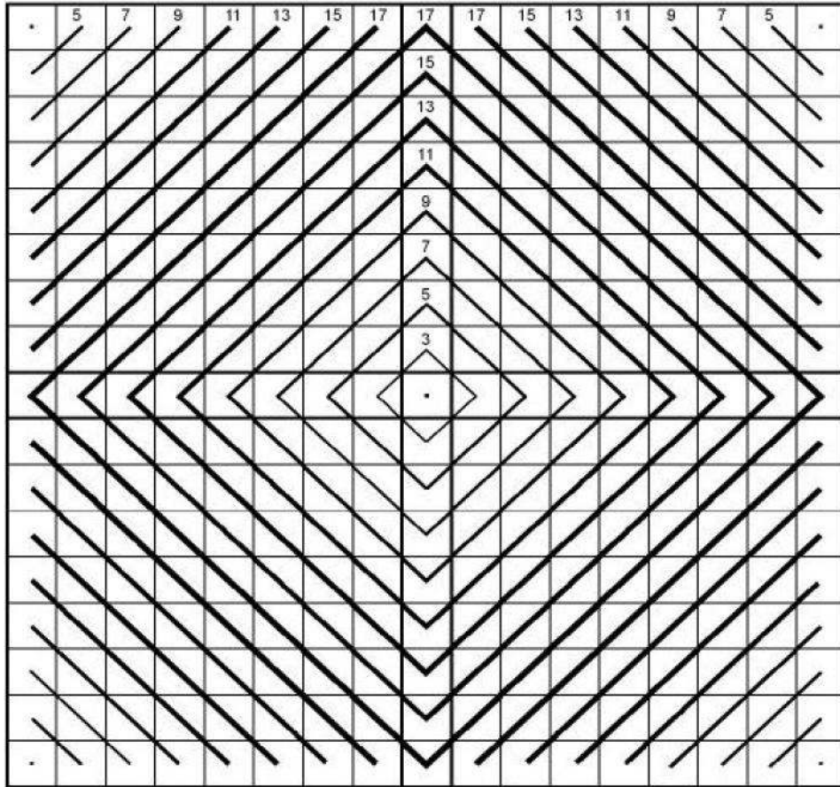
Şekil 2.5 17.Dereceden Karenin İç ve Dış Merdivenli Çerçeveleri
