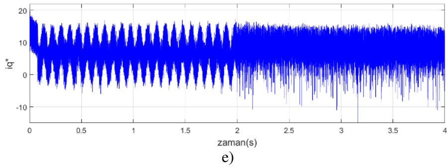
Şekil 7.5. 300 rad/s Hızda 5 Nm sabit ve 2.5 Nm dengesiz yükte t=2 s’de yöntemin devreye alınması durumunda benzetim sonuçları a)Motor Hızı b)Motor Momenti c)iabc akımları d)Idq eksen akımları e)Harmonikli iq akımı
