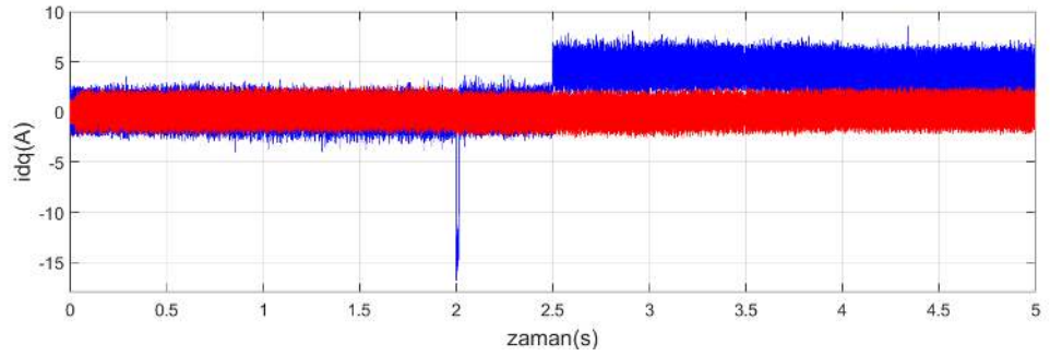
Şekil 7.4. Hızın 100 rad/s ile -50 rad/s arasında ani ve doğrusal değişimi ve yüksüz durumdan t=2.5 s’de T_y=5 Nm’ye değişmesi durumunda benzetim sonuçları a)Motor Hızı b)Motor Momenti c)Iabc akımları d)Idq eksen akımları
