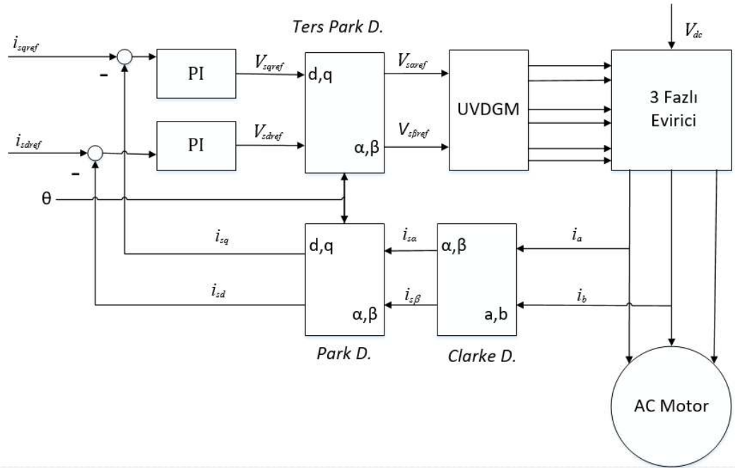
Şekil 3.3. SMSM' lerde AYK diyagramı (Akin ve Bhardwaj, 2010)
