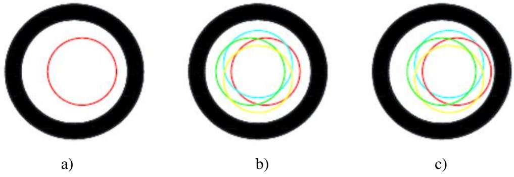
Şekil 5.1. Eksen kaçıklığı a)Statik eksen kaçıklığı b)Dinamik eksen kaçıklığı c)Karma eksen kaçıklığı (Kara, 2017)
