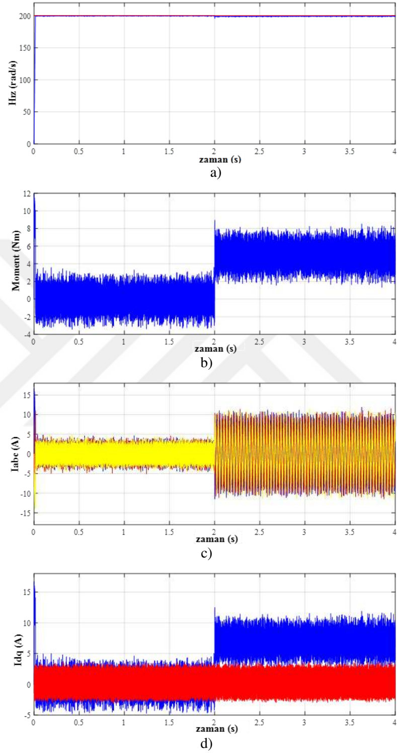
Şekil 7.2. 200 rad/s sabit hızda t=2 s’de yüksüz durumdan T_y=5\text{Nm} ’ye değişmesi durumunda benzetim sonuçları a)Motor hızı b) Motor Momenti c) Iabc akımları d)Idq akımları
