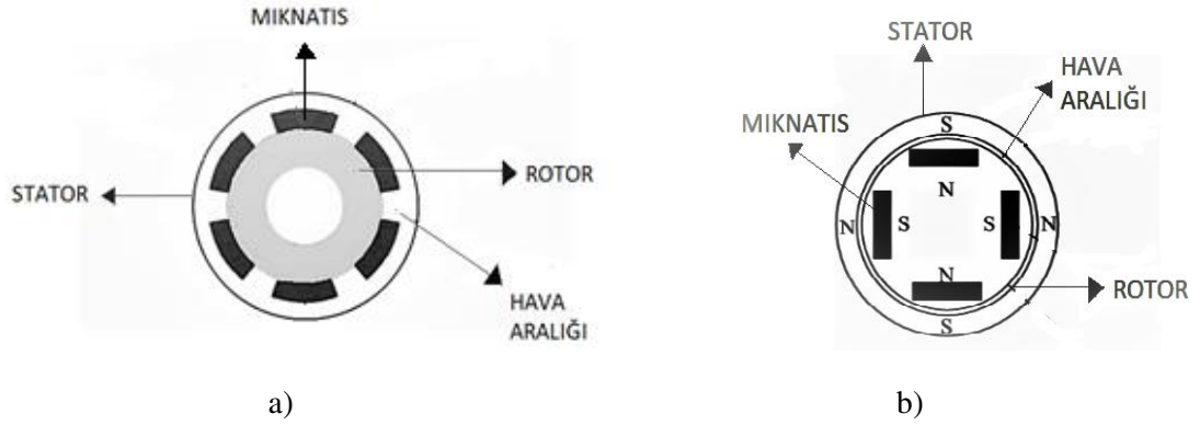
a) Yüzey mıknatıslı SMSM, b) İçten mıknatıslı SMSM
