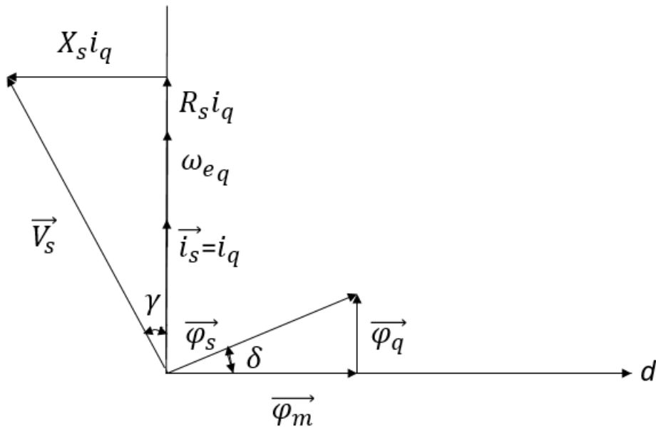
Şekil 3.4. AYK durum vektör diyagramı (Çelik ve Kürüm, 2012)
