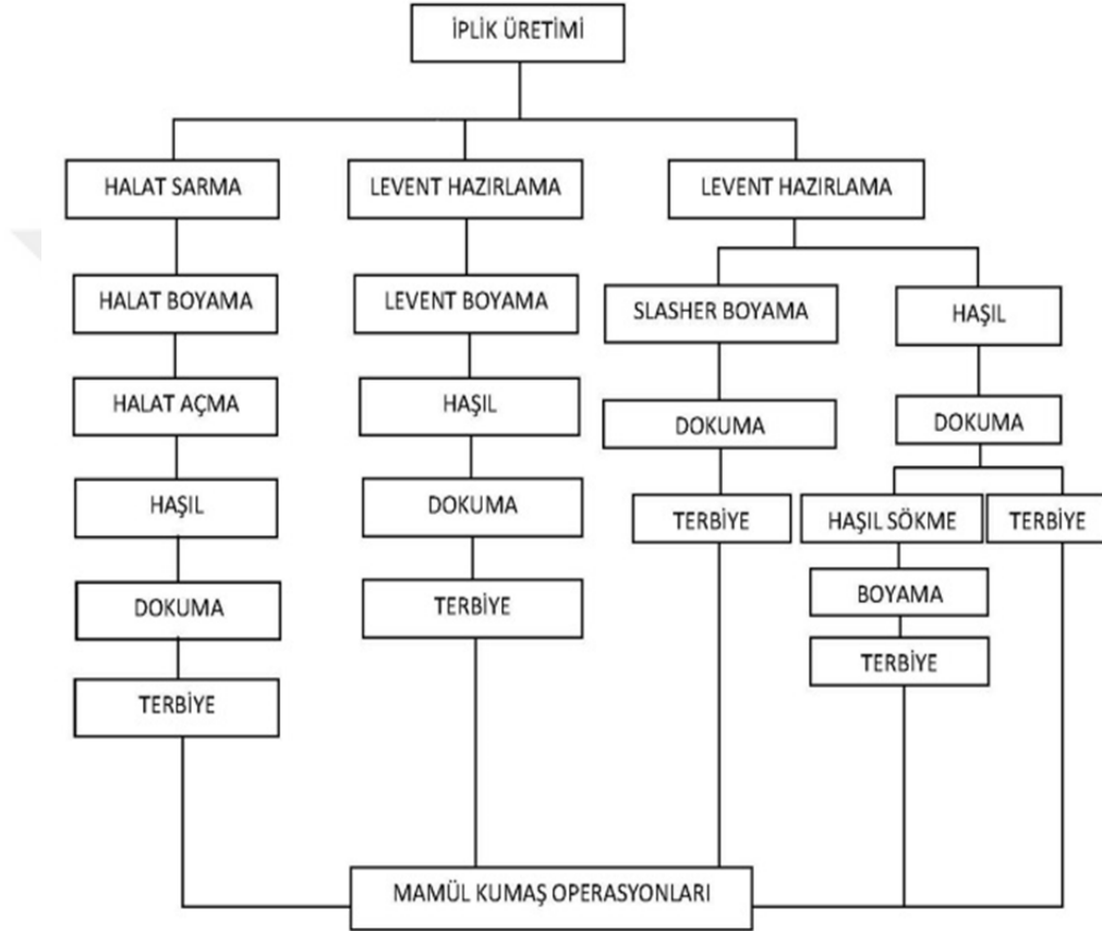
Şekil 3.3. Denim kumaş üretimi akış şeması (Çataloğlu, 2007)
