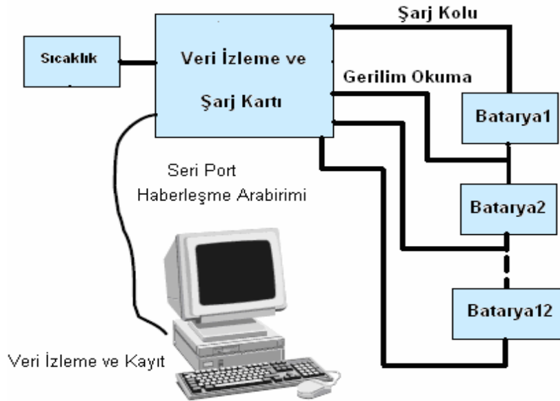
Şekil 2.4 Veri İzleme ve Şarj Sistemi Blok Diyagramı
