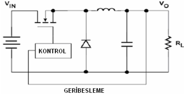
Şekil 3.3 Buck dönüştürücü
