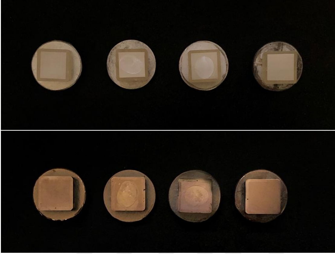
Resim 3.36. Seçilen PEKK test örneklerinin altın-palladyum film tabakasıyla kaplanması
