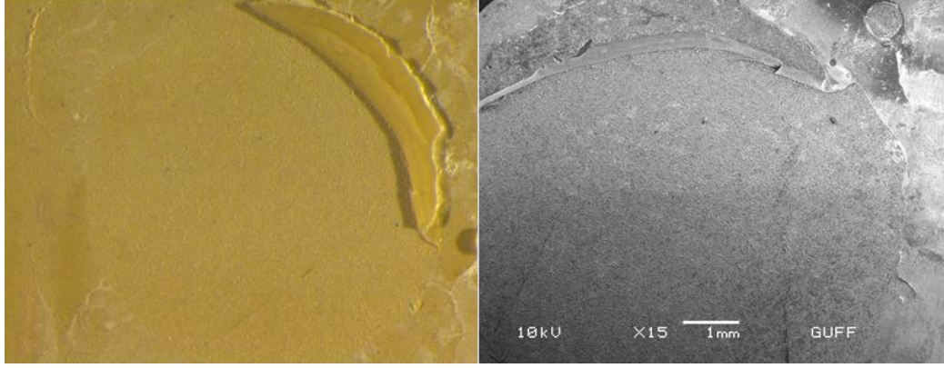
Resim 4.9. ATC+ grubu ışık mikroskobu ve SEM görüntüsü-ARI 1 skor (6. test örneği)
