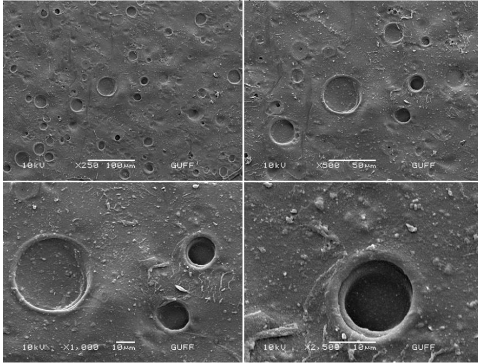
Resim 4.3. C grubuna ait iki test örneğinin x250, x500, x1000, x2500 büyütmede SEM görüntüsü
