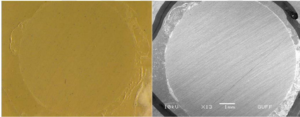
Resim 4.18. DTC- grubu ışık mikroskobu ve SEM görüntüsü-ARI 0 skor (6. test örneği)
