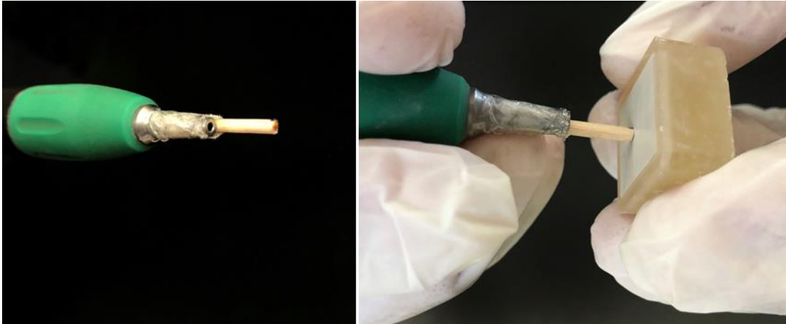
Resim 3.24. PEKK test örneğinin yüzeyi ile kumlama cihazının ucu arasındaki mesafenin her bir test örneği için sabitlenmesi
