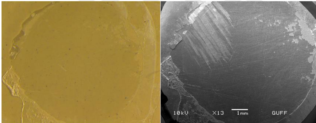
Resim 4.15. BTC- grubu ışık mikroskobu ve SEM görüntüsü-ARI 0 skor (10. test örneği)
