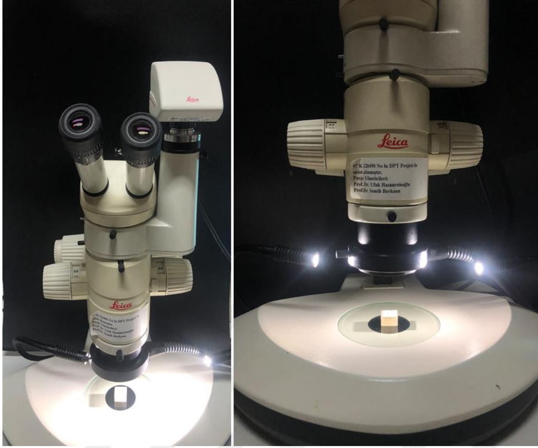
Resim 3.58. Işık mikroskobu ve test örneklerinin kırık yüzeylerinin incelenmesi
