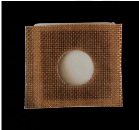
Resim 3.38. PEKK test örneği ve teflon kumaşa açılan dairesel delikler ile belirlenen bağlantı yüzeyi
