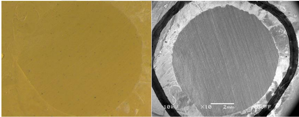
Resim 4.13. DTC+ grubu ışık mikroskobu ve SEM görüntüsü-ARI 0 skor (4. test örneği)
