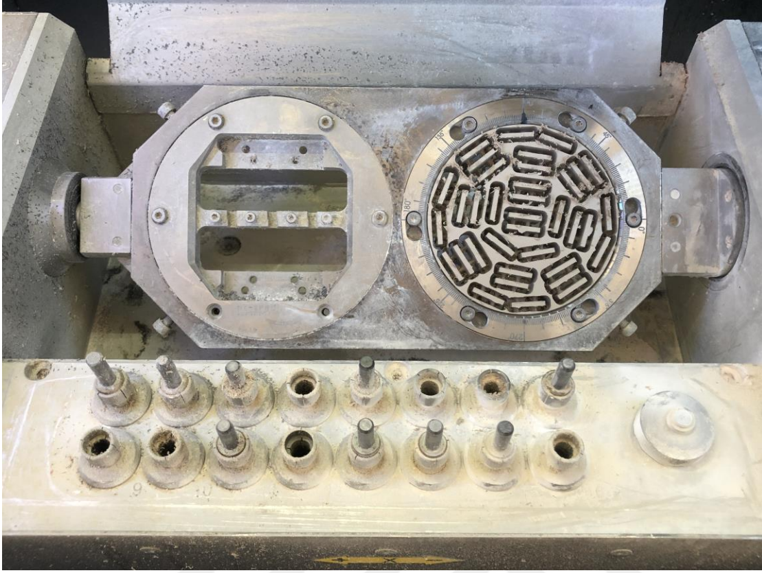
Resim 3.5. Kazıma işlemi sonrası CAD/CAM içinde PEKK diski
