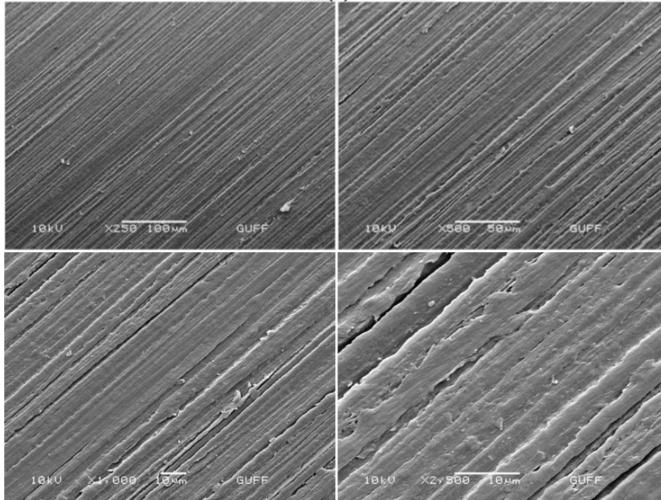
Resim 4.5. D grubuna ait iki test örneğinin x250, x500, x1000, x2500 büyütmede SEM görüntüsü
