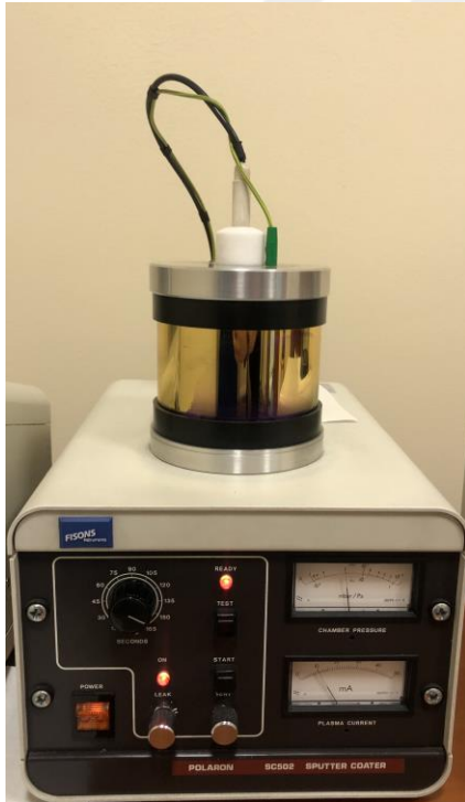
Resim 3.35. Altın-palladyum kaplama ünitesi
