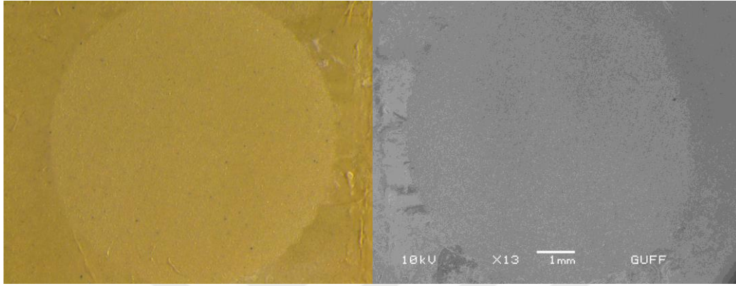
Resim 4.6. ATC+ grubu ışık mikroskobu ve SEM görüntüsü-ARI 0 skor (9. test örneği)
