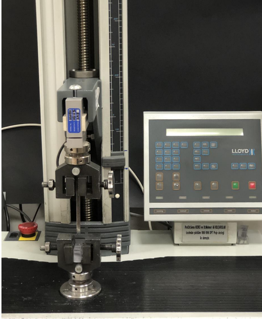
Resim 3.56. Universal test cihazı
