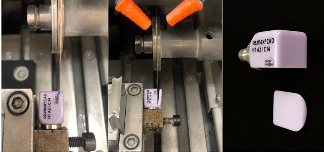
Resim 3.11. Dikey kesim sonucu elde edilen lityum disilikat cam seramik CAD/CAM blok
