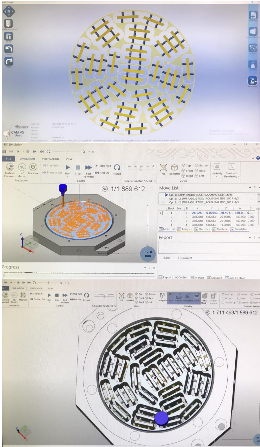
Resim 3.2. PEKK test örneklerinin CAD/CAM simülasyonu
