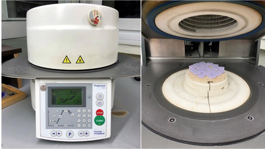
Resim 3.13. Porselen fırını ve içerisindeki lityum disilikat cam seramik test örnekleri
