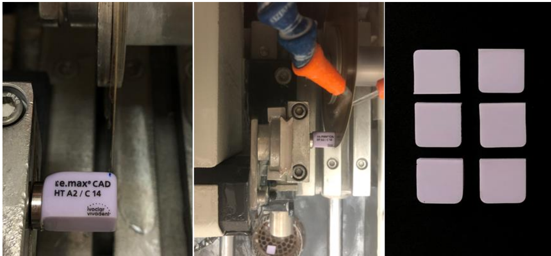
Resim 3.12. Yatay kesitler alınarak elde edilen lityum disilikat cam seramik test örnekleri
