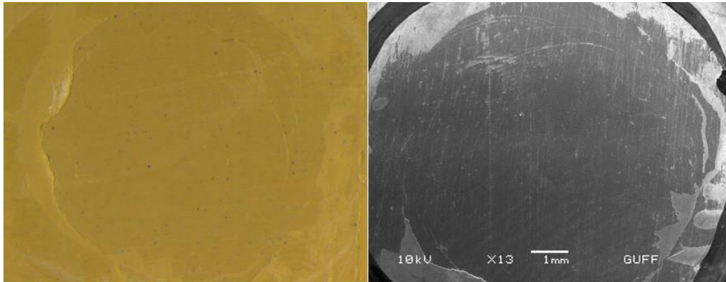
Resim 4.11. BTC+ grubu ışık mikroskobu ve SEM görüntüsü-ARI 1 skor (5. test örneği)
