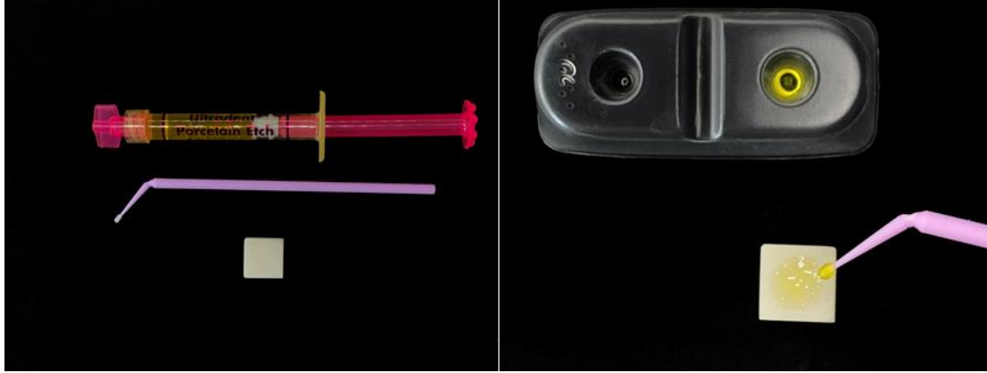
Resim 3.42. Lityum disilikat cam seramik test örneklerinin bağlantı yüzeylerine hidroflorik asit uygulanması
