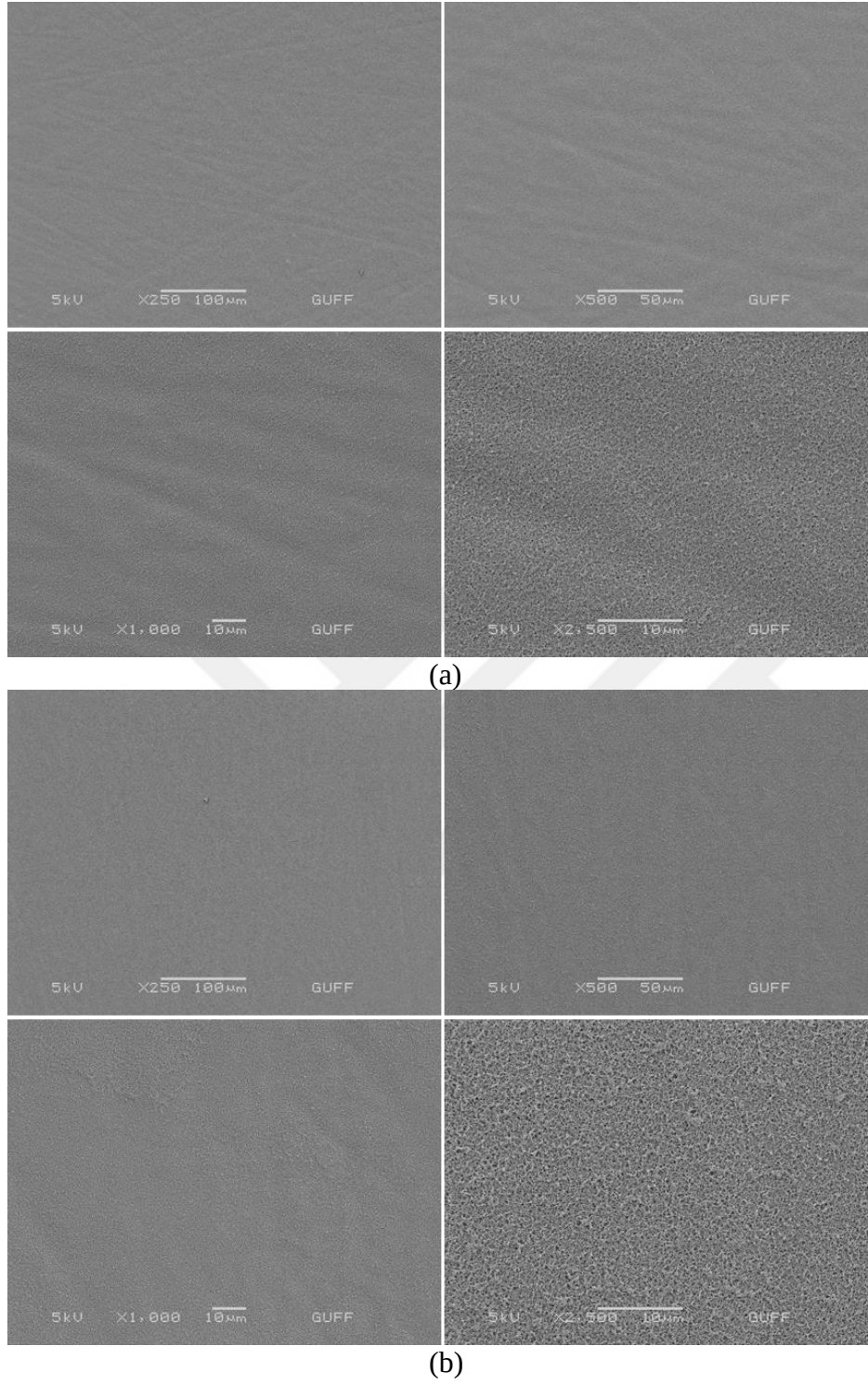
Resim 4.2. B grubuna ait iki test örneğinin x250, x500, x1000, x2500 büyütmede SEM görüntüsü
