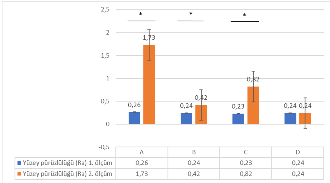
Şekil 4.1. 1. ölçüm ve 2. ölçüm yüzey pürüzlülük değerleri
