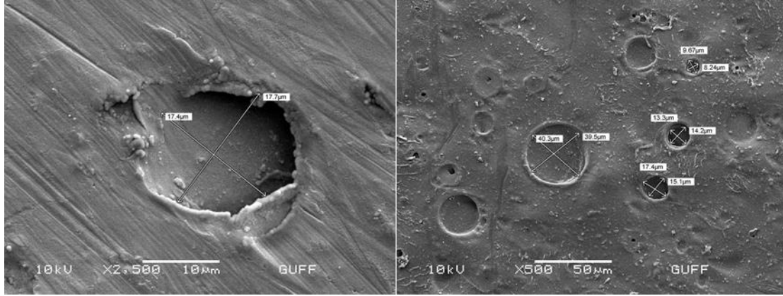
Resim 4.4. C grubuna ait iki test örneğinin gözenek büyüklüğünün ölçülmesi
