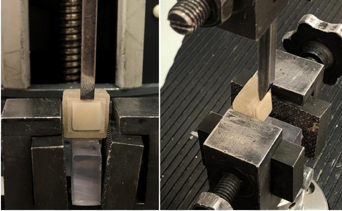
Resim 3.57. Universal test cihazının metal ucunun konumlandırılması
