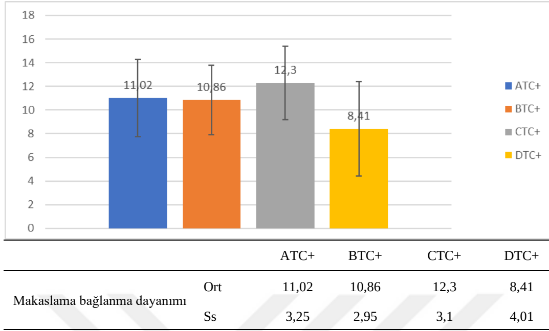
Şekil 4.5. Termal döngü uygulanan grupların makaslama bağlanma dayanımı değerleri ve standart sapma sonuçları grafiği
