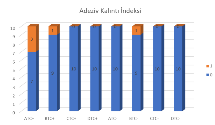
Şekil 4.6. Makaslama bağlanma dayanımı testi sonucunda oluşan ve ışık mikroskobu ile belirlenen başarısızlık tipi skorlaması grafiği
