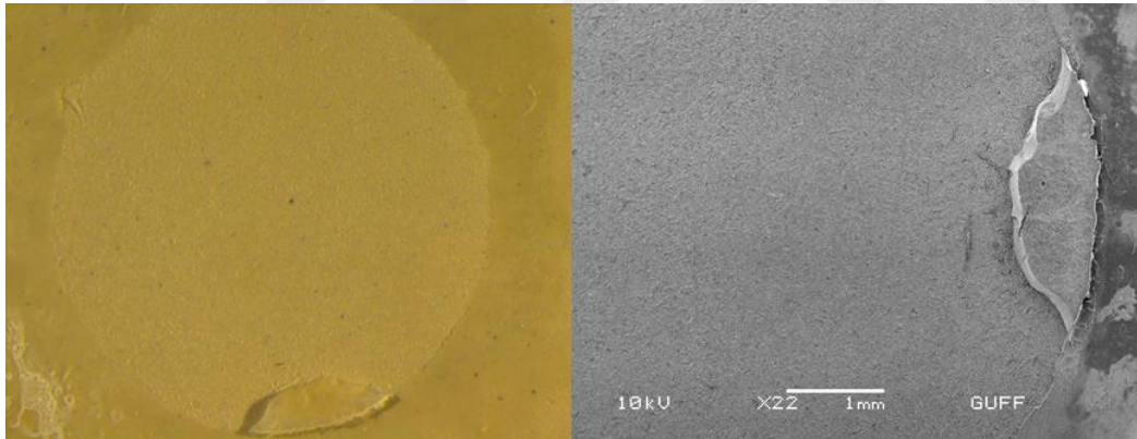
Resim 4.7. ATC+ grubu ışık mikroskobu ve SEM görüntüsü-ARI 1 skor (4. test örneği)
