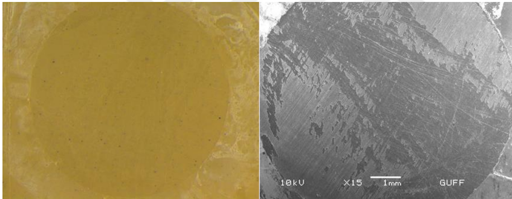
Resim 4.10. BTC+ grubu ışık mikroskobu ve SEM görüntüsü-ARI 0 skor (2. test örneği)
