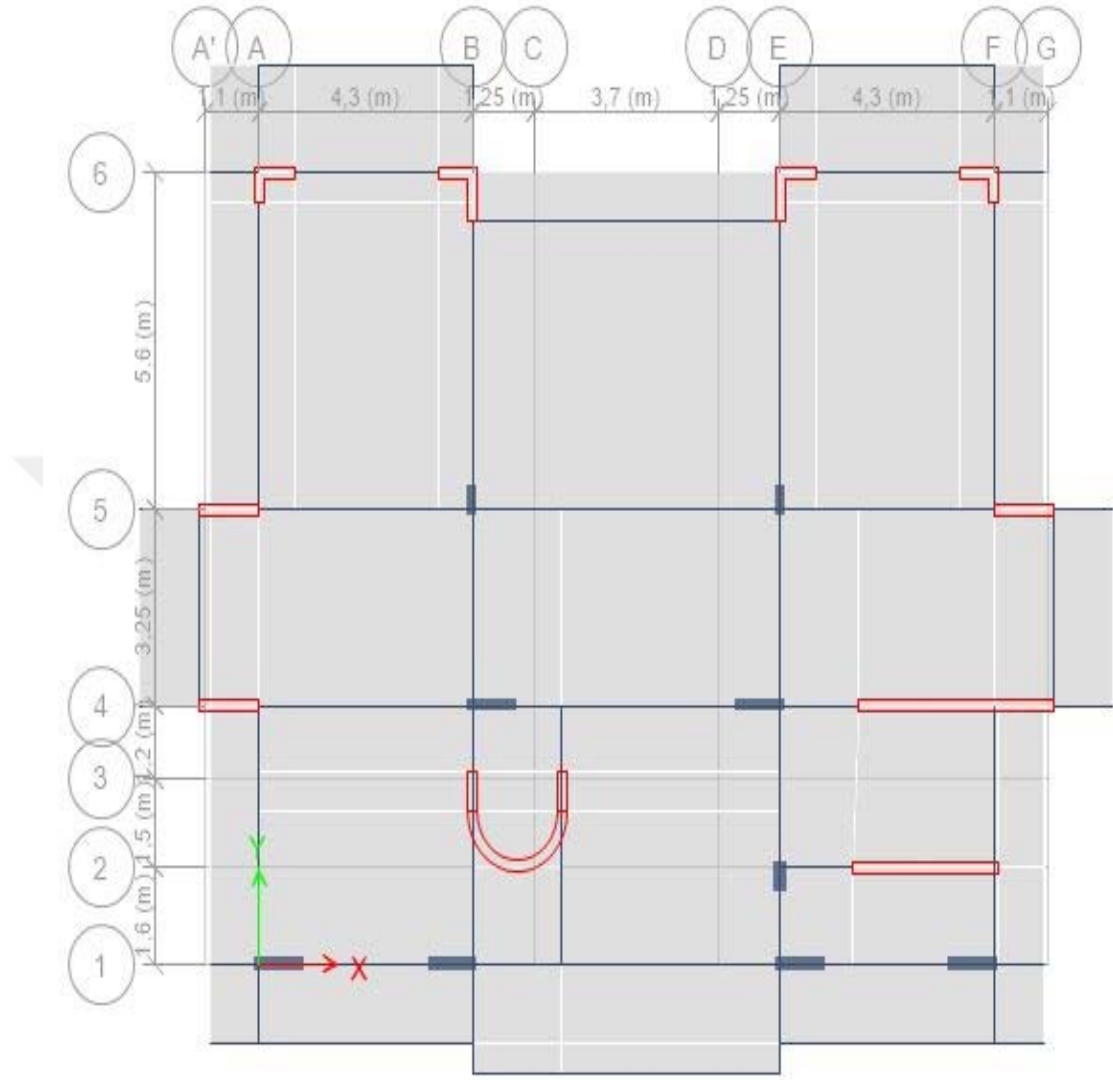
Şekil A.4 : Binanın normal kat modeli.
