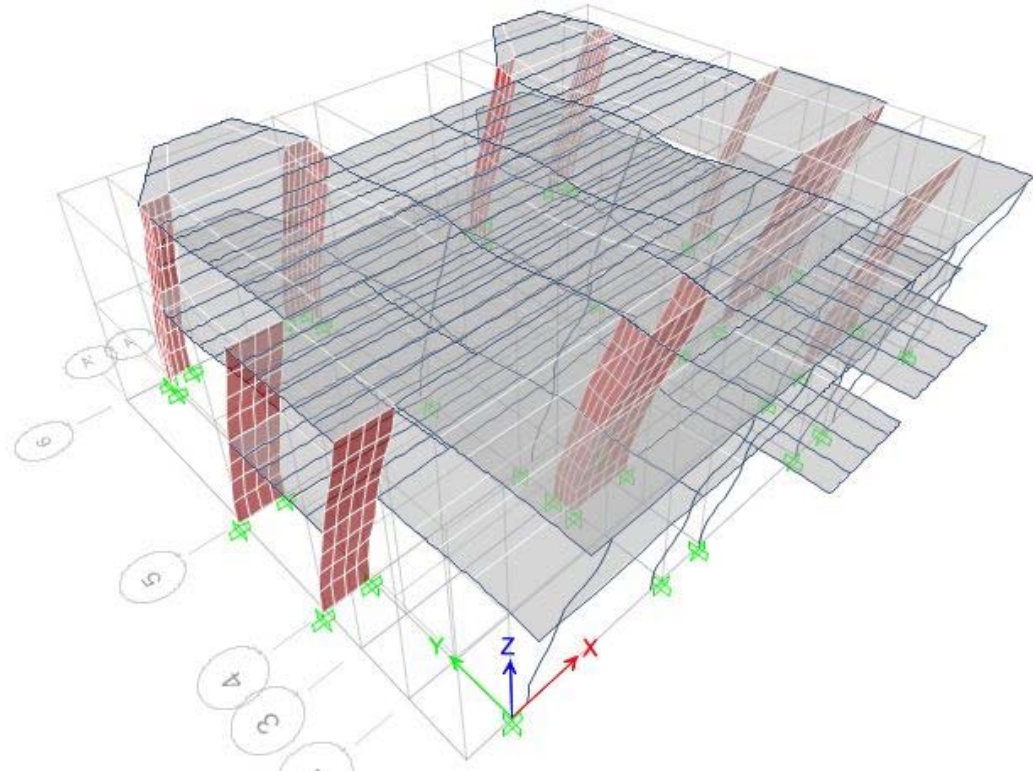
Şekil D.10 : RBTE binanın Y doğrultusu doğal periyodu.
