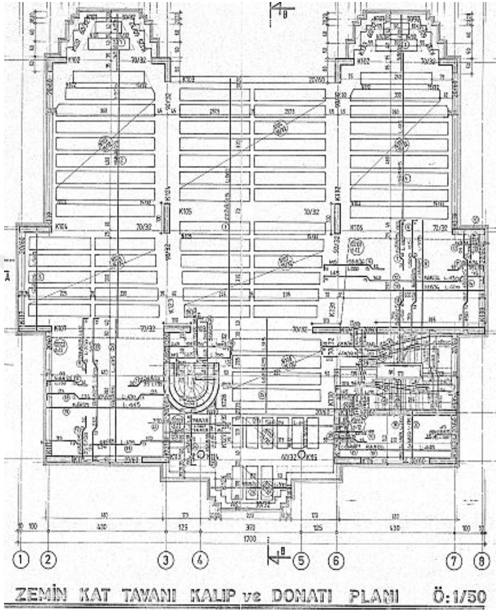
Şekil A.1 : Binanın zemin kat planı.
