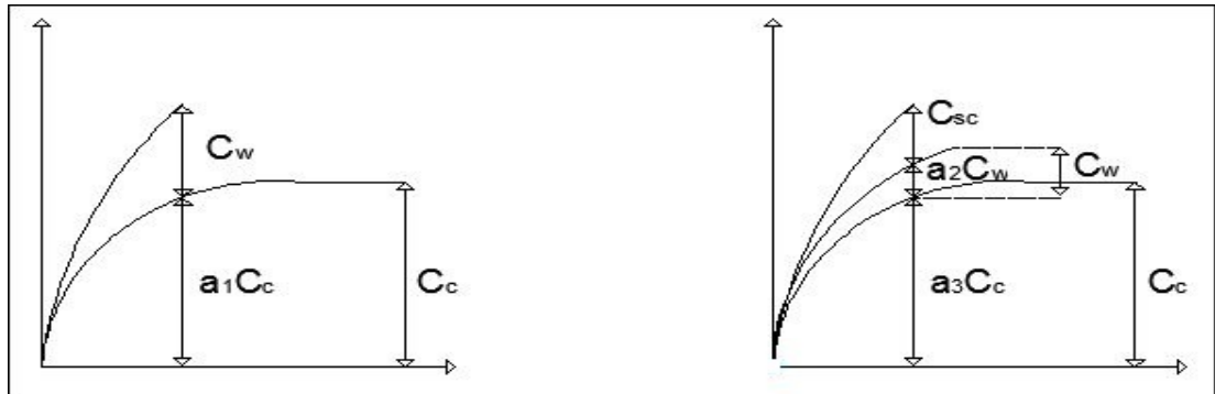
Şekil 3.2: Kat kesme kuvveti ve yer değiştirme ilişkisi.
