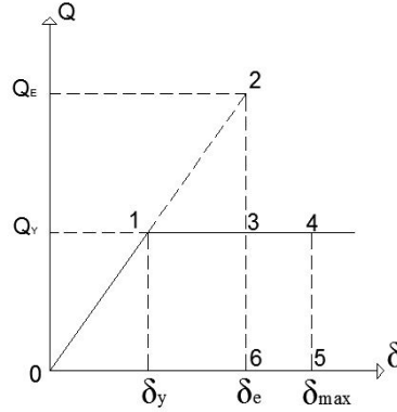
Şekil 3.1: Elastik ve elastoplastik kuvvet-yerdeğişme bağıllığı.
