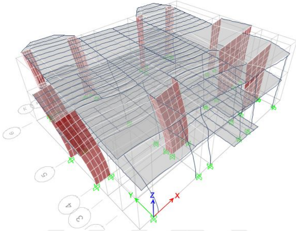
Şekil D.9 : RBTE binanın X doğrultusu doğal periyodu .
