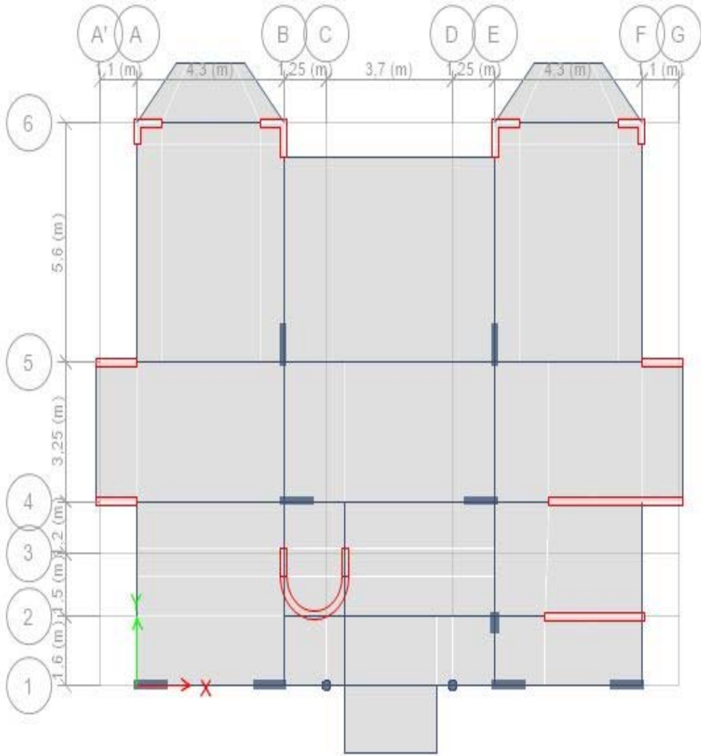
Şekil A.2 : Binanın zemin kat modeli.
