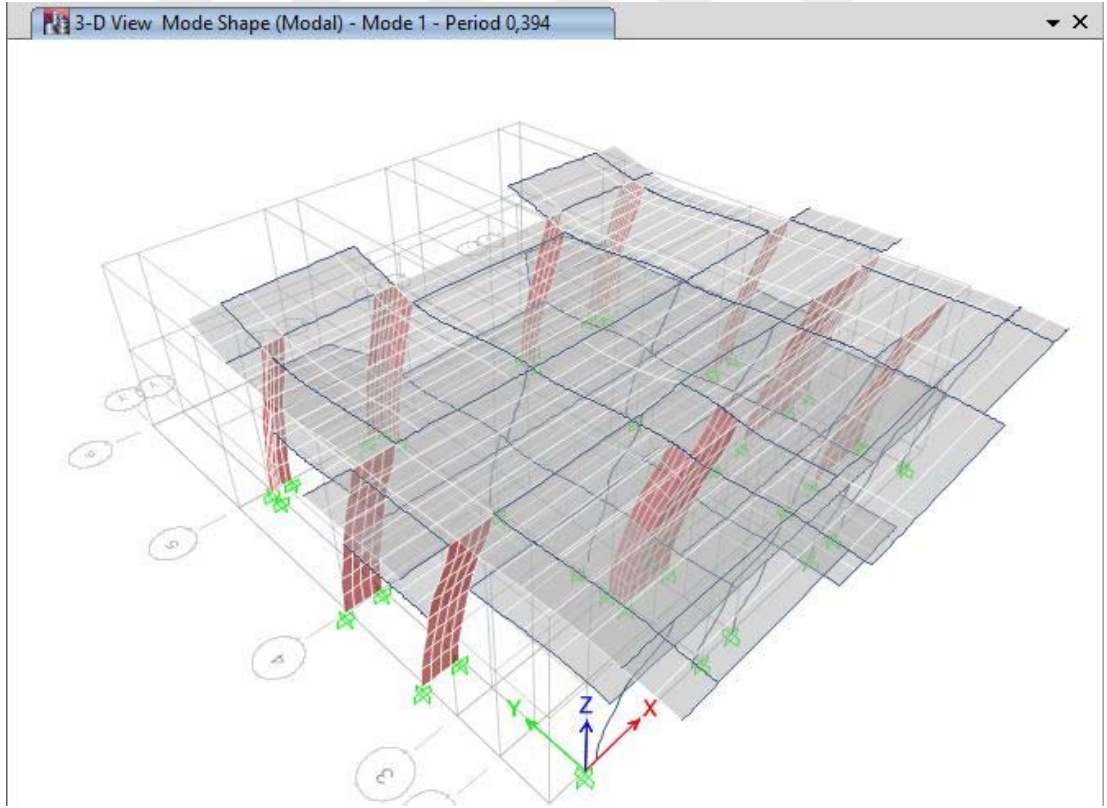
Şekil D.8 : DBYBHY binanın Y doğrultusu doğal periyodu .
