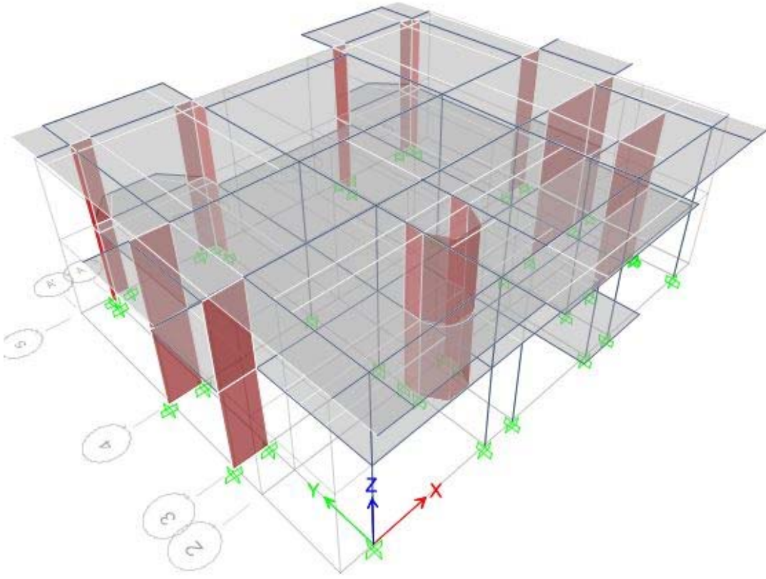
Şekil 4.1 : Yapının 3 boyutlu taşıyıcı sistem modeli.
