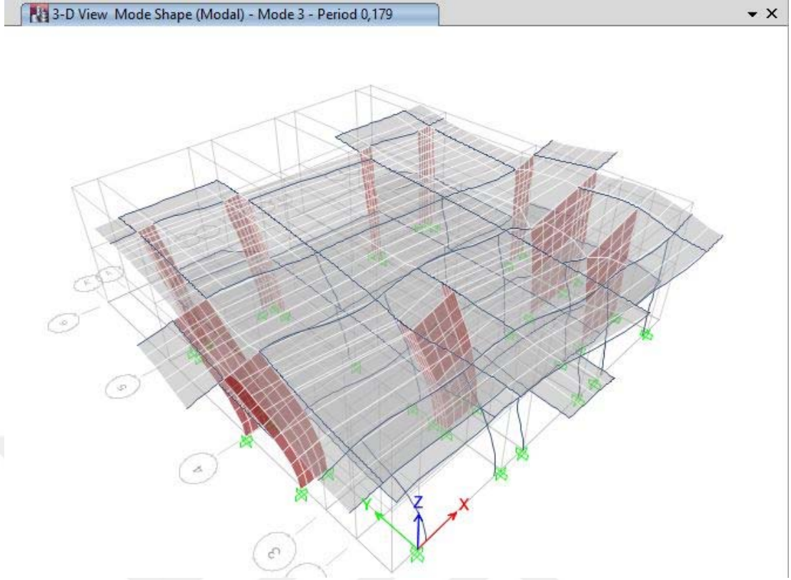
Şekil D.7 : DBYBHY binanın X doğrultusu doğal periyodu.
