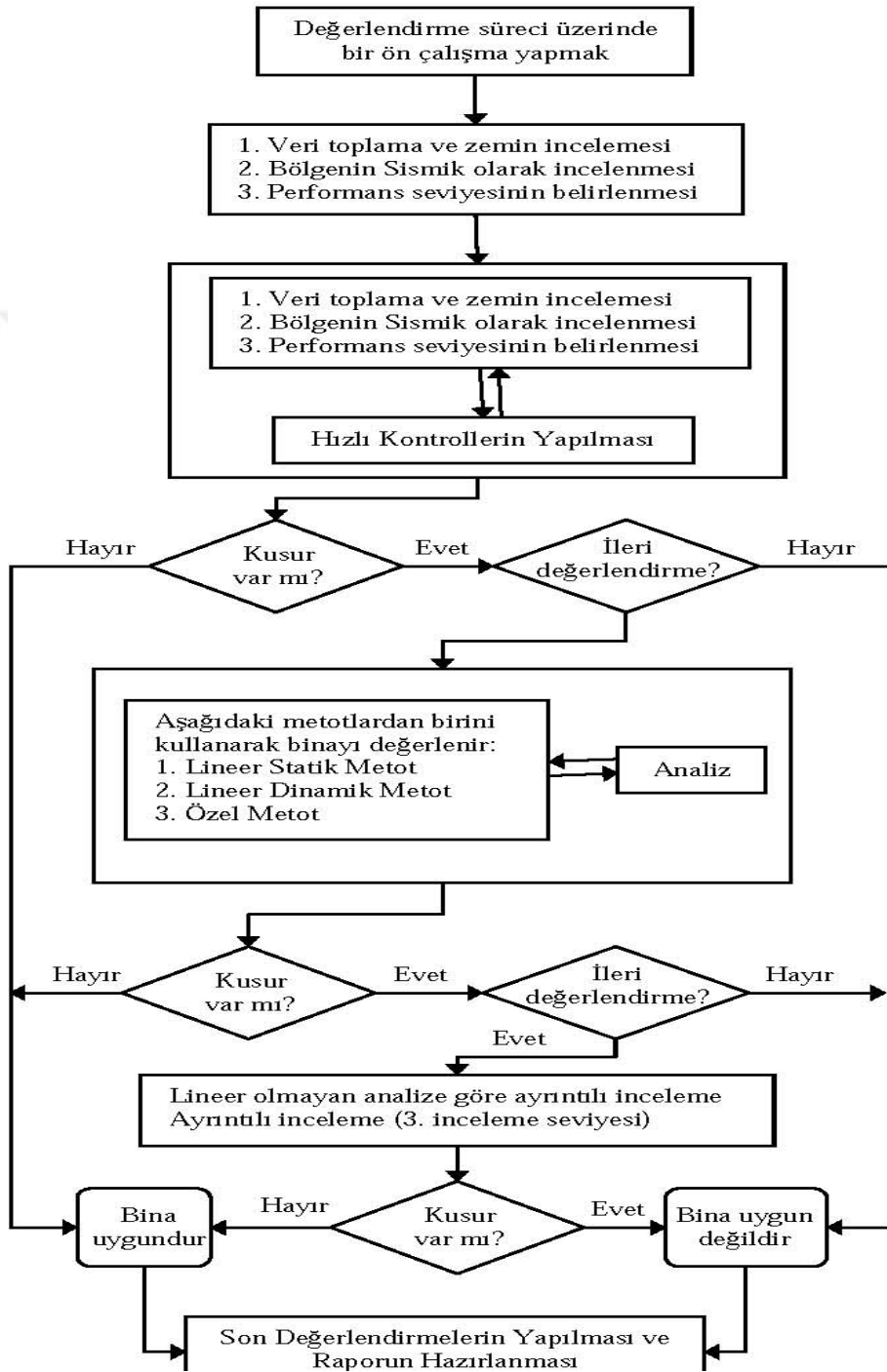
Şekil 2.1 : FEMA 310 için değerlendirme sürecini gösteren şema
