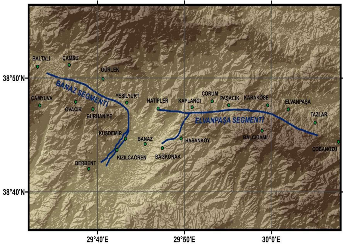
Şekil 5.1 Fay genel görünümü (Öztürk 2019).
