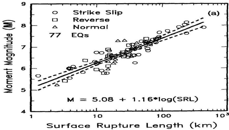
Şekil 2.10 Fay uzunluğu – fayın üretebileceği en büyük mangitüdlü deprem grafiği (Wells ve Coppersmith 1994).
