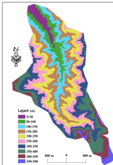
Şekil 13. Eriklimanı Havzası Yükselti Haritası
