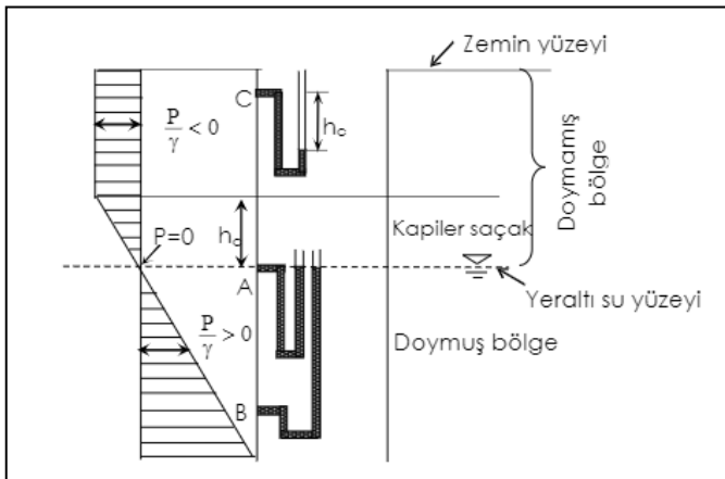
Şekil 12. Yer altı suyu bölgelerinin basınç değişimi
