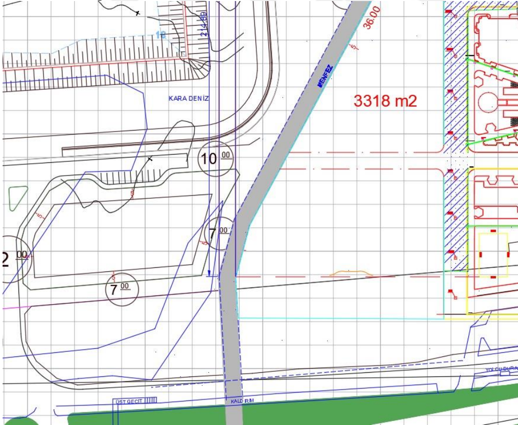
Ek 6. Menfez planı
