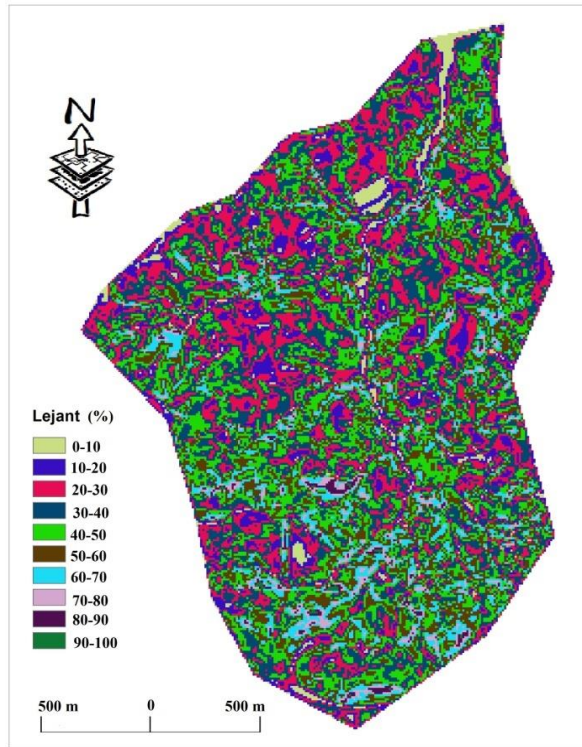
Şekil 16. Tersane havzası eğim haritası
