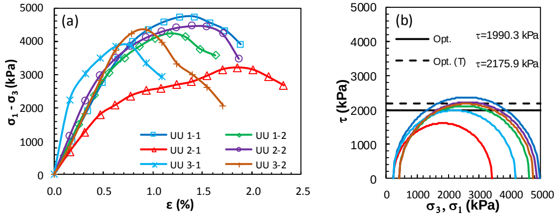
Şekil 4.83. Optimum tasarıma ait UU deney sonuçları: a) deviator gerilme-birim boy kısalması grafikleri, b) Mohr daireleri ile kırılma zarfları (Büyük ölçekli DKK, UU, 56 gün)
