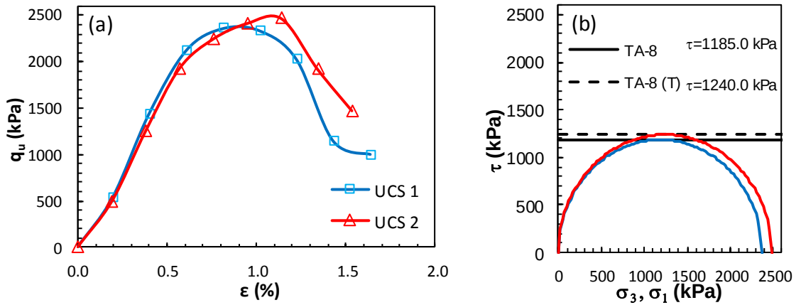
Şekil Ek 5.24. KÖ-8 numaralı tasarım: a) gerilme-birim deformasyon grafikleri ve b) Mohr daireleri (Küçük ölçekli DKK, UCS, 28 gün)
