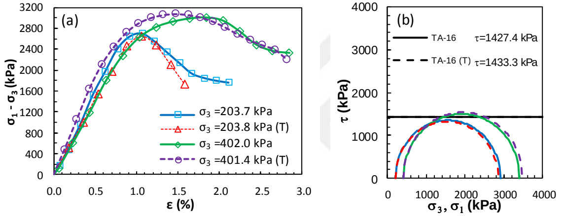
Şekil Ek 6.32. KÖ-16 numaralı tasarım: a) deviator gerilme-birim deformasyon grafikleri ve b) Mohr daireleri (Küçük ölçekli DKK, UU, 28 gün)
