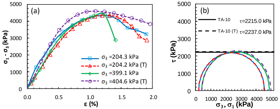
Şekil Ek 6.42. KÖ-10 numaralı tasarım: a) deviator gerilme-birim deformasyon grafikleri ve b) Mohr daireleri (Küçük ölçekli DKK, UU, 56 gün)
