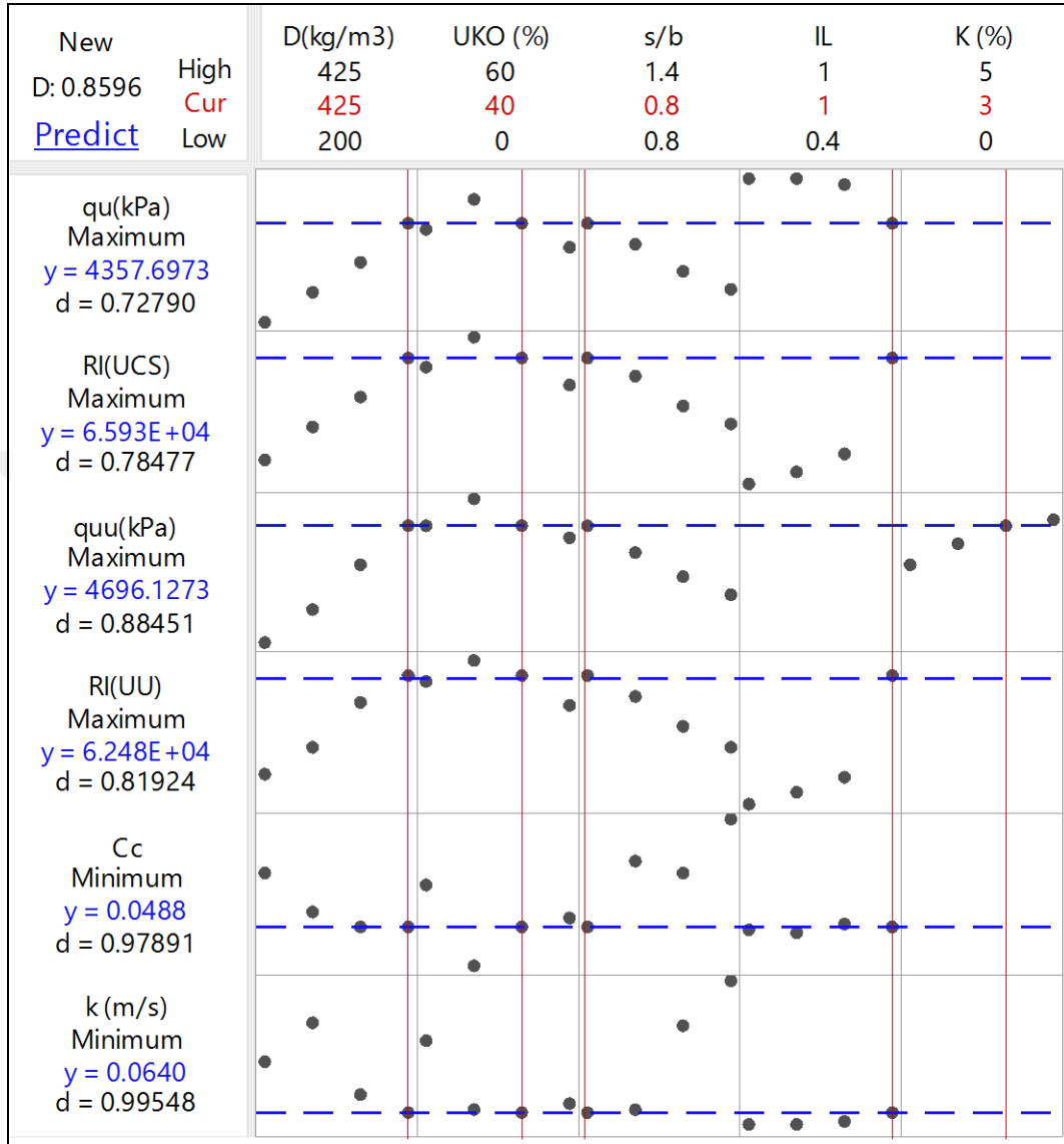
Şekil 4.89. UKO=%40 ve K=%3 için 28 günlük performans değerlerinin tahmini için optimizasyon grafiği (Not: k değeri 10 -9 ile çarpılmalıdır.)
