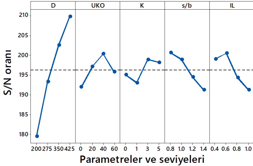
Şekil 4.44. Permeabilite katsayısı (k) için elde edilen S/N grafiği (Büyük ölçekli DKK, 28 gün)
