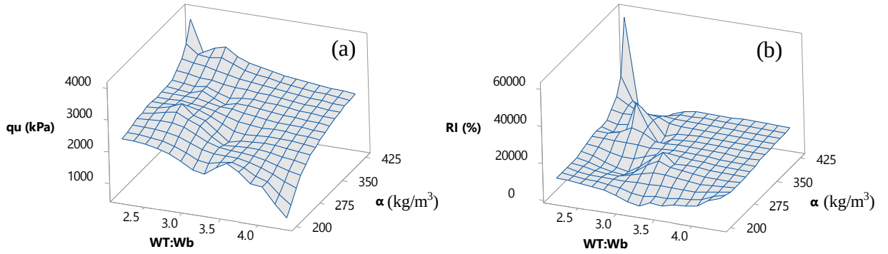
Şekil 4.26. W_T:W_b ve \alpha ile a) q_u ve b) RI arasındaki ilişki (Büyük ölçekli DKK, UCS, 56 gün)
