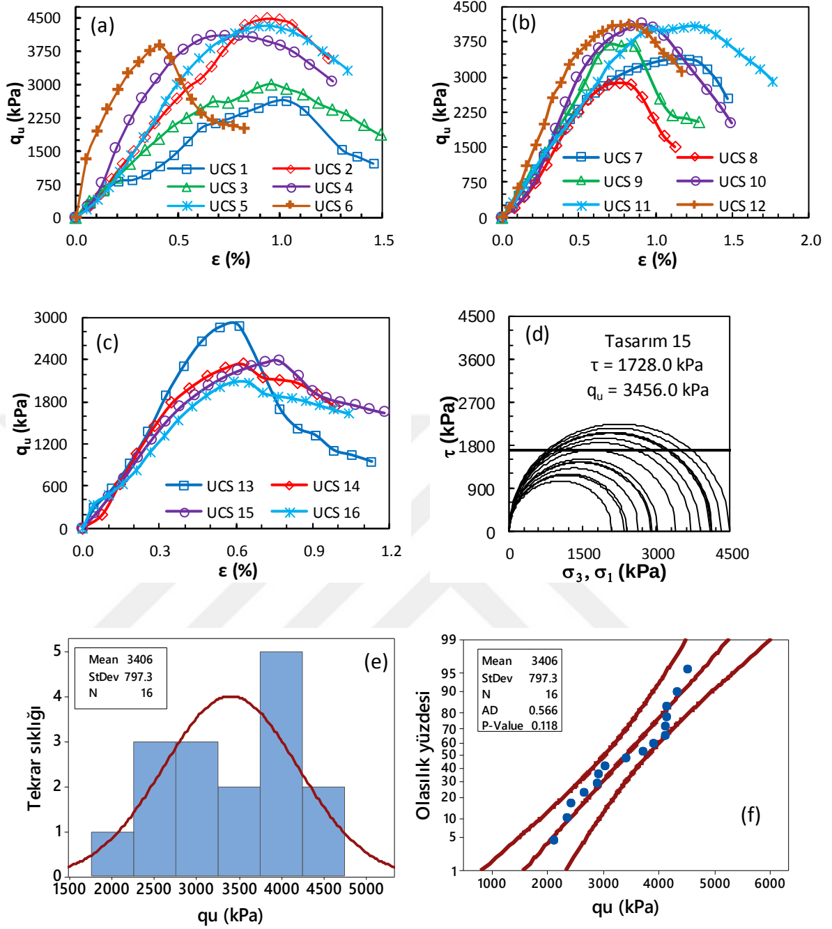
Şekil Ek 2.31. BÖ-15 numaralı kolona ait gerilme-birim deformasyon grafikleri: a) kolon üst bölgesi, b) kolon orta bölgesi, c) kolon alt bölgesi ve d) Mohr daireleri, e) histogram grafiği, f) olasılık grafiği (Büyük ölçekli DKK, UCS, 56 gün)
