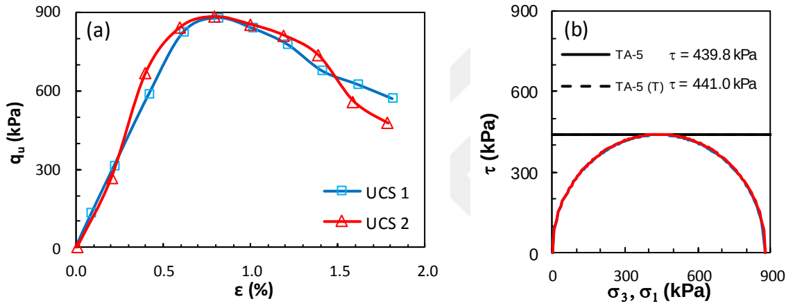
Şekil Ek 5.5. KÖ-5 numaralı tasarım: a) gerilme-birim deformasyon grafikleri ve b) Mohr daireleri (Küçük ölçekli DKK, UCS, 7 gün)
