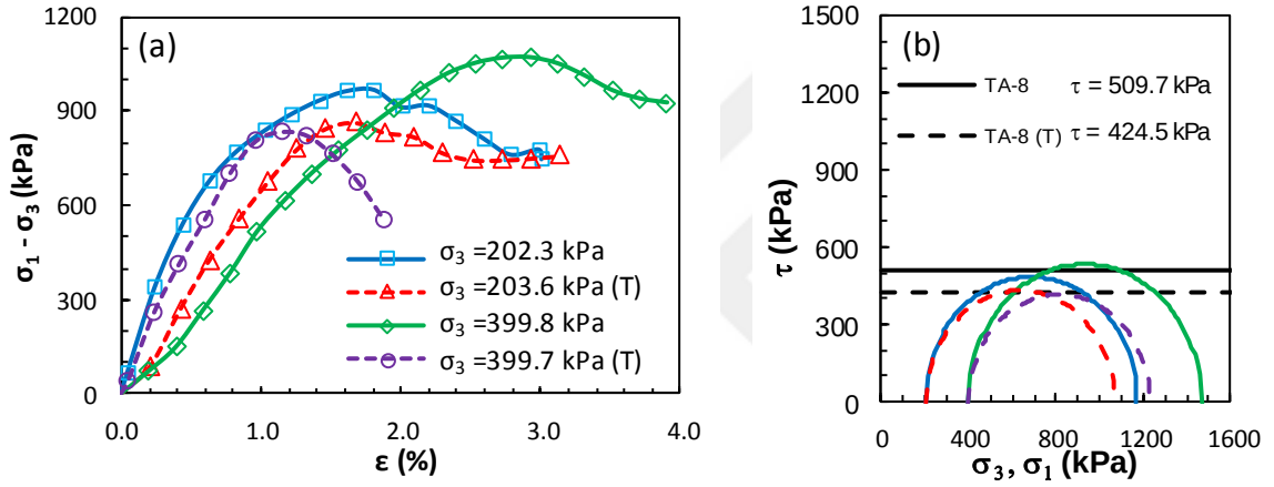
Şekil Ek 6.8. KÖ-8 numaralı tasarım: a) deviator gerilme-birim deformasyon grafikleri ve b) Mohr daireleri (Küçük ölçekli DKK, UU, 7 gün)
