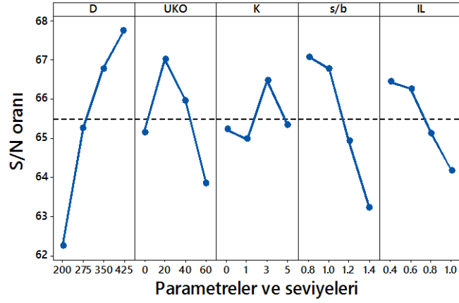
Şekil 4.30. Kolon dayanımı için elde edilen S/N grafiği (Büyük ölçekli DKK, UU, 28 gün)
