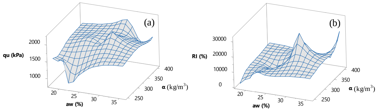
Şekil 4.5. Çimento faktörü ve çimento içeriği ile a) q_u ve b) RI arasındaki ilişki
