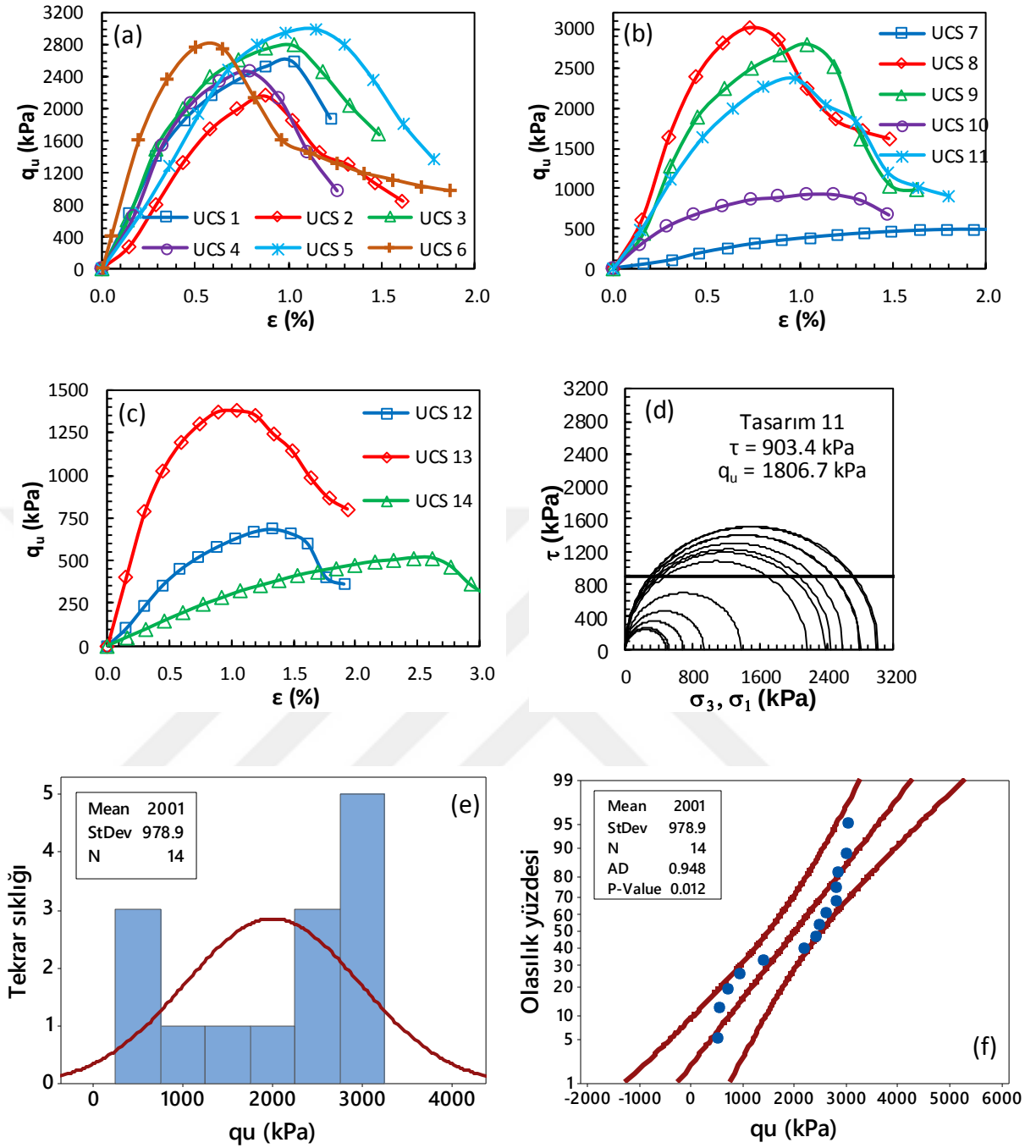
Şekil Ek 2.11. BÖ-11 numaralı kolona ait gerilme-birim deformasyon grafikleri: a) kolon üst bölgesi, b) kolon orta bölgesi, c) kolon alt bölgesi ve d) Mohr daireleri, e) histogram grafiği, f) olasılık grafiği (Büyük ölçekli DKK, UCS, 28 gün)
