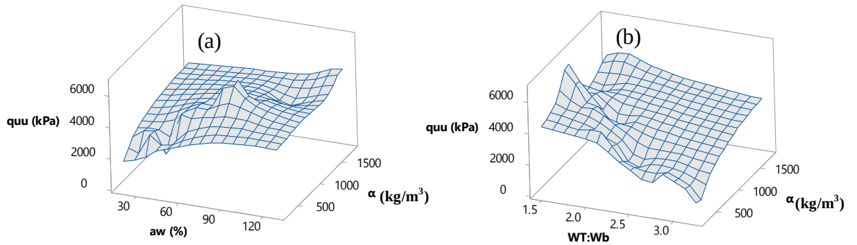
Şekil 4.66. Üç eksenli basınç dayanımının a) a_w - \alpha ve b) WT:W_b - \alpha arasındaki ilişkiler (Küçük ölçekli DKK, UU, 56 gün)
