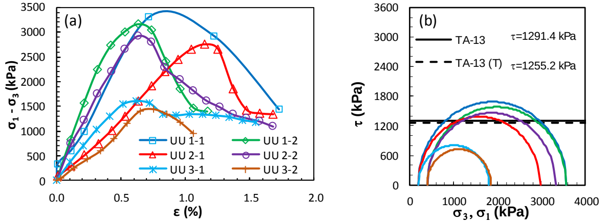
Şekil Ek 3.13. BÖ-13 numaralı kolona ait UU deney sonuçları: a) deviator gerilme-birim boy kısalması grafikleri, b) Mohr daireleri ile kırılma zarfları (Büyük ölçekli DKK, UU, 28 gün)
