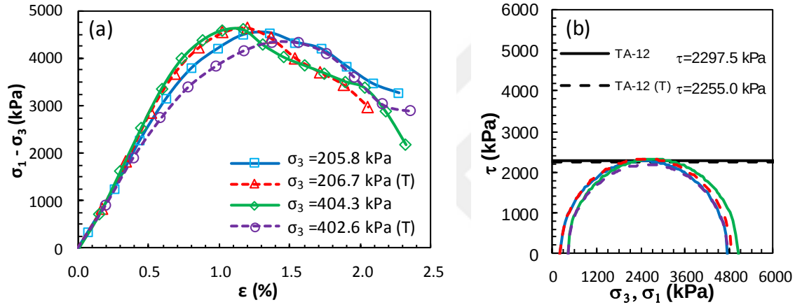
Şekil Ek 6.44. KÖ-12 numaralı tasarım: a) deviator gerilme-birim deformasyon grafikleri ve b) Mohr daireleri (Küçük ölçekli DKK, UU, 56 gün)
