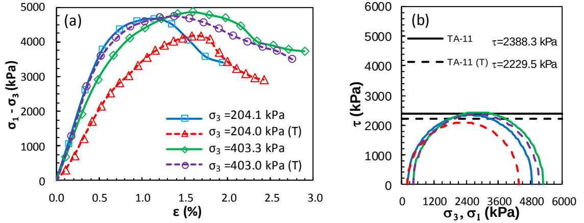
Şekil Ek 6.43. KÖ-11 numaralı tasarım: a) deviator gerilme-birim deformasyon grafikleri ve b) Mohr daireleri (Küçük ölçekli DKK, UU, 56 gün)
