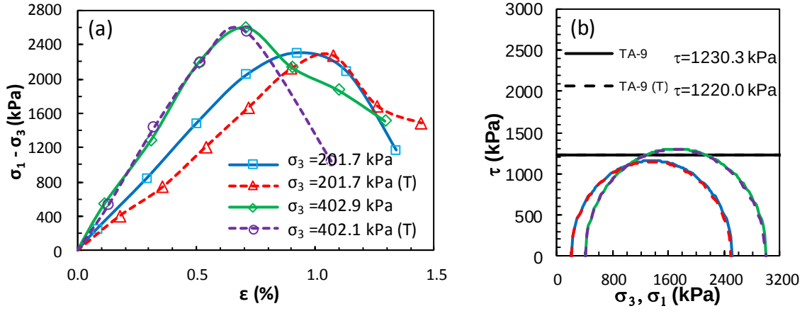
Şekil Ek 6.25. KÖ-9 numaralı tasarım: a) deviator gerilme-birim deformasyon grafikleri ve b) Mohr daireleri (Küçük ölçekli DKK, UU, 28 gün)
