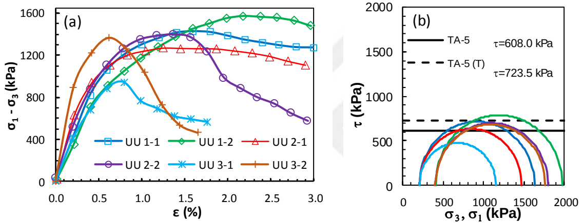
Şekil Ek 3.5. BÖ-5 numaralı kolona ait UU deney sonuçları: a) deviator gerilme-birim boy kısalması grafikleri, b) Mohr daireleri ile kırılma zarfları (Büyük ölçekli DKK, UU, 28 gün)
