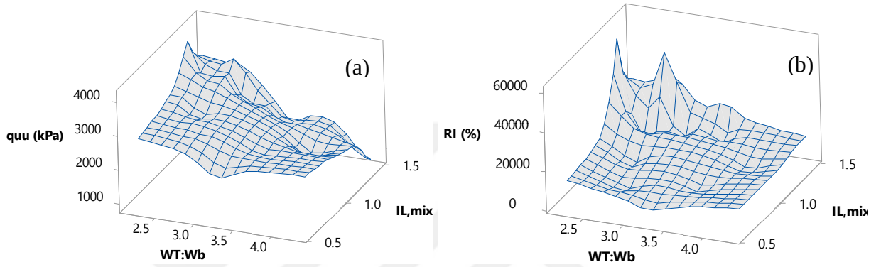
Şekil 4.37. W_T:W_b ile I_{L,mix} a) q_u ve b) RI arasındaki ilişki (Büyük ölçekli DKK, UU, 56 gün)
