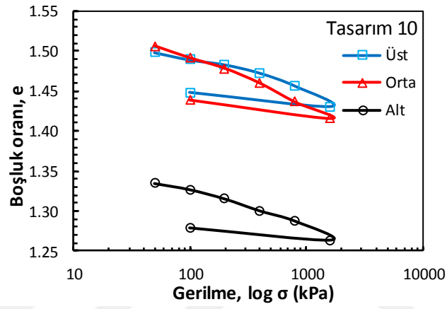
Şekil Ek 4.26. BÖ-10 numaralı kolona ait konsolidasyon deney sonucu (Büyük ölçekli DKK, 56 gün)
