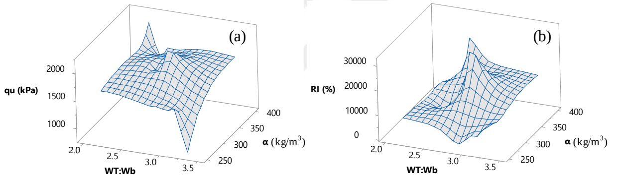
Şekil 4.6. Çimento faktörü ve karışımın toplam su/bağlayıcı ile a) q_u ve b) RI arasındaki ilişki
