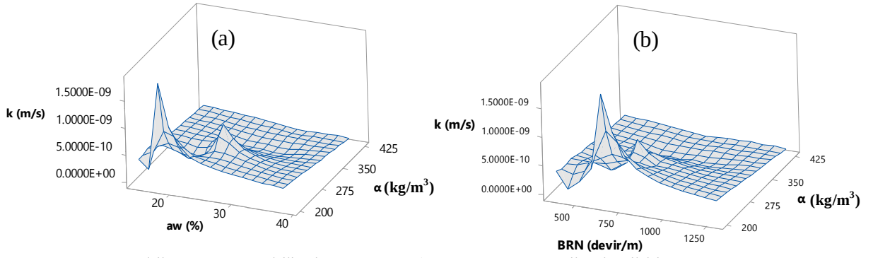
Şekil 4.48. Permeabilite katsayısının a) a_w - \alpha ve b) BRN- \alpha ile olan ilişkileri
