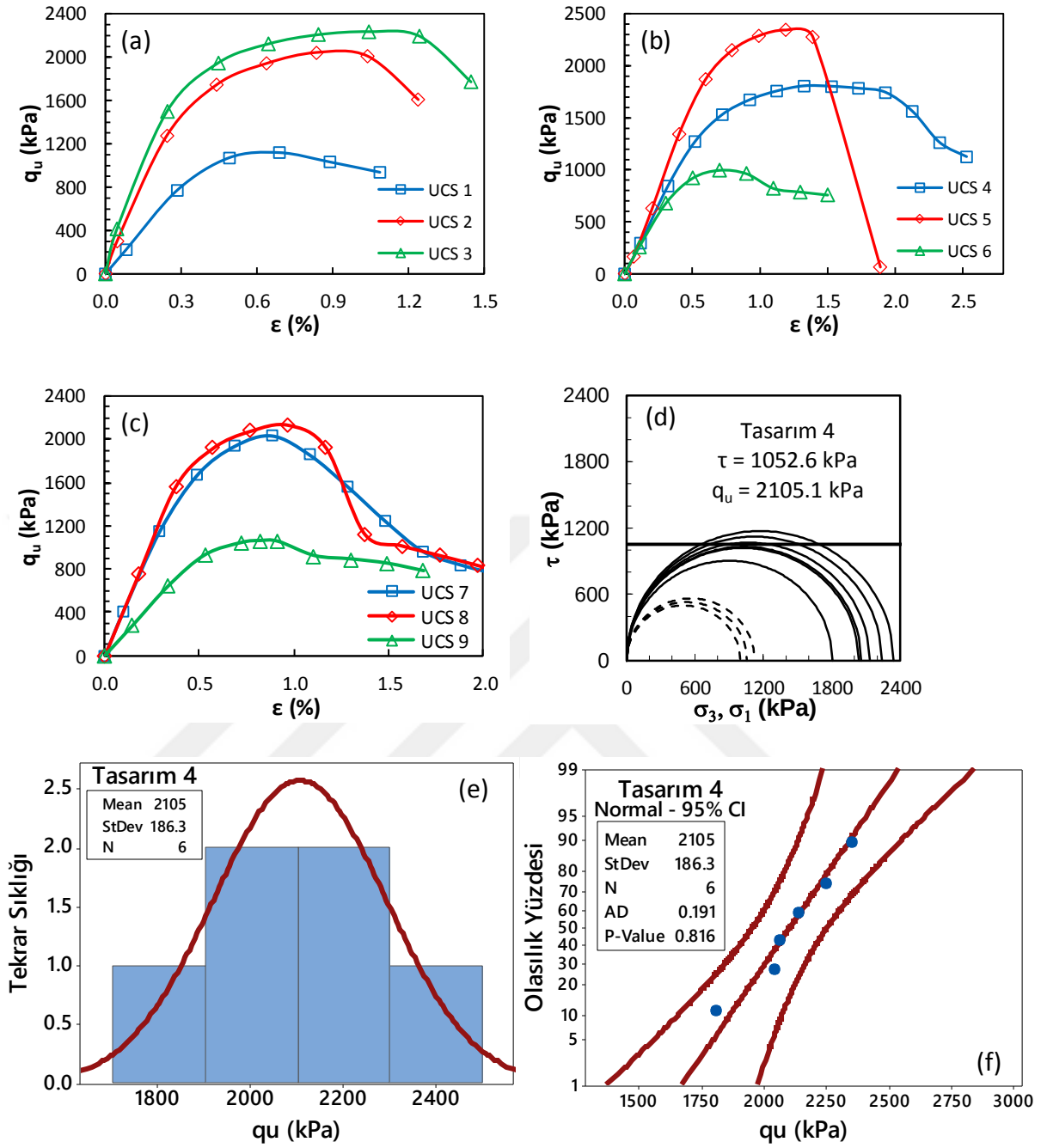
Şekil Ek 1.4. SP-4 numaralı kolona ait gerilme-birim deformasyon grafikleri: a) kolon alt bölgesi, b) kolon orta bölgesi, c) kolon üst bölgesi ve d) Mohr daireleri, e) histogram grafiği, f) olasılık grafiği (Not: UCS 1, UCS 6 ve UCS 9 deneyleri ortalamaya katılmamıştır) (Sistem parametreleri, UCS, 28 gün)
