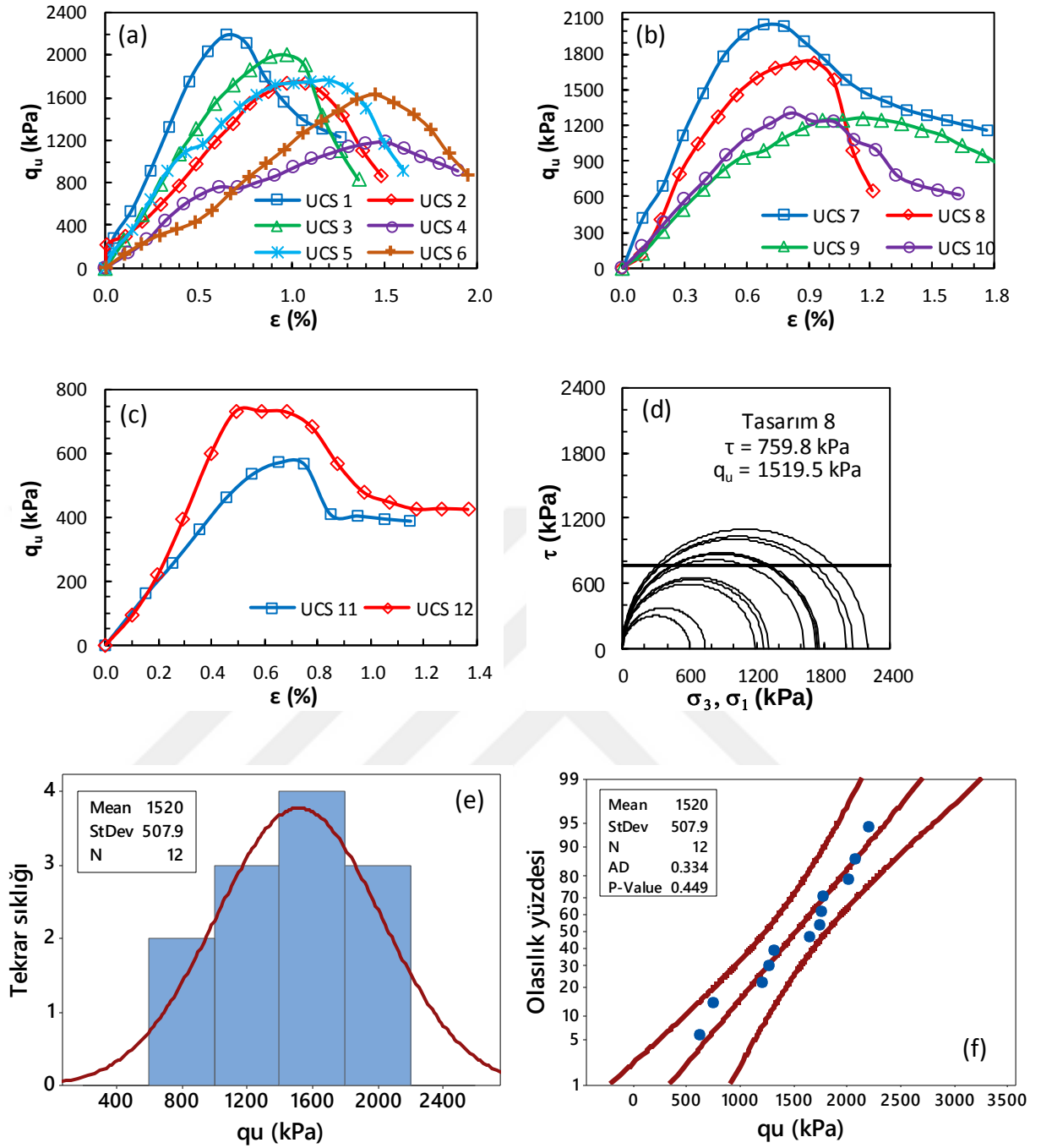
Şekil Ek 2.8. BÖ-8 numaralı kolona ait gerilme-birim deformasyon grafikleri: a) kolon üst bölgesi, b) kolon orta bölgesi, c) kolon alt bölgesi ve d) Mohr daireleri, e) histogram grafiği, f) olasılık grafiği (Büyük ölçekli DKK, UCS, 28 gün)
