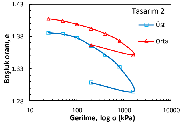
Şekil Ek 4.2. BÖ-2 numaralı kolona ait konsolidasyon deney sonucu (Büyük ölçekli DKK, 28 gün)
