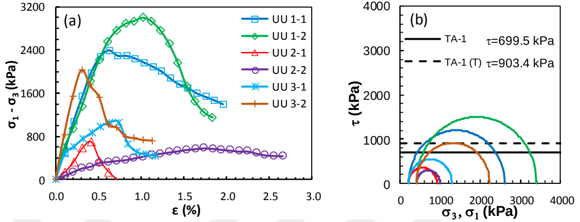
Şekil Ek 3.1. BÖ-1 numaralı kolona ait UU deney sonuçları: a) deviator gerilme-birim boy kısalması grafikleri, b) Mohr daireleri ile kırılma zarfları (Büyük ölçekli DKK, UU, 28 gün)
