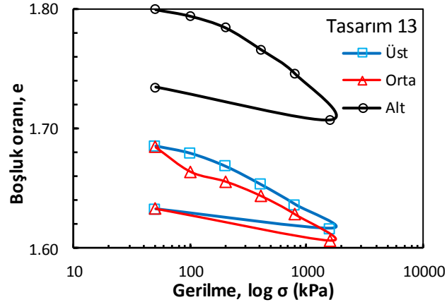
Şekil Ek 4.13. BÖ-13 numaralı kolona ait konsolidasyon deney sonucu (Büyük ölçekli DKK, 28 gün)
