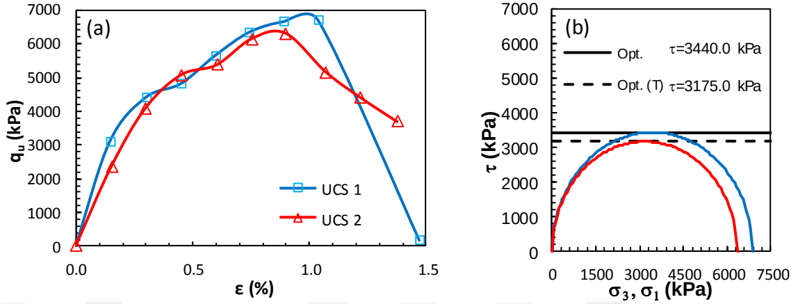
Şekil 4.90. Optimum tasarıma ait a) gerilme-birim deformasyon grafikleri ve b) Mohr daireleri (Küçük ölçekli DKK, UCS, 56 gün)
