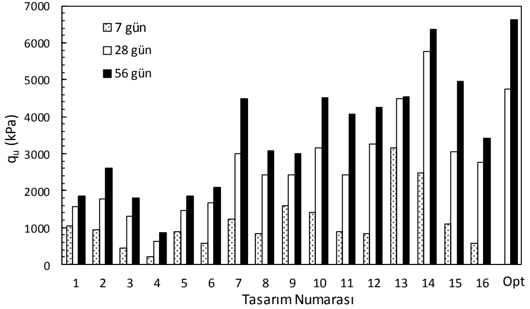
Şekil 4.55. Serbest basınç deney sonuçları (Küçük ölçekli DKK)
