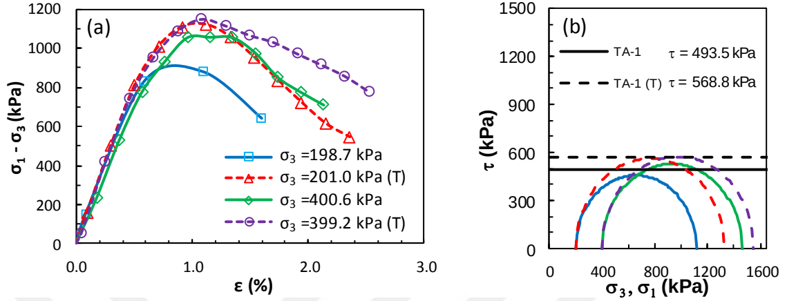
Şekil Ek 6.1. KÖ-1 numaralı tasarım: a) deviator gerilme-birim deformasyon grafikleri ve b) Mohr daireleri (Küçük ölçekli DKK, UU, 7 gün)
