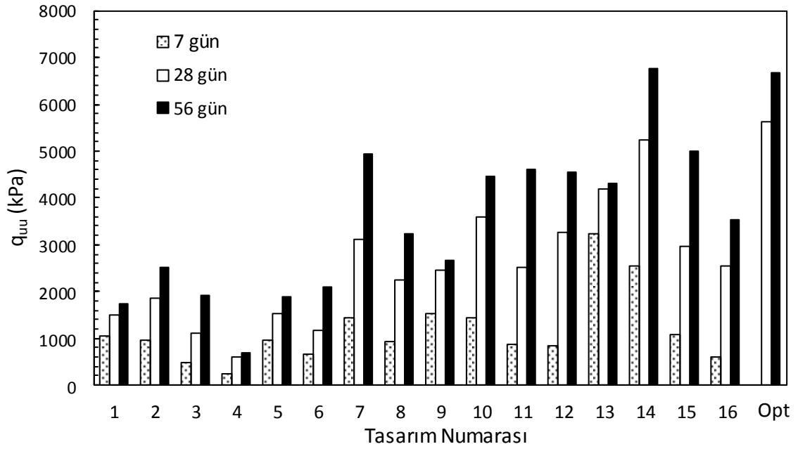
Şekil 4.64. Üç eksenli basınç deney sonuçları (Küçük ölçekli DKK)
