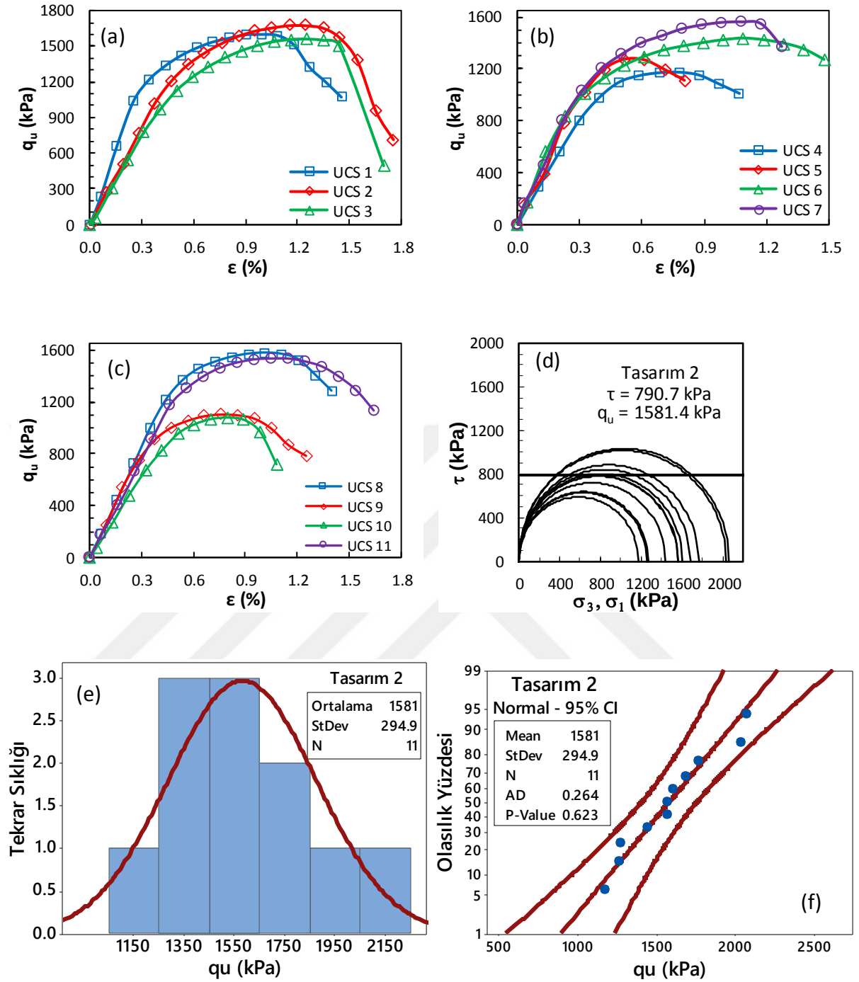
Şekil Ek 1.2. SP-2 numaralı kolona ait gerilme-birim deformasyon grafikleri: a) kolon alt bölgesi, b) kolon orta bölgesi, c) kolon üst bölgesi ve d) Mohr daireleri, e) histogram grafiği, f) olasılık grafiği (Sistem parametreleri, UCS, 28 gün)
