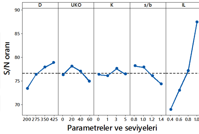
Şekil 4.31. Zemin iyileştirme derecesi için elde edilen S/N grafiği (Büyük ölçekli DKK, UU, 28 gün)
