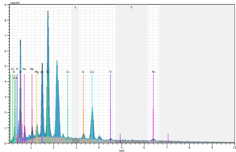
Şekil 4.118. Yüksek plastisiteli kile ait EDX analiz sonucu
