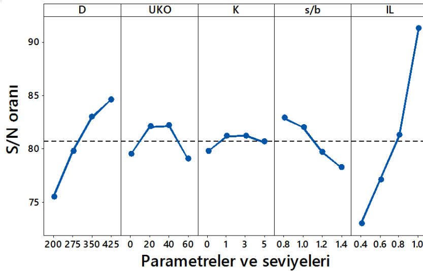
Şekil 4.54. Zemin iyileştirme derecesi için elde edilen S/N grafiği (Küçük ölçekli DKK, UCS, 56 gün)
