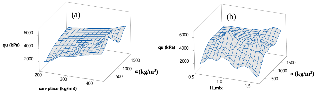
Şekil 4.56. Serbest basınç dayanımının a) \alpha_{in-place} - \alpha ve b) I_{L,mix} - \alpha arasındaki ilişkiler (Küçük ölçekli DKK, UCS, 56 gün)
