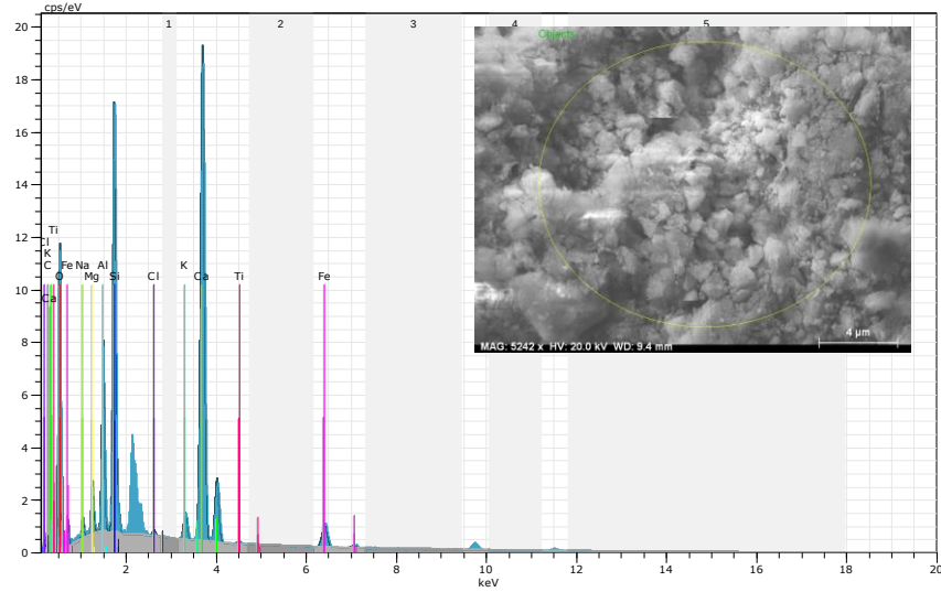
Şekil 4.133. Optimum tasarıma ait EDX sonucu (Küçük ölçekli DKK, 28 gün)
