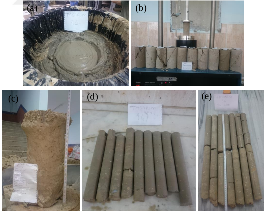
Şekil 3.65. Büyük ölçekli DKK, Tasarım 14: a) imalat sonrası görünüm, b) kayma yüzeyleri, c) imal edilen kolon, d) 28 ve e) 56 günlük karot numuneleri (büyük ölçekli DKK)
