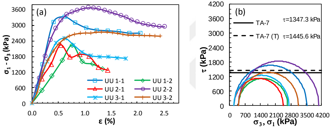
Şekil Ek 3.23. BÖ-7 numaralı kolona ait UU deney sonuçları: a) deviatör gerilme-birim boy kısalması grafikleri, b) Mohr daireleri ile kırılma zarfları (Büyük ölçekli DKK, UU, 56 gün)
