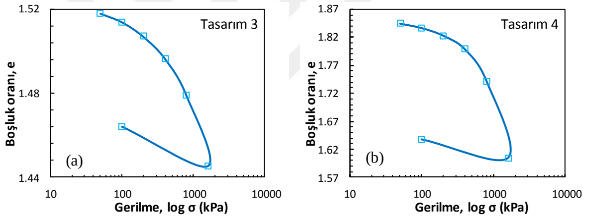
Şekil Ek 7.2. Küçük ölçekli DKK, konsolidasyon deneyi, 28 gün: a) Tasarım 3 ve b) Tasarım 4
