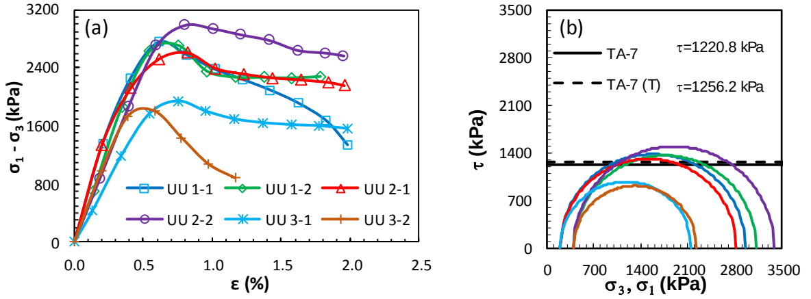
Şekil Ek 3.7. BÖ-7 numaralı kolona ait UU deney sonuçları: a) deviator gerilme-birim boy kısalması grafikleri, b) Mohr daireleri ile kırılma zarfları (Büyük ölçekli DKK, UU, 28 gün)
