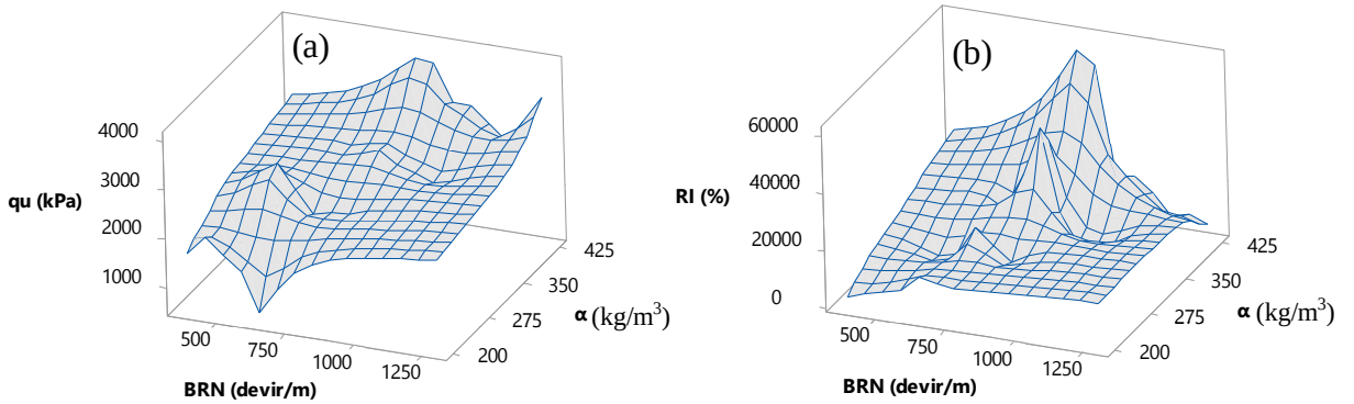
Şekil 4.27. BRN ve \alpha ile a) q_u ve b) RI arasındaki ilişki (Büyük ölçekli DKK, UCS, 56 gün)
