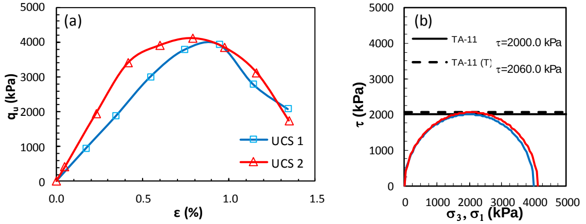
Şekil Ek 5.43. KÖ-11 numaralı tasarım: a) gerilme-birim deformasyon grafikleri ve b) Mohr daireleri (Küçük ölçekli DKK, UCS, 56 gün)
