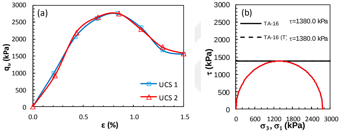
Şekil Ek 5.32. KÖ-16 numaralı tasarım: a) gerilme-birim deformasyon grafikleri ve b) Mohr daireleri (Küçük ölçekli DKK, UCS, 28 gün)
