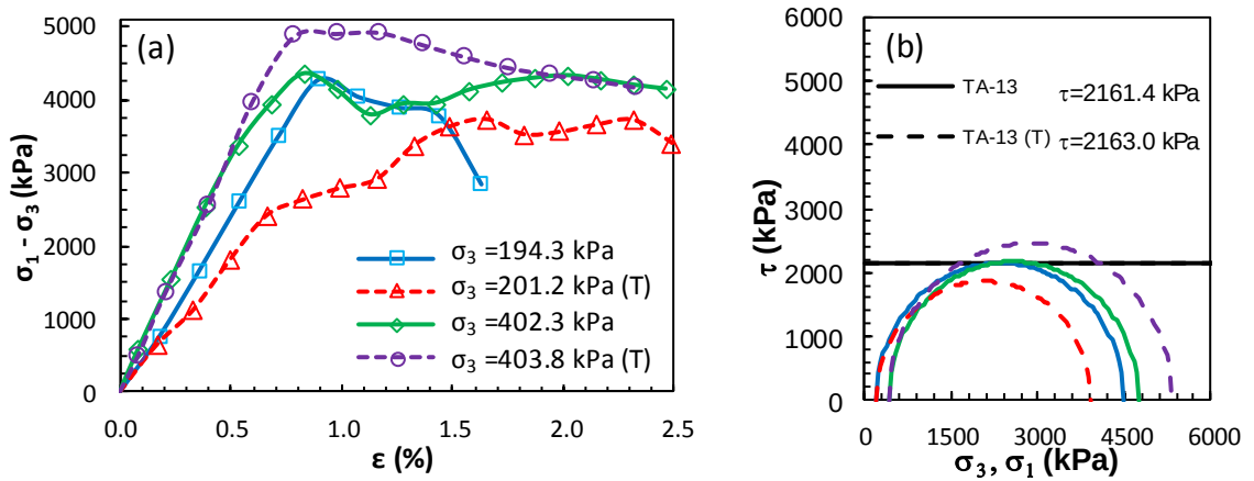
Şekil Ek 6.45. KÖ-13 numaralı tasarım: a) deviator gerilme-birim deformasyon grafikleri ve b) Mohr daireleri (Küçük ölçekli DKK, UU, 56 gün)
