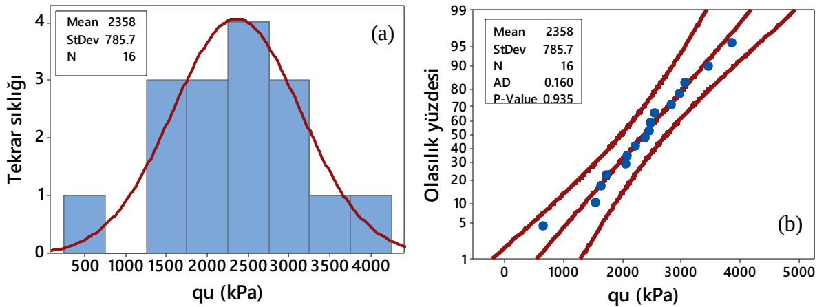
Şekil 4.20. Kolon dayanımı için elde edilen a) histogram grafiği ve b) normalolasılık grafiği (Büyük ölçekli DKK, UCS, 56 gün)
