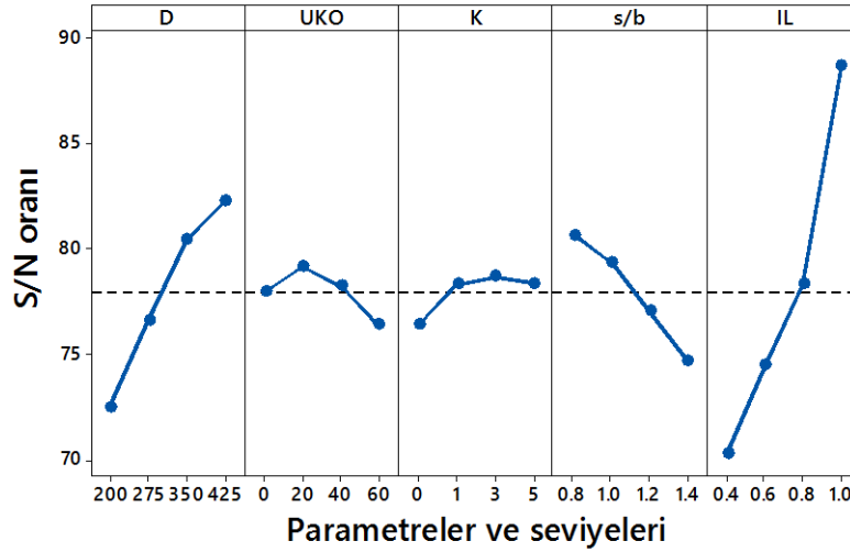
Şekil 4.61. Zemin iyileştirme derecesi için elde edilen S/N grafiği (Küçük ölçekli DKK, UU, 28 gün)
