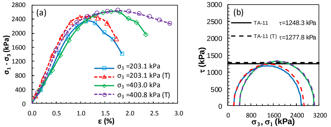
Şekil Ek 6.27. KÖ-11 numaralı tasarım: a) deviator gerilme-birim deformasyon grafikleri ve b) Mohr daireleri (Küçük ölçekli DKK, UU, 28 gün)
