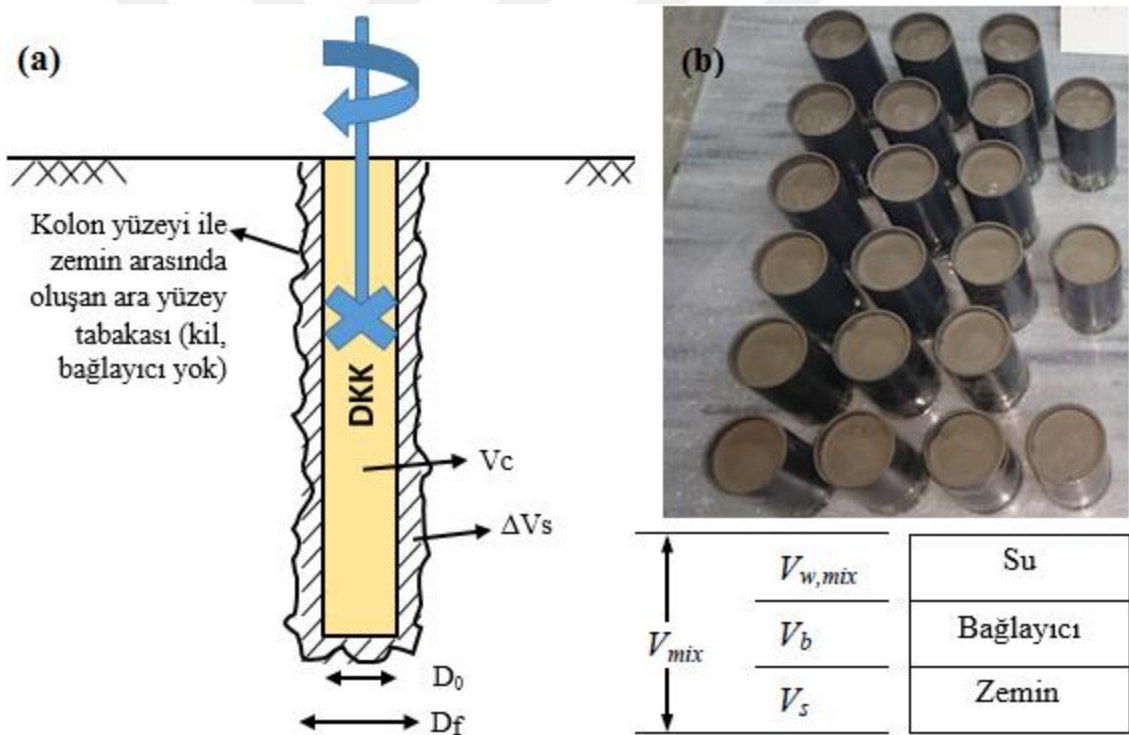
Şekil 4.104. İmalat sırasındaki farklılıklar: a) büyük ve b) küçük ölçekli DKK tasarımları
