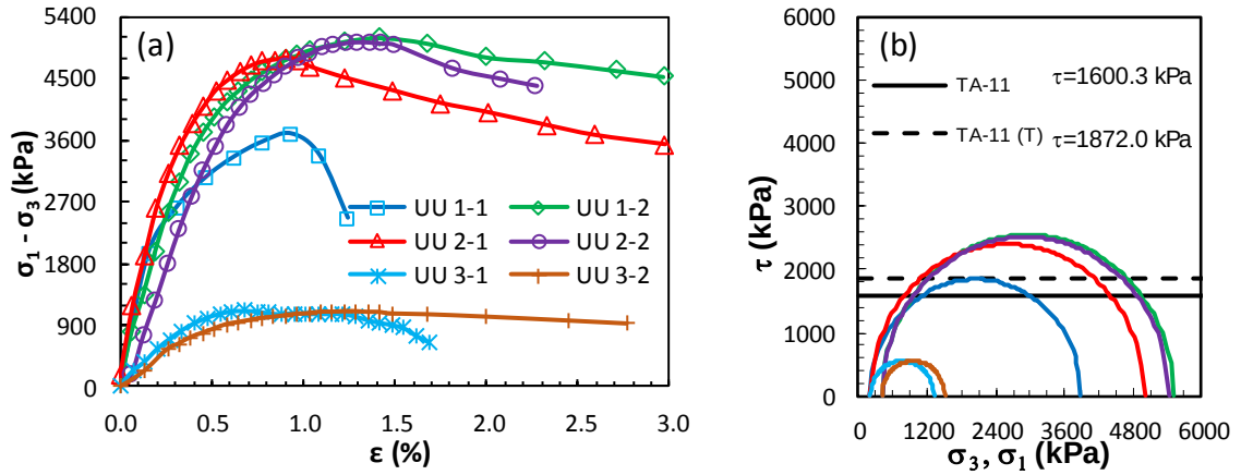
Şekil Ek 3.27. BÖ-11 numaralı kolona ait UU deney sonuçları: a) deviator gerilme-birim boy kısalması grafikleri, b) Mohr daireleri ile kırılma zarfları (Büyük ölçekli DKK, UU, 56 gün)
