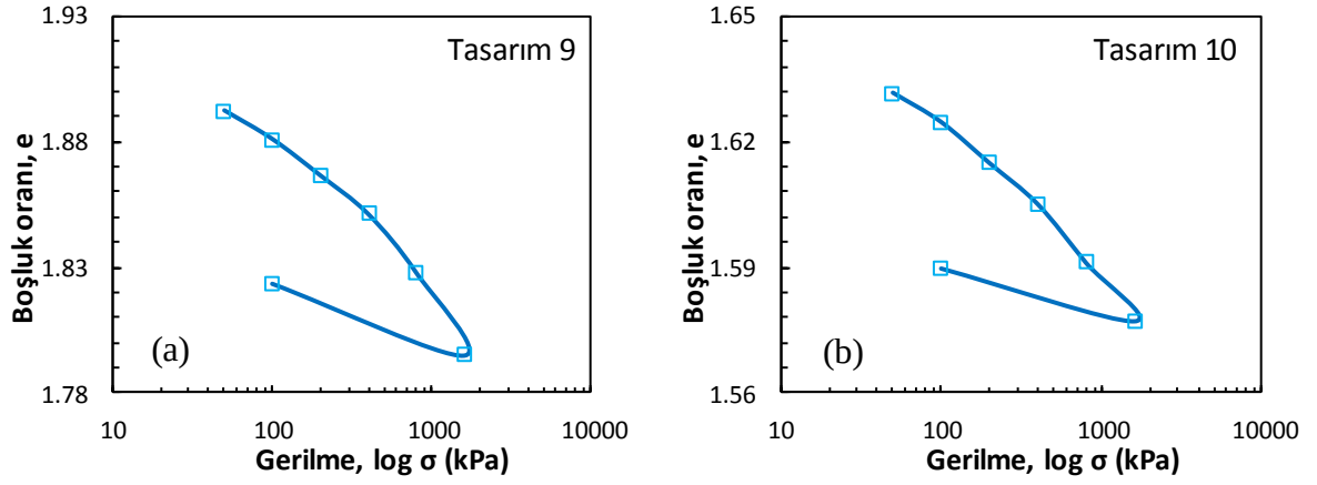
Şekil Ek 7.13. Küçük ölçekli DKK, konsolidasyon deneyi, 56 gün: a) Tasarım 9 ve b) Tasarım 10
