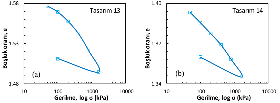
Şekil Ek 7.7. Küçük ölçekli DKK, konsolidasyon deneyi, 28 gün: a) Tasarım 13 ve b) Tasarım 14
