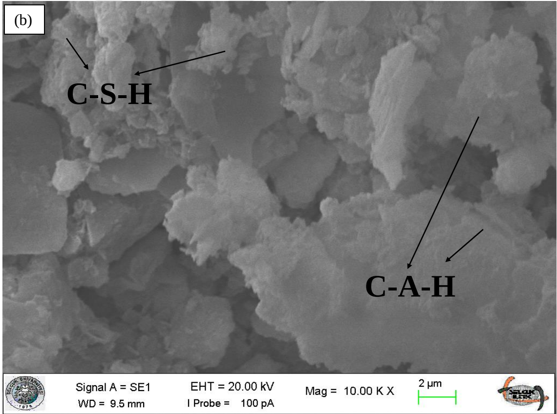
Şekil 4.128. Optimum tasarıma ait SEM görüntüleri: a) x5000, b) x10000 (Küçük ölçekli DKK, 56 gün)
