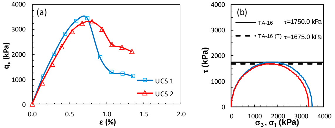
Şekil Ek 5.48. KÖ-16 numaralı tasarım: a) gerilme-birim deformasyon grafikleri ve b) Mohr daireleri (Küçük ölçekli DKK, UCS, 56 gün)
