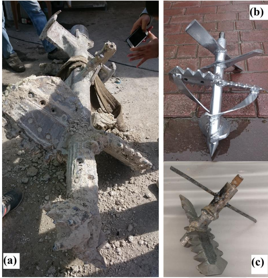
Şekil 3.19. DKK imalatında kullanılan karıştırma bıçakları a) arazi tipi ve b, c) laboratuvar tipi
