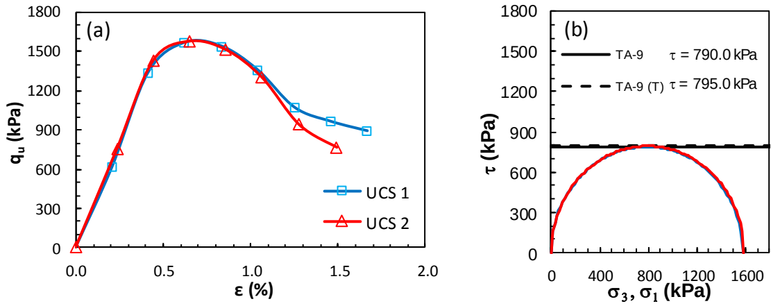
Şekil Ek 5.9. KÖ-9 numaralı tasarım: a) gerilme-birim deformasyon grafikleri ve b) Mohr daireleri (Küçük ölçekli DKK, UCS, 7 gün)
