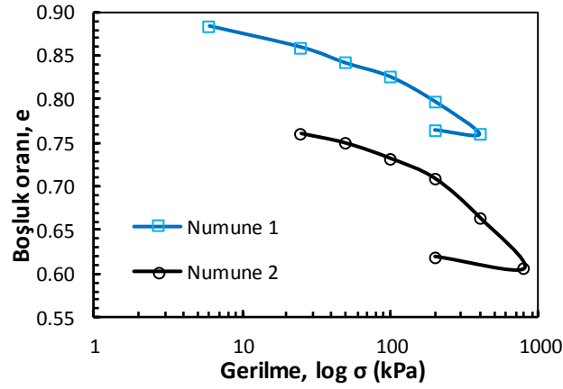
Şekil 3.12. Killi zemin için konsolidasyon deneyinden elde edilen gerilme-boşluk oranı grafikleri
