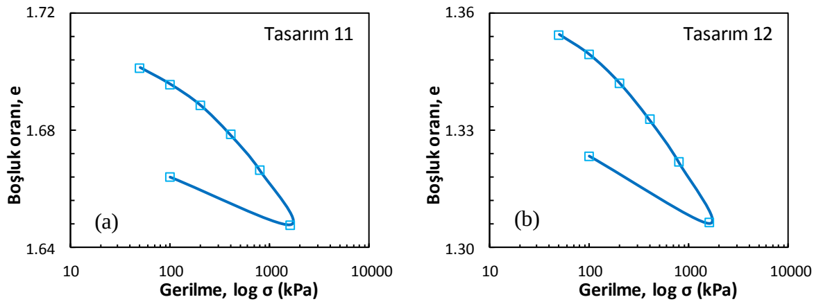
Şekil Ek 7.6. Küçük ölçekli DKK, konsolidasyon deneyi, 28 gün: a) Tasarım 11 ve b) Tasarım 12
