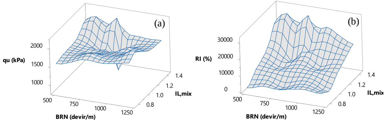
Şekil 4.8. I_{L,mix} ve BRN ile a) q_u ve b) RI arasındaki ilişki
