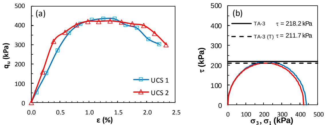
Şekil Ek 5.3. KÖ-3 numaralı tasarım: a) gerilme-birim deformasyon grafikleri ve b) Mohr daireleri (Küçük ölçekli DKK, UCS, 7 gün)
