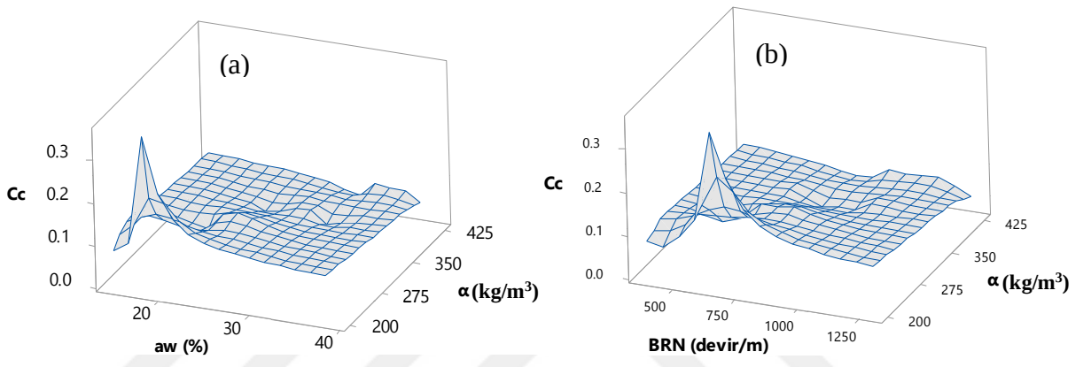
Şekil 4.43. Sıkışma indisinin a) a_w-\alpha ve b) BRN-\alpha ile olan ilişkileri (Büyük ölçekli DKK, 56 gün)
