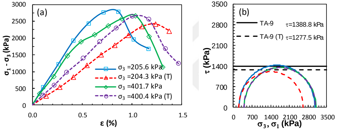
Şekil Ek 6.41. KÖ-9 numaralı tasarım: a) deviator gerilme-birim deformasyon grafikleri ve b) Mohr daireleri (Küçük ölçekli DKK, UU, 56 gün)
