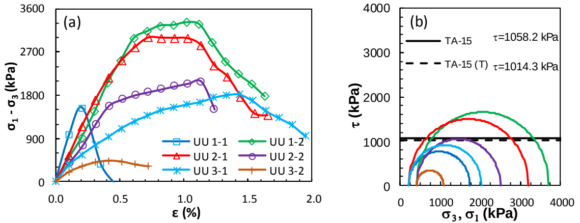
Şekil Ek 3.15. BÖ-15 numaralı kolona ait UU deney sonuçları: a) deviator gerilme-birim boy kısalması grafikleri, b) Mohr daireleri ile kırılma zarfları (Büyük ölçekli DKK, UU, 28 gün)
