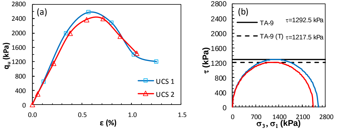
Şekil Ek 5.25. KÖ-9 numaralı tasarım: a) gerilme-birim deformasyon grafikleri ve b) Mohr daireleri (Küçük ölçekli DKK, UCS, 28 gün)
