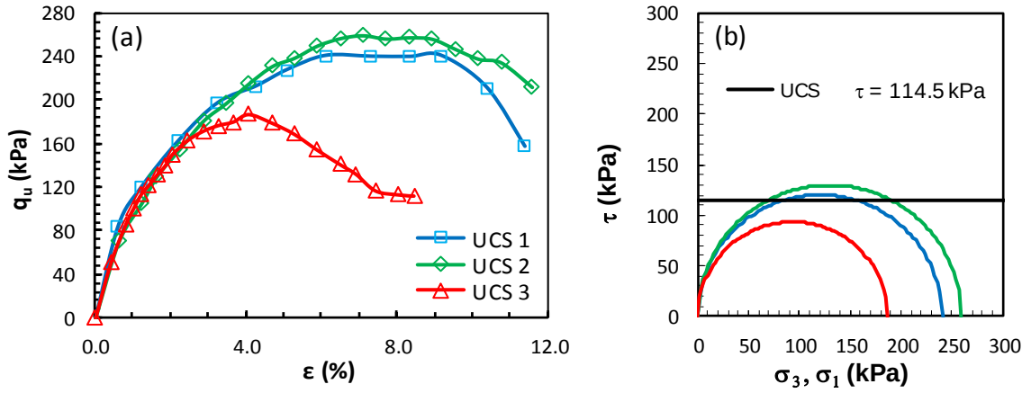
Şekil 3.10. Killi zemin için serbest basınç deneyi sonuçları: a) Gerilme-birim deformasyon grafikleri ve b) Mohr daireleri
