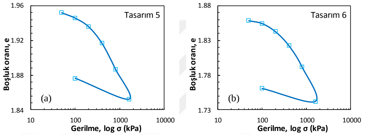
Şekil Ek 7.11. Küçük ölçekli DKK, konsolidasyon deneyi, 56 gün: a) Tasarım 5 ve b) Tasarım 6
