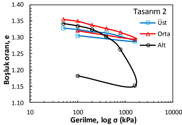
Şekil Ek 4.18. BÖ-2 numaralı kolona ait konsolidasyon deney sonucu (Büyük ölçekli DKK, 56 gün)
