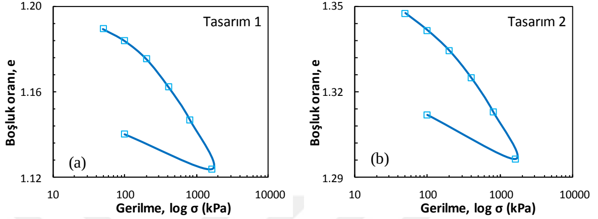
Şekil Ek 7.1. Küçük ölçekli DKK, konsolidasyon deneyi, 28 gün: a) Tasarım 1 ve b) Tasarım 2
