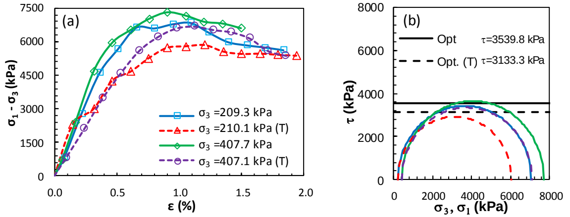
Şekil 4.92. Optimum tasarıma ait UU deney sonuçları: a) deviatör gerilme-birim boy kısalması grafikleri, b) Mohr daireleri ile kırılma zarfları (Küçük ölçekli DKK, UU, 56 gün)
