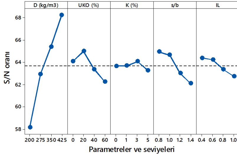
Şekil 4.19. Kolon dayanımı için elde edilen S/N grafiği (Büyük ölçekli DKK, UCS, 28 gün)
