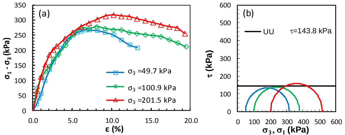
Şekil 3.11. Killi zemine ait üç eksenli basınç deneyi sonuçları: a) Deviyatör gerilme-birim deformasyon grafikleri ve b) Mohr daireleri
