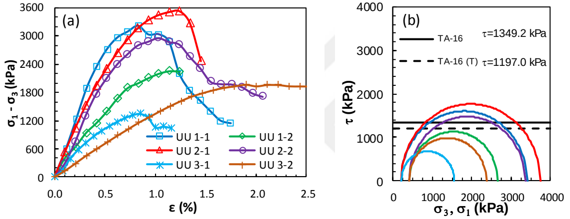
Şekil Ek 3.32. BÖ-16 numaralı kolona ait UU deney sonuçları: a) deviator gerilme-birim boy kısalması grafikleri, b) Mohr daireleri ile kırılma zarfları (Büyük ölçekli DKK, UU, 56 gün)
