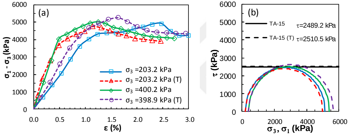
Şekil Ek 6.47. KÖ-15 numaralı tasarım: a) deviator gerilme-birim deformasyon grafikleri ve b) Mohr daireleri (Küçük ölçekli DKK, UU, 56 gün)
