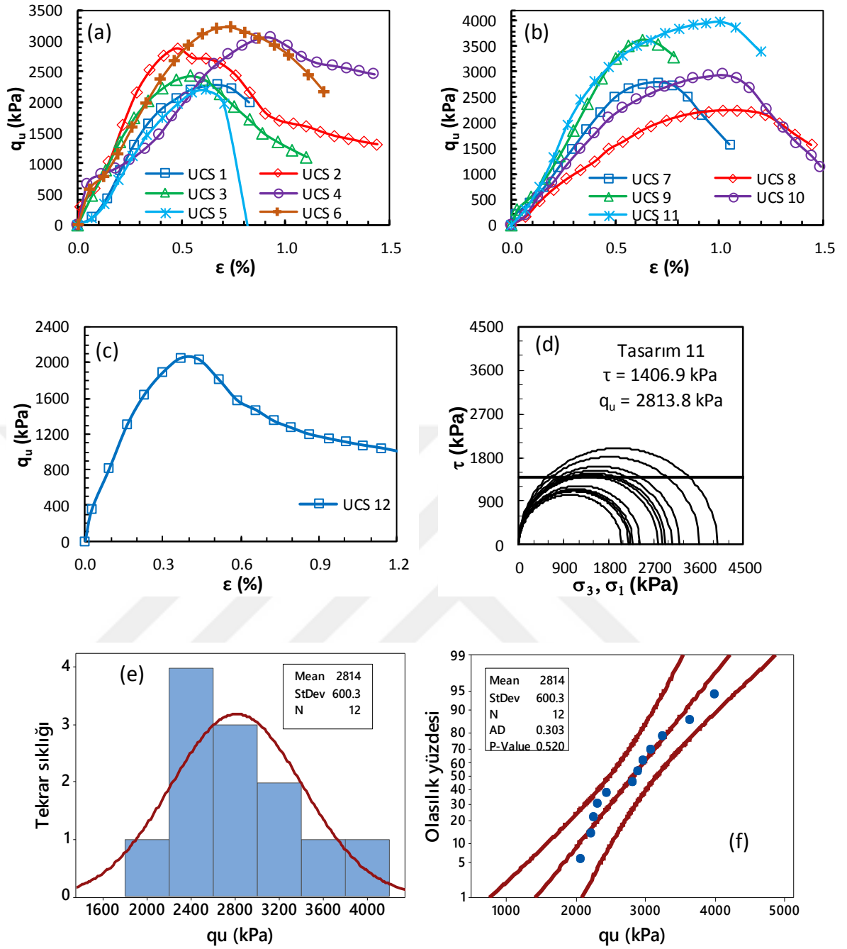
Şekil Ek 2.27. BÖ-11 numaralı kolona ait gerilme-birim deformasyon grafikleri: a) kolon üst bölgesi, b) kolon orta bölgesi, c) kolon alt bölgesi ve d) Mohr daireleri, e) histogram grafiği, f) olasılık grafiği (Büyük ölçekli DKK, UCS, 56 gün)
