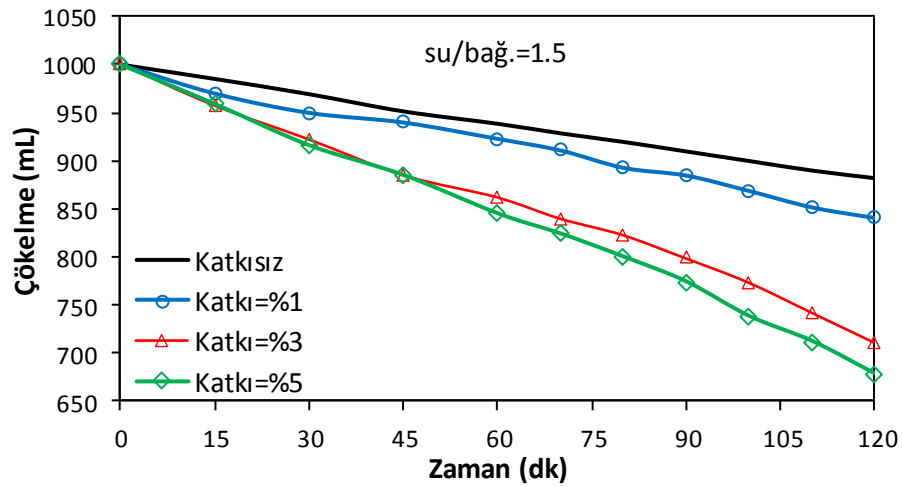
Şekil 3.50. Optima 100 katkısı ile yapılan sedimentasyon deneyi sonuçları (UKO=%60, su/bağlayıcı=1.5)
