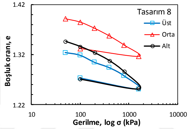
Şekil Ek 4.8. BÖ-8 numaralı kolona ait konsolidasyon deney sonucu (Büyük ölçekli DKK, 28 gün)
