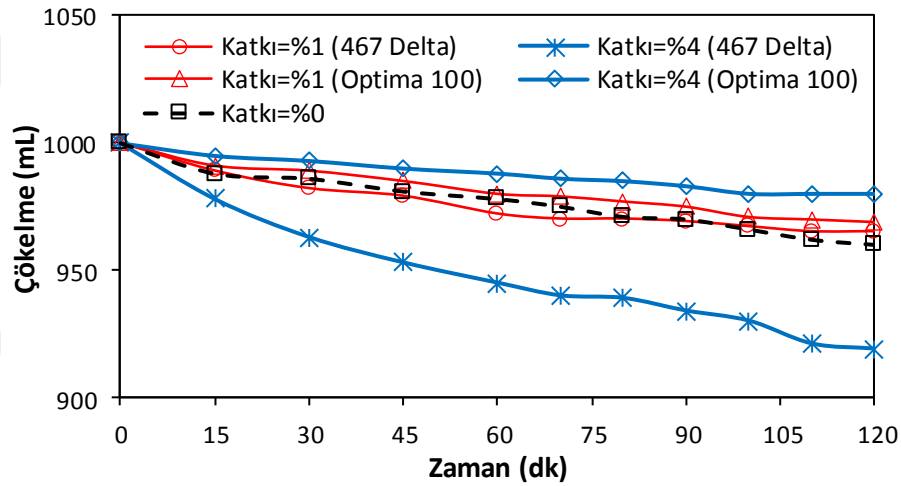
Şekil 3.45. Farklı katkıları ile yapılan sedimentasyon deneyi sonuçları (UKO=%60, su/bağlayıcı=1)
