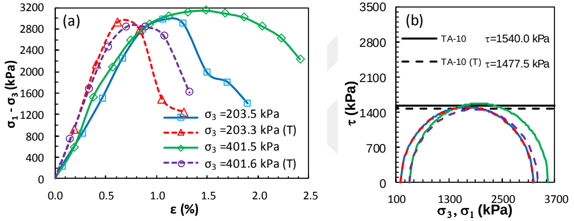
Şekil Ek 6.26. KÖ-10 numaralı tasarım: a) deviator gerilme-birim deformasyon grafikleri ve b) Mohr daireleri (Küçük ölçekli DKK, UU, 28 gün)
