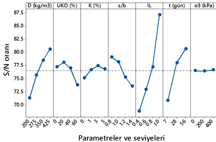
Şekil 4.106. RI için elde edilen S/N grafiği (Küçük ölçekli DKK)
