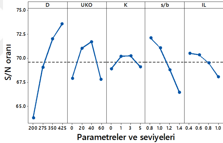
Şekil 4.62. Üç eksenli basınç dayanımı için elde edilen S/N grafiği (Küçük ölçekli DKK, UU, 56 gün)
