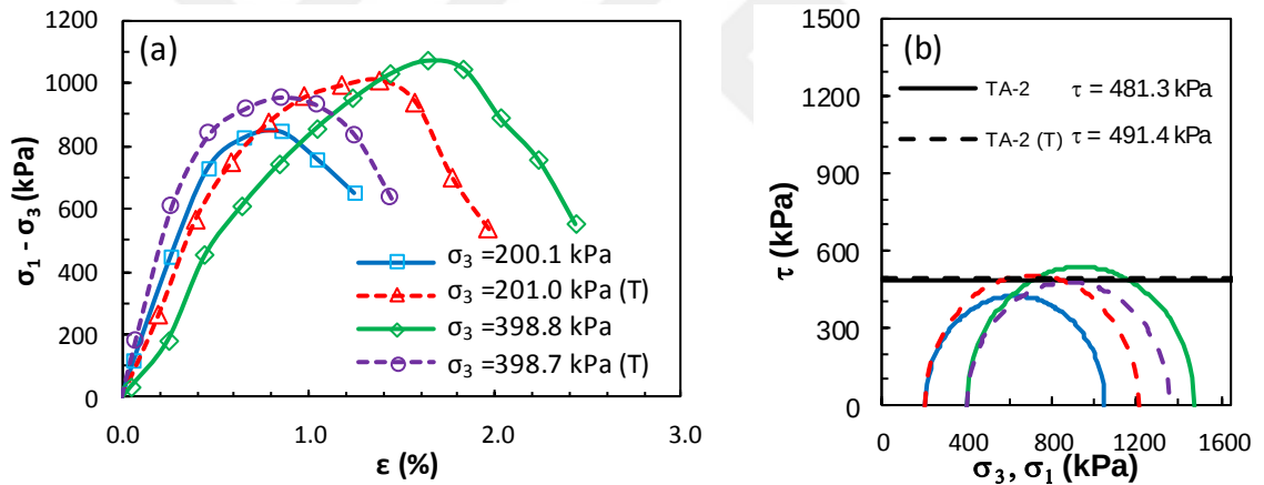
Şekil Ek 6.2. KÖ-2 numaralı tasarım: a) deviator gerilme-birim deformasyon grafikleri ve b) Mohr daireleri (Küçük ölçekli DKK, UU, 7 gün)
