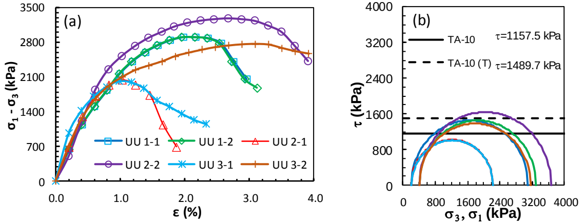
Şekil Ek 3.10. BÖ-10 numaralı kolona ait UU deney sonuçları: a) deviator gerilme-birim boy kısalması grafikleri, b) Mohr daireleri ile kırılma zarfları (Büyük ölçekli DKK, UU, 28 gün)
