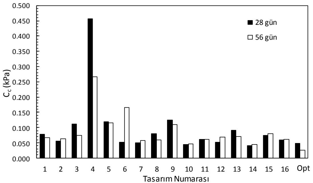
Şekil 4.69. Konsolidasyon deney sonuçları (Küçük ölçekli DKK)
