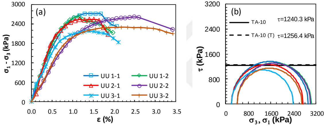
Şekil Ek 3.26. BÖ-10 numaralı kolona ait UU deney sonuçları: a) deviator gerilme-birim boy kısalması grafikleri, b) Mohr daireleri ile kırılma zarfları (Büyük ölçekli DKK, UU, 56 gün)
