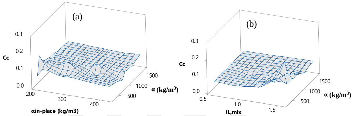
Şekil 4.70. Sıkışma indisinin a) \alpha_{in-place} - \alpha ve b) I_{L,mix} - \alpha arasındaki ilişkiler (Küçük ölçekli DKK, 56 gün)
