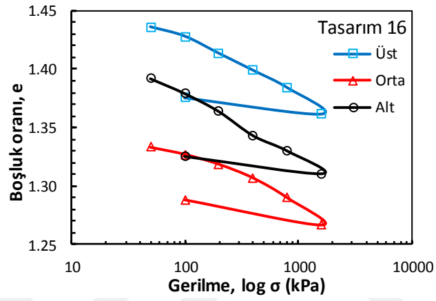
Şekil Ek 4.32. BÖ-16 numaralı kolona ait konsolidasyon deney sonucu (Büyük ölçekli DKK, 56 gün)
