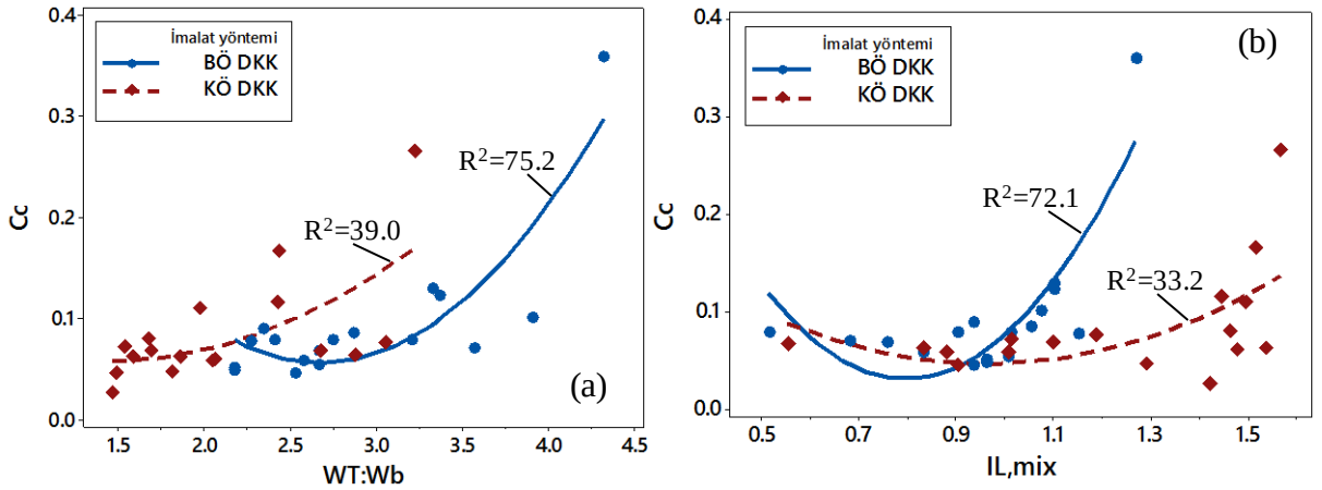
Şekil 4.101. Sıkıştırma indisinin a) W_T:W_b ve b) I_{L,mix} ile ilişkileri (Küçük ve büyük ölçekli DKK, 56 gün)
