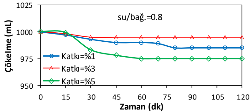
Şekil 3.47. Optima 100 katkısı ile yapılan sedimentasyon deneyi sonuçları (UKO=%60, su/bağlayıcı=0.8)
