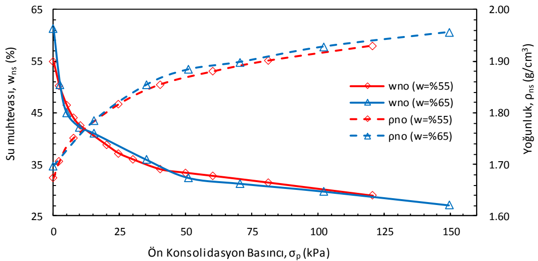
Şekil 3.31. Zeminin yoğunluk-su muhtevası-ön konsolidasyon basıncı ilişkisi ( w_{no} ve w_{ns} zeminin başlangıç ve son durumdaki su muhtevaları, \rho_{no} ve \rho_{ns} zeminin başlangıçtaki ve son durumdaki doğal yoğunluklarını göstermektedir)
