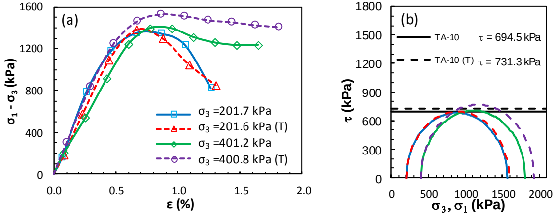
Şekil Ek 6.10. KÖ-10 numaralı tasarım: a) deviator gerilme-birim deformasyon grafikleri ve b) Mohr daireleri (Küçük ölçekli DKK, UU, 7 gün)
