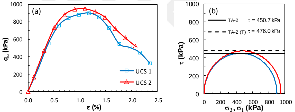
Şekil Ek 5.2. KÖ-2 numaralı tasarım: a) gerilme-birim deformasyon grafikleri ve b) Mohr daireleri (Küçük ölçekli DKK, UCS, 7 gün)
