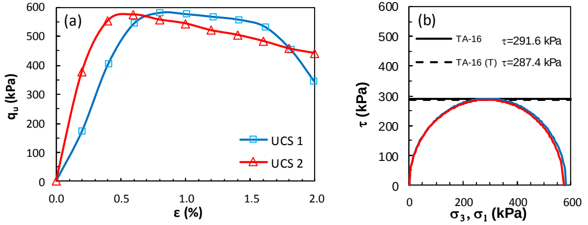
Şekil Ek 5.16. KÖ-16 numaralı tasarım: a) gerilme-birim deformasyon grafikleri ve b) Mohr daireleri (Küçük ölçekli DKK, UCS, 7 gün)
