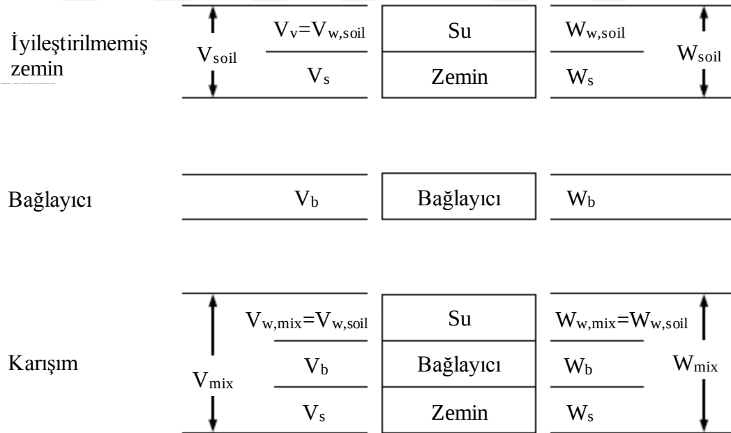
Şekil 2.10. Kuru karıştırma yöntemi için kullanılan faz diyagramı
