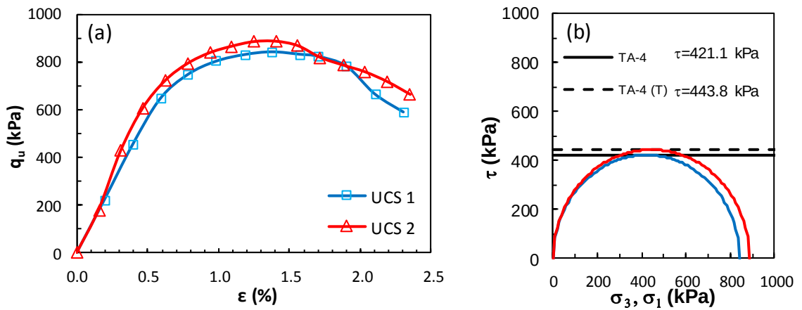
Şekil Ek 5.36. KÖ-4 numaralı tasarım: a) gerilme-birim deformasyon grafikleri ve b) Mohr daireleri (Küçük ölçekli DKK, UCS, 56 gün)
