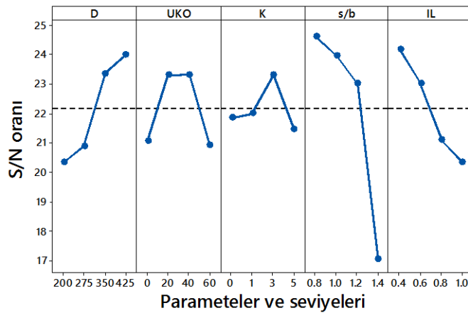
Şekil 4.68. Sıkışma indisi ( C_c ) için elde edilen S/N grafiği (Küçük ölçekli DKK, konsolidasyon, 56 gün)
