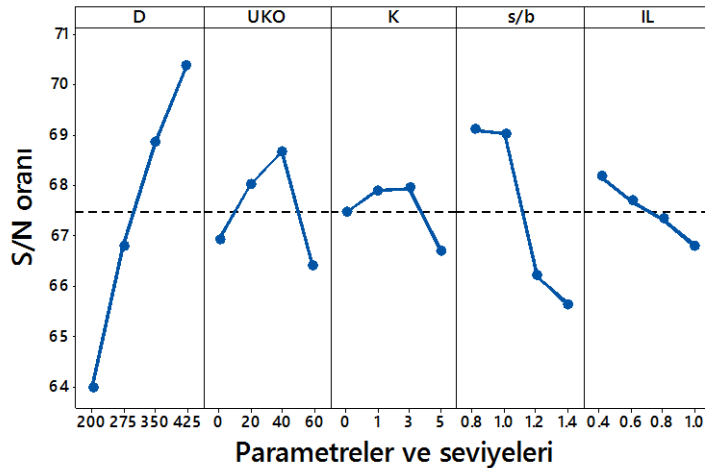
Şekil 4.33. Kolon dayanımı ( q_{uu} ) için elde edilen S/N grafiği (Büyük ölçekli DKK, UU, 56 gün)
