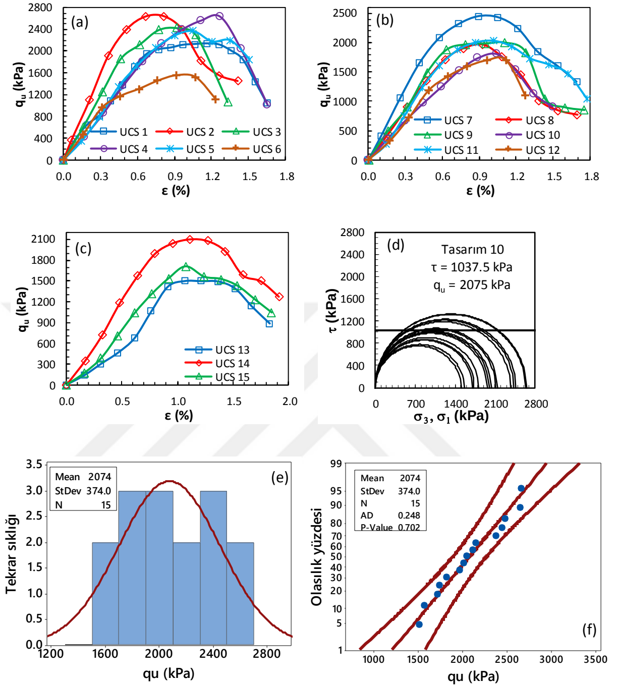
Şekil Ek 2.10. BÖ-10 numaralı kolona ait gerilme-birim deformasyon grafikleri: a) kolon üst bölgesi, b) kolon orta bölgesi, c) kolon alt bölgesi ve d) Mohr daireleri, e) histogram grafiği, f) olasılık grafiği (Büyük ölçekli DKK, UCS, 28 gün)
