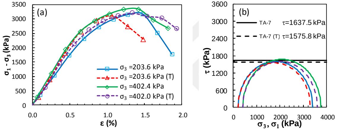
Şekil Ek 6.23. KÖ-7 numaralı tasarım: a) deviator gerilme-birim deformasyon grafikleri ve b) Mohr daireleri (Küçük ölçekli DKK, UU, 28 gün)
