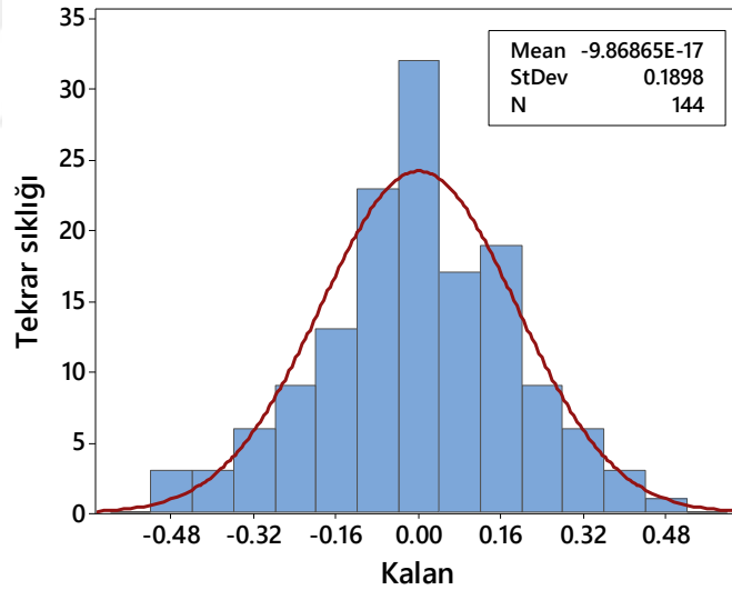
Şekil 4.110. RI sonuçları için geliştirilen modeldeki hataların histogram grafiği (Küçük ölçekli DKK)
