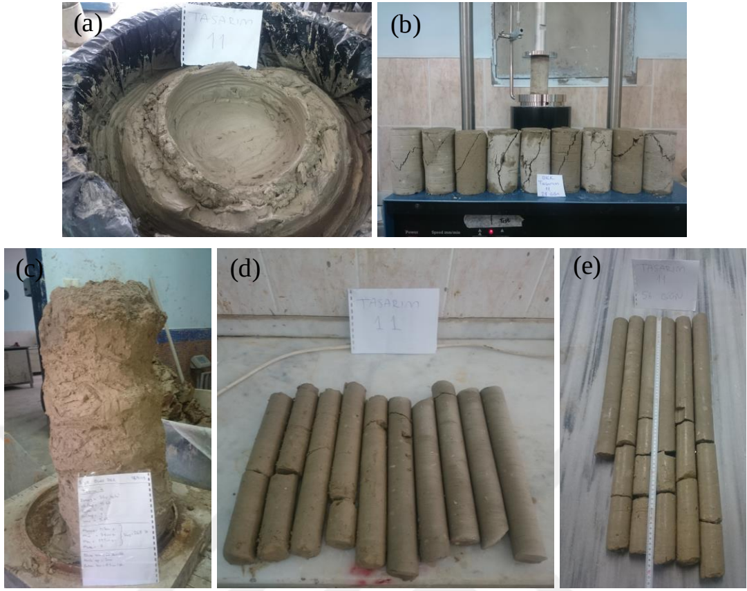
Şekil 3.62. Büyük ölçekli DKK, Tasarım 11: a) imalat sonrası görünüm, b) kayma yüzeyleri, c) imal edilen kolon, d) 28 ve e) 56 günlük karot numuneleri (büyük ölçekli DKK)
