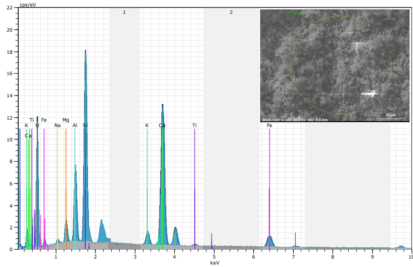
Şekil 4.130. Tasarım 4'e ait EDX analizi sonucu (Küçük ölçekli DKK, 56 gün)
