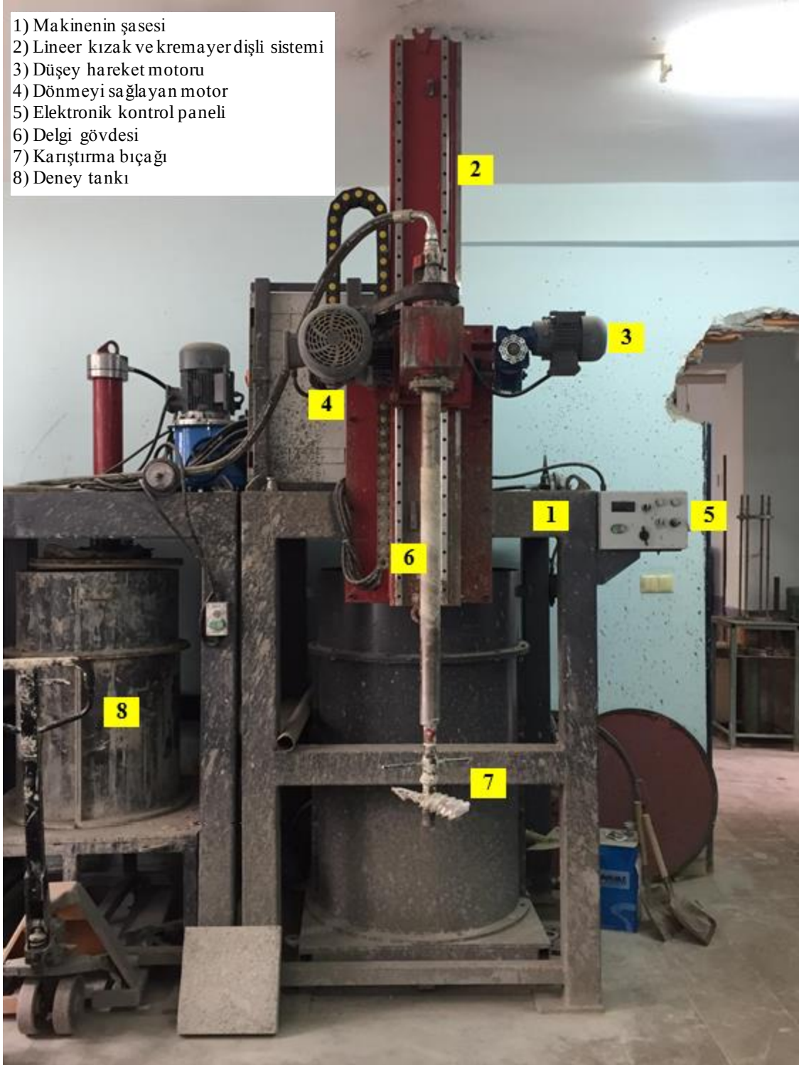
Şekil 3.17. Laboratuvar tipi derin karıştırma makinesinin imal edilmiş hali
