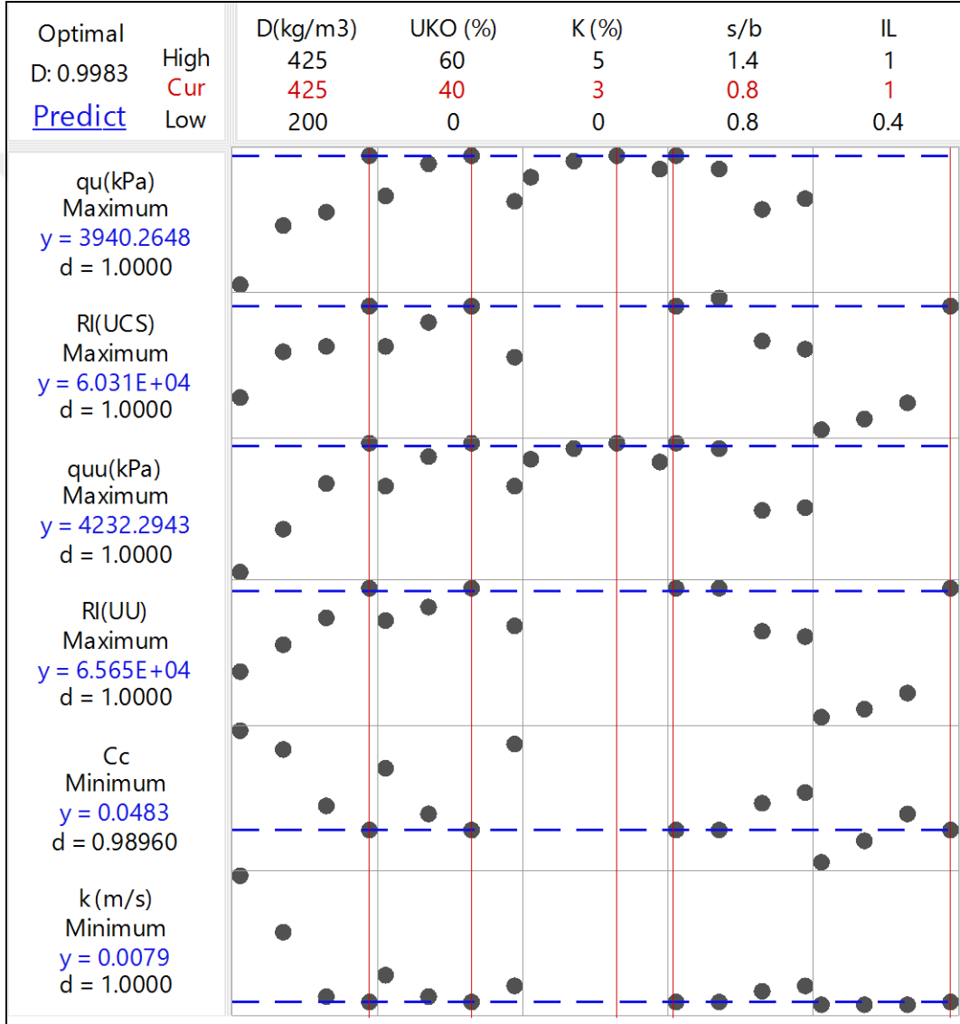
Şekil 4.78. Optimizasyon grafiği (Büyük ölçekli DKK, 56 gün)
