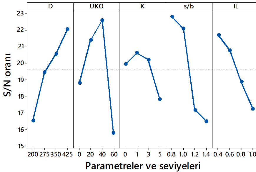
Şekil 4.39. Sıkışma indisi (Cc) için elde edilen S/N grafiği (Büyük ölçekli DKK, konsolidasyon, 28 gün)
