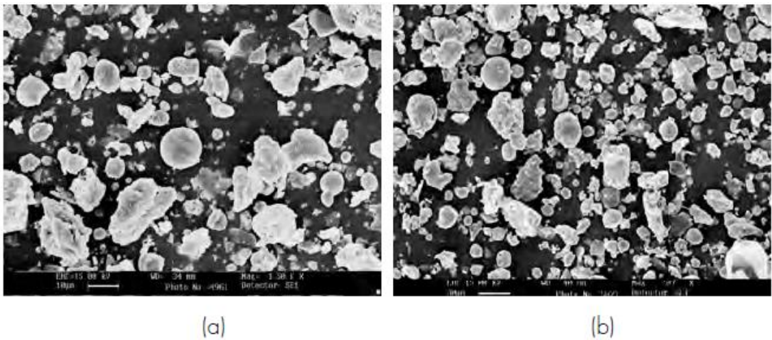
Şekil 3.14. Seyitömer uçucu külünün morfolojik yapısına ait fotoğraflar: a) ve b) taneciklerin genel dağılımı (x500 ve x1500) (Türker ve ark., 2009)
