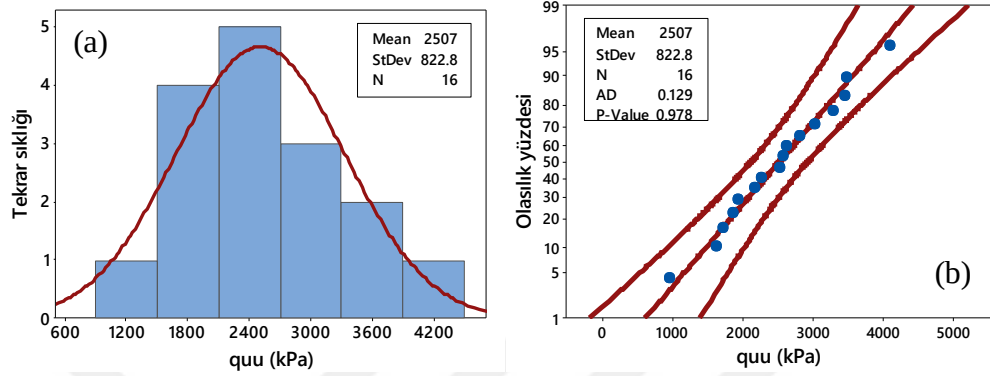
Şekil 4.32. Kolon dayanımı için elde edilen a) histogram grafiği ve b) normalolasılık grafiği (Büyük ölçekli DKK, UU, 56 gün)
