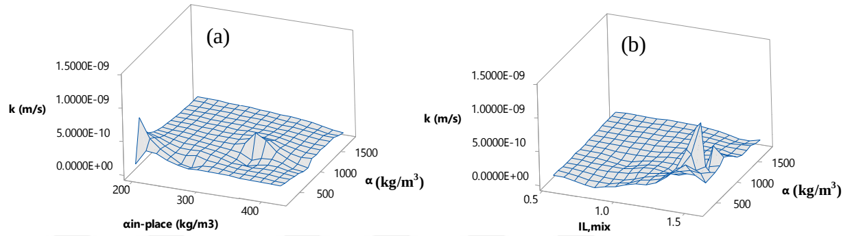
Şekil 4.75. Permeabilite katsayısının a) \alpha_{in-place} - \alpha ve b) IL_{mix} - \alpha arasındaki ilişkiler (Küçük ölçekli DKK, 56 gün)
