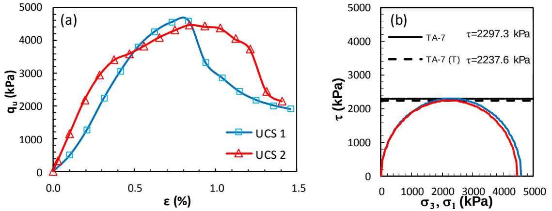
Şekil Ek 5.39. KÖ-7 numaralı tasarım: a) gerilme-birim deformasyon grafikleri ve b) Mohr daireleri (Küçük ölçekli DKK, UCS, 56 gün)
