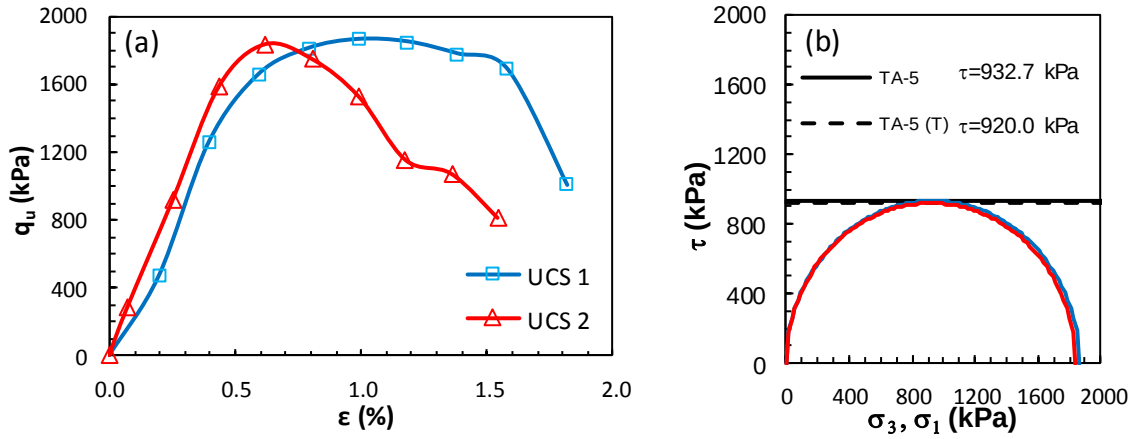
Şekil Ek 5.37. KÖ-5 numaralı tasarım: a) gerilme-birim deformasyon grafikleri ve b) Mohr daireleri (Küçük ölçekli DKK, UCS, 56 gün)
