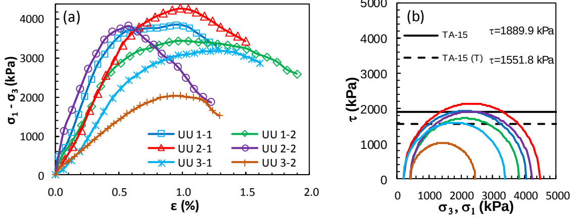
Şekil Ek 3.31. BÖ-15 numaralı kolona ait UU deney sonuçları: a) deviator gerilme-birim boy kısalması grafikleri, b) Mohr daireleri ile kırılma zarfları (Büyük ölçekli DKK, UU, 56 gün)
