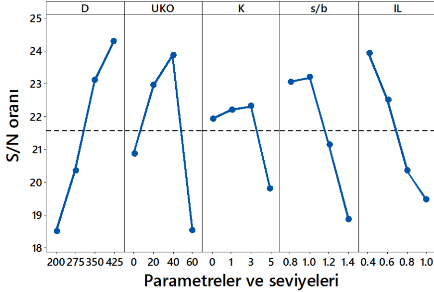
Şekil 4.40. Cc için elde edilen S/N grafiği (Büyük ölçekli DKK, konsolidasyon, 56 gün)
