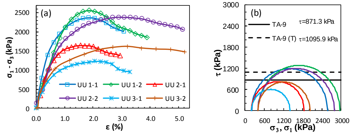
Şekil Ek 3.9. BÖ-9 numaralı kolona ait UU deney sonuçları: a) deviator gerilme-birim boy kısalması grafikleri, b) Mohr daireleri ile kırılma zarfları (Büyük ölçekli DKK, UU, 28 gün)
