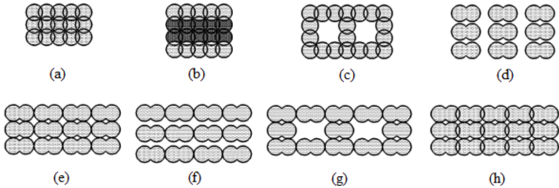
Şekil 2.9. Derin karıştırma kolon tipleri: a) blok tipi, b) duvar tipi, c) kafes tipi, d) kolon tipi, e) kesişen kolon tipi, f) kesişen duvar tipi, g) kesişen kafes tipi, h) kesişen blok tipi
