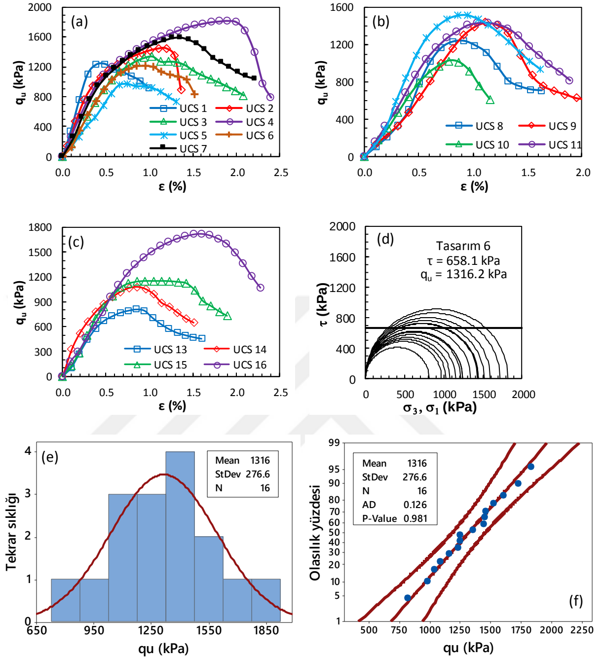
Şekil Ek 2.6. BÖ-6 numaralı kolona ait gerilme-birim deformasyon grafikleri: a) kolon üst bölgesi, b) kolon orta bölgesi, c) kolon alt bölgesi ve d) Mohr daireleri, e) histogram grafiği, f) olasılık grafiği (Büyük ölçekli DKK, UCS, 28 gün)
