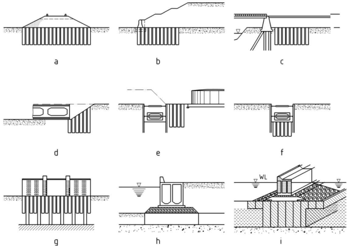
Şekil 2.8. Derin karıştırma yönteminin uygulama alanları: a) yoldolgu altında oturmalara kontrol etmek, duraylılığı sağlamak, b) şev tabanının stabilitesinde, c) köprü ayağında farklı oturmalara karşı, d) yamaç eğiminin stabilitesini sağlamak, e) komşu yapılardan gelen etkileri azaltmak, f) destekli kazılarda taban kabarmasına karşı, g) kazıklı temellerin yanıl direncini artırmak için, h) deniz tabanında taşıma gücünü artırmak amacıyla, i) dalgakıran altında taşıma gücünün artırılması amacıyla
