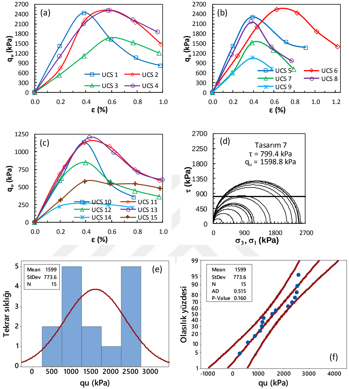
Şekil Ek 2.7. BÖ-7 numaralı kolona ait gerilme-birim deformasyon grafikleri: a) kolon üst bölgesi, b) kolon orta bölgesi, c) kolon alt bölgesi ve d) Mohr daireleri, e) histogram grafiği, f) olasılık grafiği (Büyük ölçekli DKK, UCS, 28 gün)
