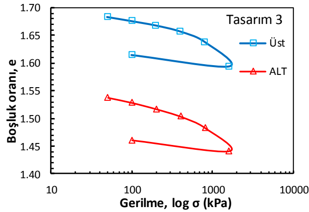
Şekil Ek 4.3. BÖ-3 numaralı kolona ait konsolidasyon deney sonucu (Büyük ölçekli DKK, 28 gün)
