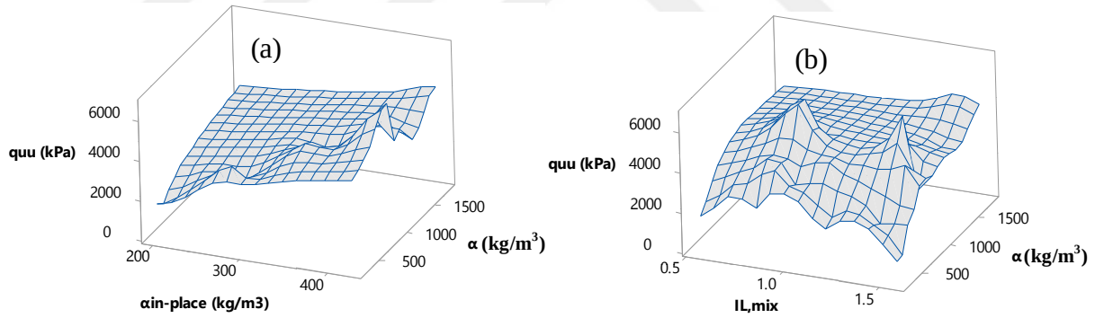
Şekil 4.65. Üç eksenli basınç dayanımının a) \alpha_{in-place} - \alpha ve b) IL_{mix} - \alpha arasındaki ilişkiler (Küçük ölçekli DKK, UU, 56 gün)
