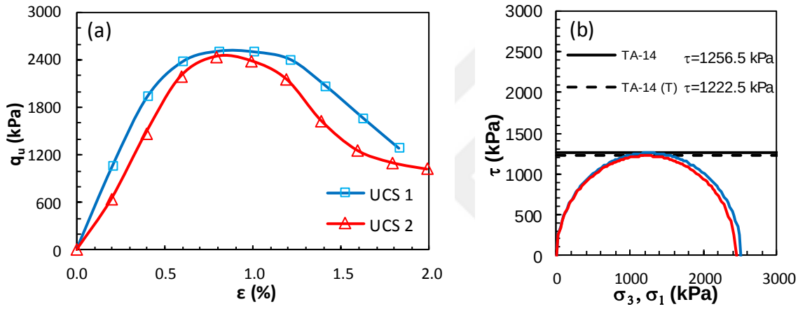
Şekil Ek 5.14. KÖ-14 numaralı tasarım: a) gerilme-birim deformasyon grafikleri ve b) Mohr daireleri (Küçük ölçekli DKK, UCS, 7 gün)
