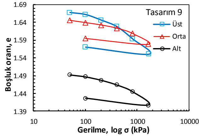
Şekil Ek 4.9. BÖ-9 numaralı kolona ait konsolidasyon deney sonucu (Büyük ölçekli DKK, 28 gün)
