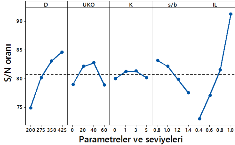
Şekil 4.63. Zemin iyileştirme derecesi için elde edilen S/N grafiği (Küçük ölçekli DKK, UU, 56 gün)
