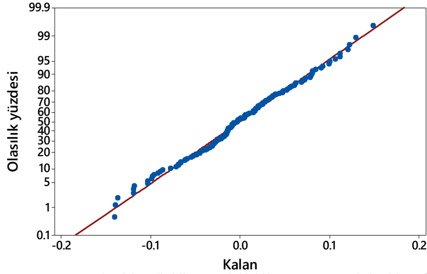
Şekil 4.107. Dayanım sonuçları için geliştirilen modeldeki hataların normal olasılık grafiği (Küçük ölçekli DKK)
