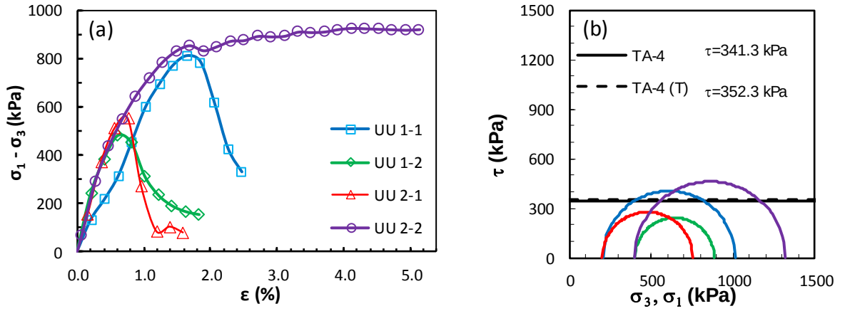
Şekil Ek 3.4. BÖ-4 numaralı kolona ait UU deney sonuçları: a) deviator gerilme-birim boy kısalması grafikleri, b) Mohr daireleri ile kırılma zarfları (Büyük ölçekli DKK, UU, 28 gün)
