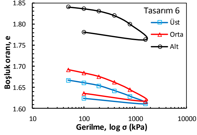
Şekil Ek 4.22. BÖ-6 numaralı kolona ait konsolidasyon deney sonucu (Büyük ölçekli DKK, 56 gün)
