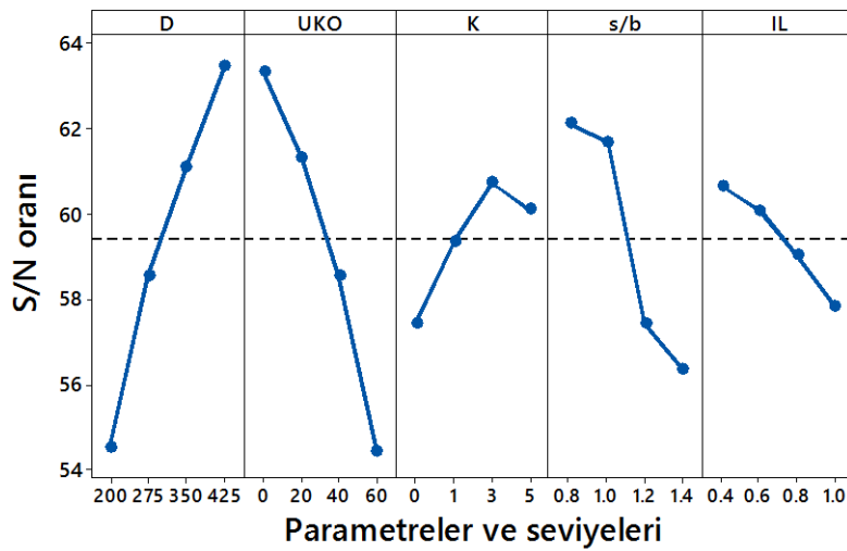
Şekil 4.49. Serbest basınç dayanımı için elde edilen S/N grafiği (Küçük ölçekli DKK, UCS, 7 gün)
