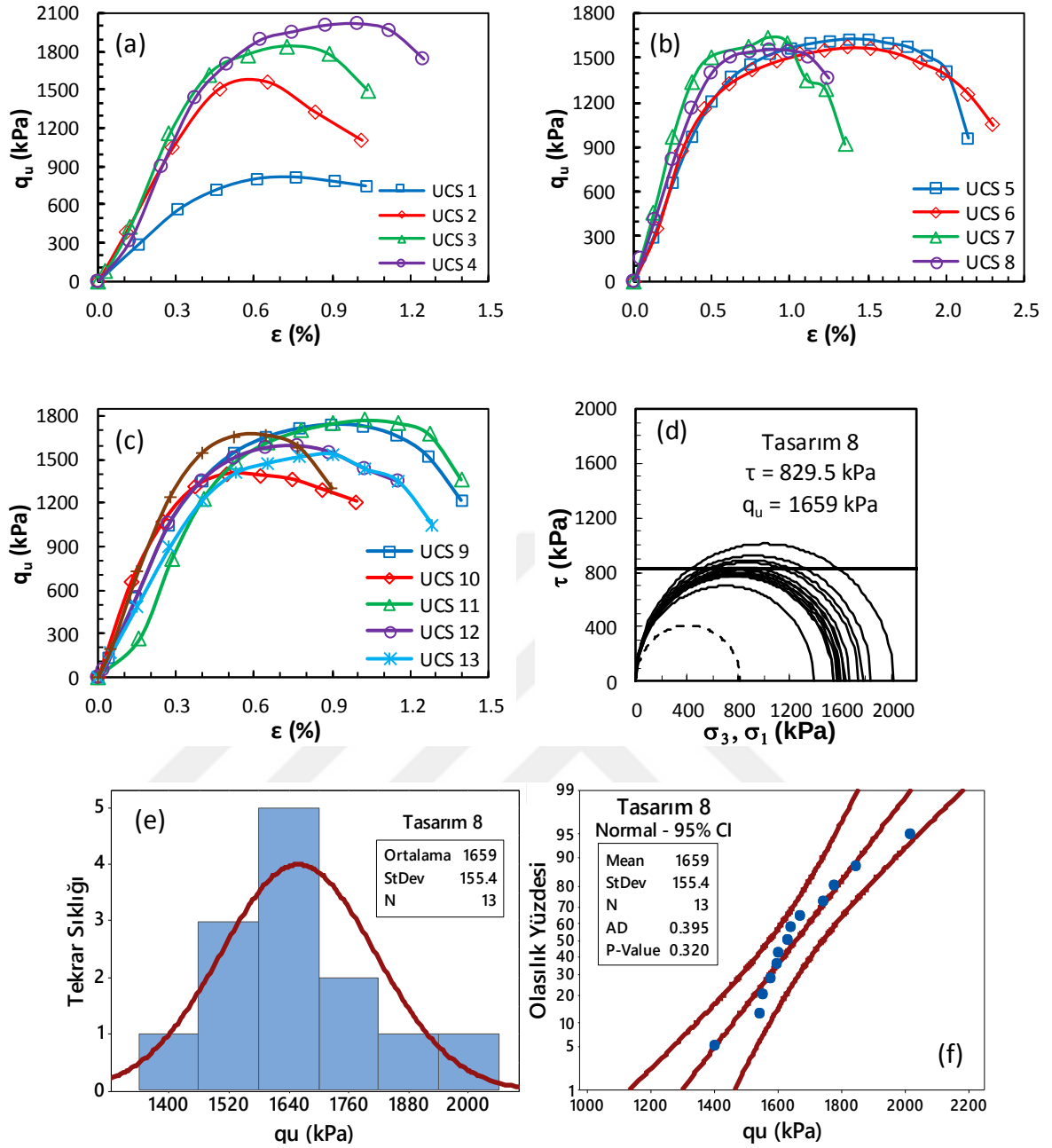
Şekil Ek 1.8. SP-8 numaralı kolona ait gerilme-birim deformasyon grafikleri: a) kolon alt bölgesi, b) kolon orta bölgesi, c) kolon üst bölgesi ve d) Mohr daireleri, e) histogram grafiği, f) olasılık grafiği (Not: UCS 1 deneyi ortalamaya katılmamıştır) (Sistem parametreleri, UCS, 28 gün)
