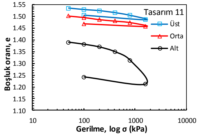
Şekil Ek 4.27. BÖ-11 numaralı kolona ait konsolidasyon deney sonucu (Büyük ölçekli DKK, 56 gün)
