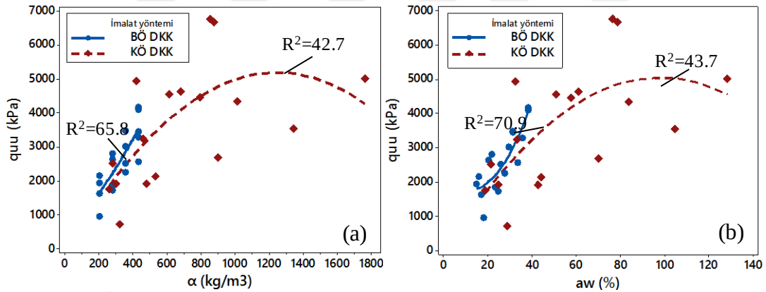
Şekil 4.98. Üç eksenli basınç dayanımının a) \alpha ve b) a_w ile ilişkileri (Küçük ve büyük ölçekli DKK, 56 gün)
