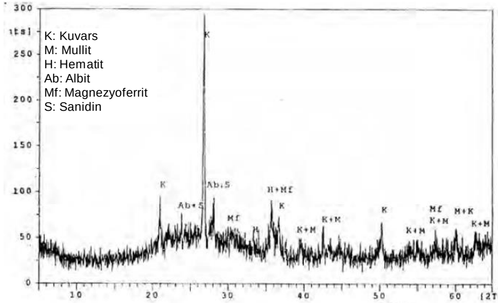
Şekil 3.13. Seyitömer uçucu külünün mineralojik bileşimine ait X-ışınları difraktogramı (Türker ve ark., 2009)
