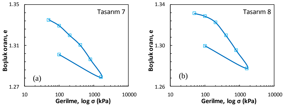
Şekil Ek 7.12. Küçük ölçekli DKK, konsolidasyon deneyi, 56 gün: a) Tasarım 7 ve b) Tasarım 8
