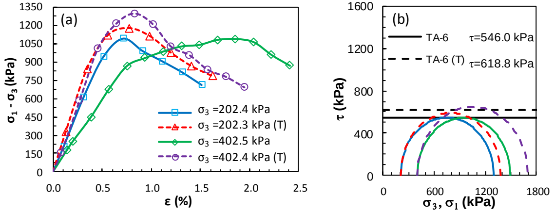
Şekil Ek 6.22. KÖ-6 numaralı tasarım: a) deviator gerilme-birim deformasyon grafikleri ve b) Mohr daireleri (Küçük ölçekli DKK, UU, 28 gün)
