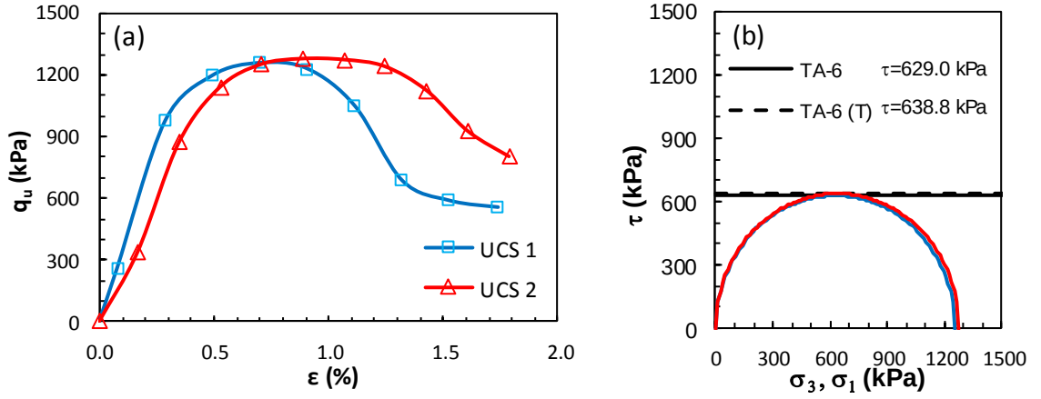
Şekil Ek 5.22. KÖ-6 numaralı tasarım: a) gerilme-birim deformasyon grafikleri ve b) Mohr daireleri (Küçük ölçekli DKK, UCS, 28 gün)
