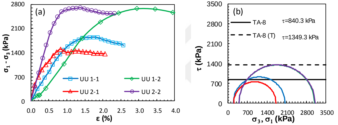
Şekil Ek 3.8. BÖ-8 numaralı kolona ait UU deney sonuçları: a) deviator gerilme-birim boy kısalması grafikleri, b) Mohr daireleri ile kırılma zarfları (Büyük ölçekli DKK, UU, 28 gün)
