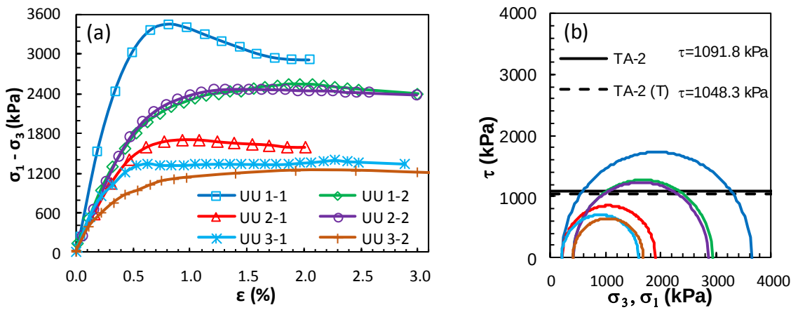
Şekil Ek 3.18. BÖ-2 numaralı kolona ait UU deney sonuçları: a) deviatör gerilme-birim boy kısalması grafikleri, b) Mohr daireleri ile kırılma zarfları (Büyük ölçekli DKK, UU, 56 gün)
