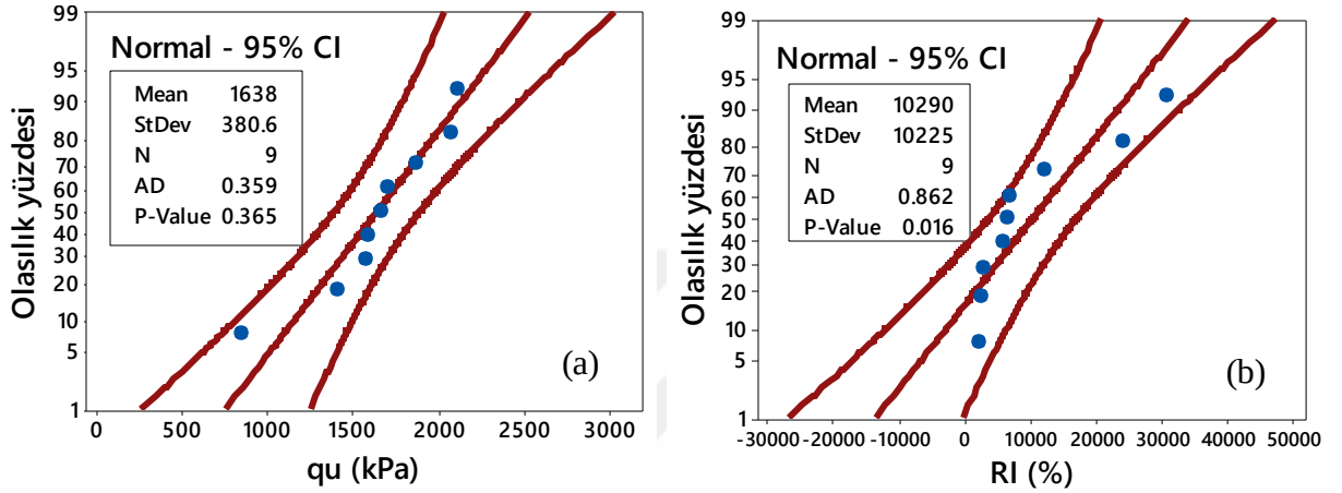
Şekil 4.11. a) Dayanım ve b) zemin iyileştirme oranı için normal olasılık grafikleri (Sistem parametrelerinin araştırılması)
