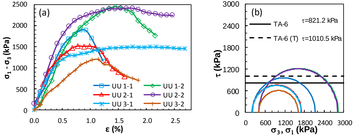
Şekil Ek 3.22. BÖ-6 numaralı kolona ait UU deney sonuçları: a) deviatör gerilme-birim boy kısalması grafikleri, b) Mohr daireleri ile kırılma zarfları (Büyük ölçekli DKK, UU, 56 gün)
