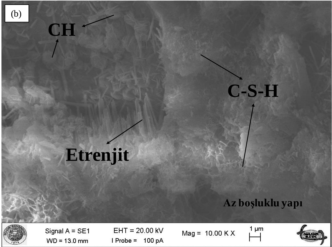
Şekil 4.126. Tasarım 14'e ait SEM görüntüleri: a) x5000, b) x10000 (Küçük ölçekli DKK, 56 gün)
