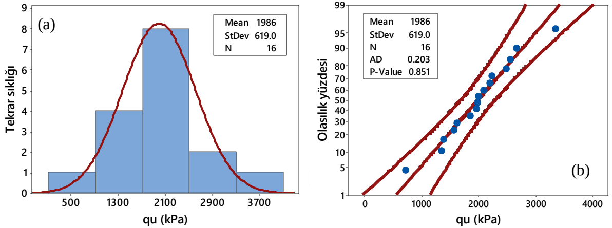
Şekil 4.29. Kolon dayanımı için elde edilen a) histogram grafiği ve b) normal olasılık grafiği (Büyük ölçekli DKK, UU, 28 gün)
