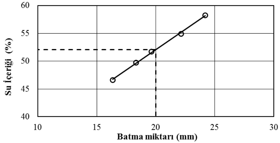
Şekil 3.6. Düşen koni yöntemi ile likit limit tayini
