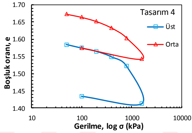
Şekil Ek 4.20. BÖ-4 numaralı kolona ait konsolidasyon deney sonucu (Büyük ölçekli DKK, 56 gün)
