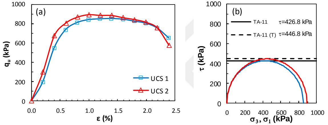
Şekil Ek 5.11. KÖ-11 numaralı tasarım: a) gerilme-birim deformasyon grafikleri ve b) Mohr daireleri (Küçük ölçekli DKK, UCS, 7 gün)
