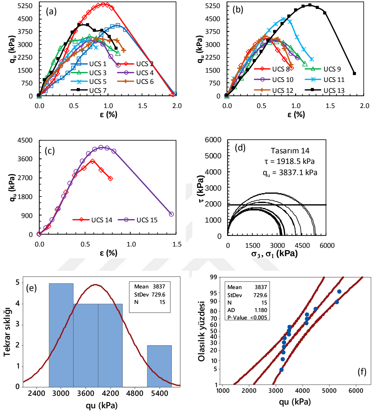
Şekil Ek 2.30. BÖ-14 numaralı kolona ait gerilme-birim deformasyon grafikleri: a) kolon üst bölgesi, b) kolon orta bölgesi, c) kolon alt bölgesi ve d) Mohr daireleri, e) histogram grafiği, f) olasılık grafiği (Büyük ölçekli DKK, UCS, 56 gün)
