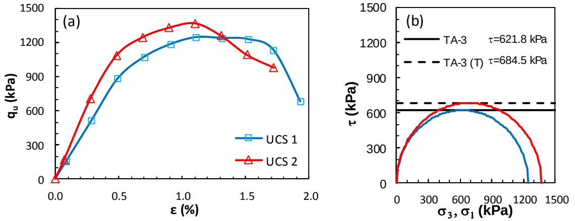
Şekil Ek 5.19. KÖ-3 numaralı tasarım: a) gerilme-birim deformasyon grafikleri ve b) Mohr daireleri (Küçük ölçekli DKK, UCS, 28 gün)
