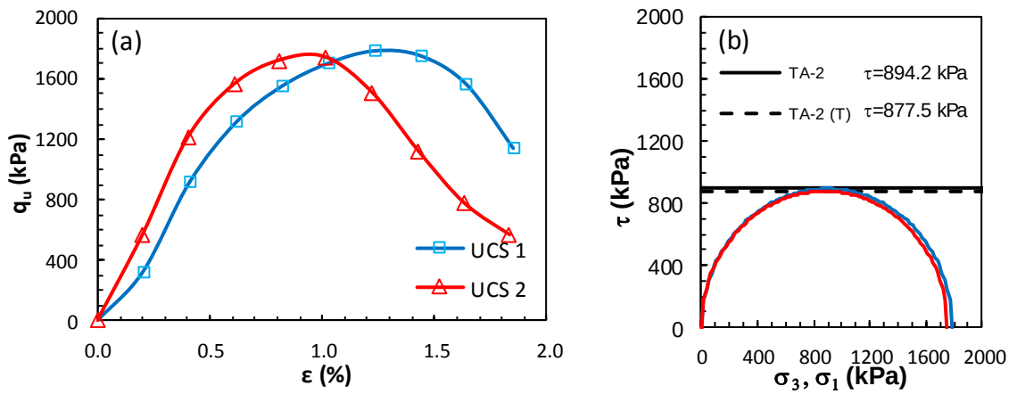
Şekil Ek 5.18. KÖ-2 numaralı tasarım: a) gerilme-birim deformasyon grafikleri ve b) Mohr daireleri (Küçük ölçekli DKK, UCS, 28 gün)
