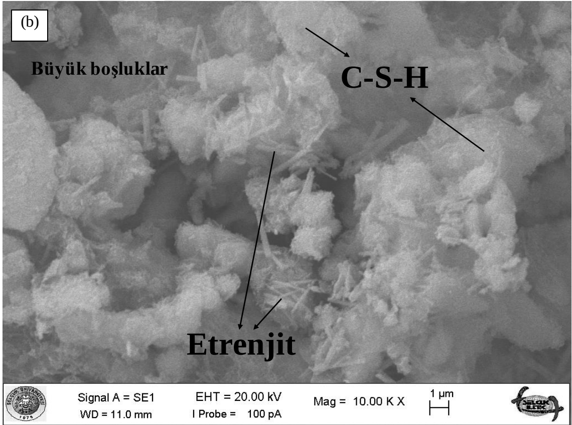
Şekil 4.124. Tasarım 4'e ait SEM görüntüsü: a) x5000, b) x10000 (Küçük ölçekli DKK, 56 gün)
