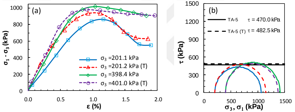
Şekil Ek 6.5. KÖ-5 numaralı tasarım: a) deviyör gerilme-birim deformasyon grafikleri ve b) Mohr daireleri (Küçük ölçekli DKK, UU, 7 gün)
