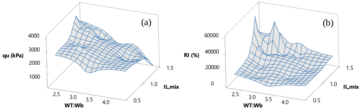
Şekil 4.28. W_T:W_b ile I_{L,mix} a) q_u ve b) RI arasındaki ilişki (Büyük ölçekli DKK, UCS, 56 gün)
