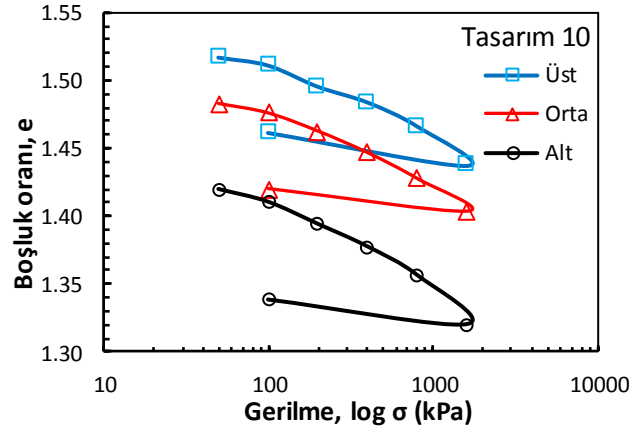
Şekil Ek 4.10. BÖ-10 numaralı kolona ait konsolidasyon deney sonucu (Büyük ölçekli DKK, 28 gün)
