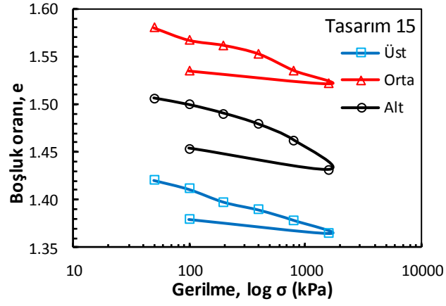
Şekil Ek 4.31. BÖ-15 numaralı kolona ait konsolidasyon deney sonucu (Büyük ölçekli DKK, 56 gün)
