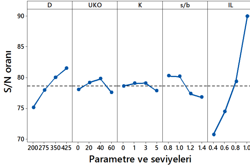
Şekil 4.34. Zemin iyileştirme derecesi için elde edilen S/N grafiği (Büyük ölçekli DKK, UU, 56 gün)
