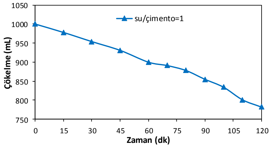
Şekil 4.1. Çimento enjeksiyonunun çökme deneyi sonucu
