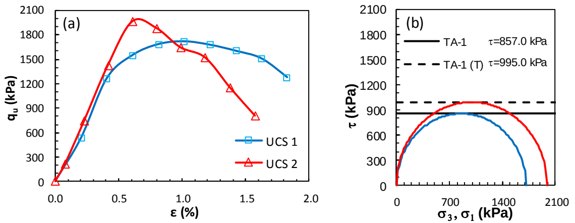
Şekil Ek 5.33. KÖ-1 numaralı tasarım: a) gerilme-birim deformasyon grafikleri ve b) Mohr daireleri (Küçük ölçekli DKK, UCS, 56 gün)
