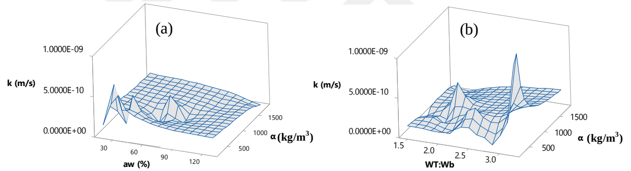
Şekil 4.76. Permeabilite katsayısının a) a_w - \alpha ve b) WT:Wb - \alpha arasındaki ilişkiler (Küçük ölçekli DKK, 56 gün)
