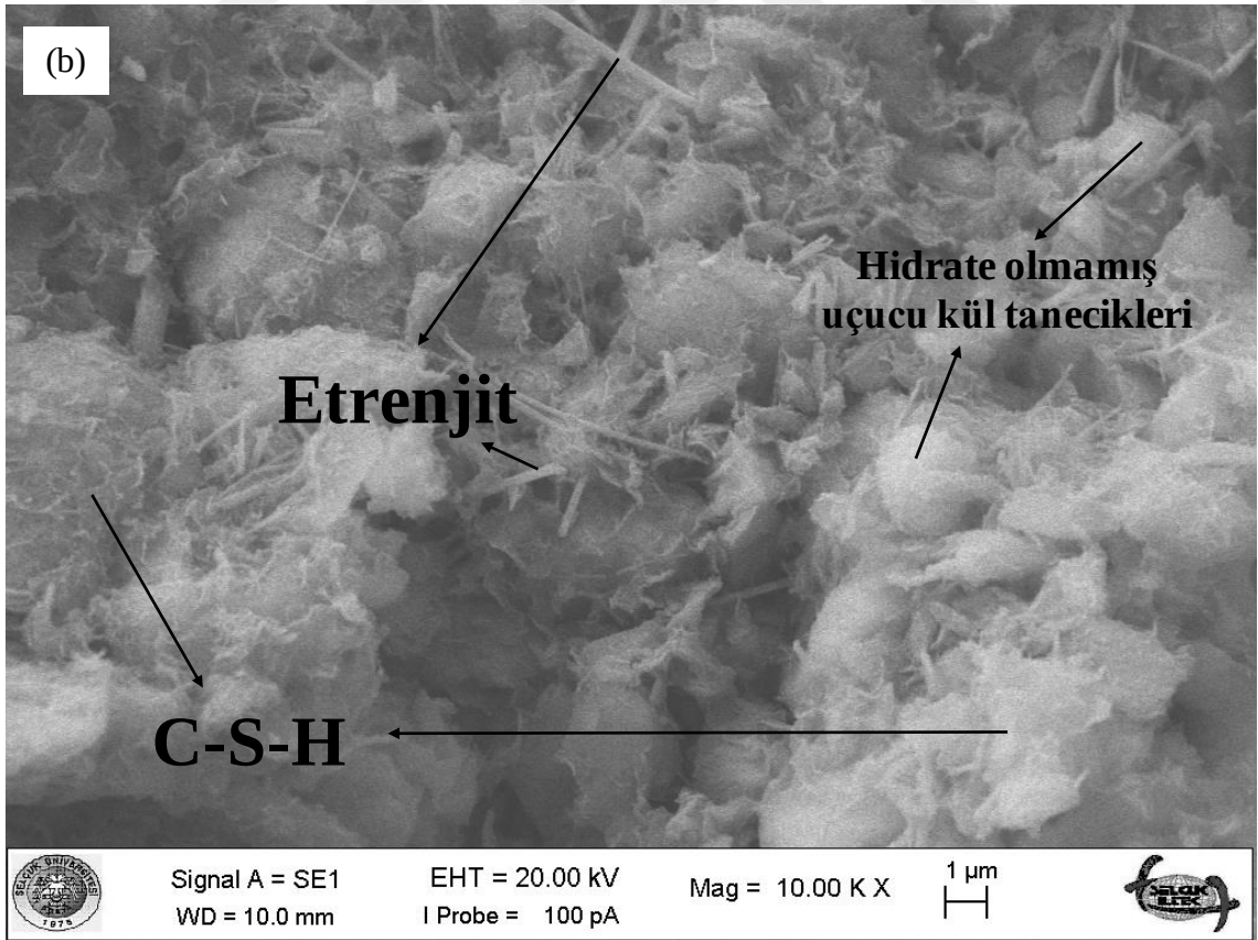
Şekil 4.136. Tasarım 4'e ait SEM görüntüleri: a) x5000, b) x10000 (Büyük ölçekli DKK, 56 gün)
