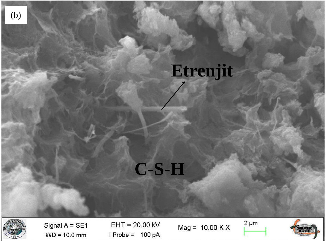
Şekil 4.140. Optimum tasarıma ait SEM görüntüleri: a) x5000, b) x10000 (Büyük ölçekli DKK, 56 gün)
