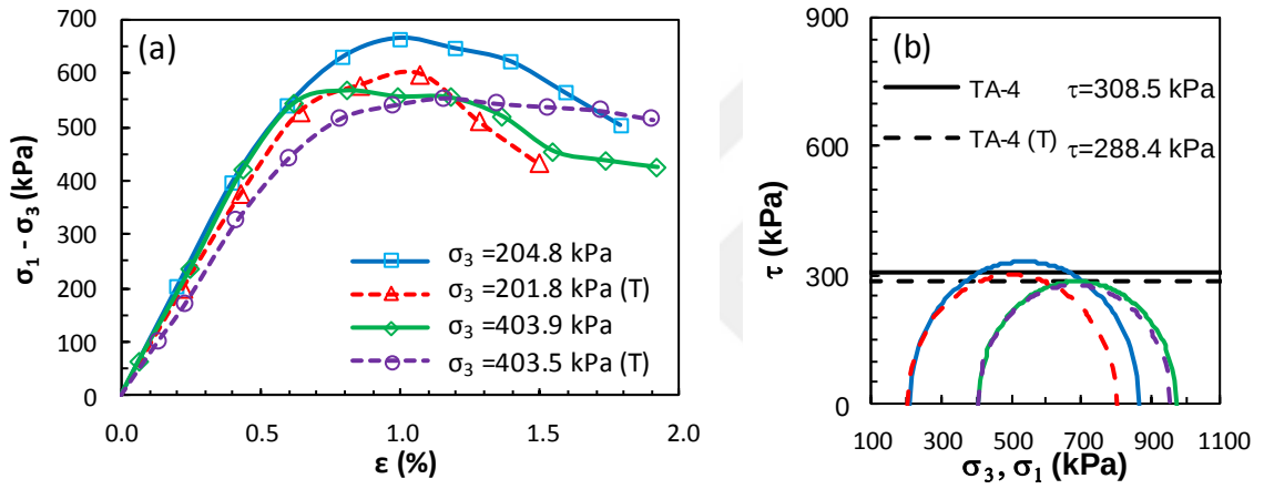
Şekil Ek 6.20. KÖ-4 numaralı tasarım: a) deviator gerilme-birim deformasyon grafikleri ve b) Mohr daireleri (Küçük ölçekli DKK, UU, 28 gün)
