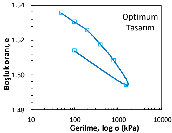
Şekil 4.94. Optimum tasarıma ait konsolidasyon deney sonuçları (Küçük ölçekli DKK, 28 gün)
