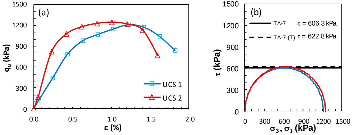
Şekil Ek 5.7. KÖ-7 numaralı tasarım: a) gerilme-birim deformasyon grafikleri ve b) Mohr daireleri (Küçük ölçekli DKK, UCS, 7 gün)
