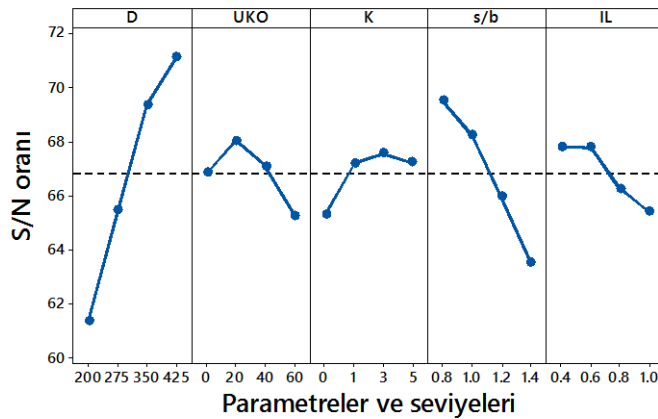
Şekil 4.60. Üç eksenli basınç dayanımı için elde edilen S/N grafiği (Küçük ölçekli DKK, UU, 28 gün)
