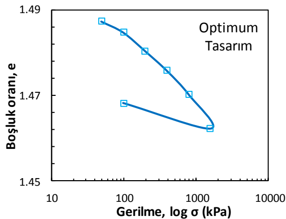
Şekil 4.95. Optimum tasarıma ait konsolidasyon deney sonuçları (Büyük ölçekli DKK, 56 gün)
