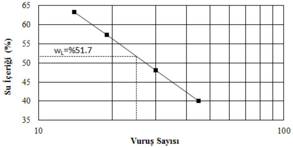
Şekil 3.5. Casagrande yöntemi ile likit limit tayini
