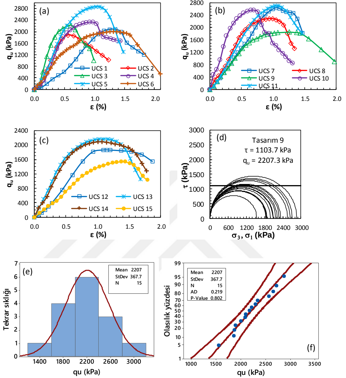
Şekil Ek 2.25. BÖ-9 numaralı kolona ait gerilme-birim deformasyon grafikleri: a) kolon üst bölgesi, b) kolon orta bölgesi, c) kolon alt bölgesi ve d) Mohr daireleri, e) histogram grafiği, f) olasılık grafiği (Büyük ölçekli DKK, UCS, 56 gün)
