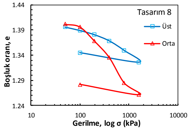
Şekil Ek 4.24. BÖ-8 numaralı kolona ait konsolidasyon deney sonucu (Büyük ölçekli DKK, 56 gün)
