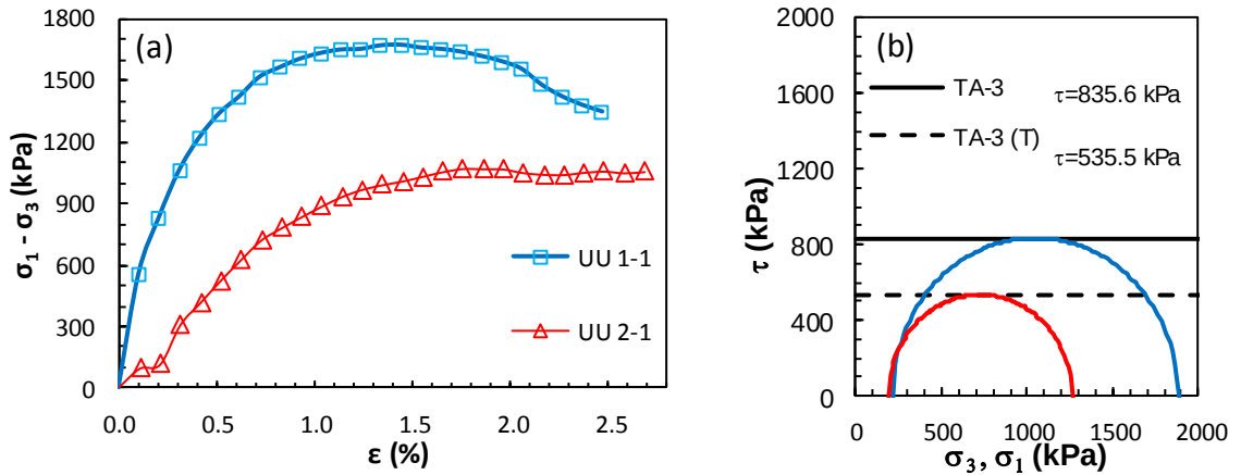
Şekil Ek 3.3. BÖ-3 numaralı kolona ait UU deney sonuçları: a) deviator gerilme-birim boy kısalması grafikleri, b) Mohr daireleri ile kırılma zarfları (Büyük ölçekli DKK, UU, 28 gün)
