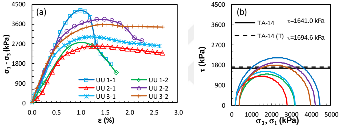
Şekil Ek 3.14. BÖ-14 numaralı kolona ait UU deney sonuçları: a) deviator gerilme-birim boy kısalması grafikleri, b) Mohr daireleri ile kırılma zarfları (Büyük ölçekli DKK, UU, 28 gün)
