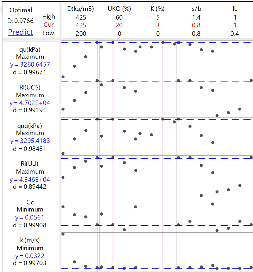
Şekil 4.77. Optimizasyon grafiği (Büyük ölçekli DKK, 28 gün)
