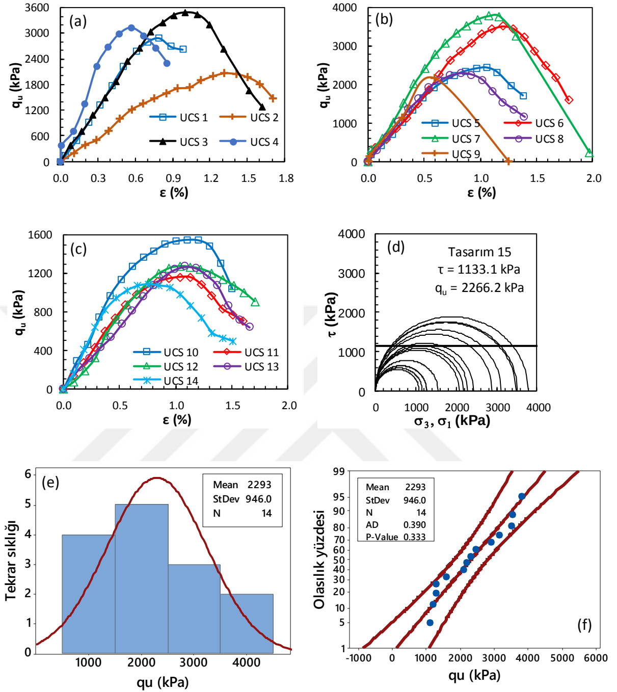
Şekil Ek 2.15. BÖ-15 numaralı kolona ait gerilme-birim deformasyon grafikleri: a) kolon üst bölgesi, b) kolon orta bölgesi, c) kolon alt bölgesi ve d) Mohr daireleri, e) histogram grafiği, f) olasılık grafiği (Büyük ölçekli DKK, UCS, 28 gün)
