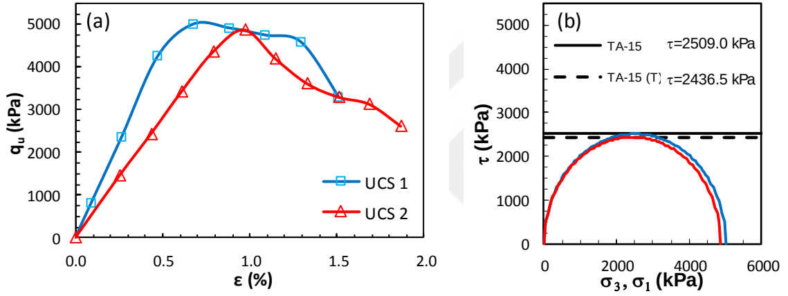
Şekil Ek 5.47. KÖ-15 numaralı tasarım: a) gerilme-birim deformasyon grafikleri ve b) Mohr daireleri (Küçük ölçekli DKK, UCS, 56 gün)
