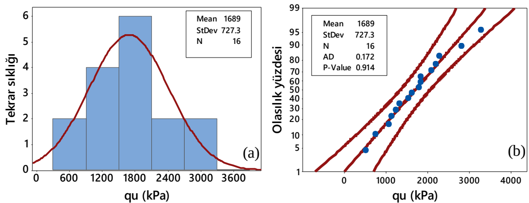
Şekil 4.18. Kolon dayanımı için elde edilen a) histogram grafiği ve b) normalolasılık grafiği (Büyük ölçekli DKK, UCS, 28 gün)
