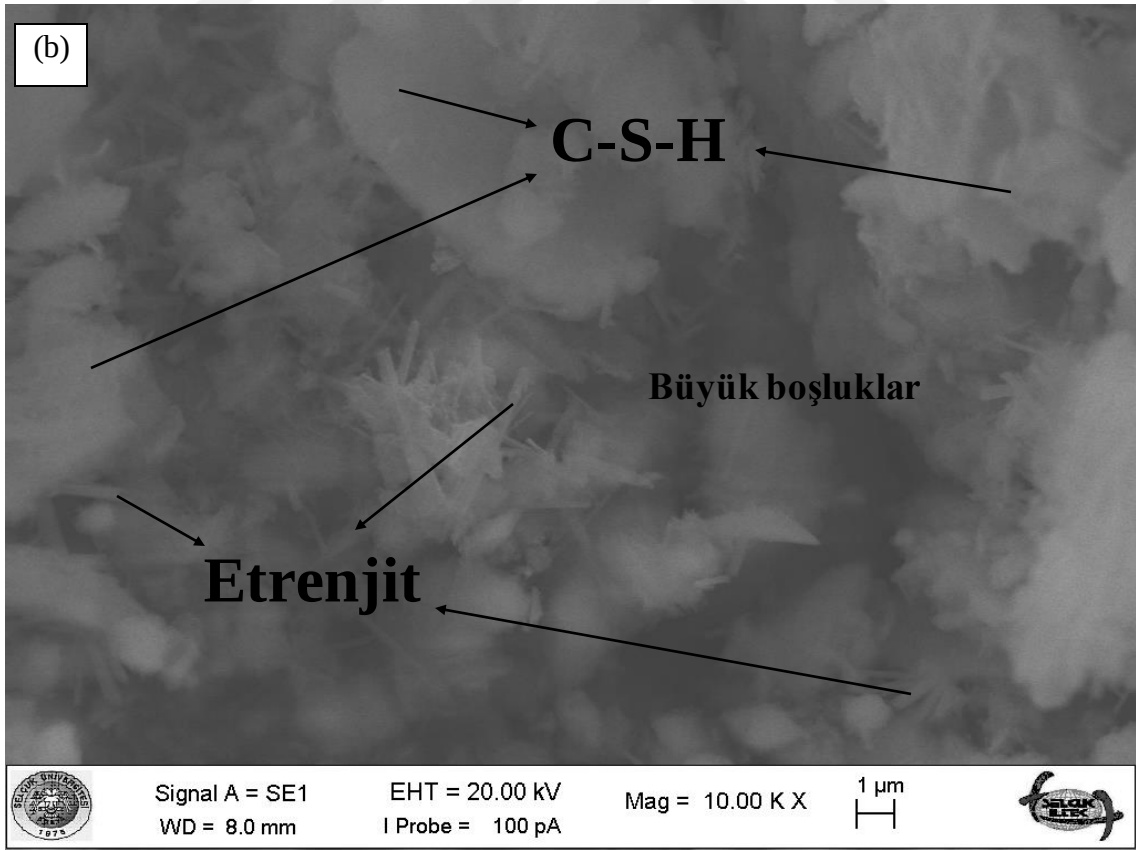
Şekil 4.123. Tasarım 4'e ait SEM görüntüsü: a) x5000, b) x10000 (Küçük ölçekli DKK, 28 gün)
