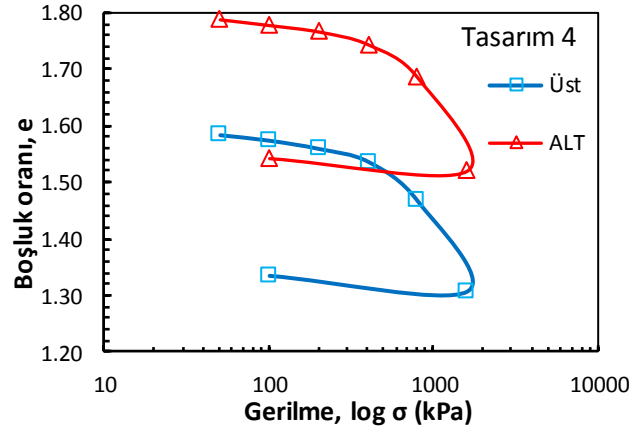
Şekil Ek 4.4. BÖ-4 numaralı kolona ait konsolidasyon deney sonucu (Büyük ölçekli DKK, 28 gün)
