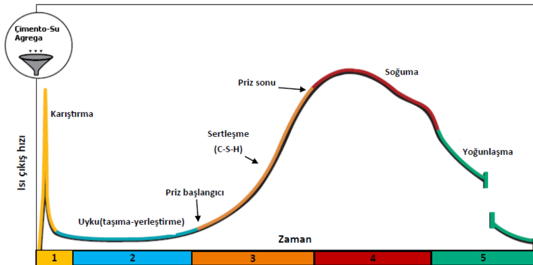
Şekil 2.3. Hidratasyon reaksiyonu süreçleri (Kosmatka ve ark., 2006)
