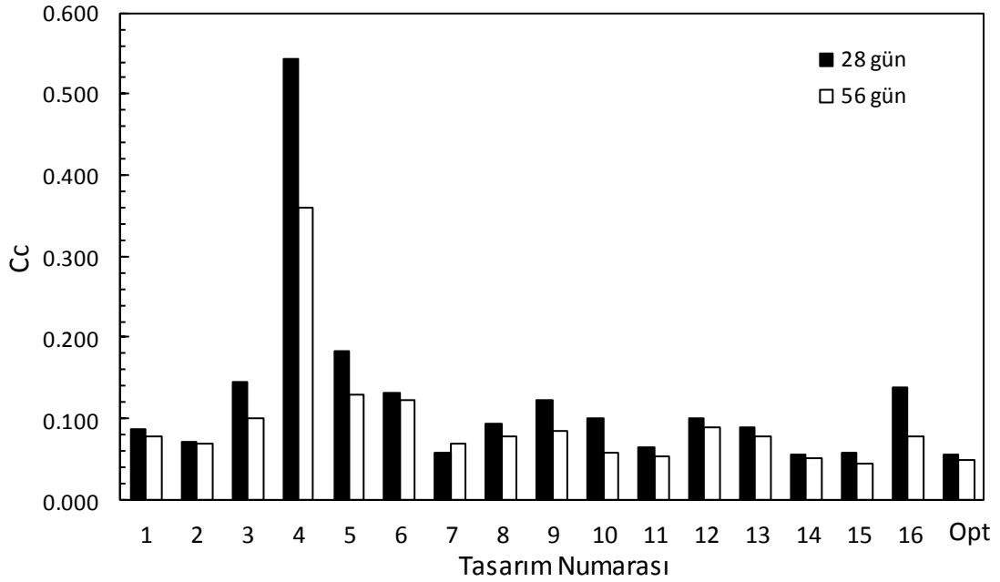
Şekil 4.41. Konsolidasyon deney sonuçları (Büyük ölçekli DKK)
