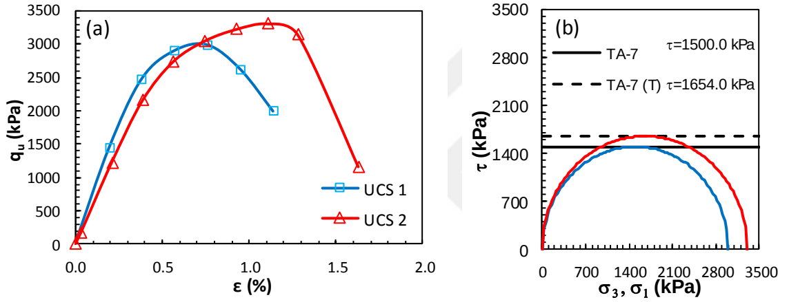
Şekil Ek 5.23. KÖ-7 numaralı tasarım: a) gerilme-birim deformasyon grafikleri ve b) Mohr daireleri (Küçük ölçekli DKK, UCS, 28 gün)
