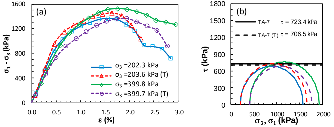
Şekil Ek 6.7. KÖ-7 numaralı tasarım: a) deviator gerilme-birim deformasyon grafikleri ve b) Mohr daireleri (Küçük ölçekli DKK, UU, 7 gün)
