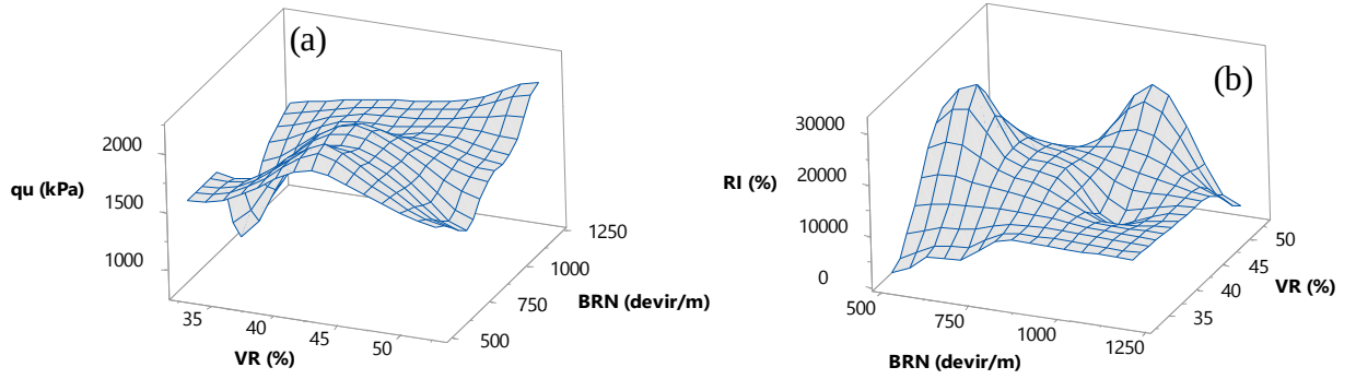
Şekil 4.10. VR ve BRN ile a) q_u ve b) RI arasındaki ilişki
