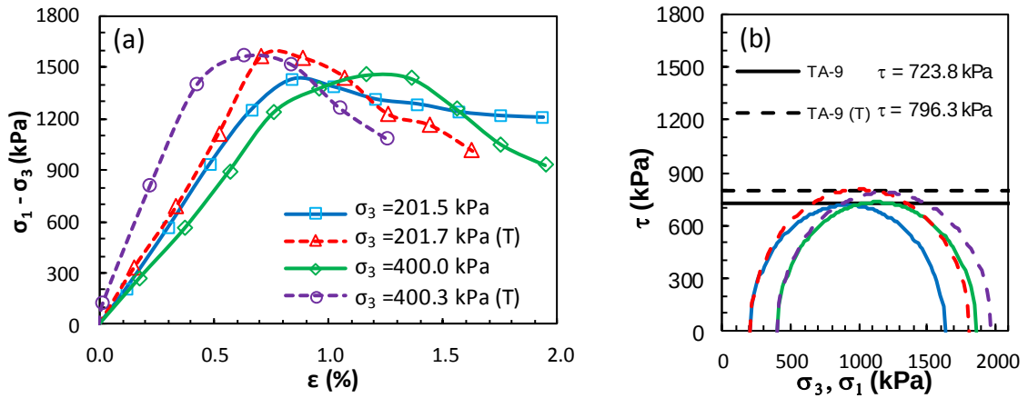
Şekil Ek 6.9. KÖ-9 numaralı tasarım: a) deviator gerilme-birim deformasyon grafikleri ve b) Mohr daireleri (Küçük ölçekli DKK, UU, 7 gün)
