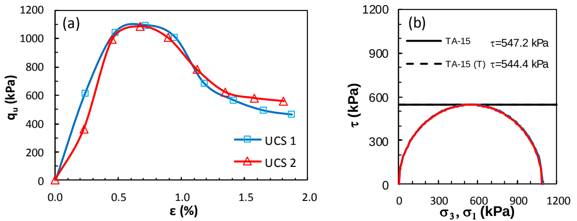
Şekil Ek 5.15. KÖ-15 numaralı tasarım: a) gerilme-birim deformasyon grafikleri ve b) Mohr daireleri (Küçük ölçekli DKK, UCS, 7 gün)
