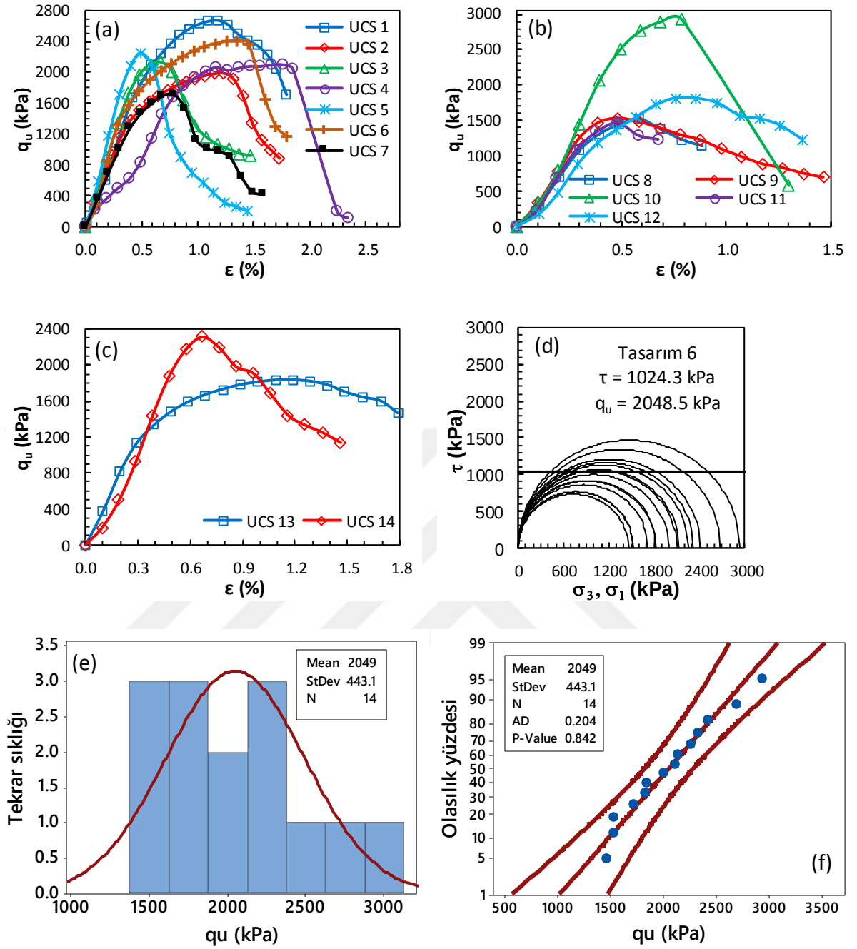
Şekil Ek 2.22. BÖ-6 numaralı kolona ait gerilme-birim deformasyon grafikleri: a) kolon üst bölgesi, b) kolon orta bölgesi, c) kolon alt bölgesi ve d) Mohr daireleri, e) histogram grafiği, f) olasılık grafiği (Büyük ölçekli DKK, UCS, 56 gün)
