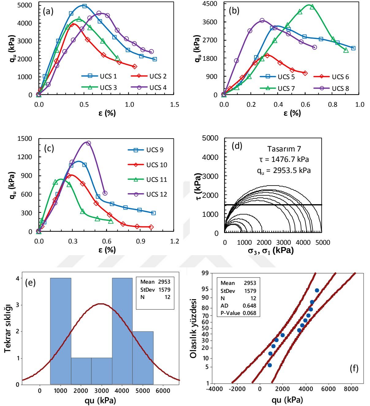
Şekil Ek 2.23. BÖ-7 numaralı kolona ait gerilme-birim deformasyon grafikleri: a) kolon üst bölgesi, b) kolon orta bölgesi, c) kolon alt bölgesi ve d) Mohr daireleri, e) histogram grafiği, f) olasılık grafiği (Büyük ölçekli DKK, UCS, 56 gün)
