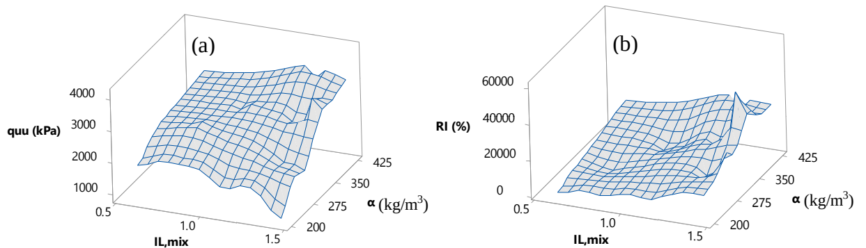
Şekil 4.36. I_{L,mix} ve \alpha ile a) q_{uu} ve b) RI arasındaki ilişki (Büyük ölçekli DKK, UU, 56 gün)
