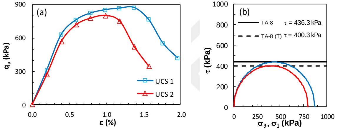
Şekil Ek 5.8. KÖ-8 numaralı tasarım: a) gerilme-birim deformasyon grafikleri ve b) Mohr daireleri (Küçük ölçekli DKK, UCS, 7 gün)
