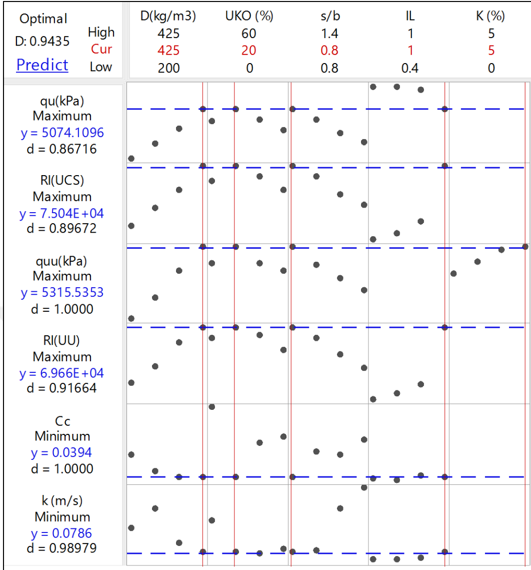
Şekil 4.87. Optimizasyon grafiği (Küçük ölçekli DKK, 28 gün) Not: k değeri 10^{-9} ile çarpılmalıdır.
