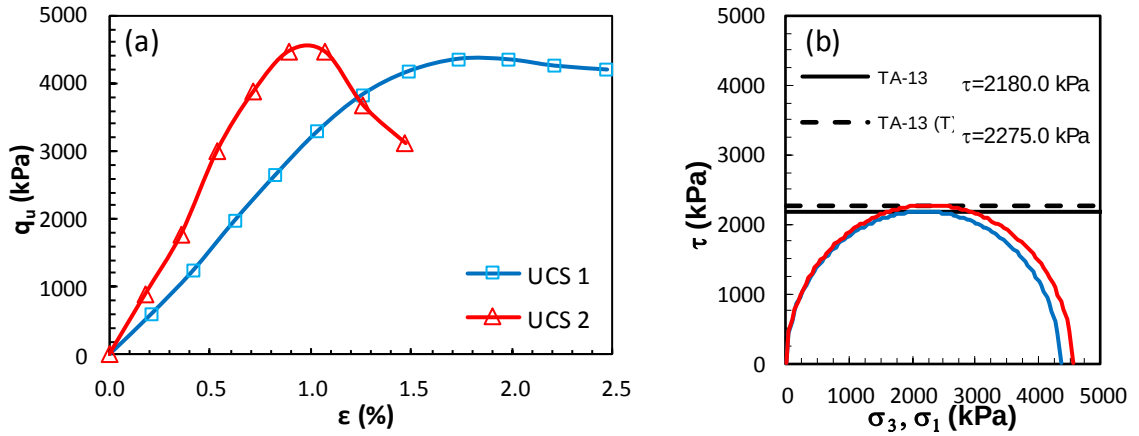
Şekil Ek 5.45. KÖ-13 numaralı tasarım: a) gerilme-birim deformasyon grafikleri ve b) Mohr daireleri (Küçük ölçekli DKK, UCS, 56 gün)
