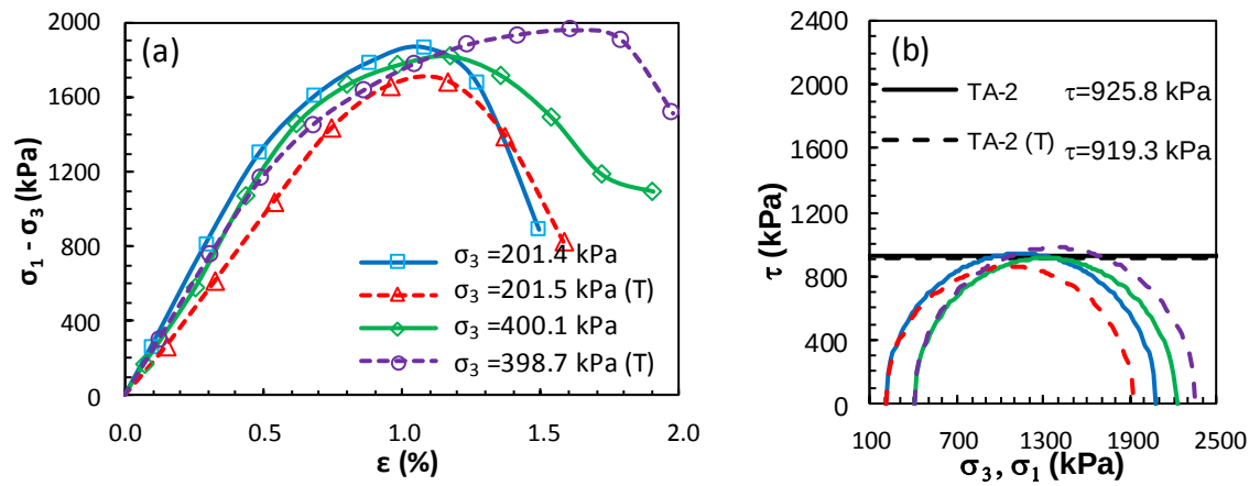
Şekil Ek 6.18. KÖ-2 numaralı tasarım: a) deviator gerilme-birim deformasyon grafikleri ve b) Mohr daireleri (Küçük ölçekli DKK, UU, 28 gün)
