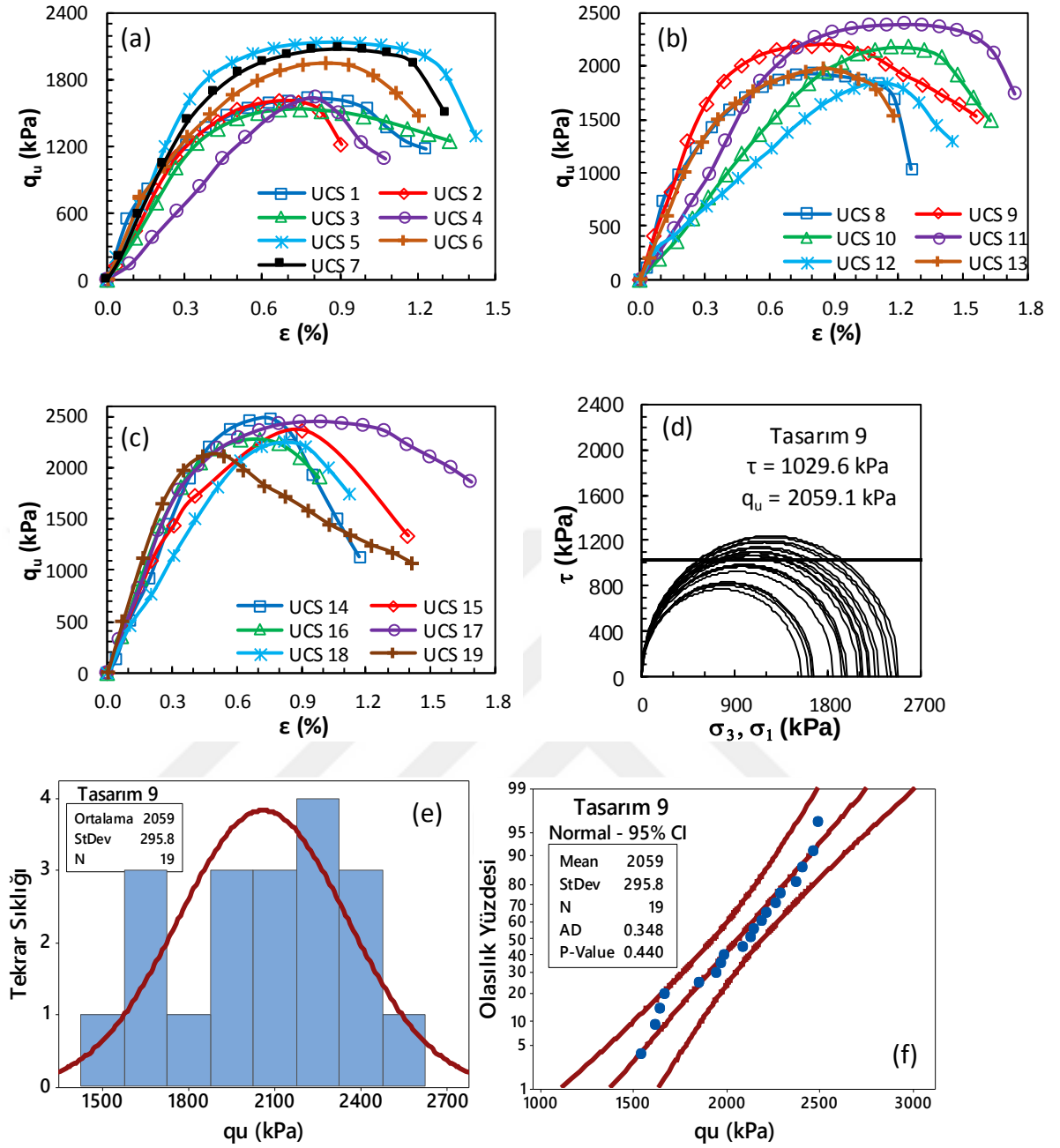
Şekil Ek 1.9. SP-9 numaralı kolona ait gerilme-birim deformasyon grafikleri: a) kolon alt bölgesi, b) kolon orta bölgesi, c) kolon üst bölgesi ve d) Mohr daireleri, e) histogram grafiği, f) olasılık grafiği (Sistem parametreleri, UCS, 28 gün)
