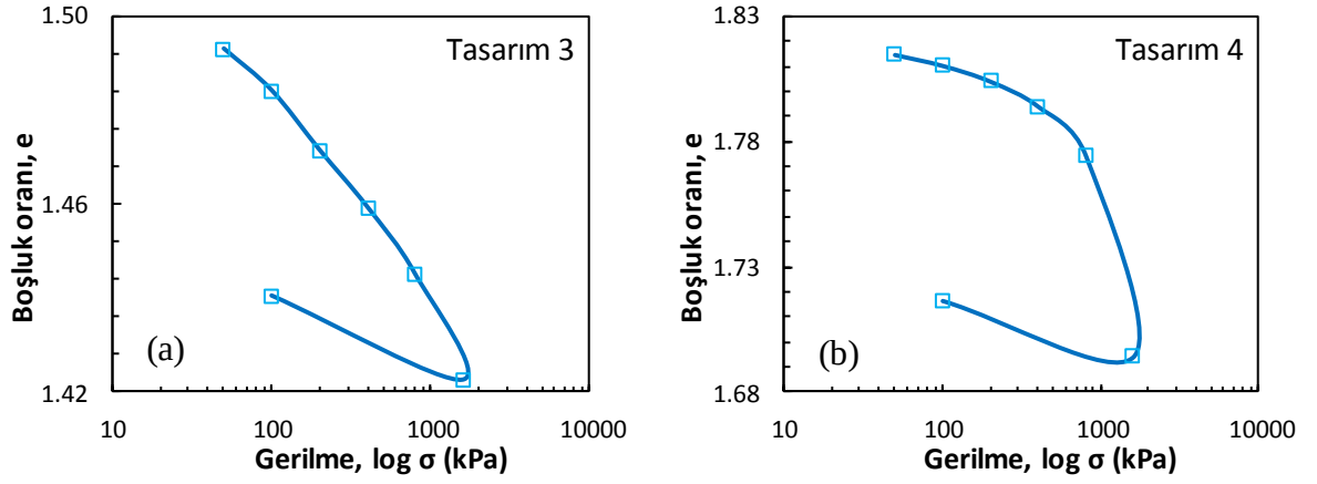
Şekil Ek 7.10. Küçük ölçekli DKK, konsolidasyon deneyi, 56 gün: a) Tasarım 3 ve b) Tasarım 4
