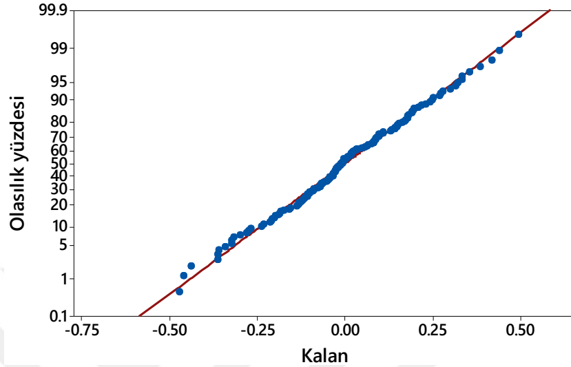
Şekil 4.109. RI sonuçları için geliştirilen modeldeki hataların normal olasılık grafiği (Küçük ölçekli DKK)
