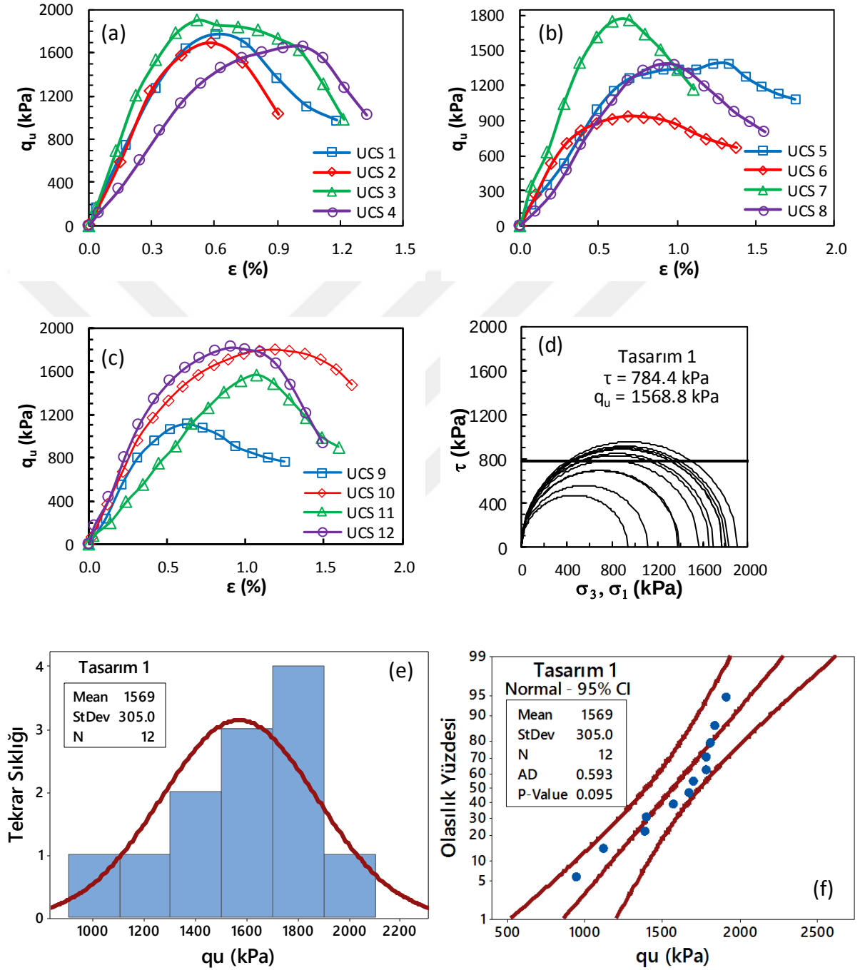
Şekil Ek 1.1. SP-1 numaralı kolona ait gerilme-birim deformasyon grafikleri: a) kolon alt bölgesi, b) kolon orta bölgesi, c) kolon üst bölgesi ve d) Mohr daireleri, e) histogram grafiği, f) olasılık grafiği (Sistem parametreleri, UCS, 28 gün)
