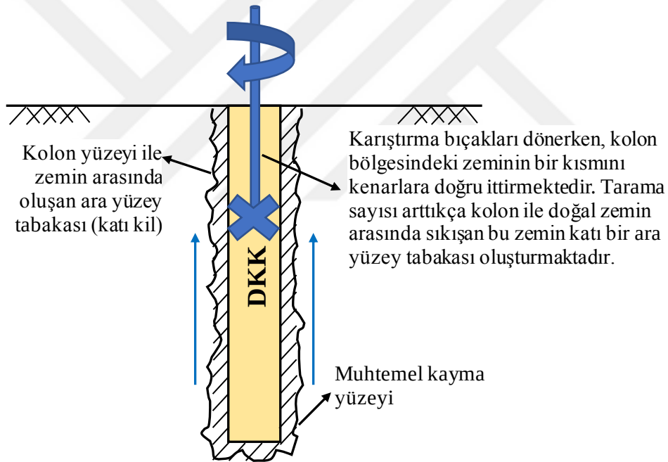
Şekil 4.2. Kolon yüzeyi ile iyileştirilecek zemin arasında oluşan ara yüzey tabakası
