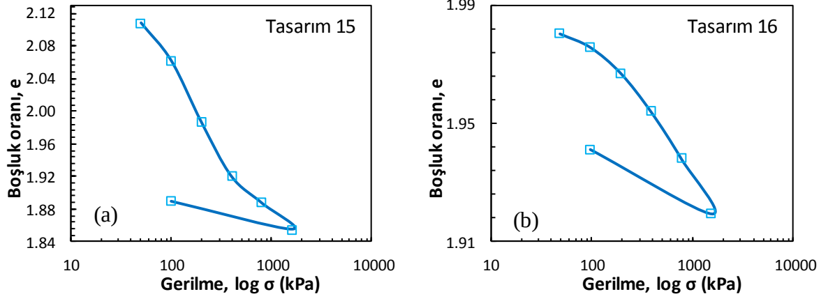
Şekil Ek 7.16. Küçük ölçekli DKK, konsolidasyon deneyi, 56 gün: a) Tasarım 15 ve b) Tasarım 16
