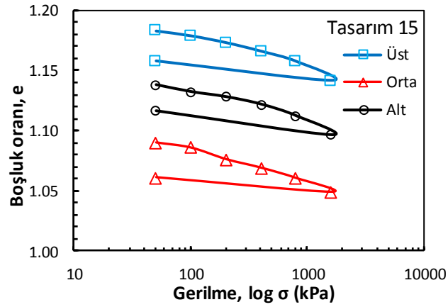
Şekil Ek 4.15. BÖ-15 numaralı kolona ait konsolidasyon deney sonucu (Büyük ölçekli DKK, 28 gün)
