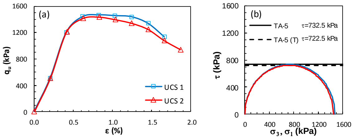
Şekil Ek 5.21. KÖ-5 numaralı tasarım: a) gerilme-birim deformasyon grafikleri ve b) Mohr daireleri (Küçük ölçekli DKK, UCS, 28 gün)
