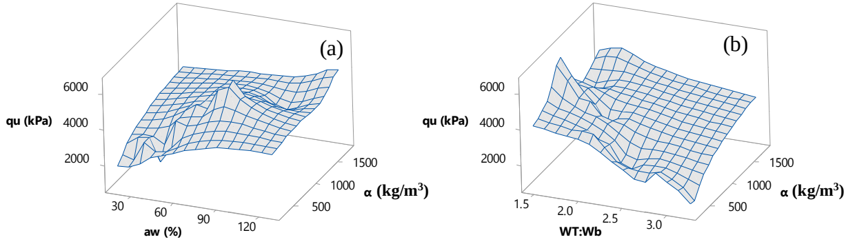
Şekil 4.57. Serbest basınç dayanımının a) a_w - \alpha ve b) W_T:W_b - \alpha arasındaki ilişkiler (Küçük ölçekli DKK, UCS, 56 gün)
