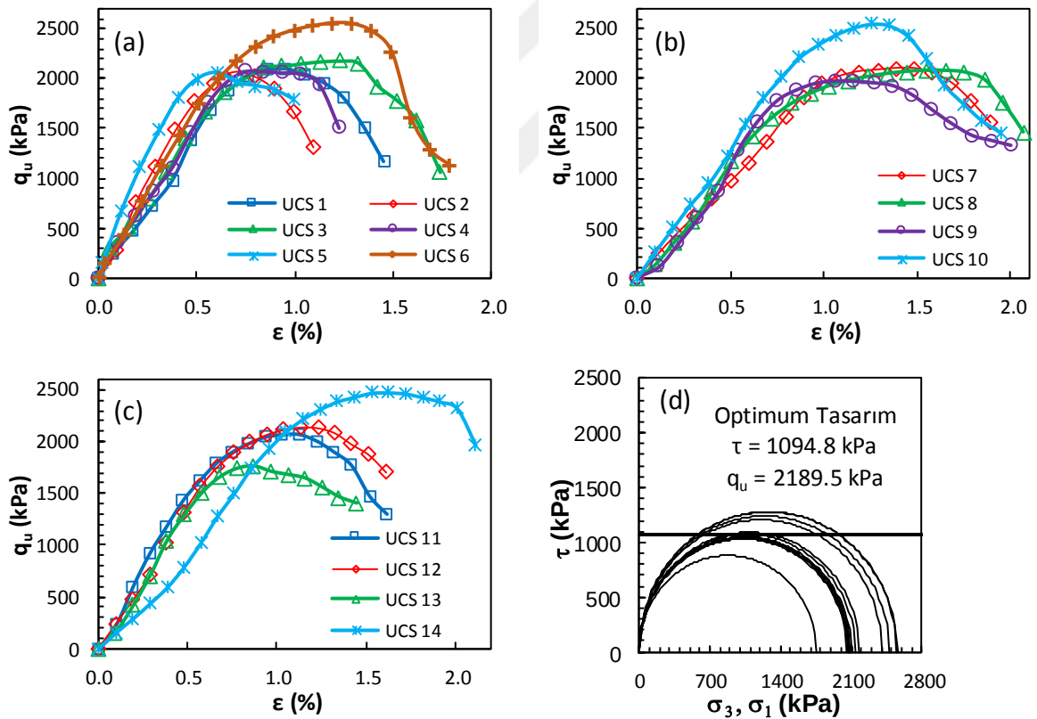
Şekil 4.17. Optimum tasarıma ait gerilme-birim deformasyon grafikleri: a) kolon üst bölgesi, b) kolon orta bölgesi, c) kolon alt bölgesi ve d) mohr daireleri
