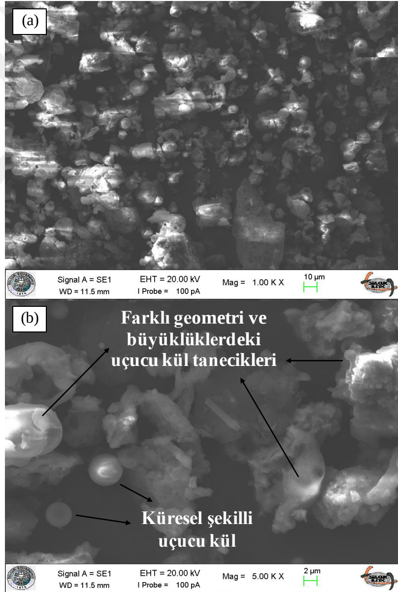
Şekil 4.119. Uçucu küle ait SEM görüntüleri: a) x1000, b) x5000
