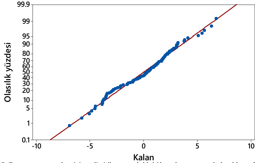
Şekil 4.113. Dayanım sonuçları için geliştirilen modeldeki hataların normal olasılık grafiği (Büyük ölçekli DKK)
