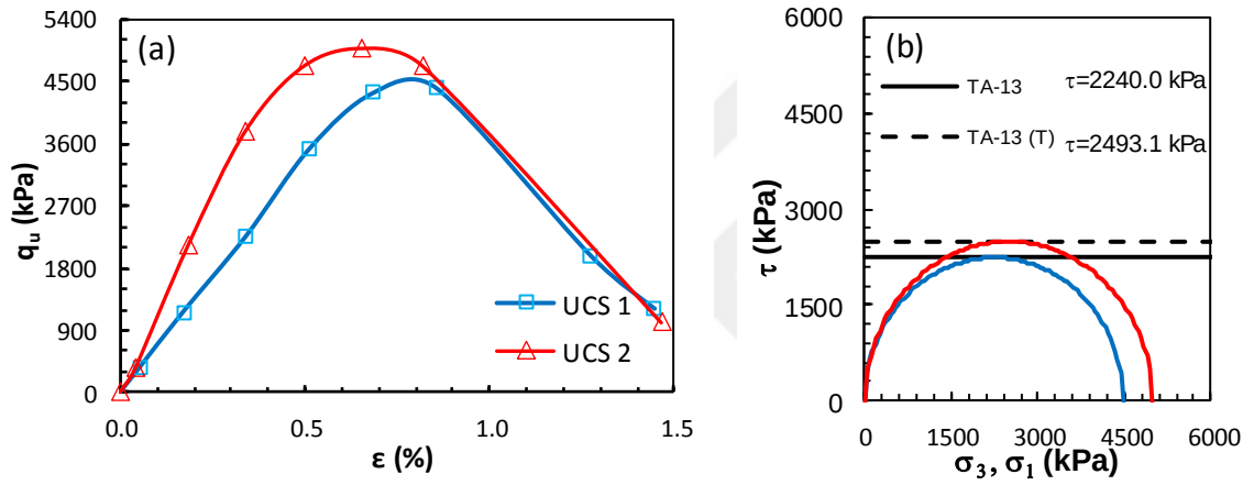
Şekil Ek 5.29. KÖ-13 numaralı tasarım: a) gerilme-birim deformasyon grafikleri ve b) Mohr daireleri (Küçük ölçekli DKK, UCS, 28 gün)
