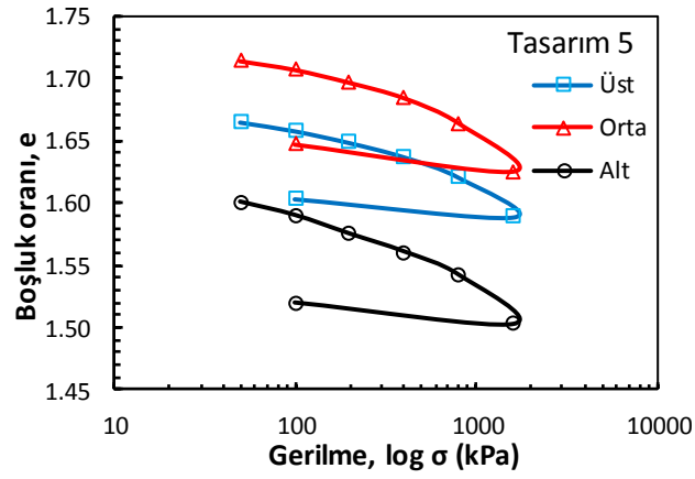
Şekil Ek 4.21. BÖ-5 numaralı kolona ait konsolidasyon deney sonucu (Büyük ölçekli DKK, 56 gün)
