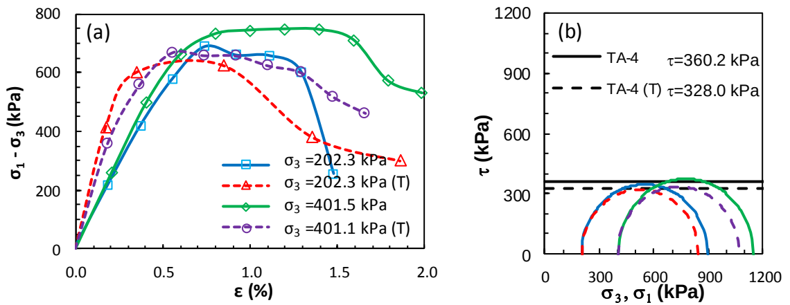
Şekil Ek 6.36. KÖ-4 numaralı tasarım: a) deviator gerilme-birim deformasyon grafikleri ve b) Mohr daireleri (Küçük ölçekli DKK, UU, 56 gün)
