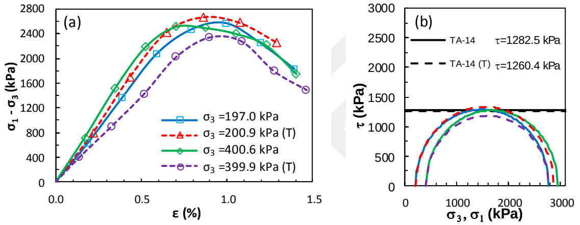
Şekil Ek 6.14. KÖ-14 numaralı tasarım: a) deviator gerilme-birim deformasyon grafikleri ve b) Mohr daireleri (Küçük ölçekli DKK, UU, 7 gün)
