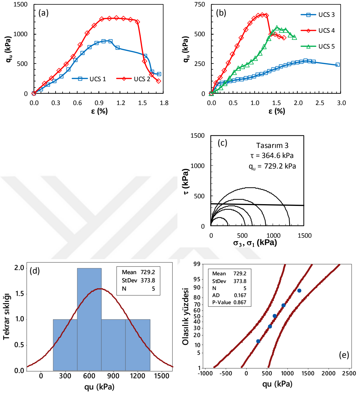
Şekil Ek 2.3. BÖ-3 numaralı kolona ait gerilme-birim deformasyon grafikleri: a) kolon üst bölgesi, b) kolon alt bölgesi ve c) Mohr daireleri, d) histogram grafiği, e) olasılık grafiği (Büyük ölçekli DKK, UCS, 28 gün)
