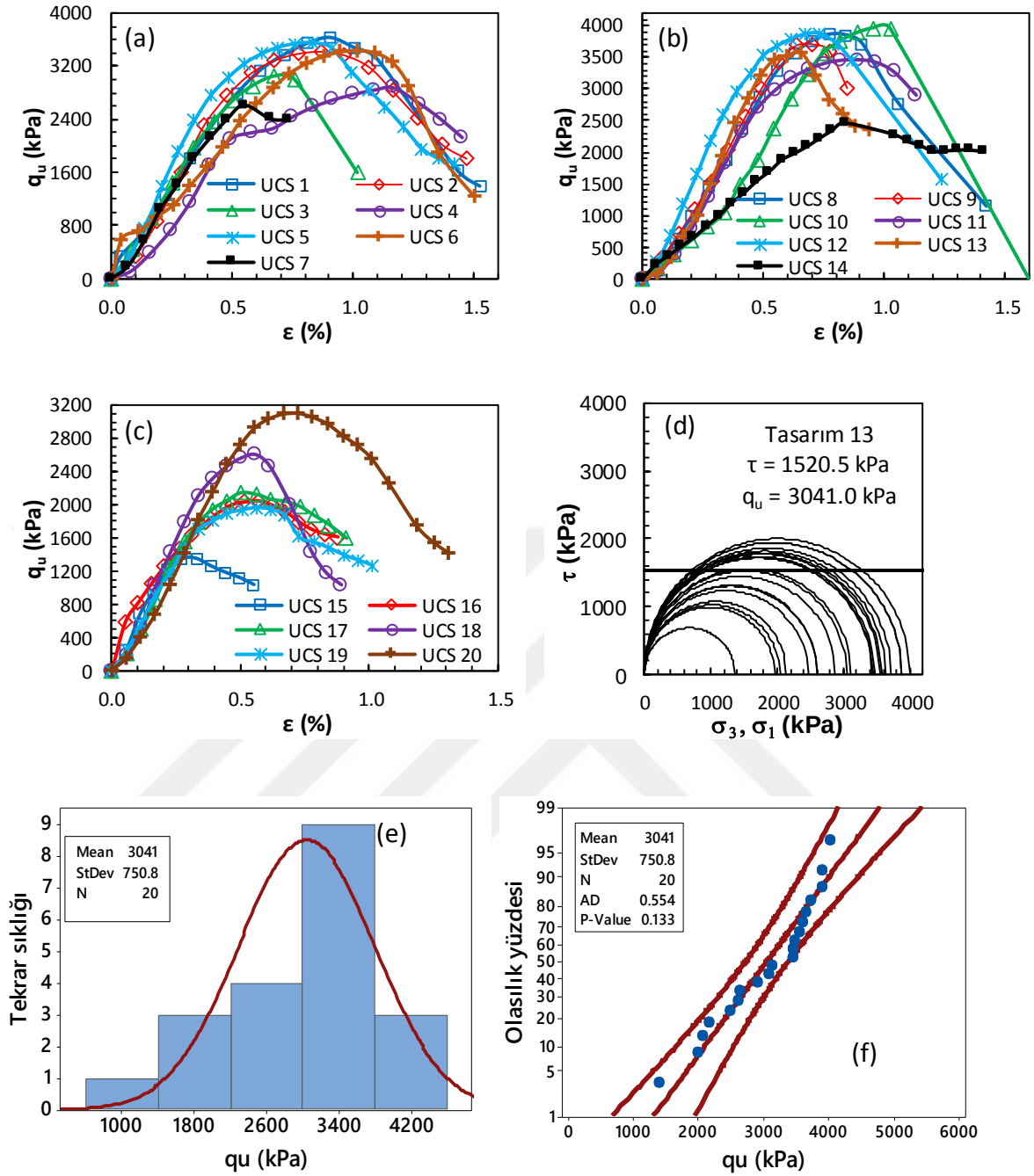
Şekil Ek 2.29. BÖ-13 numaralı kolona ait gerilme-birim deformasyon grafikleri: a) kolon üst bölgesi, b) kolon orta bölgesi, c) kolon alt bölgesi ve d) Mohr daireleri, e) histogram grafiği, f) olasılık grafiği (Büyük ölçekli DKK, UCS, 56 gün)
