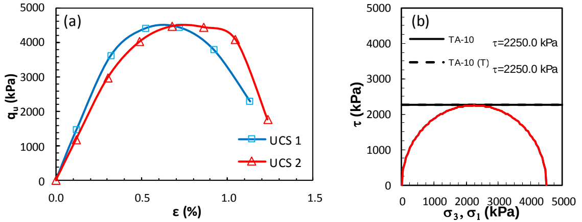
Şekil Ek 5.42. KÖ-10 numaralı tasarım: a) gerilme-birim deformasyon grafikleri ve b) Mohr daireleri (Küçük ölçekli DKK, UCS, 56 gün)
