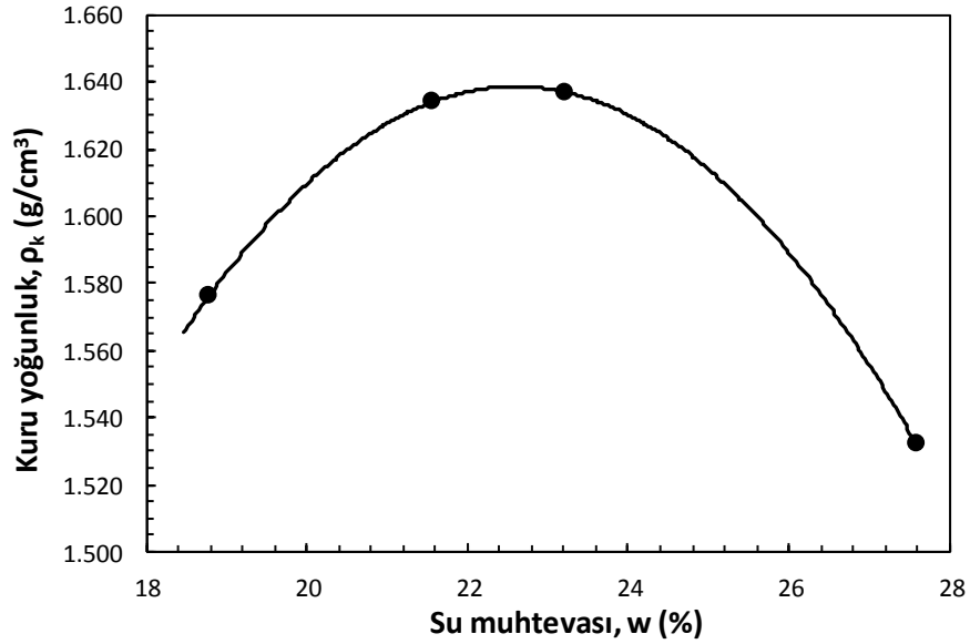
Şekil 3.8. Kompaksiyon deneyinden elde edilen su muhtevası-kuru yoğunluk grafiği
