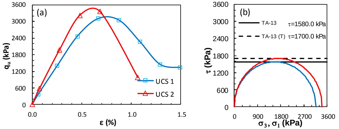
Şekil Ek 5.13. KÖ-13 numaralı tasarım: a) gerilme-birim deformasyon grafikleri ve b) Mohr daireleri (Küçük ölçekli DKK, UCS, 7 gün)
