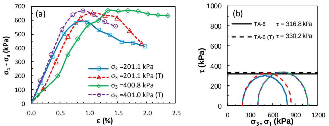
Şekil Ek 6.6. KÖ-6 numaralı tasarım: a) deviyör gerilme-birim deformasyon grafikleri ve b) Mohr daireleri (Küçük ölçekli DKK, UU, 7 gün)
