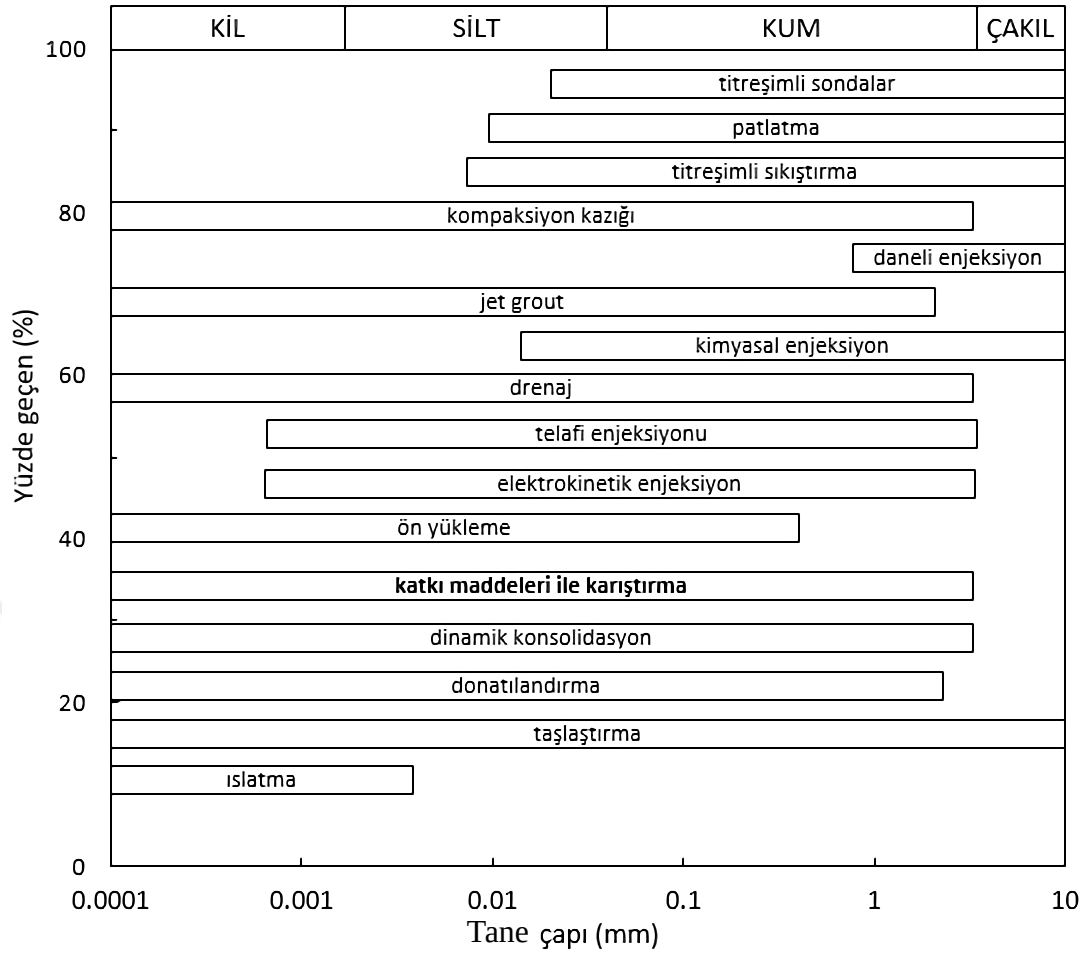
Şekil 2.2. Zemin iyileştirme yöntemlerinin tane boyutuna göre ayrımı (Mitchell, 1981)
