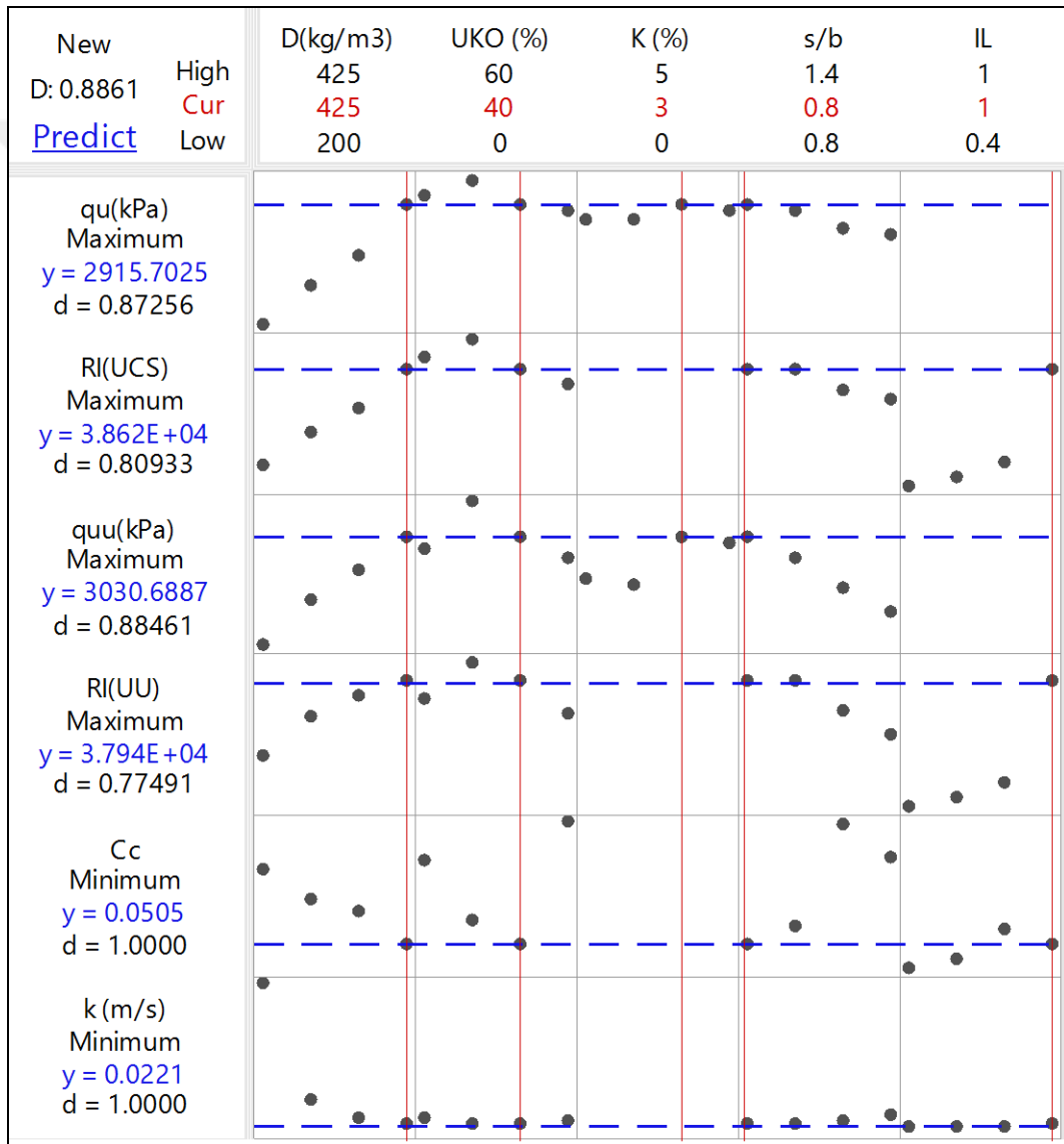
Şekil 4.79. UKO=%40 için 28 günlük performans değerlerinin tahmini için optimizasyon grafiği Not: k değeri 10^{-9} ile çarpılmalıdır.
