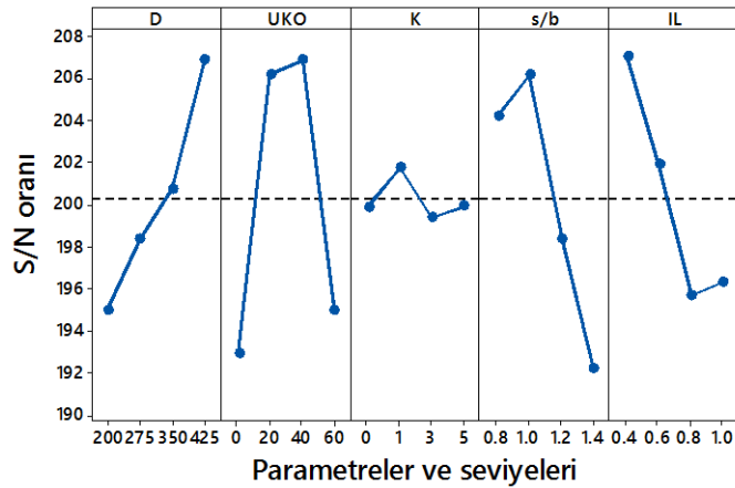
Şekil 4.73. Permeabilite katsayısı (k) için elde edilen S/N grafiği (Küçük ölçekli DKK, 56 gün)
