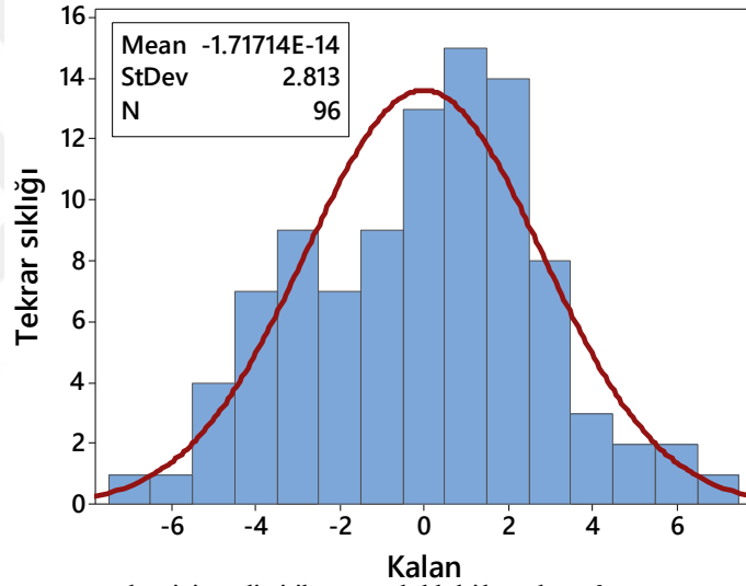
Şekil 4.114. Dayanım sonuçları için geliştirilen modeldeki hataların histogram grafiği (Büyük ölçekli DKK)
