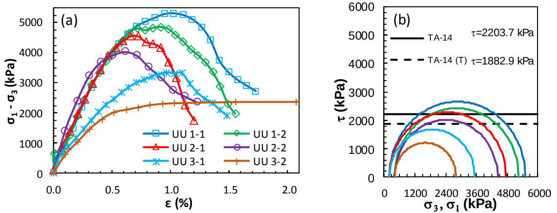
Şekil Ek 3.30. BÖ-14 numaralı kolona ait UU deney sonuçları: a) deviator gerilme-birim boy kısalması grafikleri, b) Mohr daireleri ile kırılma zarfları (büyük ölçekli DKK, 56 gün)
