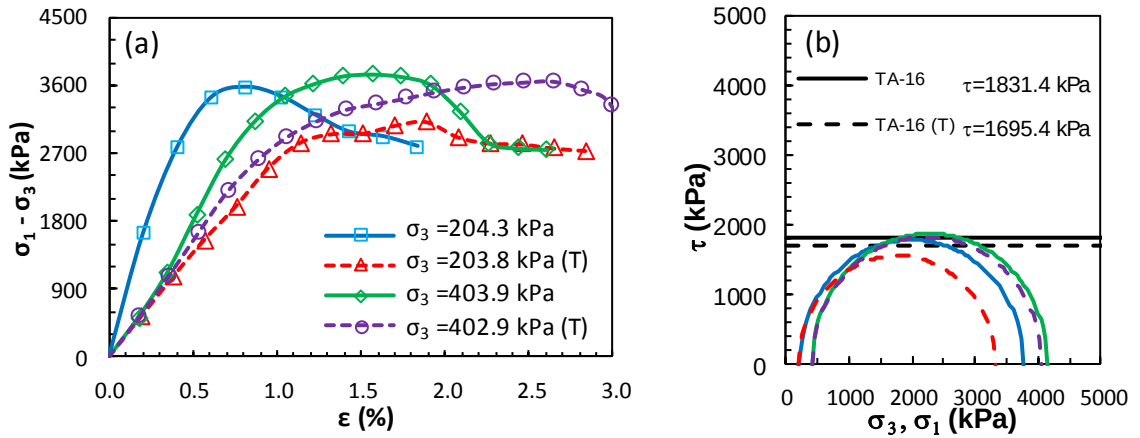
Şekil Ek 6.48. KÖ-16 numaralı tasarım: a) deviator gerilme-birim deformasyon grafikleri ve b) Mohr daireleri (Küçük ölçekli DKK, UU, 56 gün)
