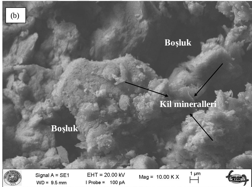
Şekil 4.117. Yüksek plastisiteli kile ait SEM görüntüleri: a) x5000, b) x10000
