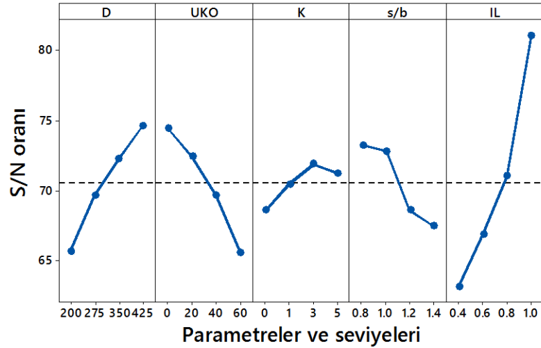
Şekil 4.50. Zemin iyileştirme derecesi için elde edilen S/N grafiği (Küçük ölçekli DKK, UCS, 7 gün)
