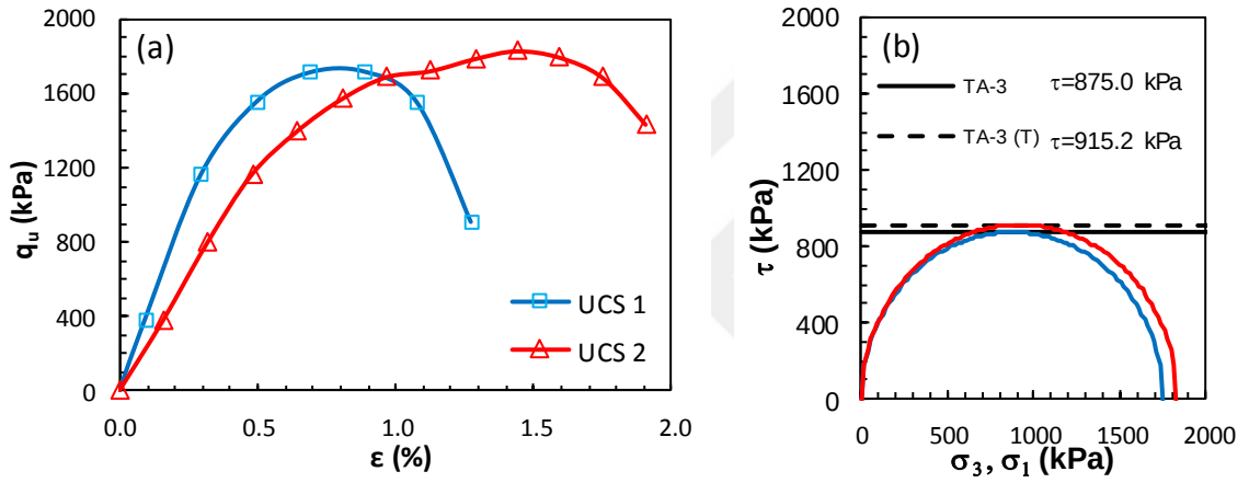
Şekil Ek 5.35. KÖ-3 numaralı tasarım: a) gerilme-birim deformasyon grafikleri ve b) Mohr daireleri (Küçük ölçekli DKK, UCS, 56 gün)
