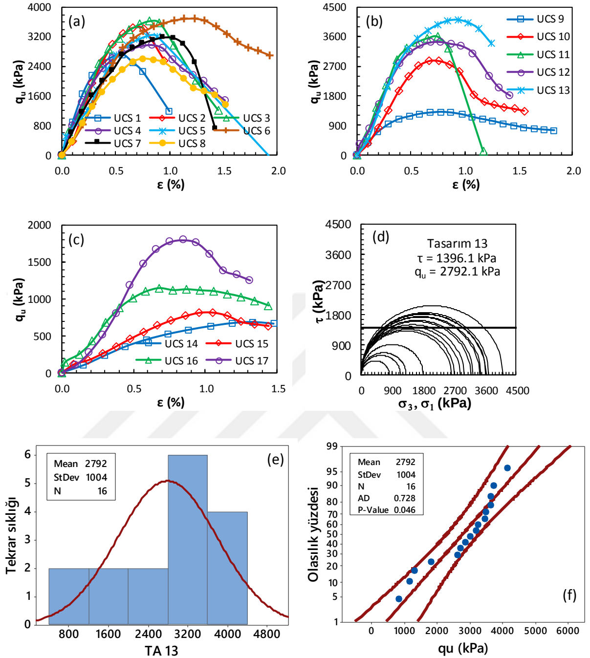
Şekil Ek 2.13. BÖ-13 numaralı kolona ait gerilme-birim deformasyon grafikleri: a) kolon üst bölgesi, b) kolon orta bölgesi, c) kolon alt bölgesi ve d) Mohr daireleri, e) histogram grafiği, f) olasılık grafiği (Büyük ölçekli DKK, UCS, 28 gün)
