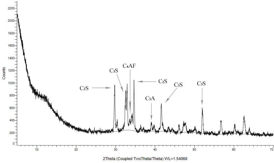
Şekil 4.122. CEM 1 42.5 R çimentosunun XRD analizi sonucu
