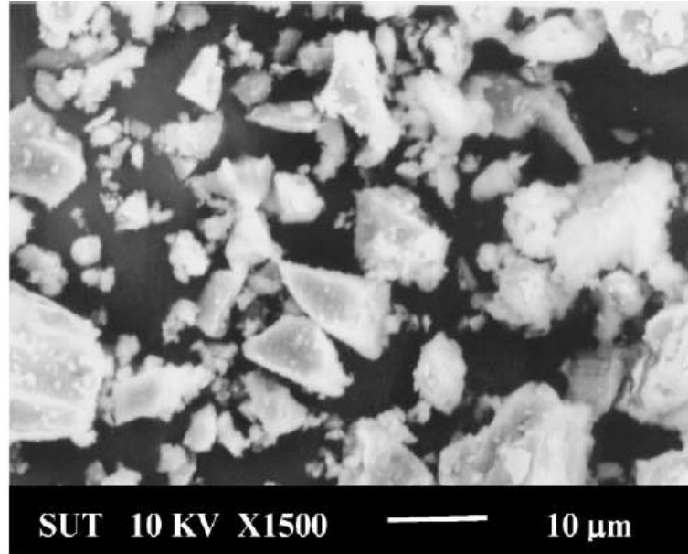
Şekil 4.121. CEM 1 42.5 R çimentosunun SEM görüntüsü
