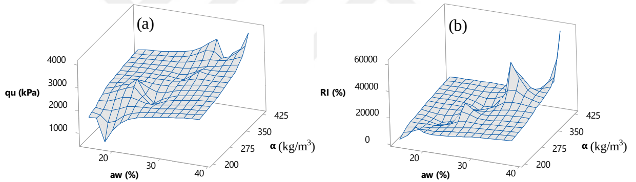
Şekil 4.25. a_w ve \alpha ile a) q_u ve b) RI arasındaki ilişki (Büyük ölçekli DKK, UCS, 56 gün)
