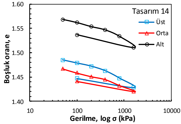
Şekil Ek 4.30. BÖ-14 numaralı kolona ait konsolidasyon deney sonucu (Büyük ölçekli DKK, 56 gün)
