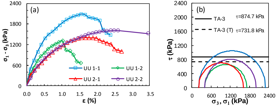
Şekil Ek 3.19. BÖ-3 numaralı kolona ait UU deney sonuçları: a) deviatör gerilme-birim boy kısalması grafikleri, b) Mohr daireleri ile kırılma zarfları (Büyük ölçekli DKK, UU, 56 gün)
