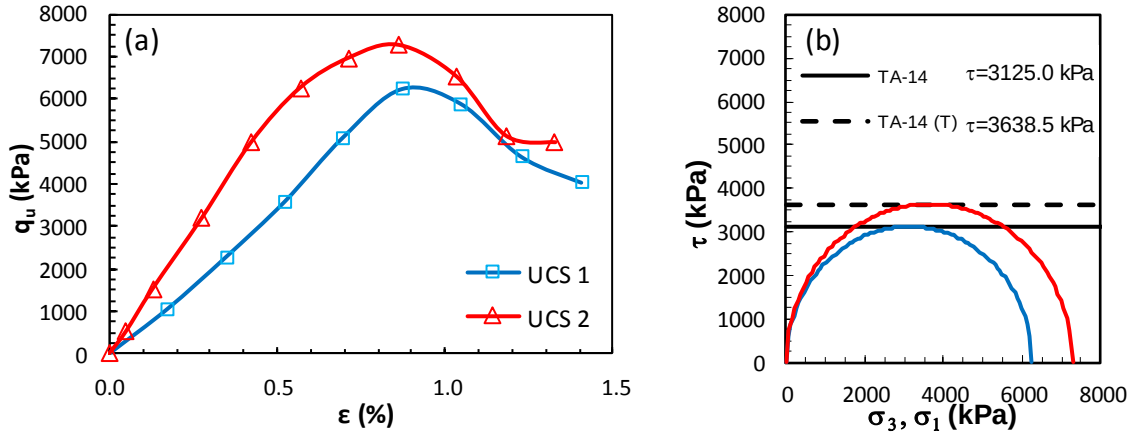
Şekil Ek 5.46. KÖ-14 numaralı tasarım: a) gerilme-birim deformasyon grafikleri ve b) Mohr daireleri (Küçük ölçekli DKK, UCS, 56 gün)
