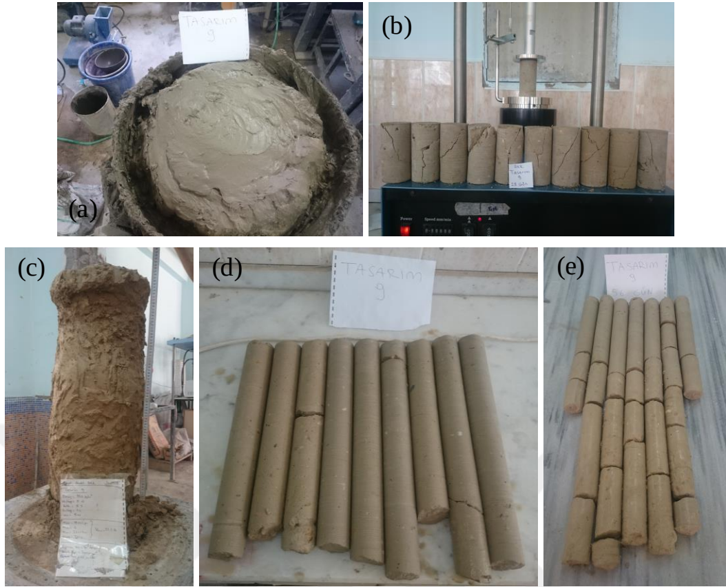
Şekil 3.60. Büyük ölçekli DKK, Tasarım 9: a) imalat sonrası görünüm, b) kayma yüzeyleri, c) imal edilen kolon, d) 28 ve e) 56 günlük karot numuneleri (büyük ölçekli DKK)
