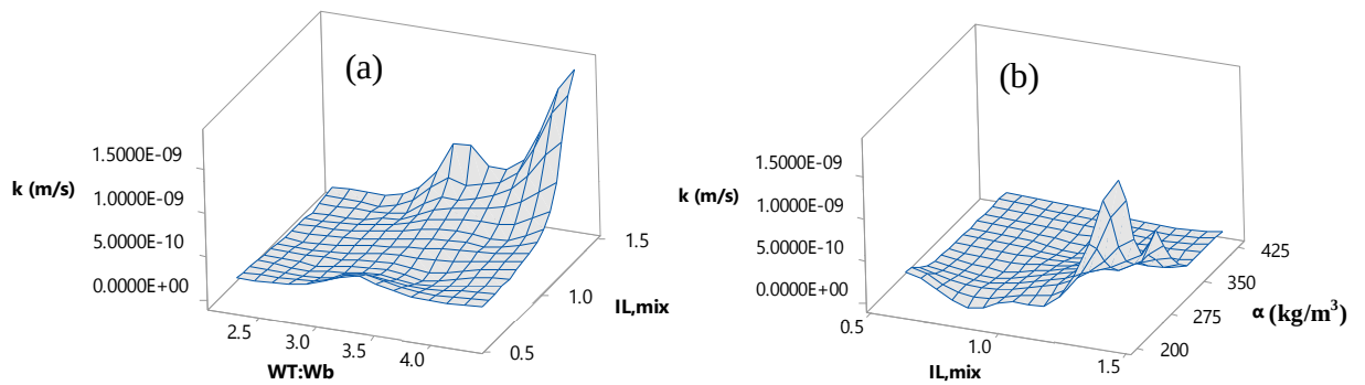
Şekil 4.47. Permeabilite katsayısının a) W_T:W_b - I_{L,mix} ve b) I_{L,mix} - \alpha ile olan ilişkileri
