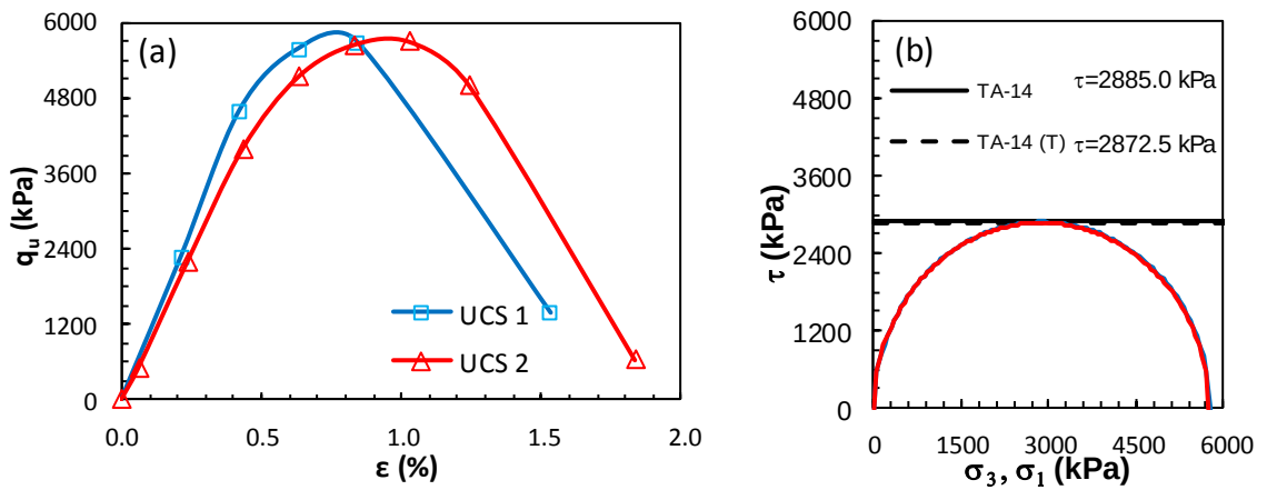
Şekil Ek 5.30. KÖ-14 numaralı tasarım: a) gerilme-birim deformasyon grafikleri ve b) Mohr daireleri (Küçük ölçekli DKK, UCS, 28 gün)
