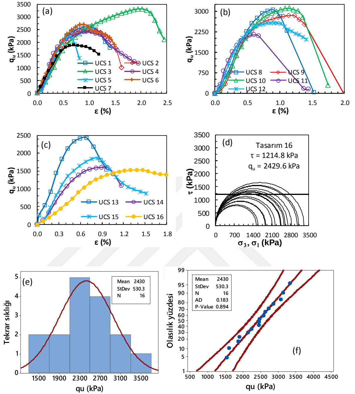
Şekil Ek 2.32. BÖ-16 numaralı kolona ait gerilme-birim deformasyon grafikleri: a) kolon üst bölgesi, b) kolon orta bölgesi, c) kolon alt bölgesi ve d) Mohr daireleri, e) histogram grafiği, f) olasılık grafiği (Büyük ölçekli DKK, UCS, 56 gün)
