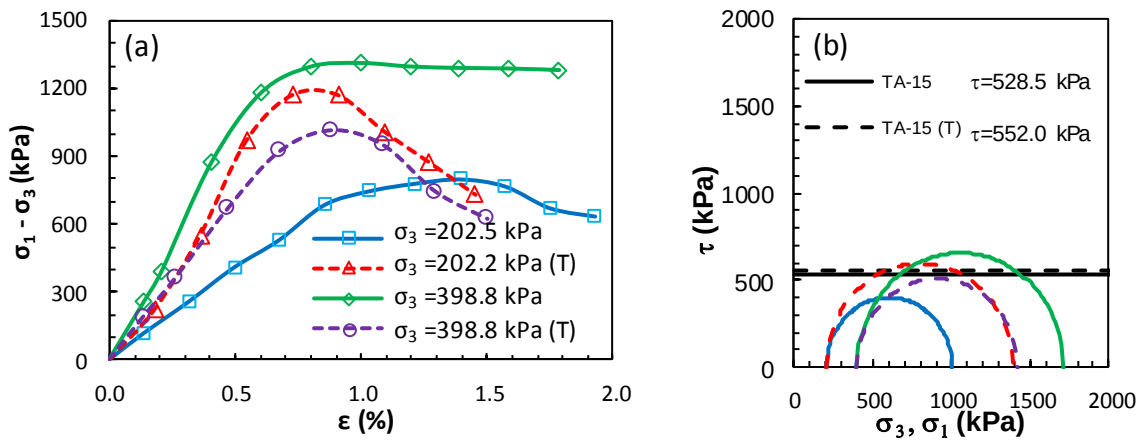
Şekil Ek 6.15. KÖ-15 numaralı tasarım: a) deviator gerilme-birim deformasyon grafikleri ve b) Mohr daireleri (Küçük ölçekli DKK, UU, 7 gün)
