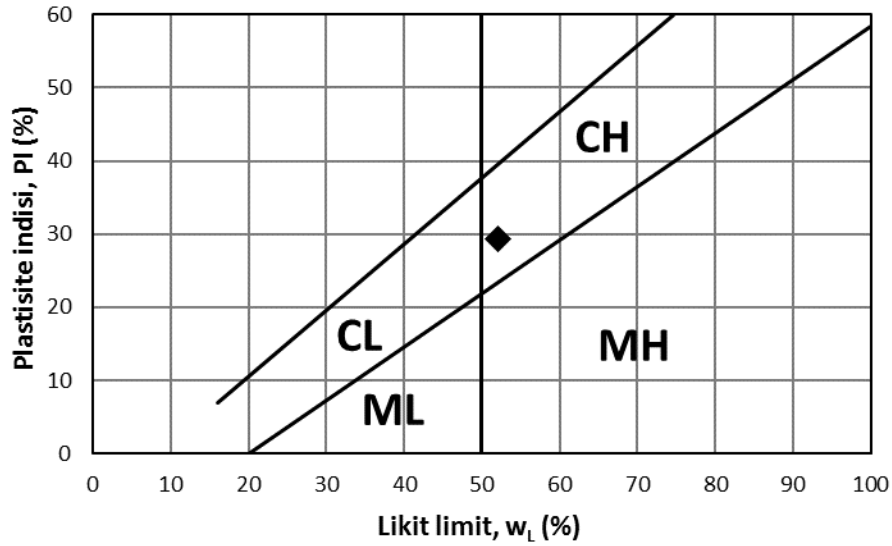
Şekil 3.7. USCS'ye göre zemin sınıfının belirlenmesi
