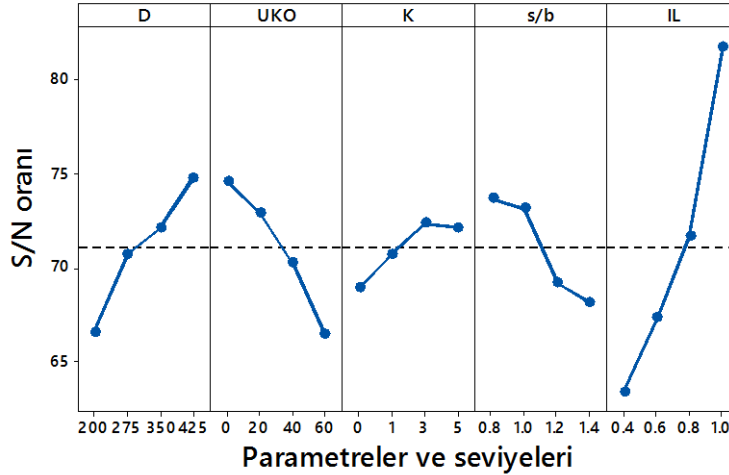
Şekil 4.59. Zemin iyileştirme derecesi için elde edilen S/N grafiği (Küçük ölçekli DKK, UU, 7 gün)
