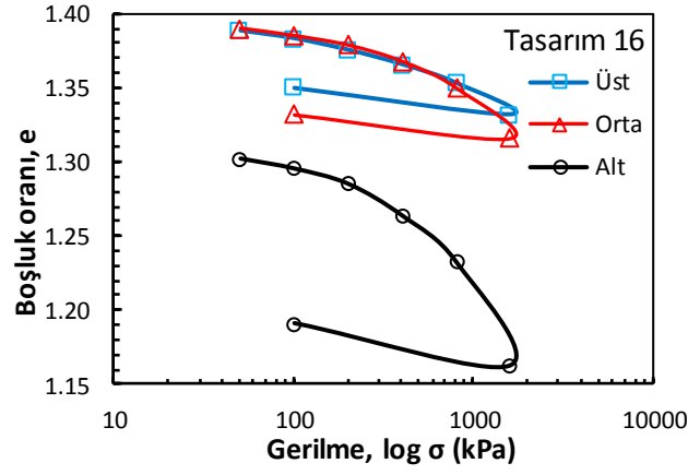
Şekil Ek 4.16. BÖ-16 numaralı kolona ait konsolidasyon deney sonucu (Büyük ölçekli DKK, 28 gün)
