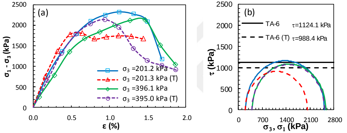
Şekil Ek 6.38. KÖ-6 numaralı tasarım: a) deviator gerilme-birim deformasyon grafikleri ve b) Mohr daireleri (Küçük ölçekli DKK, UU, 56 gün)
