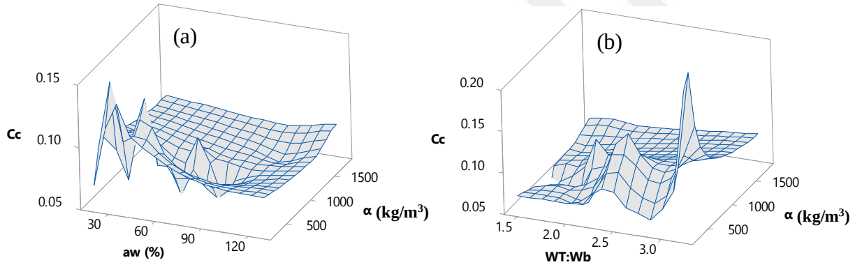
Şekil 4.71. Sıkışma indisinin a) a_w - \alpha ve b) WT:Wb - \alpha arasındaki ilişkiler (Küçük ölçekli DKK, 56 gün)
