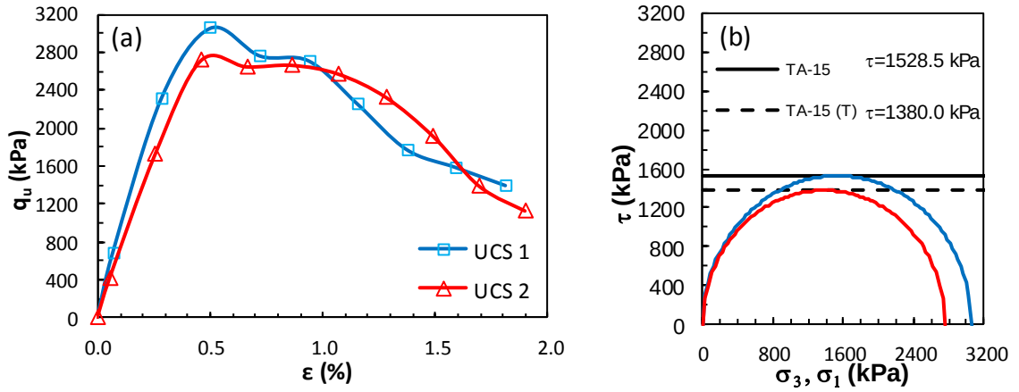
Şekil Ek 5.31. KÖ-15 numaralı tasarım: a) gerilme-birim deformasyon grafikleri ve b) Mohr daireleri (Küçük ölçekli DKK, UCS, 28 gün)
