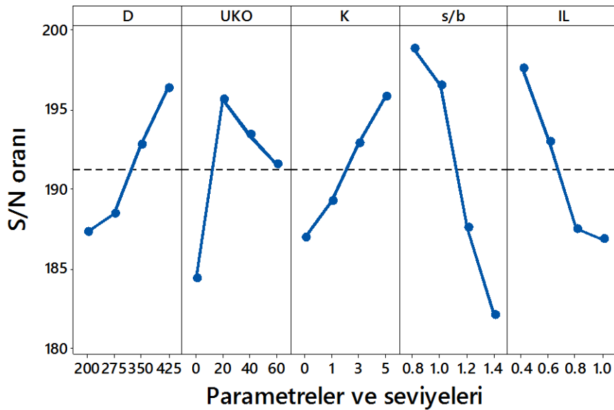
Şekil 4.72. Permeabilite katsayısı (k) için elde edilen S/N grafiği (Küçük ölçekli DKK, 28 gün)
