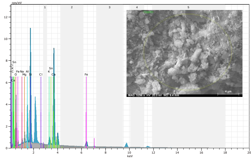
Şekil 4.134. Optimum tasarıma ait EDX sonucu (Küçük ölçekli DKK, 56 gün)
