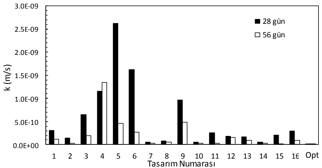
Şekil 4.74. Permeabilite deney sonuçları (Küçük ölçekli DKK)
