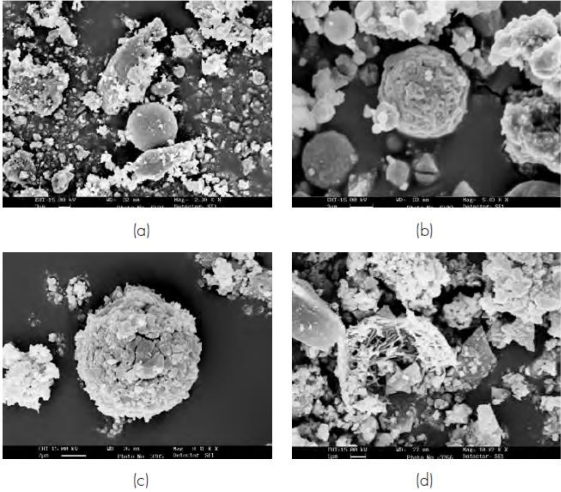
Şekil 3.15. Seyitömer uçucu külünün mikroyapısı: (a) Magnezyoferrit küresi (x8100), (b) Demir oksit kaplı tanecik (x5000), (c) Alkali feldispatlar (x2500), (d) Mullit kristalleri (x10000) (Türker ve ark., 2009)
