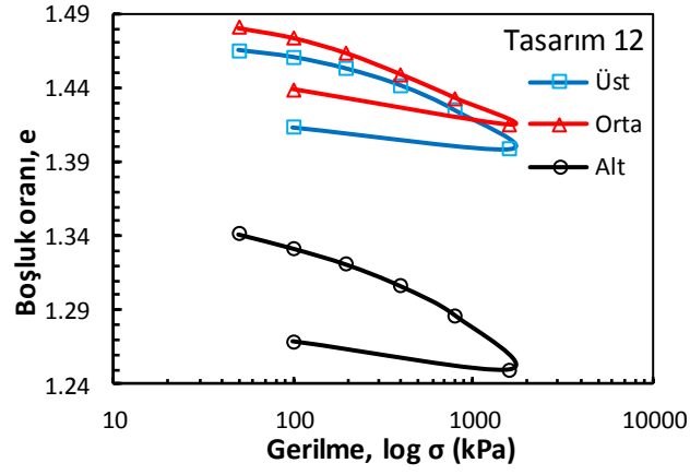
Şekil Ek 4.28. BÖ-12 numaralı kolona ait konsolidasyon deney sonucu (Büyük ölçekli DKK, 56 gün)
