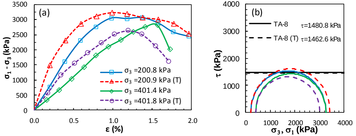
Şekil Ek 6.40. KÖ-8 numaralı tasarım: a) deviator gerilme-birim deformasyon grafikleri ve b) Mohr daireleri (Küçük ölçekli DKK, UU, 56 gün)
