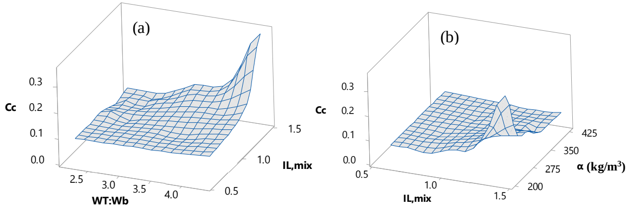
Şekil 4.42. Sıkışma indisinin a) W_T:W_b-IL_{mix} ve b) IL_{mix}-\alpha ile olan ilişkileri (Büyük ölçekli DKK, 56 gün)
