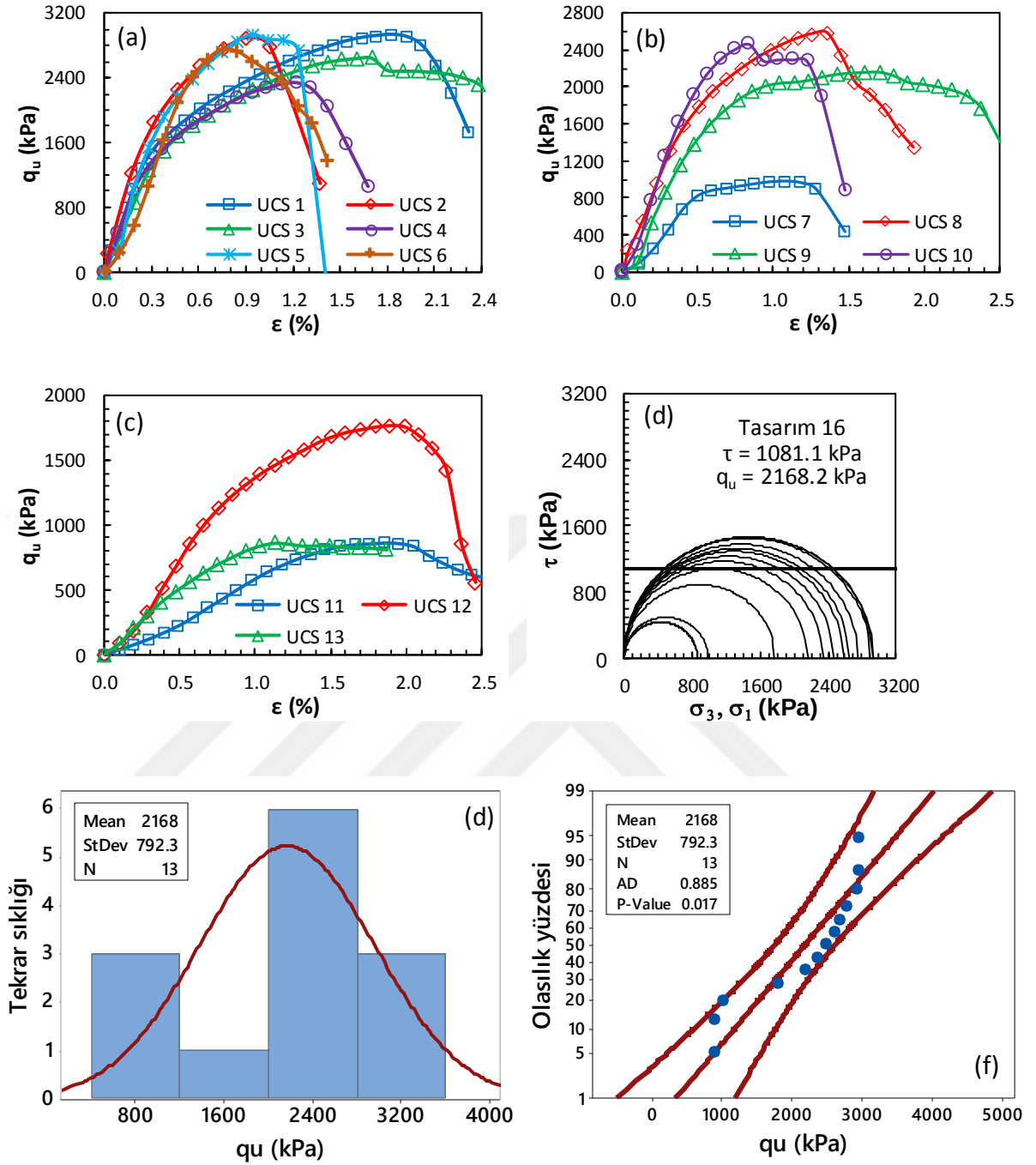
Şekil Ek 2.16. BÖ-16 numaralı kolona ait gerilme-birim deformasyon grafikleri: a) kolon üst bölgesi, b) kolon orta bölgesi, c) kolon alt bölgesi ve d) Mohr daireleri, e) histogram grafiği, f) olasılık grafiği (Büyük ölçekli DKK, UCS, 28 gün)
