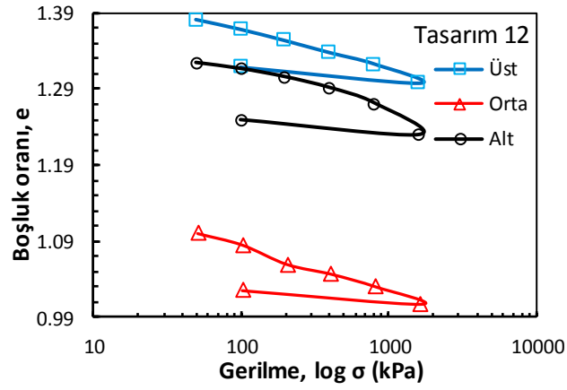
Şekil Ek 4.12. BÖ-12 numaralı kolona ait konsolidasyon deney sonucu (Büyük ölçekli DKK, 28 gün)
