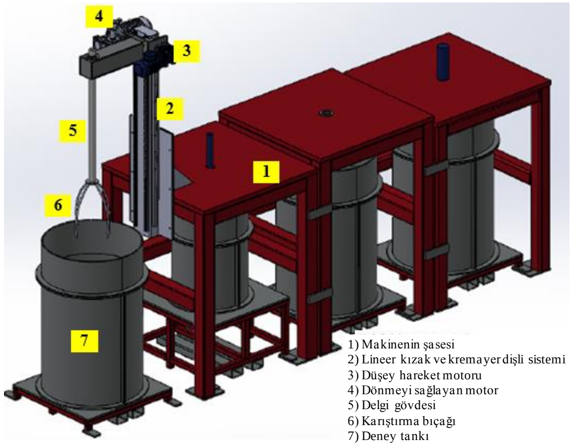
Şekil 3.16. Laboratuvar tipi derin karıştırma makinesinin teknik çizimi
