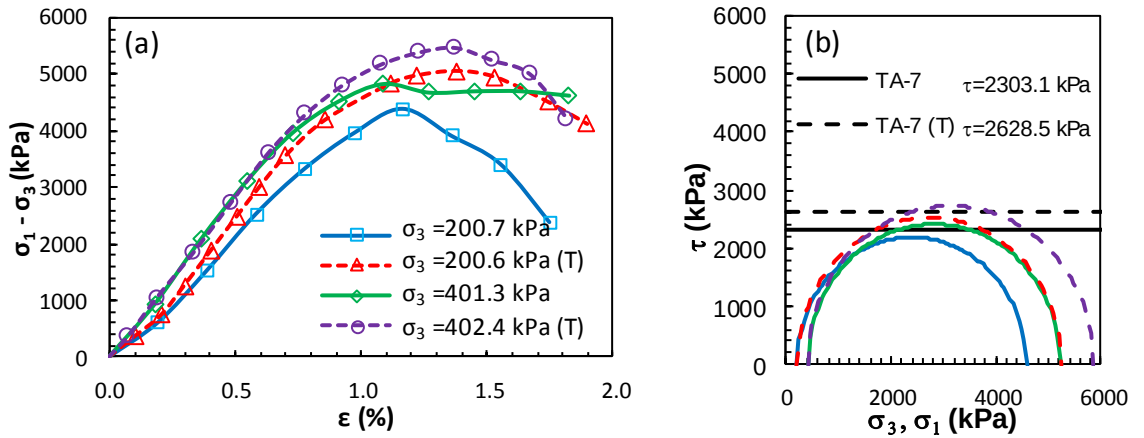
Şekil Ek 6.39. KÖ-7 numaralı tasarım: a) deviator gerilme-birim deformasyon grafikleri ve b) Mohr daireleri (Küçük ölçekli DKK, UU, 56 gün)
