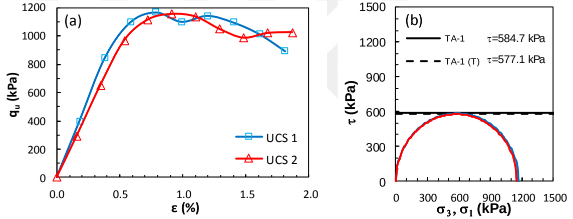
Şekil Ek 5.17. KÖ-1 numaralı tasarım: a) gerilme-birim deformasyon grafikleri ve b) Mohr daireleri (Küçük ölçekli DKK, UCS, 28 gün)
