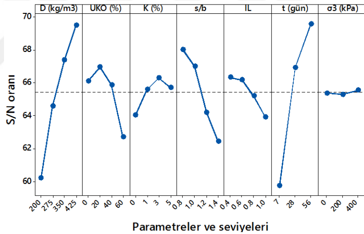
Şekil 4.105. \sigma_1 - \sigma_3 için elde edilen S/N grafiği (Küçük ölçekli DKK)
