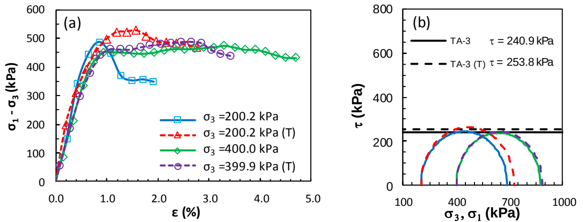
Şekil Ek 6.3. KÖ-3 numaralı tasarım: a) deviator gerilme-birim deformasyon grafikleri ve b) Mohr daireleri (Küçük ölçekli DKK, UU, 7 gün)
