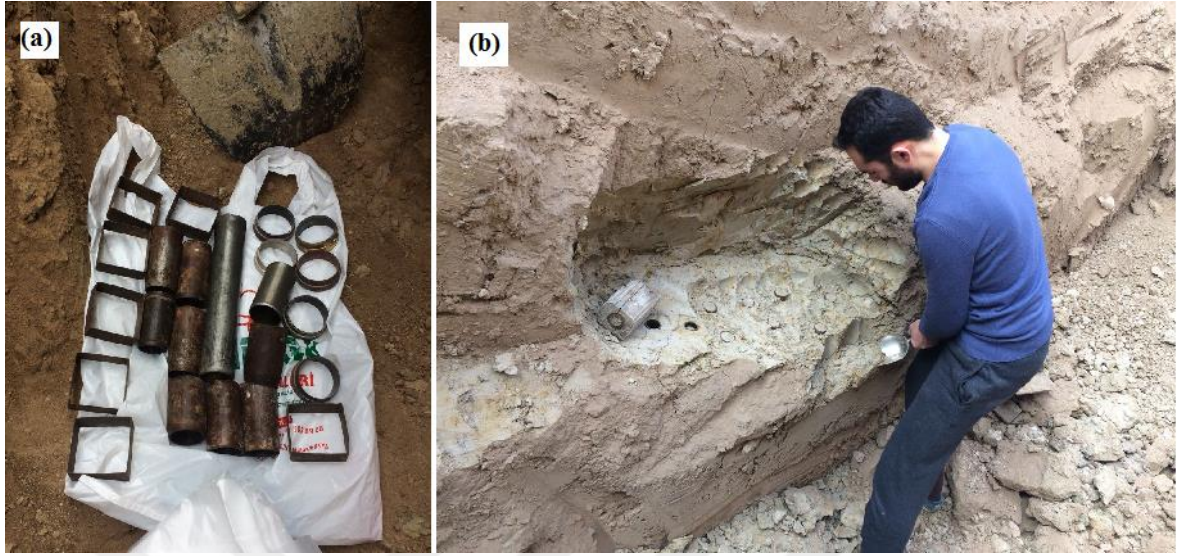
Şekil 3.9. a) Örselenmemiş zemin örneklerinin alınabilmesi için kullanılan kalıplar, b) kazı çukurunda kalıpların zemine çakılması ve numune alınması
