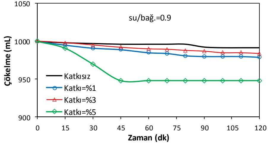
Şekil 3.48. Optima 100 katkısı ile yapılan sedimentasyon deneyi sonuçları (UKO=%60, su/bağlayıcı=0.9)
