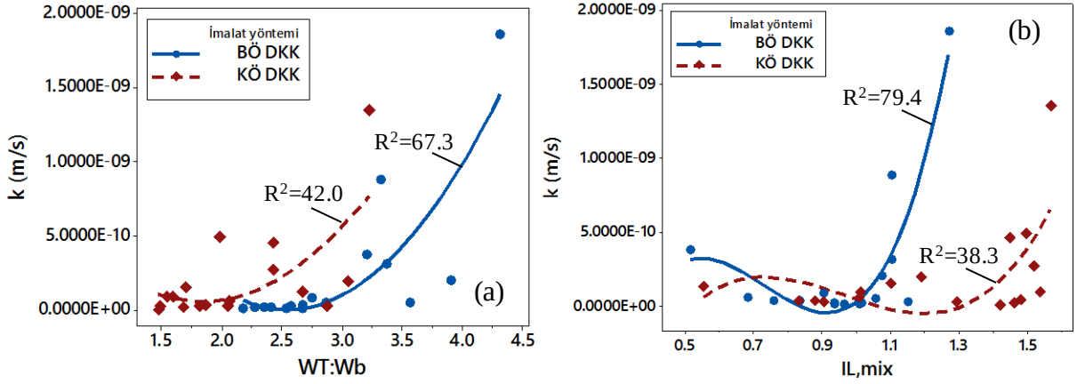
Şekil 4.103. Permeabilite katsayısının a) W_T:W_b ve b) IL_{mix} ile ilişkileri (Küçük ve büyük ölçekli DKK, 56 gün)
