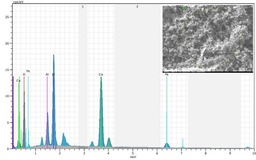
Şekil 4.129. Tasarım 4'e ait EDX analizi sonucu (Küçük ölçekli DKK, 28 gün)
