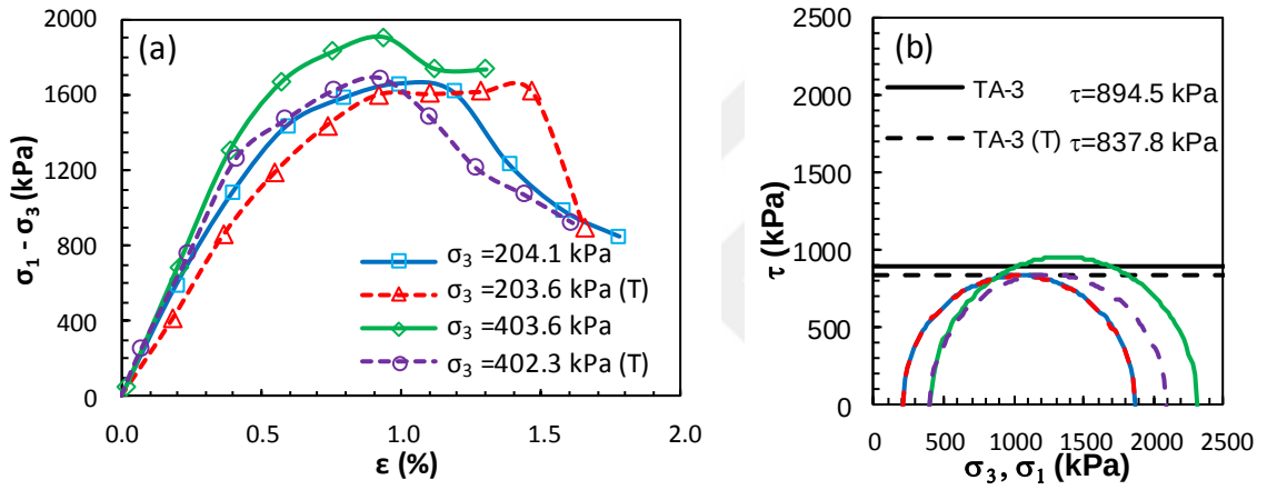
Şekil Ek 6.35. KÖ-3 numaralı tasarım: a) deviator gerilme-birim deformasyon grafikleri ve b) Mohr daireleri (Küçük ölçekli DKK, UU, 56 gün)
