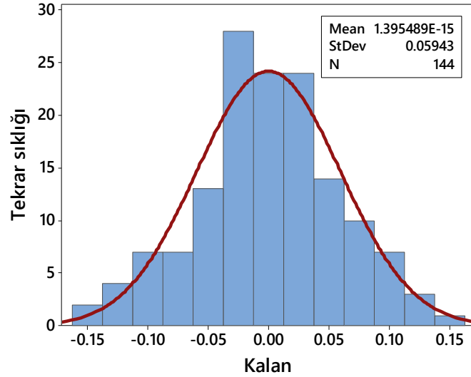
Şekil 4.108. Dayanım sonuçları için geliştirilen modeldeki hataların histogram grafiği (Küçük ölçekli DKK)
