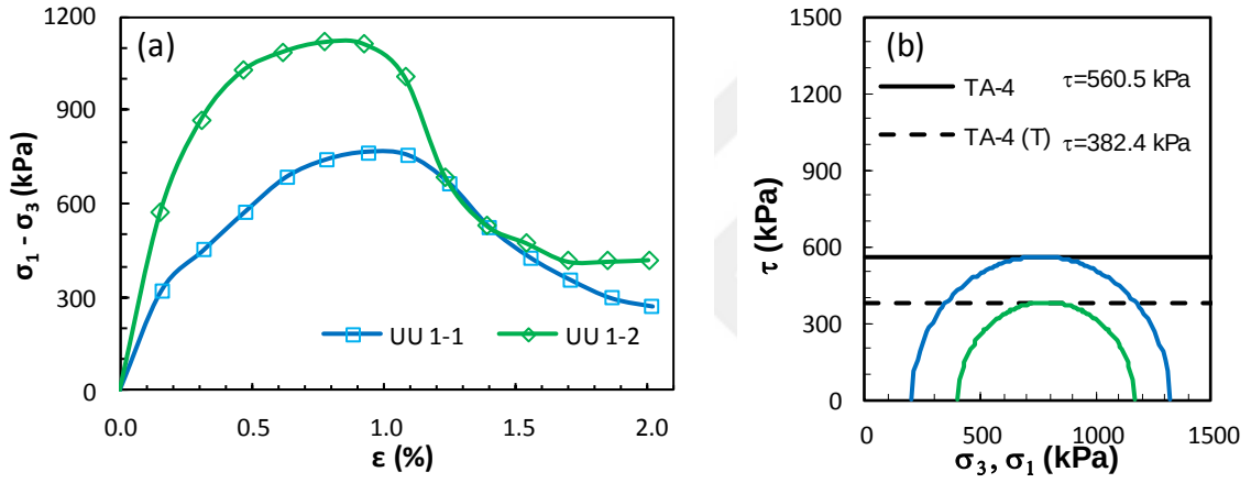
Şekil Ek 3.20. BÖ-4 numaralı kolona ait UU deney sonuçları: a) deviatör gerilme-birim boy kısalması grafikleri, b) Mohr daireleri ile kırılma zarfları (Büyük ölçekli DKK, UU, 56 gün)
