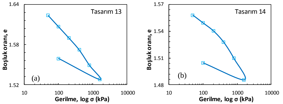
Şekil Ek 7.15. Küçük ölçekli DKK, konsolidasyon deneyi, 56 gün: a) Tasarım 13 ve b) Tasarım 14
