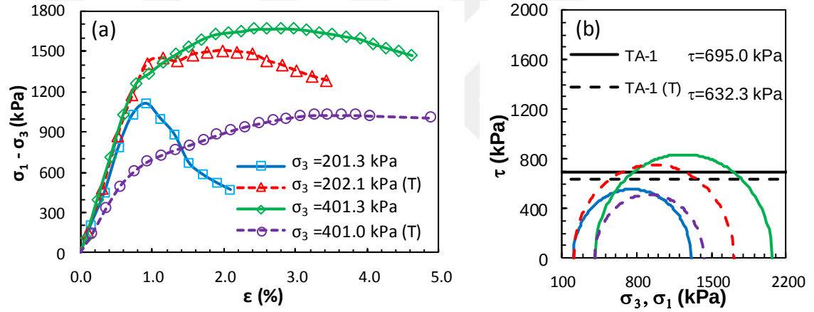
Şekil Ek 6.17. KÖ-1 numaralı tasarım: a) deviator gerilme-birim deformasyon grafikleri ve b) Mohr daireleri (Küçük ölçekli DKK, UU, 28 gün)
