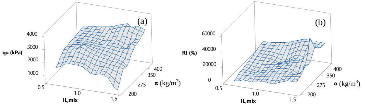
Şekil 4.24. I_{L,mix} ve \alpha ile a) q_u ve b) RI arasındaki ilişki (Büyük ölçekli DKK, UCS, 56 gün)
