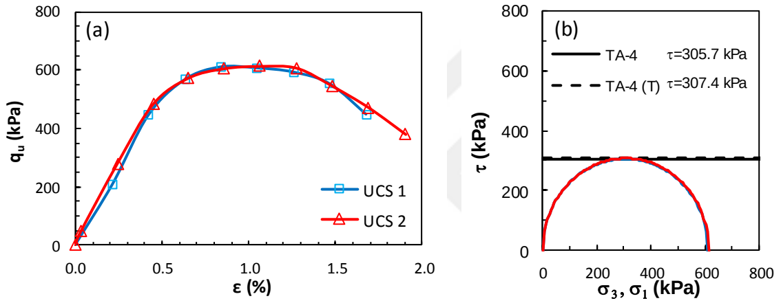
Şekil Ek 5.20. KÖ-4 numaralı tasarım: a) gerilme-birim deformasyon grafikleri ve b) Mohr daireleri (Küçük ölçekli DKK, UCS, 28 gün)
