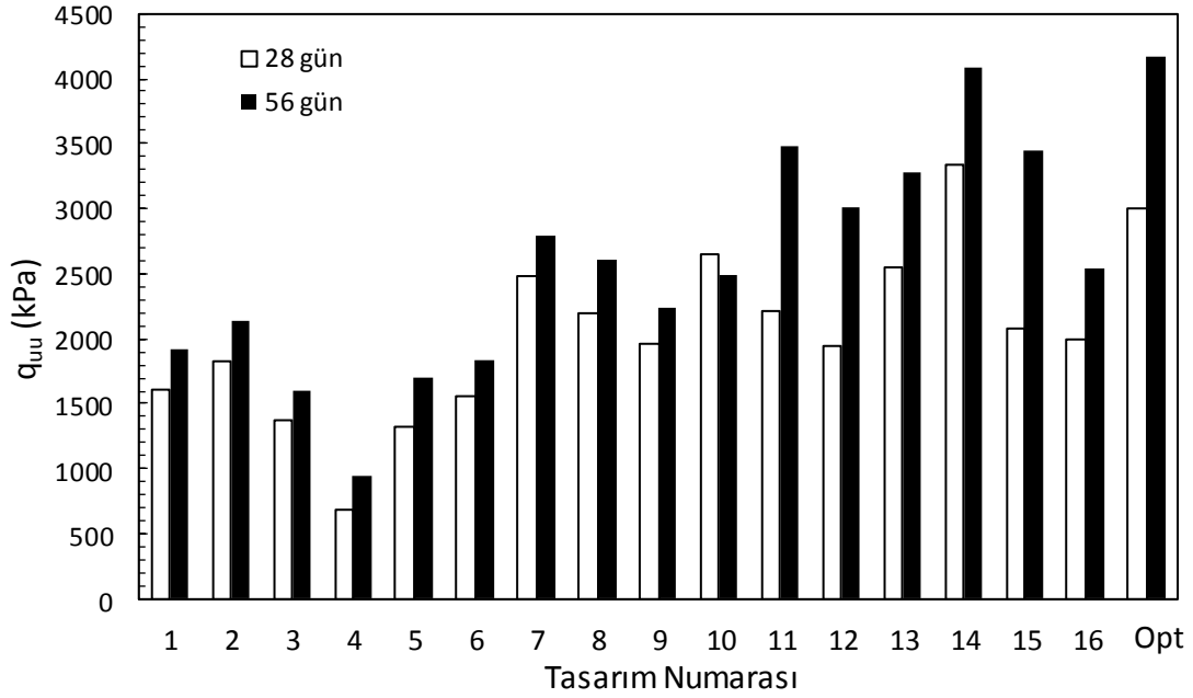
Şekil 4.35. Üç eksenli basınç deney sonuçları (Büyük ölçekli DKK, UU)
