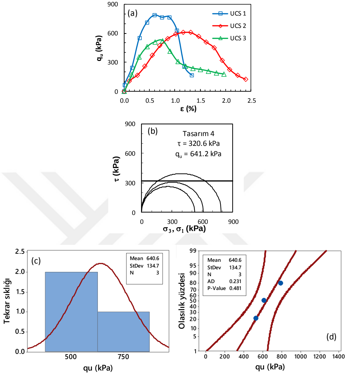
Şekil Ek 2.20. BÖ-4 numaralı kolona ait gerilme-birim deformasyon grafikleri: a) kolon üst bölgesi, b) Mohr daireleri, c) histogram grafiği, d) olasılık grafiği (Büyük ölçekli DKK, UCS, 56 gün)
