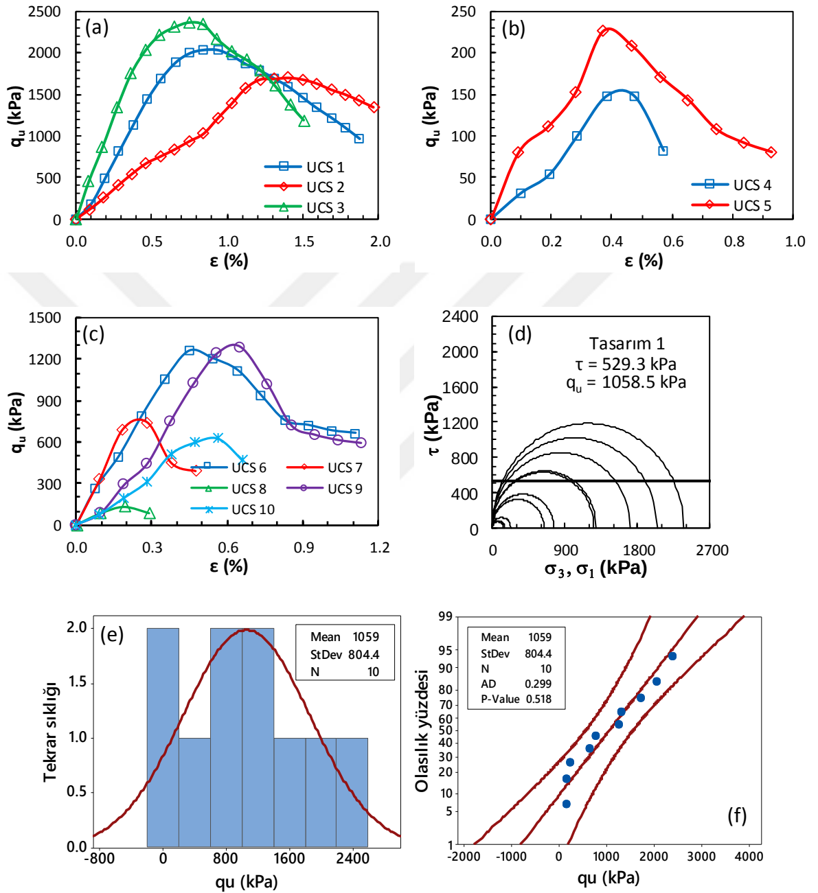
Şekil Ek 2.1 BÖ-1 numaralı kolona ait gerilme-birim deformasyon grafikleri: a) kolon üst bölgesi, b) kolon orta bölgesi, c) kolon alt bölgesi ve d) Mohr daireleri, e) histogram grafiği, f) olasılık grafiği (Büyük ölçekli DKK, UCS, 28 gün)
