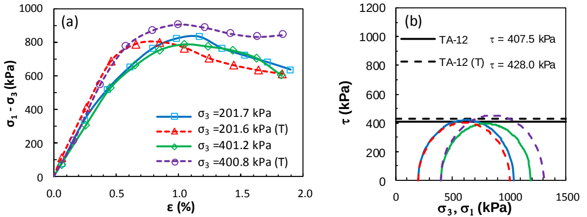
Şekil Ek 6.12. KÖ-12 numaralı tasarım: a) deviator gerilme-birim deformasyon grafikleri ve b) Mohr daireleri (Küçük ölçekli DKK, UU, 7 gün)
