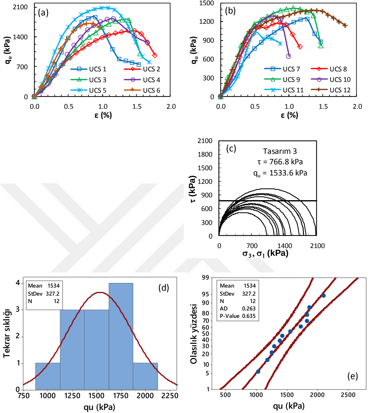
Şekil Ek 2.19. BÖ-3 numaralı kolona ait gerilme-birim deformasyon grafikleri: a) kolon üst bölgesi, b) kolon alt bölgesi ve c) Mohr daireleri, d) histogram grafiği, e) olasılık grafiği (Büyük ölçekli DKK, UCS, 56 gün)
