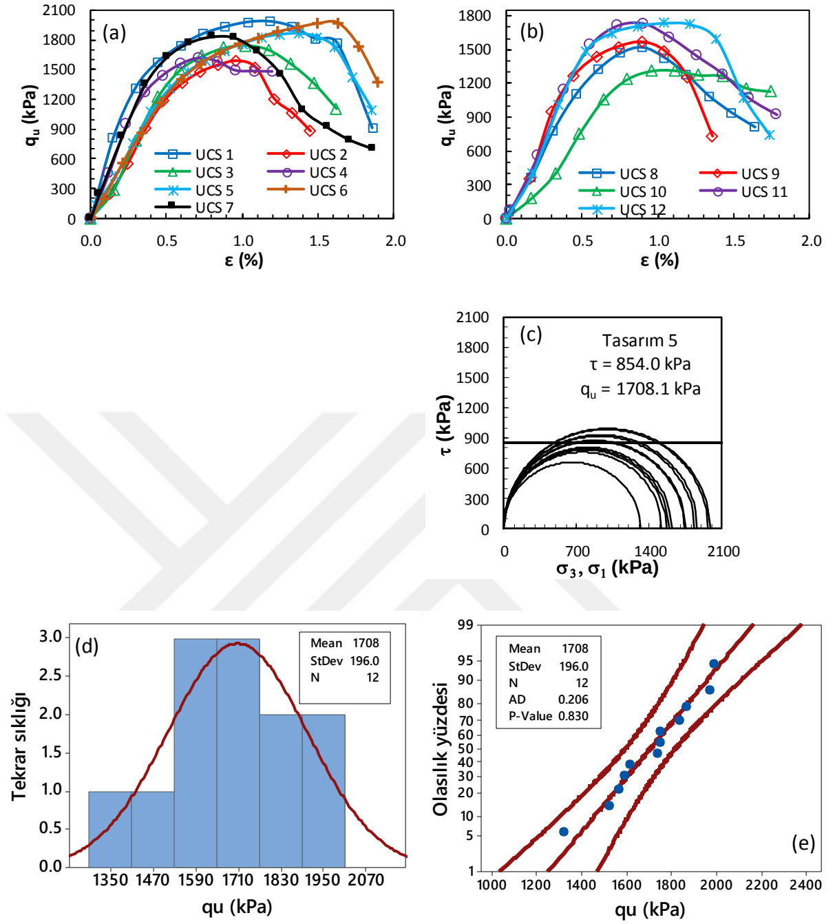
Şekil Ek 2.21. BÖ-5 numaralı kolona ait gerilme-birim deformasyon grafikleri: a) kolon üst bölgesi, b) kolon orta bölgesi ve c) Mohr daireleri, d) histogram grafiği, e) olasılık grafiği (Büyük ölçekli DKK, UCS, 56 gün)
