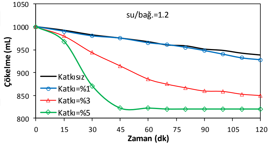
Şekil 3.49. Optima 100 katkısı ile yapılan sedimentasyon deneyi sonuçları (UKO=%60, su/bağlayıcı=1.2)
