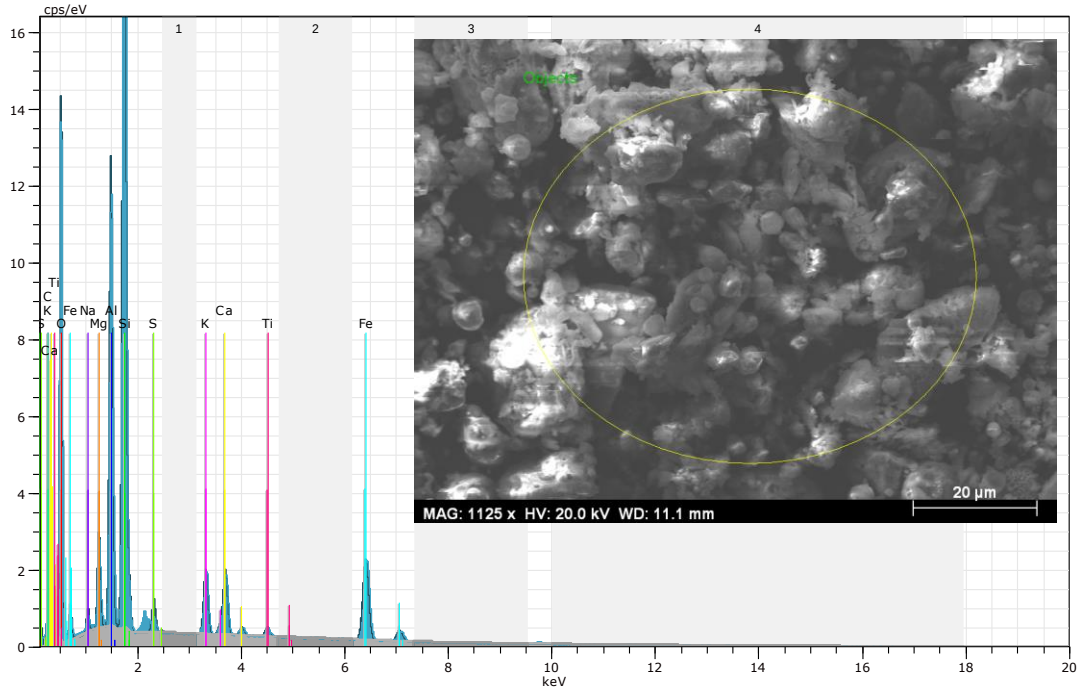
Şekil 4.120. Uçucu küle ait EDX analiz sonucu
