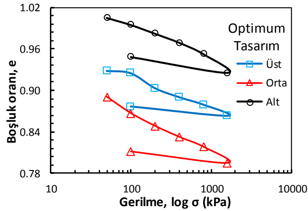
Şekil 4.85. Optimum tasarıma ait konsolidasyon deney sonuçları (Büyük ölçekli DKK, 28 gün)
