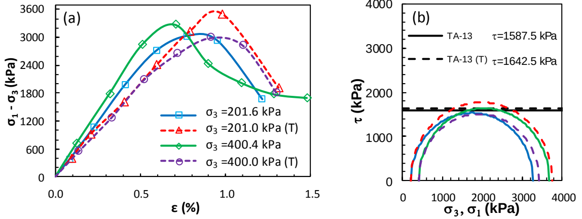
Şekil Ek 6.13. KÖ-13 numaralı tasarım: a) deviator gerilme-birim deformasyon grafikleri ve b) Mohr daireleri (Küçük ölçekli DKK, UU, 7 gün)
