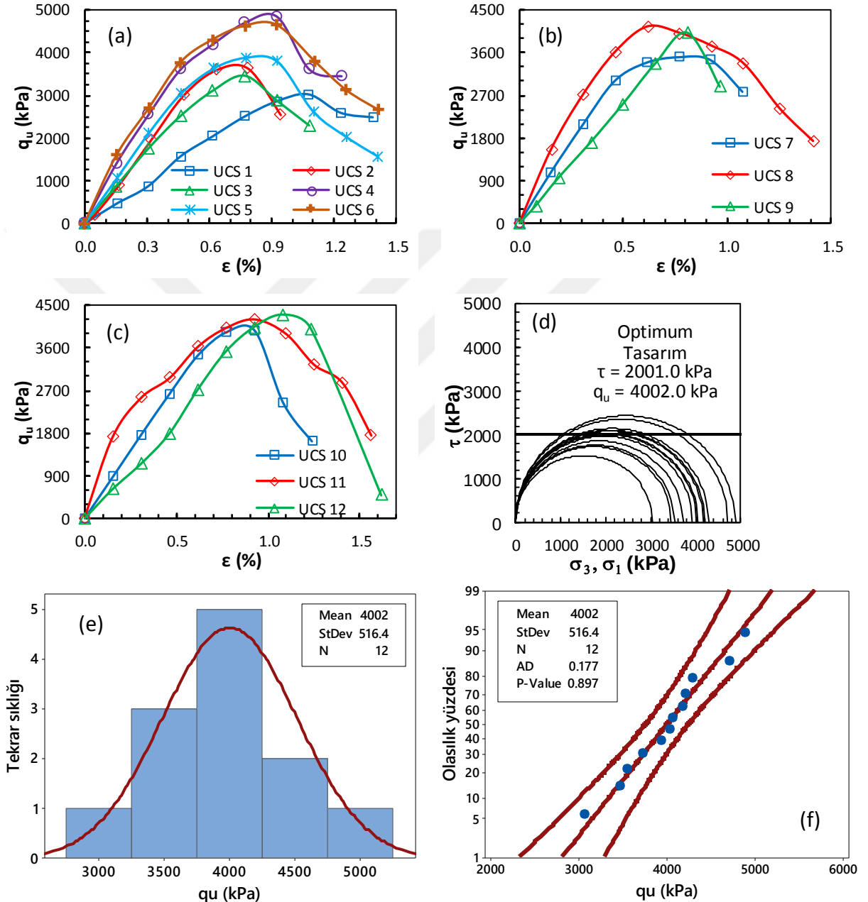
Şekil 4.81. Optimum tasarıma ait gerilme-birim deformasyon grafikleri: a) kolon üst bölgesi, b) kolon orta bölgesi, c) kolon alt bölgesi ve d) Mohr daireleri, e) histogram grafiği, f) olasılık grafiği (Büyük ölçekli DKK, UCS, 56 gün)
