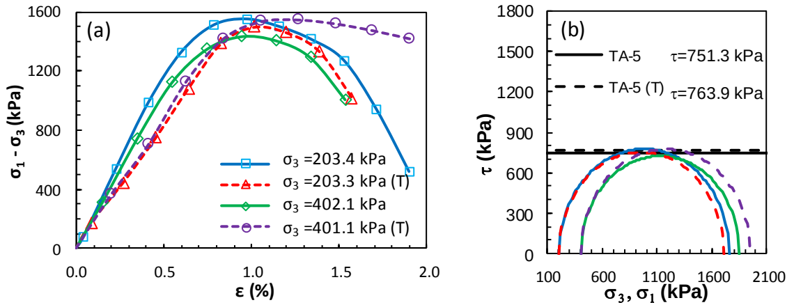
Şekil Ek 6.21. KÖ-5 numaralı tasarım: a) deviator gerilme-birim deformasyon grafikleri ve b) Mohr daireleri (Küçük ölçekli DKK, UU, 28 gün)
