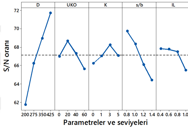
Şekil 4.51. Serbest basınç dayanımı için elde edilen S/N grafiği (Küçük ölçekli DKK, UCS, 28 gün)
