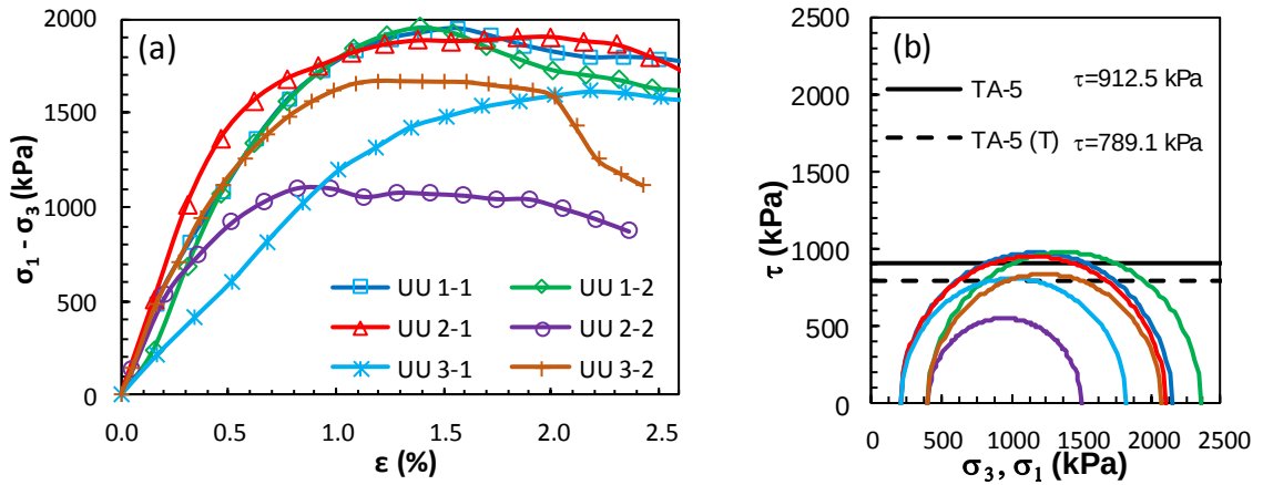
Şekil Ek 3.21. BÖ-5 numaralı kolona ait UU deney sonuçları: a) deviatör gerilme-birim boy kısalması grafikleri, b) Mohr daireleri ile kırılma zarfları (Büyük ölçekli DKK, UU, 56 gün)
