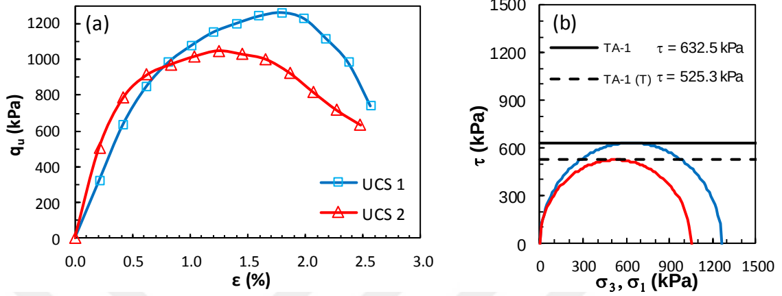
Şekil Ek 5.1. KÖ-1 numaralı tasarım: a) gerilme-birim deformasyon grafikleri ve b) Mohr daireleri (Küçük ölçekli DKK, UCS, 7 gün)
