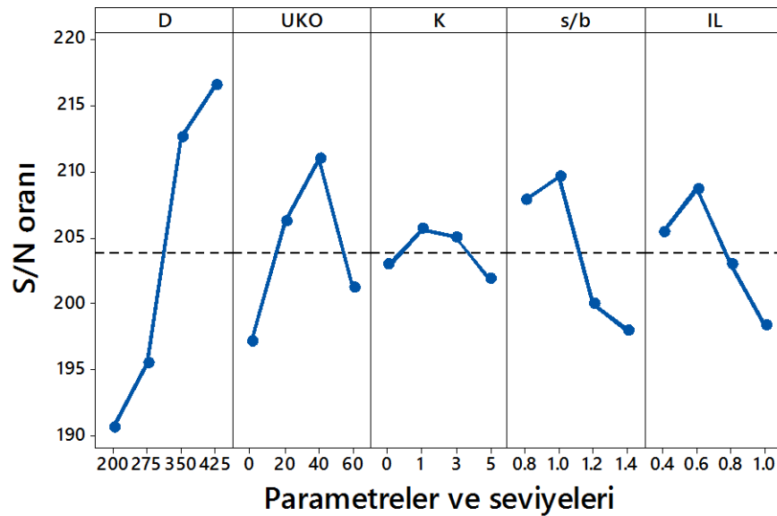
Şekil 4.45. Permeabilite katsayısı (k) için elde edilen S/N grafiği (Büyük ölçekli DKK, 56 gün)
