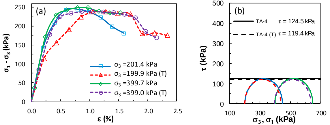
Şekil Ek 6.4. KÖ-4 numaralı tasarım: a) deviyör gerilme-birim deformasyon grafikleri ve b) Mohr daireleri (Küçük ölçekli DKK, UU, 7 gün)
