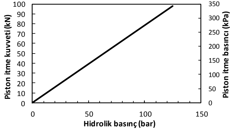
Şekil 3.22. Hidrolik pistonun çalışma basıncı-yük-gerilme ilişkisi (gerilme hesabı için 60 cm çapında yükleme başlığı dikkate alınmıştır)
