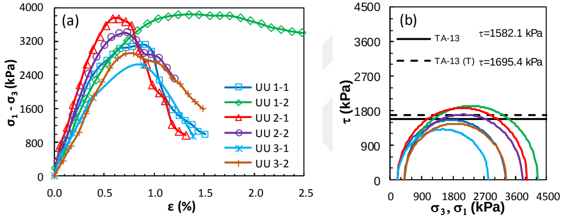
Şekil Ek 3.29. BÖ-13 numaralı kolona ait UU deney sonuçları: a) deviator gerilme-birim boy kısalması grafikleri, b) Mohr daireleri ile kırılma zarfları (Büyük ölçekli DKK, UU, 56 gün)
