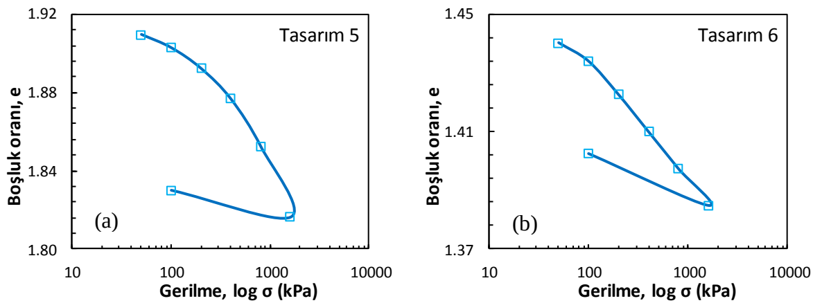
Şekil Ek 7.3. Küçük ölçekli DKK, konsolidasyon deneyi, 28 gün: a) Tasarım 5 ve b) Tasarım 6
