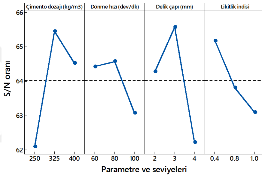
Şekil 4.12. Kolon dayanımı için elde edilen S/N grafiği (Sistem parametrelerinin araştırılması)
