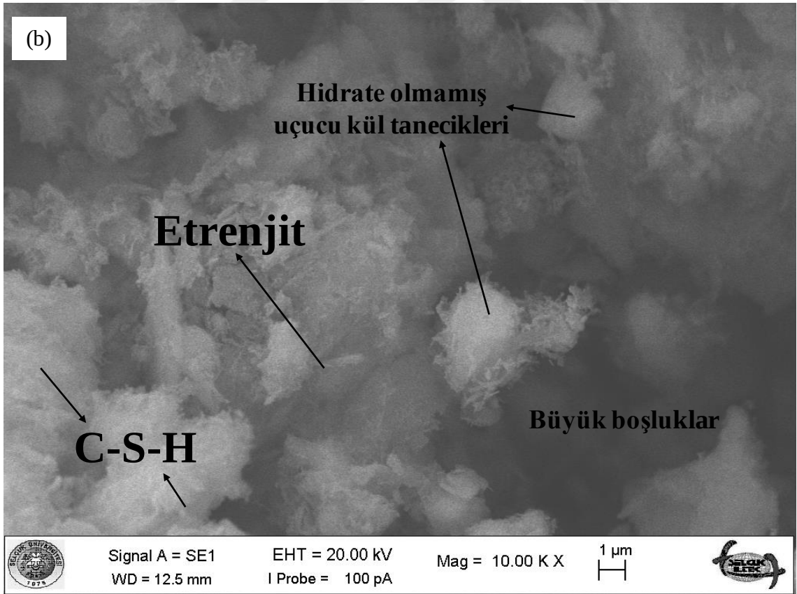
Şekil 4.135. Tasarım 4'e ait SEM görüntüleri: a) x5000, b) x10000 (Büyük ölçekli DKK, 28 gün)
