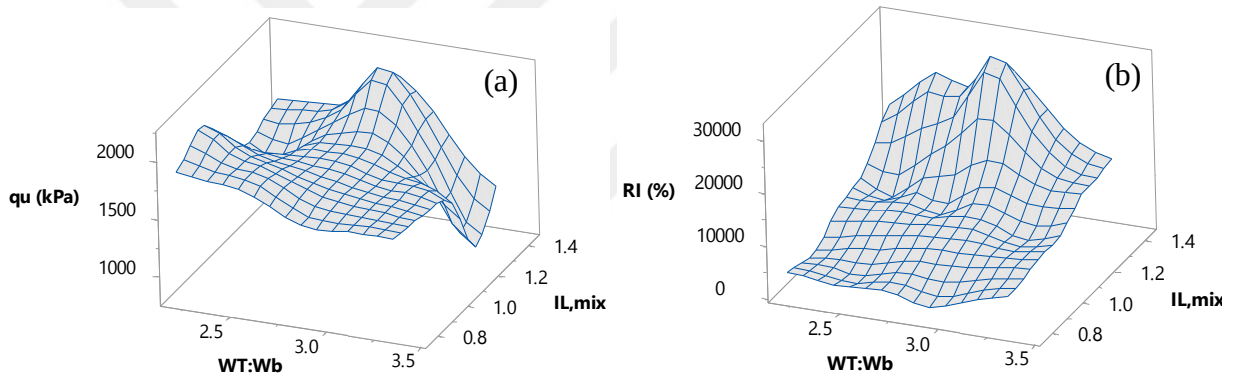
Şekil 4.9. I_{L,mix} ve W_T:W_b ile a) q_u ve b) RI arasındaki ilişki
