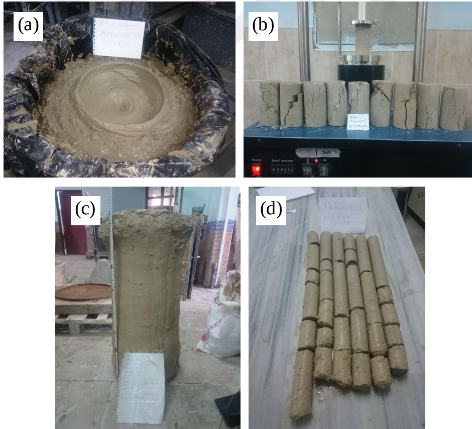
Şekil 4.16. Optimum durumda imaledilen DKK: a) imalat sonrası görünüm, b) karot numunelerinin kayma yüzeyleri, c) imal edilen kolon ve d) alınan karot numuneleri (Sistem parametrelerinin araştırılması)
