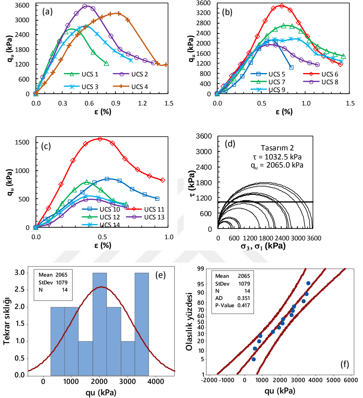
Şekil Ek 2.18. BÖ-2 numaralı kolona ait gerilme-birim deformasyon grafikleri: a) kolon üst bölgesi, b) kolon orta bölgesi, c) kolon alt bölgesi ve d) Mohr daireleri, e) histogram grafiği, f) olasılık grafiği (Büyük ölçekli DKK, UCS, 56 gün)
