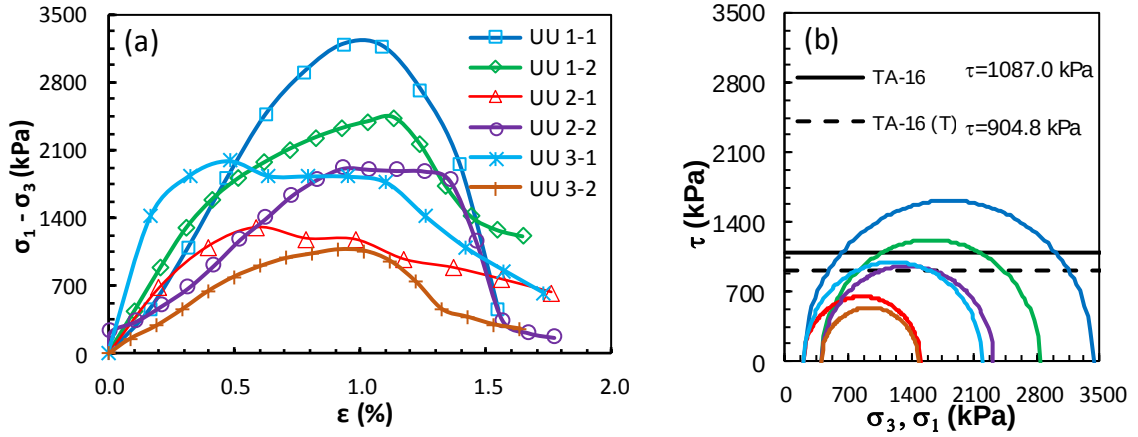
Şekil Ek 3.16. BÖ-16 numaralı kolona ait UU deney sonuçları: a) deviatör gerilme-birim boy kısalması grafikleri, b) Mohr daireleri ile kırılma zarfları (Büyük ölçekli DKK, UU, 28 gün)
