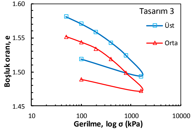
Şekil Ek 4.19. BÖ-3 numaralı kolona ait konsolidasyon deney sonucu (Büyük ölçekli DKK, 56 gün)
