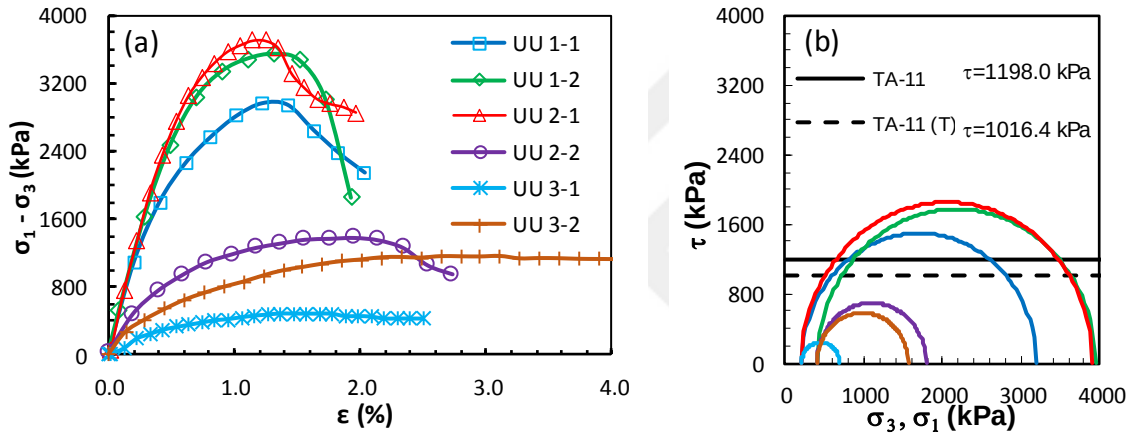
Şekil Ek 3.11. BÖ-11 numaralı kolona ait UU deney sonuçları: a) deviator gerilme-birim boy kısalması grafikleri, b) Mohr daireleri ile kırılma zarfları (Büyük ölçekli DKK, UU, 28 gün)
