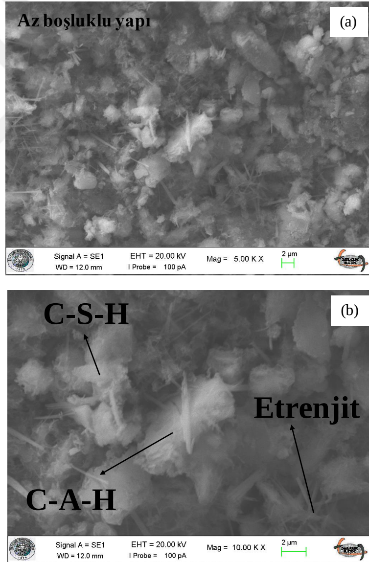
Şekil 4.139. Optimum tasarıma ait SEM görüntüleri: a) x5000, b) x10000 (Büyük ölçekli DKK, 28 gün)
