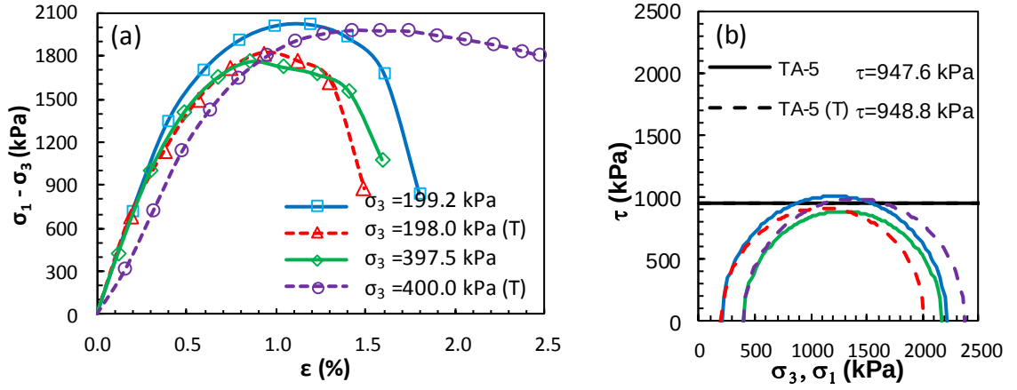
Şekil Ek 6.37. KÖ-5 numaralı tasarım: a) deviator gerilme-birim deformasyon grafikleri ve b) Mohr daireleri (Küçük ölçekli DKK, UU, 56 gün)
