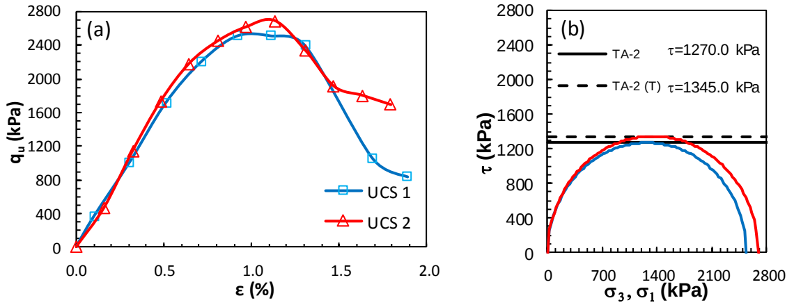
Şekil Ek 5.34. KÖ-2 numaralı tasarım: a) gerilme-birim deformasyon grafikleri ve b) Mohr daireleri (Küçük ölçekli DKK, UCS, 56 gün)
