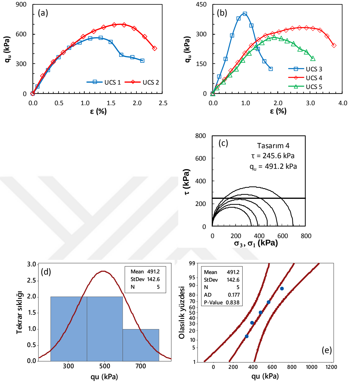
Şekil Ek 2.4. BÖ-4 numaralı kolona ait gerilme-birim deformasyon grafikleri: a) kolon üst bölgesi, b) kolon alt bölgesi ve d) Mohr daireleri, e) histogram grafiği, f) olasılık grafiği (Büyük ölçekli DKK, UCS, 28 gün)
