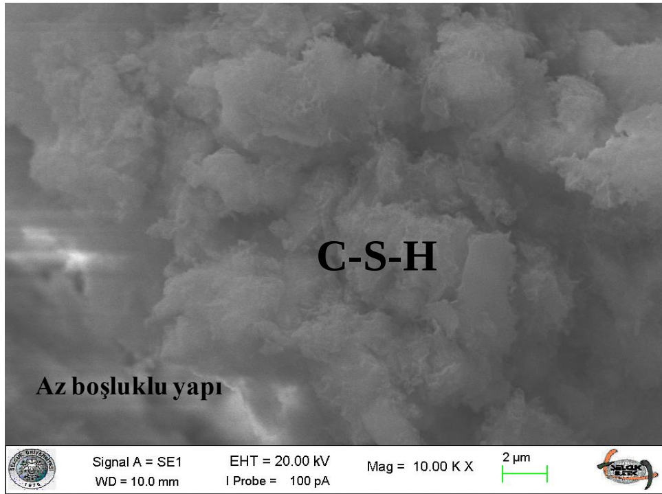
Şekil 4.127. Optimum tasarıma ait SEM görüntüleri (Küçük ölçekli DKK, 28 gün)
