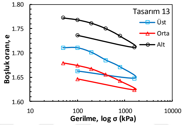
Şekil Ek 4.29. BÖ-13 numaralı kolona ait konsolidasyon deney sonucu (Büyük ölçekli DKK, 56 gün)
