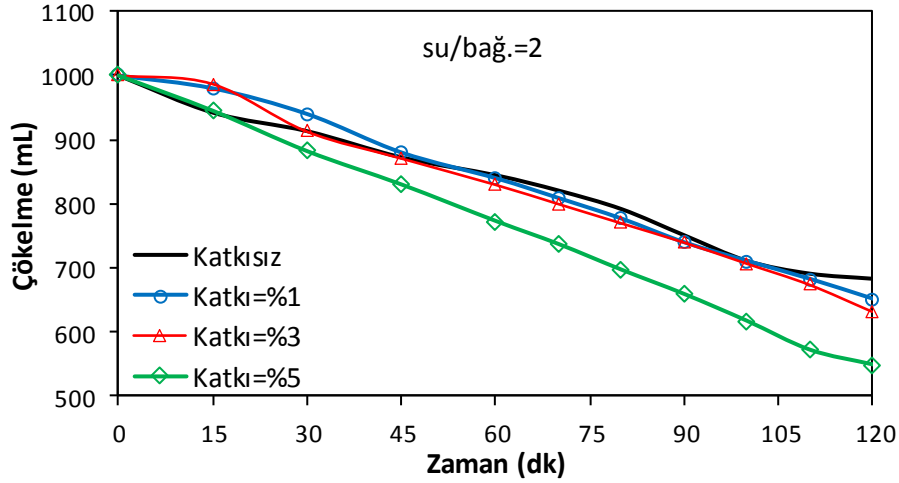
Şekil 3.51. Optima 100 katkısı ile yapılan sedimentasyon deneyi sonuçları (UKO=%60, su/bağlayıcı=2)
