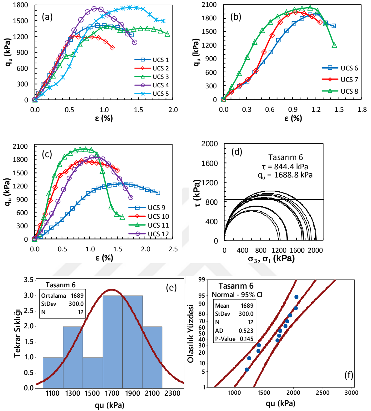
Şekil Ek 1.6. SP-6 numaralı kolona ait gerilme-birim deformasyon grafikleri: a) kolon alt bölgesi, b) kolon orta bölgesi, c) kolon üst bölgesi ve d) Mohr daireleri, e) histogram grafiği, f) olasılık grafiği (Sistem parametreleri, UCS, 28 gün)
