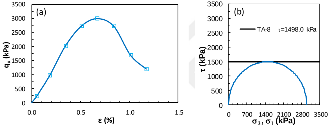
Şekil Ek 5.41. KÖ-9 numaralı tasarım: a) gerilme-birim deformasyon grafikleri ve b) Mohr daireleri (Küçük ölçekli DKK, UCS, 56 gün)
