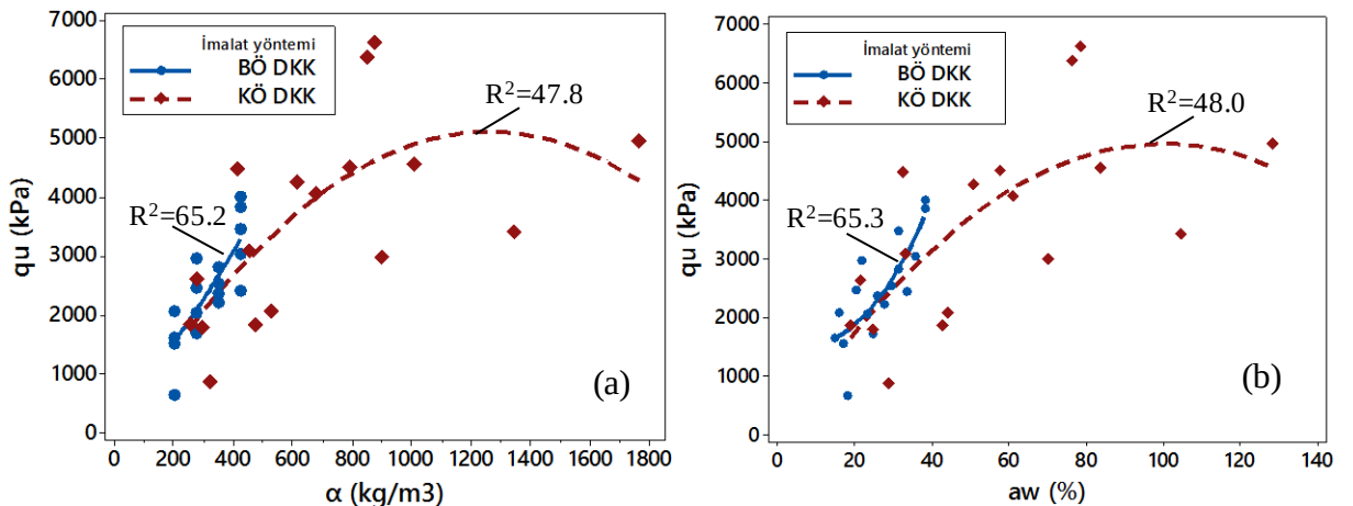
Şekil 4.96. Serbest basınç dayanımının a) \alpha ve b) a_w ile ilişkileri (Küçük ve büyük ölçekli DKK, 56 gün)
