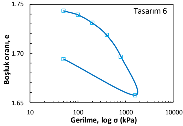
Şekil Ek 4.6. BÖ-6 numaralı kolona ait konsolidasyon deney sonucu (Büyük ölçekli DKK, 28 gün)
