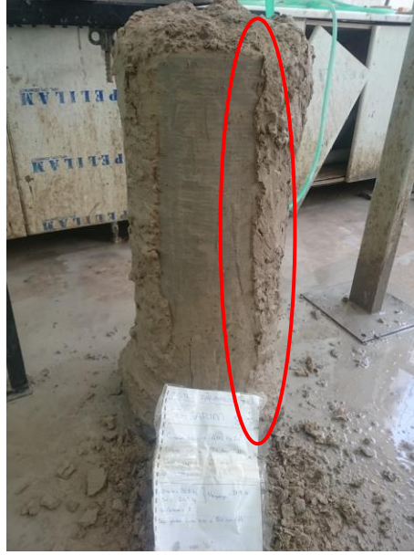
Şekil 4.2. Kolon yüzeyi ile iyileştirilecek zemin arasında oluşan ara yüzey tabakası
