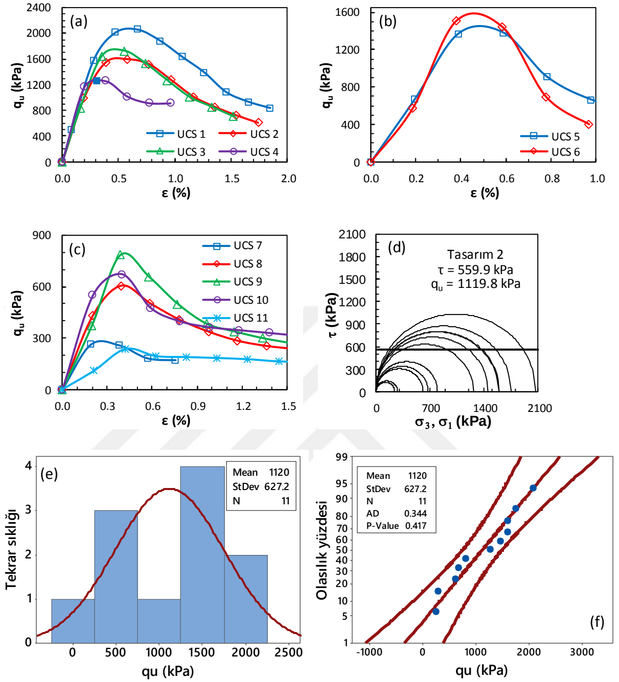
Şekil Ek 2.2. BÖ-2 numaralı kolona ait gerilme-birim deformasyon grafikleri: a) kolon üst bölgesi, b) kolon orta bölgesi, c) kolon alt bölgesi ve d) Mohr daireleri, e) histogram grafiği, f) olasılık grafiği (Büyük ölçekli DKK, UCS, 28 gün)
