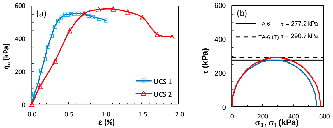
Şekil Ek 5.6. KÖ-6 numaralı tasarım: a) gerilme-birim deformasyon grafikleri ve b) Mohr daireleri (Küçük ölçekli DKK, UCS, 7 gün)
