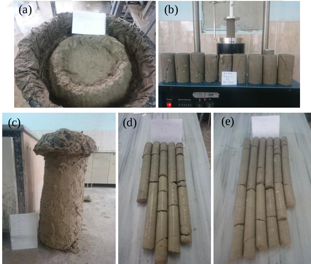
Şekil 3.63. Büyük ölçekli DKK, Tasarım 12: a) imalat sonrası görünüm, b) kayma yüzeyleri, c) imal edilen kolon, d) 28 ve e) 56 günlük karot numuneleri (büyük ölçekli DKK)
