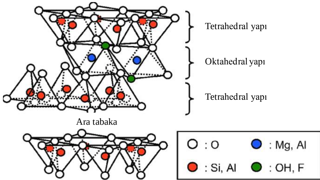
Şekil 2.1. Smektit grubu killerin mineral yapısı (Ino ve ark., 2011)
