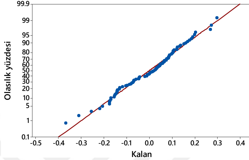
Şekil 4.115. RI sonuçları için geliştirilen modeldeki hataların normal olasılık grafiği (Büyük ölçekli DKK)
