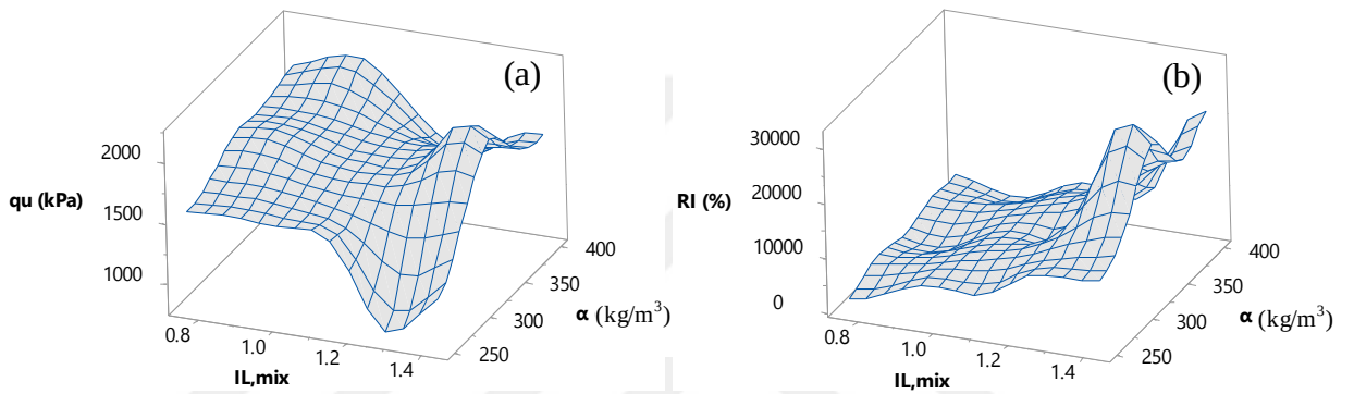
Şekil 4.4. Çimento faktörü ve karışımın likitlik indisi ile a) q_u ve b) RI arasındaki ilişki
