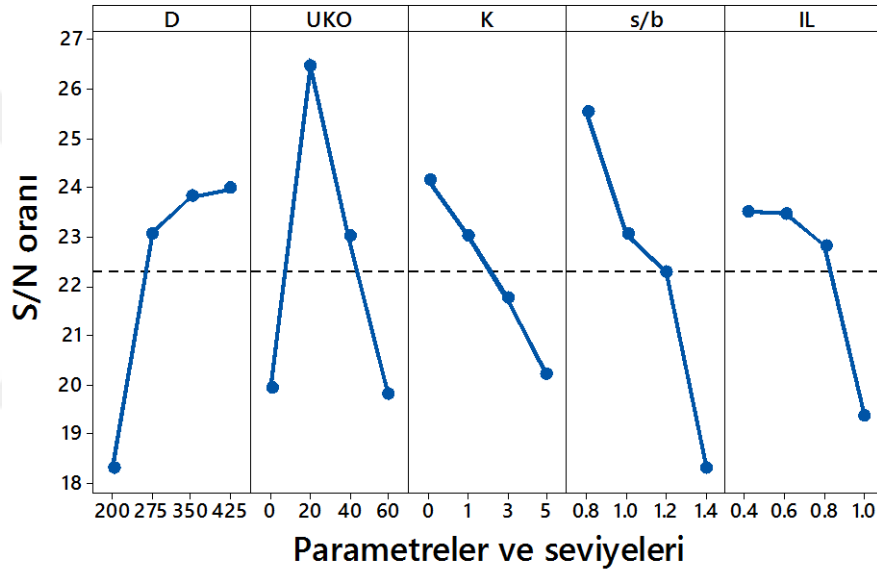
Şekil 4.67. Sıkışma indisi (Cc) için elde edilen S/N grafiği (Küçük ölçekli DKK, konsolidasyon, 28 gün)
