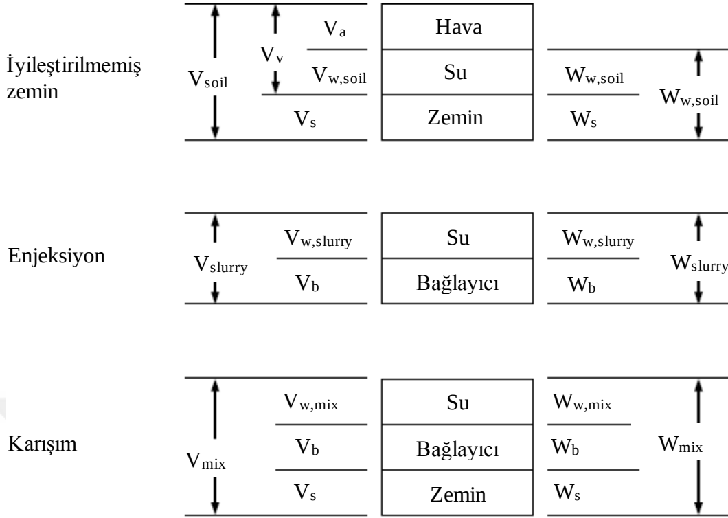
Şekil 2.11. Islak karıştırma yöntemi için kullanılan faz diyagramı
