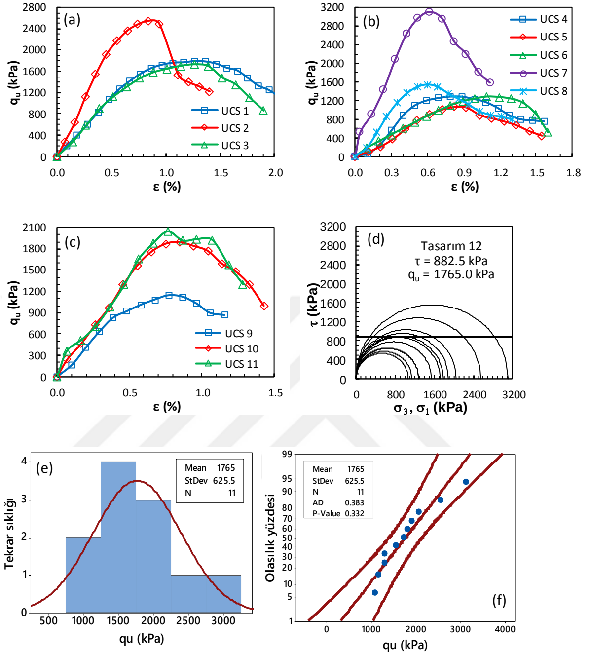
Şekil Ek 2.12. BÖ-12 numaralı kolona ait gerilme-birim deformasyon grafikleri: a) kolon üst bölgesi, b) kolon orta bölgesi, c) kolon alt bölgesi ve d) Mohr daireleri, e) histogram grafiği, f) olasılık grafiği (Büyük ölçekli DKK, UCS, 28 gün)
