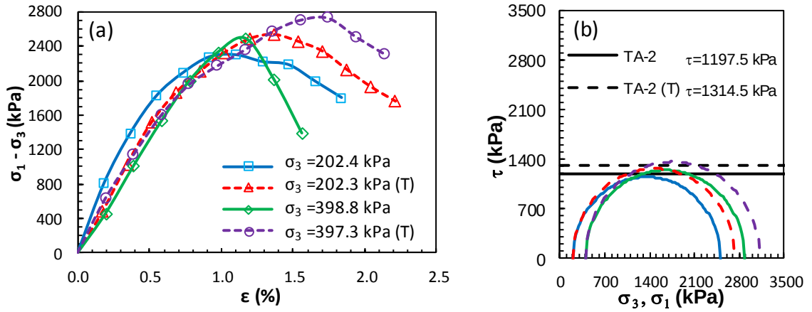
Şekil Ek 6.34. KÖ-2 numaralı tasarım: a) deviator gerilme-birim deformasyon grafikleri ve b) Mohr daireleri (Küçük ölçekli DKK, UU, 56 gün)
