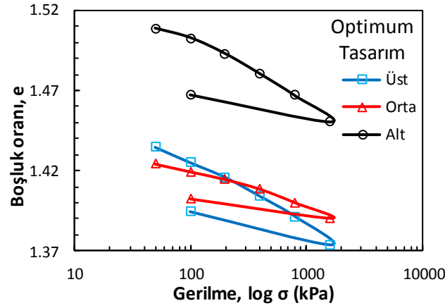
Şekil 4.86. Optimum tasarıma ait konsolidasyon deney sonuçları (Büyük ölçekli DKK, 56 gün)
