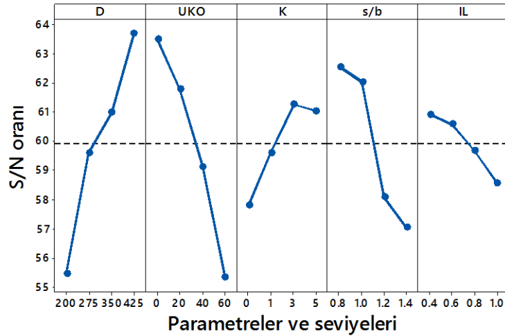
Şekil 4.58. Üç eksenli basınç dayanımı için elde edilen S/N grafiği (Küçük ölçekli DKK, UU, 7 gün)
