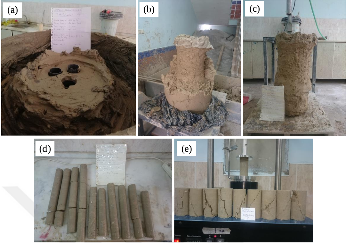
Şekil 3.41. SP-7 numaralı DKK: a) imalat sonrası görünüm, b) kolon tanktan çıkarılırken, c) imal edilen kolon, d) alınan karot numuneleri, e) UCS deneyindeki kayma yüzeyi (Sistem parametrelerinin araştırılması)
