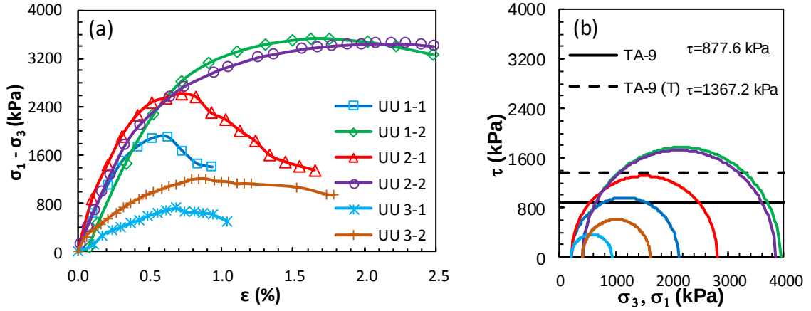
Şekil Ek 3.25. BÖ-9 numaralı kolona ait UU deney sonuçları: a) deviator gerilme-birim boy kısalması grafikleri, b) Mohr daireleri ile kırılma zarfları (Büyük ölçekli DKK, UU, 56 gün)
