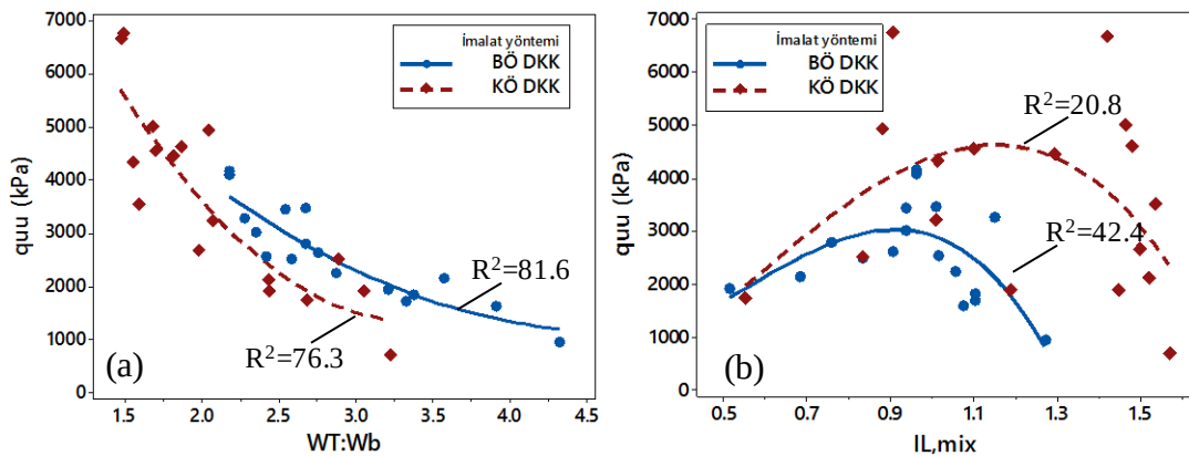
Şekil 4.99. Üç eksenli basınç dayanımının a) W_T:W_b ve b) I_{L,mix} ile ilişkileri (Küçük ve büyük ölçekli DKK, 56 gün)
