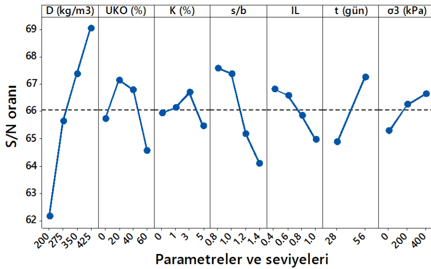
Şekil 4.111. \sigma_1 - \sigma_3 için elde edilen S/N grafiği (Büyük ölçekli DKK)
