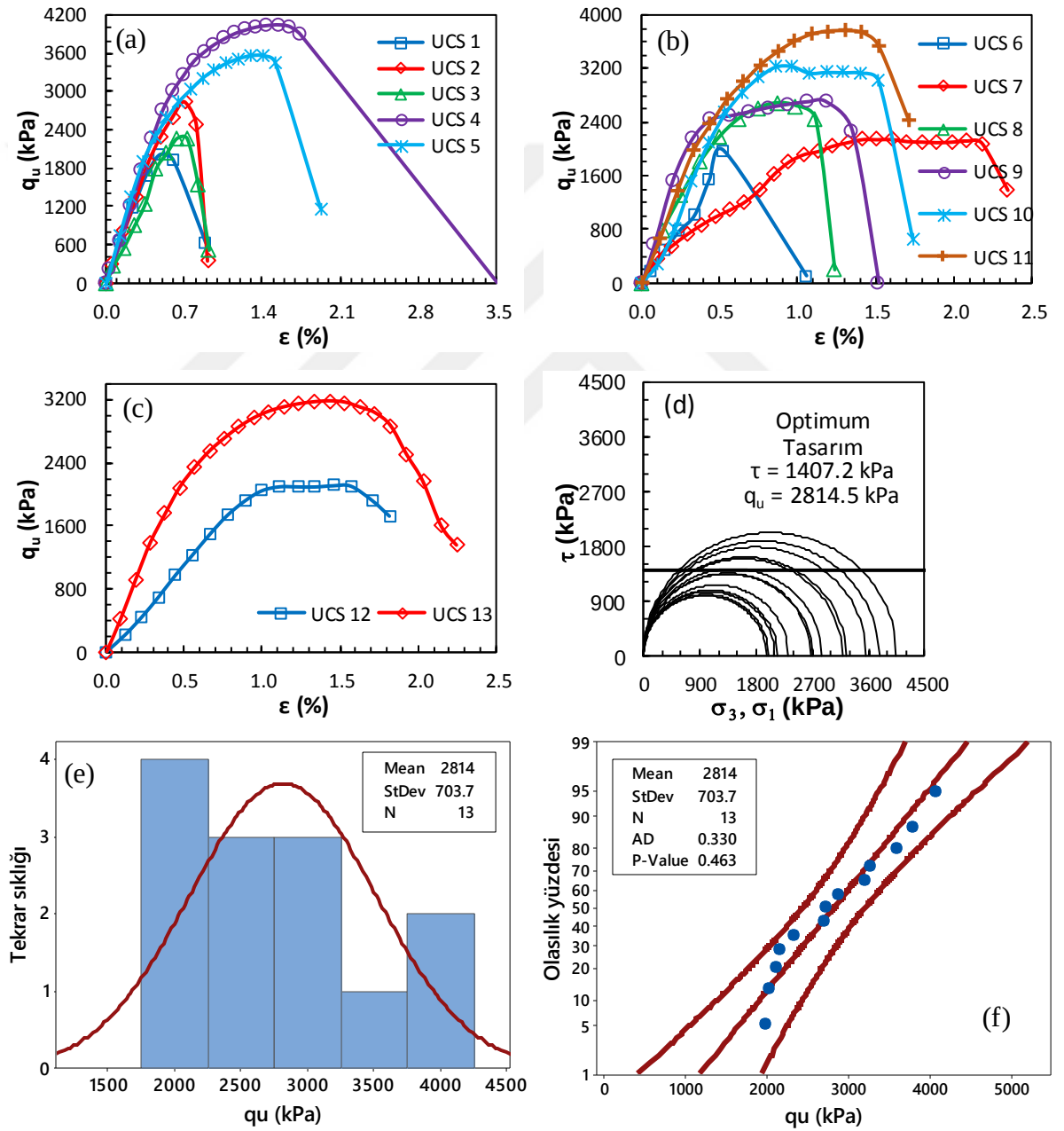
Şekil 4.82. Optimum tasarıma ait gerilme-birim deformasyon grafikleri: a) kolon üst bölgesi, b) kolon orta bölgesi, c) kolon alt bölgesi ve d) Mohr daireleri, e) histogram grafiği, f) olasılık grafiği (Büyük ölçekli DKK, UCS, 28 gün)
