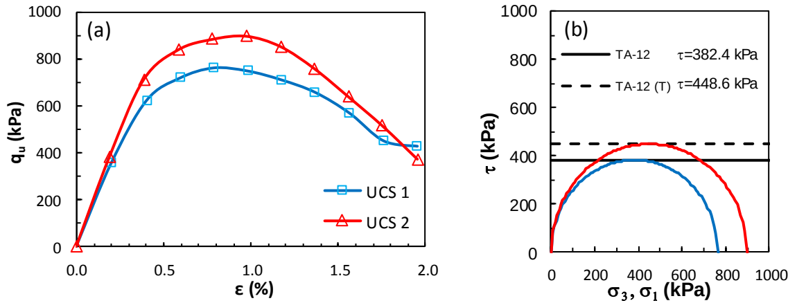
Şekil Ek 5.12. KÖ-12 numaralı tasarım: a) gerilme-birim deformasyon grafikleri ve b) Mohr daireleri (Küçük ölçekli DKK, UCS, 7 gün)
