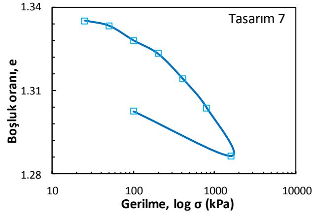
Şekil Ek 4.7. BÖ-7 numaralı kolona ait konsolidasyon deney sonucu (Büyük ölçekli DKK, 28 gün)
