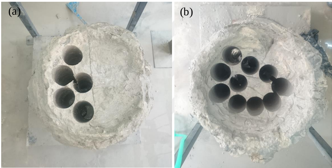
Şekil 3.68. Uçucu kül katkılı kolonlardan karot alınması: a) 28 gün sonra, b) 56 gün sonra
