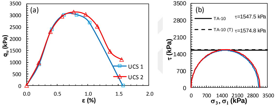
Şekil Ek 5.26. KÖ-10 numaralı tasarım: a) gerilme-birim deformasyon grafikleri ve b) Mohr daireleri (Küçük ölçekli DKK, UCS, 28 gün)
