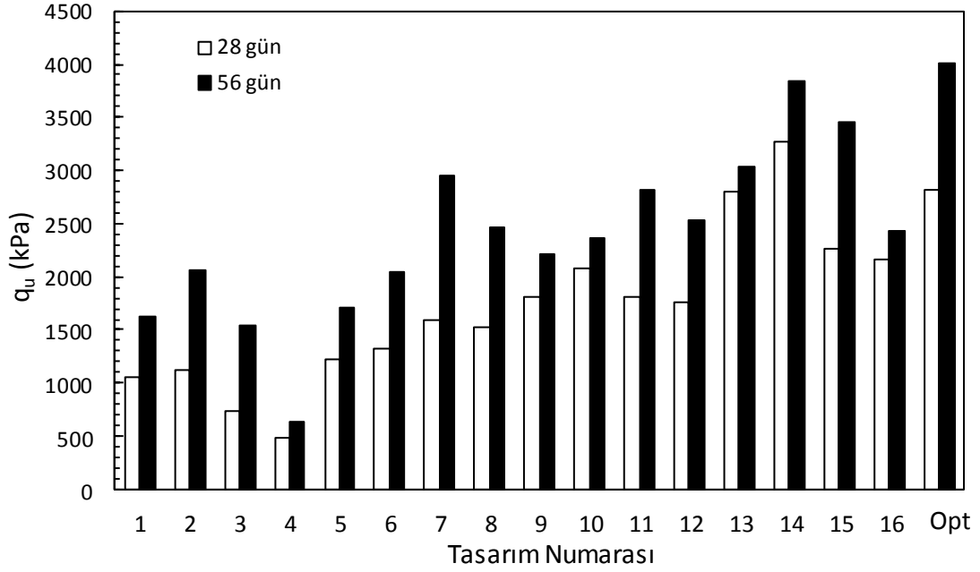
Şekil 4.23. Serbest basınç deney sonuçları (Büyük ölçekli DKK, UCS)
