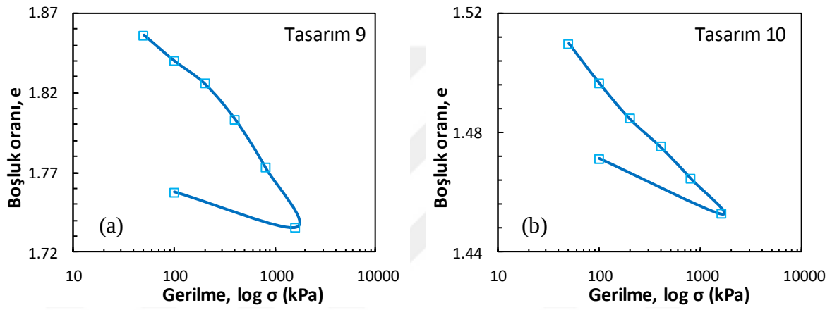
Şekil Ek 7.5. Küçük ölçekli DKK, konsolidasyon deneyi, 28 gün: a) Tasarım 9 ve b) Tasarım 10
