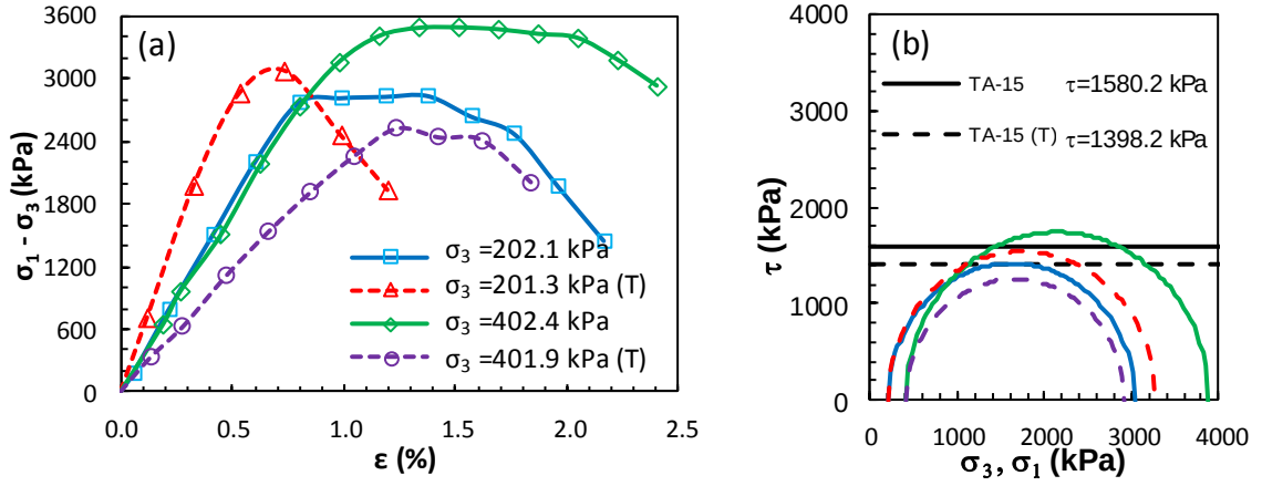
Şekil Ek 6.31. KÖ-15 numaralı tasarım: a) deviator gerilme-birim deformasyon grafikleri ve b) Mohr daireleri (Küçük ölçekli DKK, UU, 28 gün)
