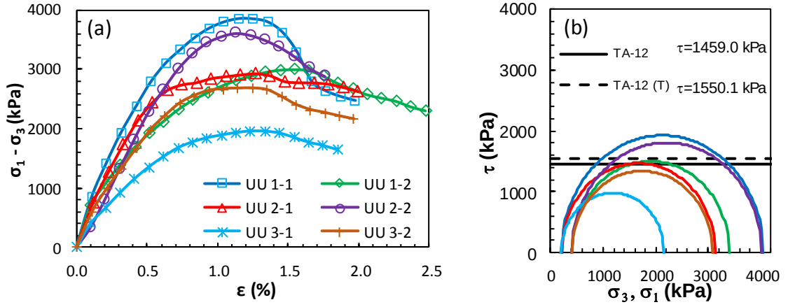
Şekil Ek 3.28. BÖ-12 numaralı kolona ait UU deney sonuçları: a) deviator gerilme-birim boy kısalması grafikleri, b) Mohr daireleri ile kırılma zarfları (Büyük ölçekli DKK, UU, 56 gün)
