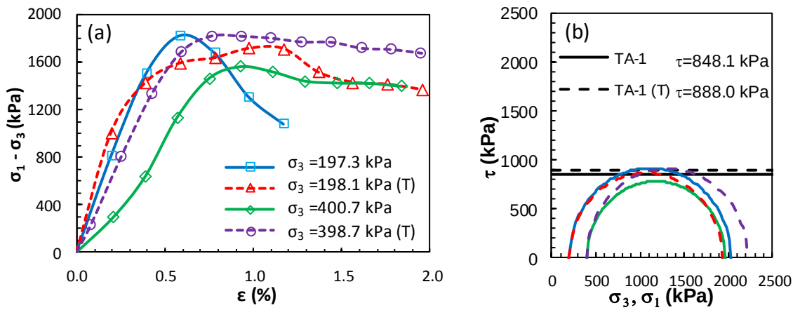
Şekil Ek 6.33. KÖ-1 numaralı tasarım: a) deviator gerilme-birim deformasyon grafikleri ve b) Mohr daireleri (Küçük ölçekli DKK, UU, 56 gün)
