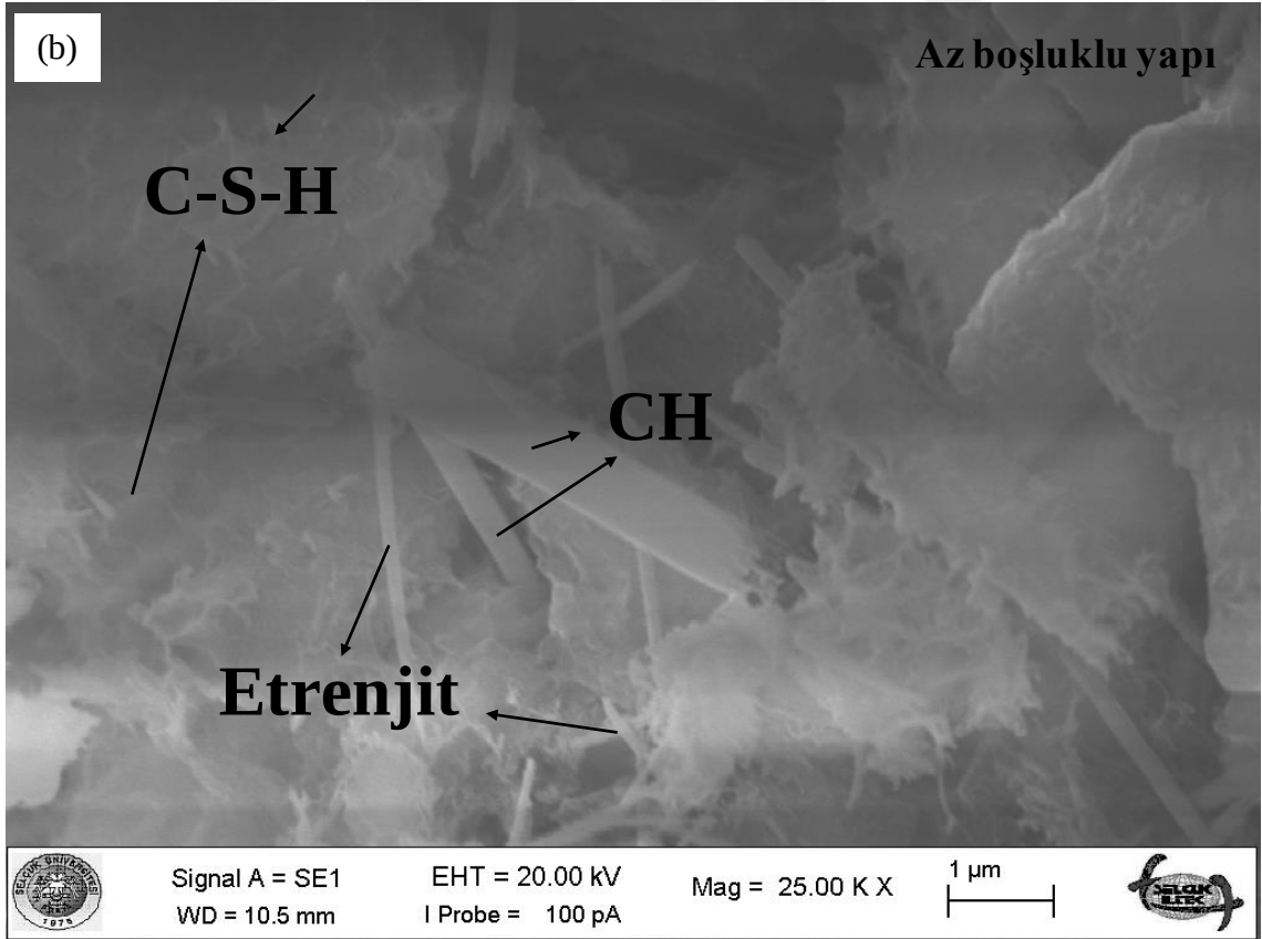
Şekil 4.137. Tasarım 14'e ait SEM görüntüleri: a) x10000, b) x25000 (Büyük ölçekli DKK, 28 gün)
