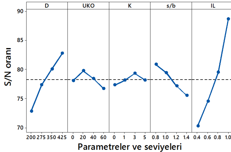
Şekil 4.52. Zemin iyileştirme derecesi için elde edilen S/N grafiği (Küçük ölçekli DKK, UCS, 28 gün)
