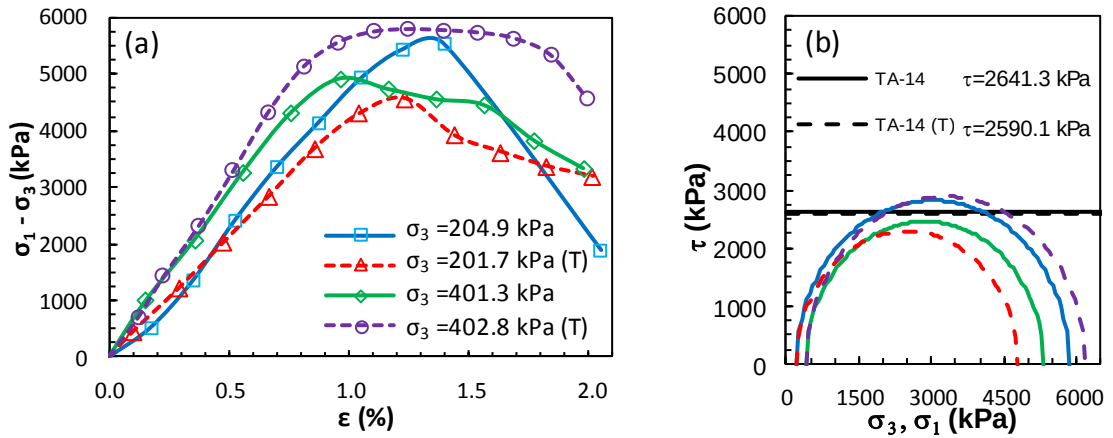
Şekil Ek 6.30. KÖ-14 numaralı tasarım: a) deviator gerilme-birim deformasyon grafikleri ve b) Mohr daireleri (Küçük ölçekli DKK, UU, 28 gün)
