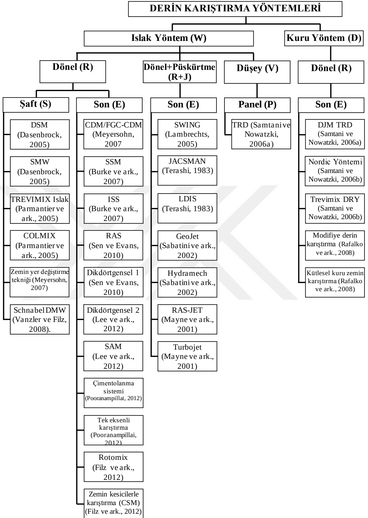
Şekil 2.4. DKK imalat yöntemlerinin sınıflandırılması (Bruce 2000a, b)
