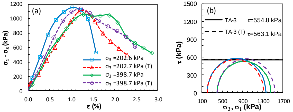
Şekil Ek 6.19. KÖ-3 numaralı tasarım: a) deviator gerilme-birim deformasyon grafikleri ve b) Mohr daireleri (Küçük ölçekli DKK, UU, 28 gün)
