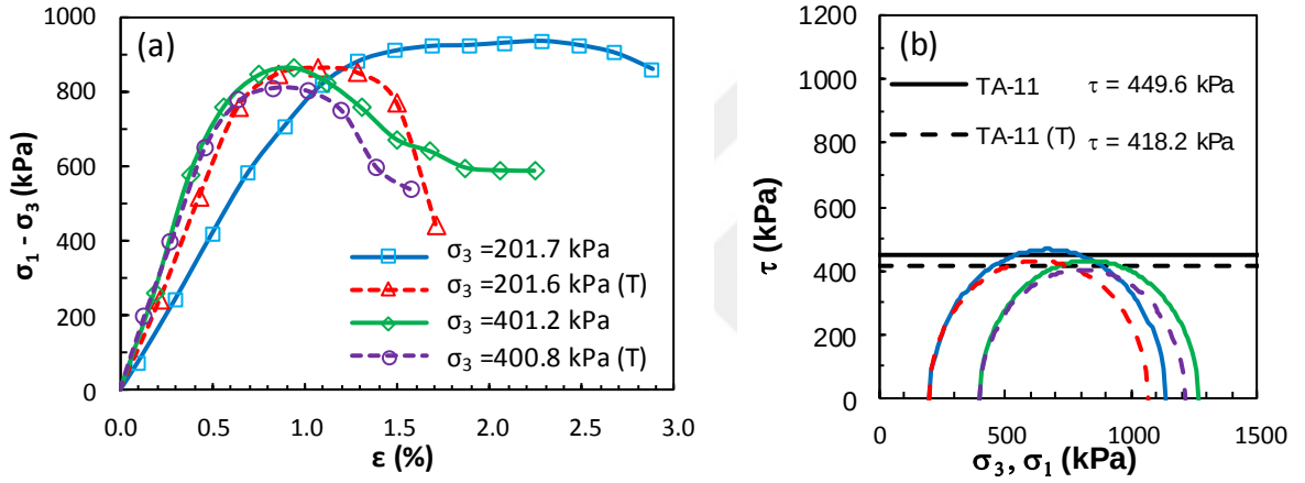
Şekil Ek 6.11. KÖ-11 numaralı tasarım: a) deviator gerilme-birim deformasyon grafikleri ve b) Mohr daireleri (Küçük ölçekli DKK, UU, 7 gün)
