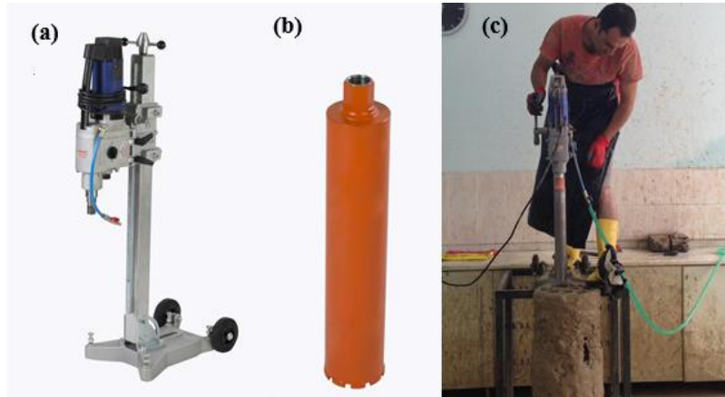
Şekil 3.23. a) Karot makinesi, b) 60 mm çaplı karot ucu ve c) karot alınması
