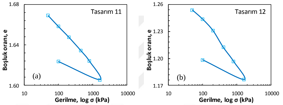
Şekil Ek 7.14. Küçük ölçekli DKK, konsolidasyon deneyi, 56 gün: a) Tasarım 11 ve b) Tasarım 12
