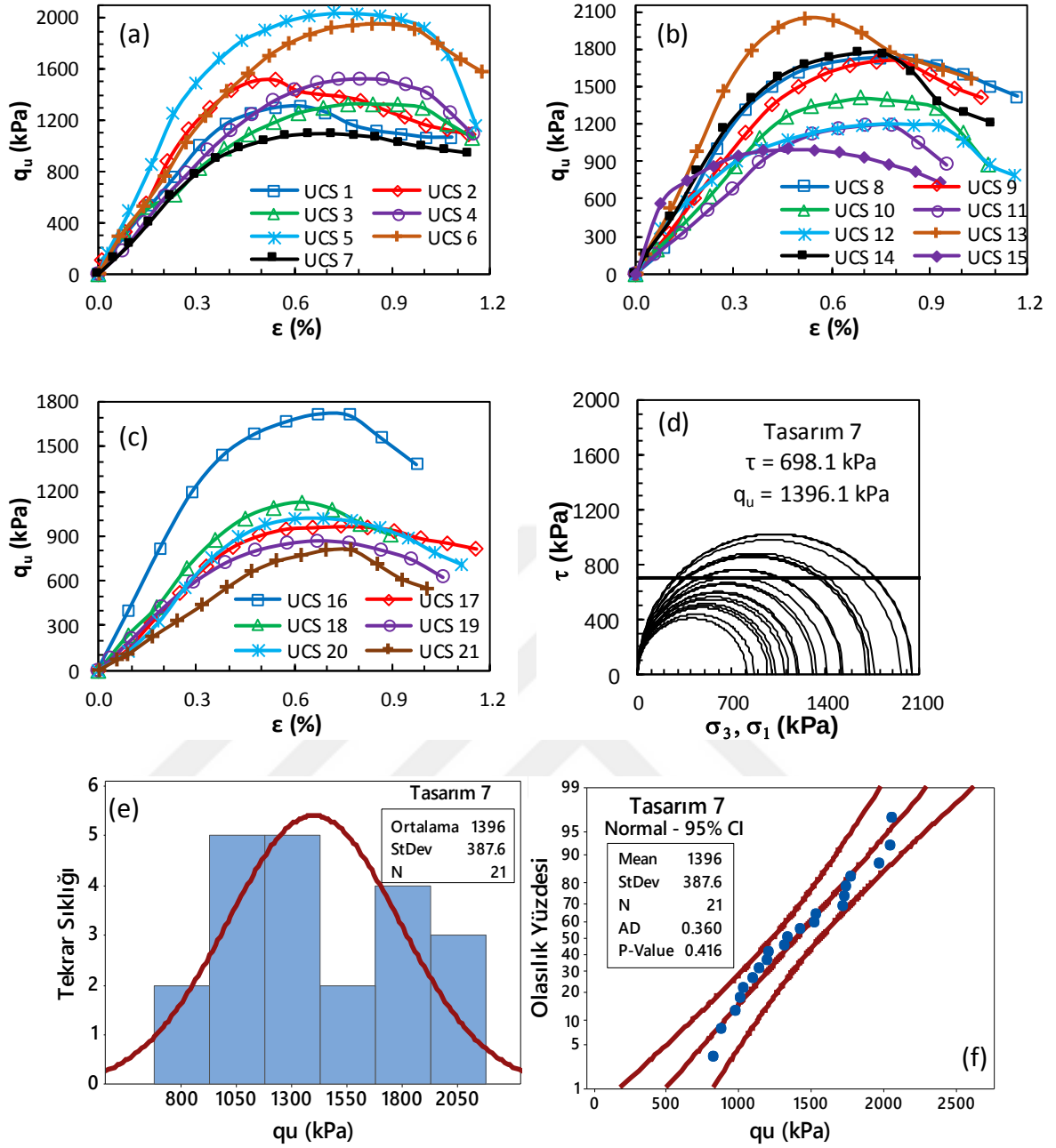
Şekil Ek 1.7. SP-7 numaralı kolona ait gerilme-birim deformasyon grafikleri: a) kolon alt bölgesi, b) kolon orta bölgesi, c) kolon üst bölgesi ve d) Mohr daireleri, e) histogram grafiği, f) olasılık grafiği (Sistem parametreleri, UCS, 28 gün)
