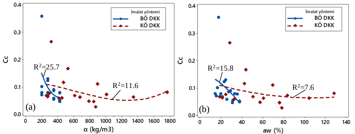
Şekil 4.100. Sıkışma indisinin a) \alpha ve b) a_w ile ilişkileri (Küçük ve büyük ölçekli DKK, 56 gün)
