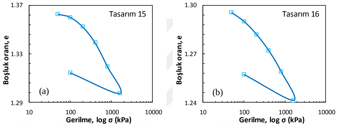
Şekil Ek 7.8. Küçük ölçekli DKK, konsolidasyon deneyi, 28 gün: a) Tasarım 15 ve b) Tasarım 16
