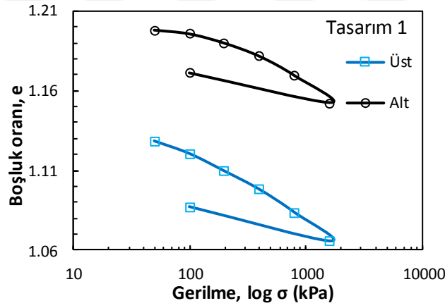
Şekil Ek 4.17. BÖ-1 numaralı kolona ait konsolidasyon deney sonucu (Büyük ölçekli DKK, 56 gün)
