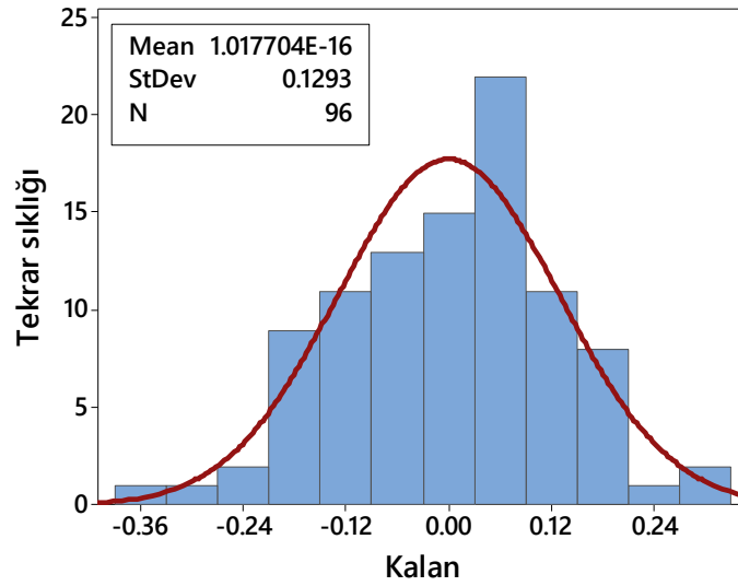
Şekil 4.116. RI sonuçları için geliştirilen modeldeki hataların histogram grafiği (Büyük ölçekli DKK)
