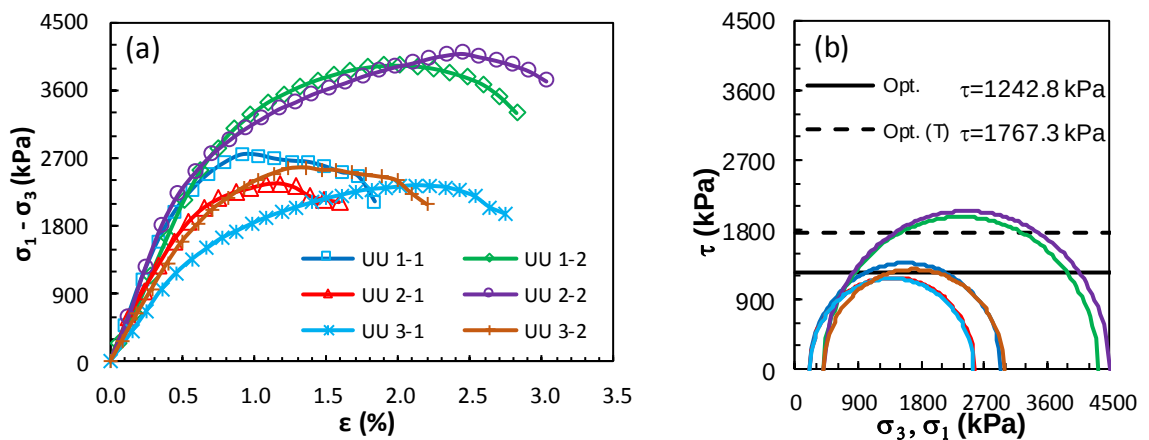
Şekil 4.84. Optimum tasarıma ait UU deney sonuçları: a) deviator gerilme-birim boy kısalması grafikleri, b) Mohr daireleri ile kırılma zarfları (Büyük ölçekli DKK, UU, 28 gün)
