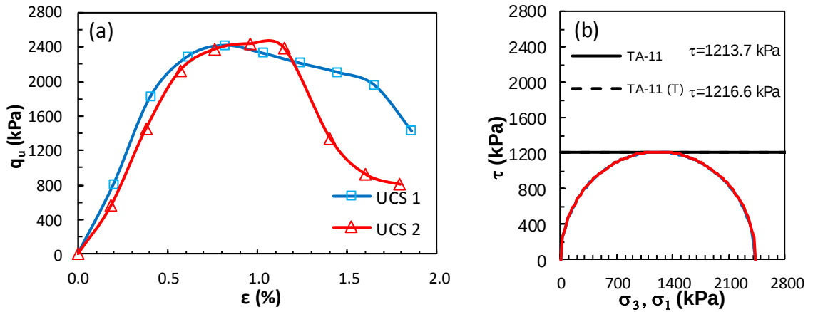
Şekil Ek 5.27. KÖ-11 numaralı tasarım: a) gerilme-birim deformasyon grafikleri ve b) Mohr daireleri (Küçük ölçekli DKK, UCS, 28 gün)
