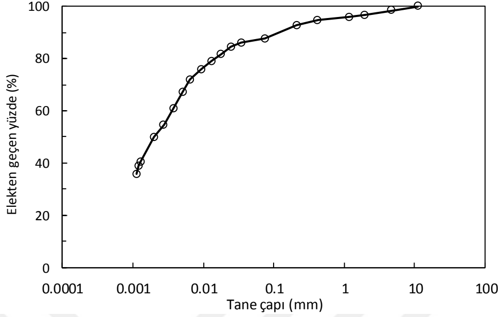
Şekil 3.4. Zeminin tane dağılımı
