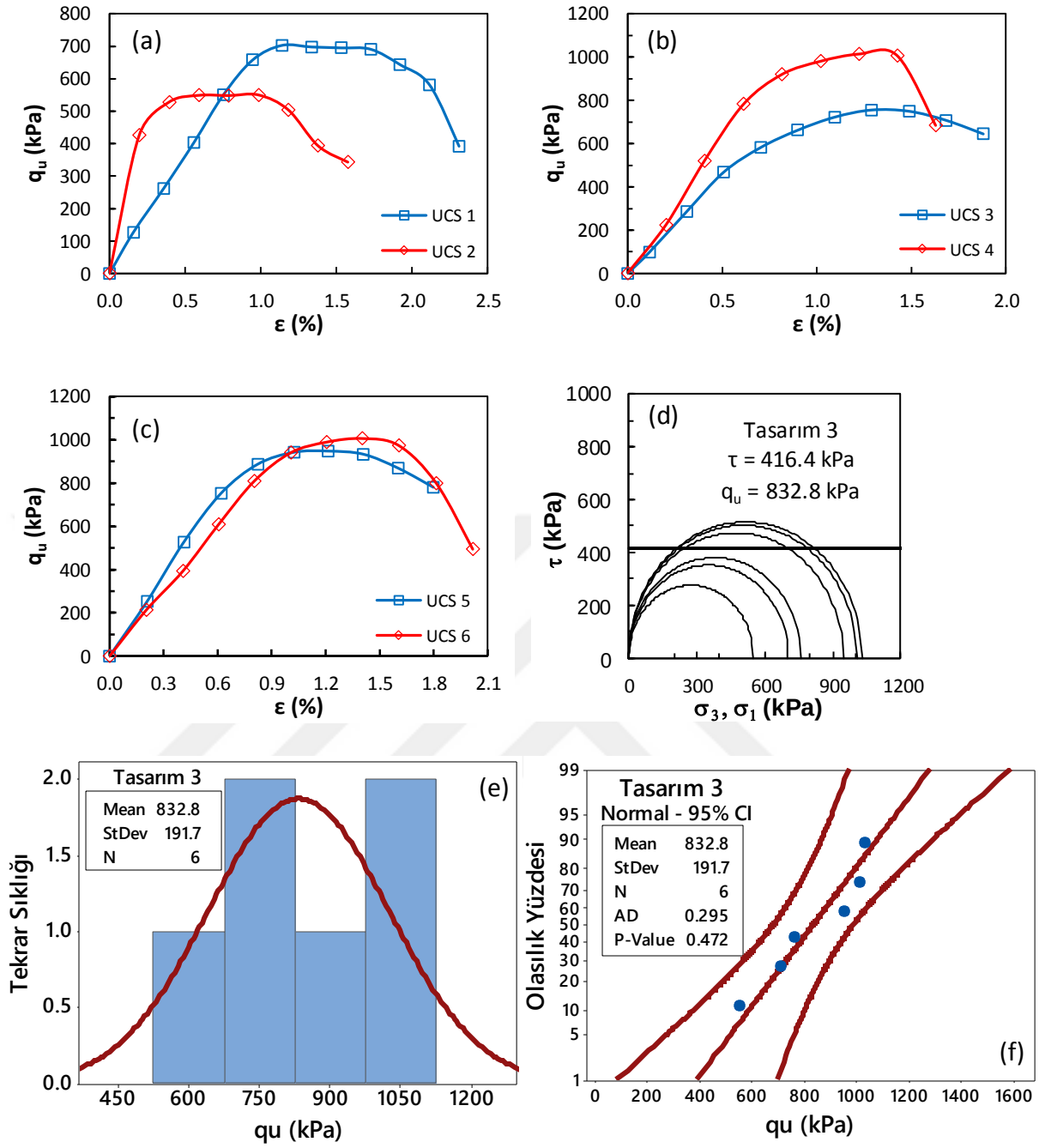
Şekil Ek 1.3. SP-3 numaralı kolona ait gerilme-birim deformasyon grafikleri: a) kolon alt bölgesi, b) kolon orta bölgesi, c) kolon üst bölgesi ve d) Mohr daireleri, e) histogram grafiği, f) olasılık grafiği (Sistem parametreleri, UCS, 28 gün)
