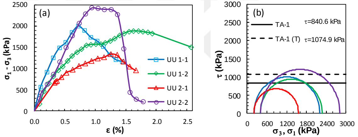
Şekil Ek 3.17. BÖ-1 numaralı kolona ait UU deney sonuçları: a) deviatör gerilme-birim boy kısalması grafikleri, b) Mohr daireleri ile kırılma zarfları (Büyük ölçekli DKK, UU, 56 gün)
