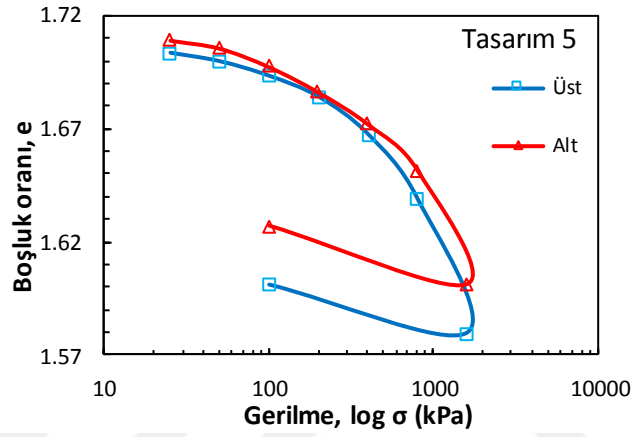
Şekil Ek 4.5. BÖ-5 numaralı kolona ait konsolidasyon deney sonucu (Büyük ölçekli DKK, 28 gün)
