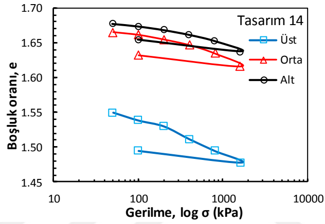
Şekil Ek 4.14. BÖ-14 numaralı kolona ait konsolidasyon deney sonucu (Büyük ölçekli DKK, 28 gün)
