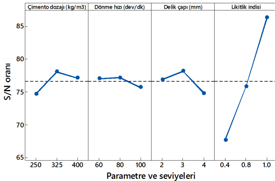
Şekil 4.13. Zemin iyileştirme derecesi için elde edilen S/N grafiği (Sistem parametrelerinin araştırılması)
