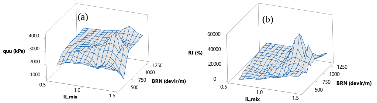
Şekil 4.38. BRN ve I_{L,mix} ile a) q_{uu} ve b) RI arasındaki ilişki (Büyük ölçekli DKK, UU, 56 gün)
