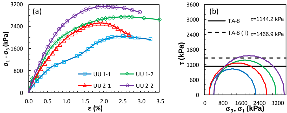
Şekil Ek 3.24. BÖ-8 numaralı kolona ait UU deney sonuçları: a) deviatör gerilme-birim boy kısalması grafikleri, b) Mohr daireleri ile kırılma zarfları (Büyük ölçekli DKK, UU, 56 gün)
