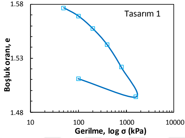
Şekil Ek 4.1. BÖ-1 numaralı kolona ait konsolidasyon deney sonucu (Büyük ölçekli DKK, 28 gün)
