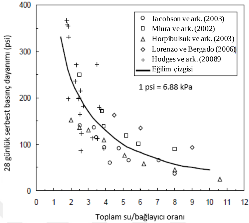
Şekil 2.12. Karışımın toplam su/bağlayıcı oranı ile dayanım arasındaki ilişki (FHWA, 2013'den değiştirilerek)
