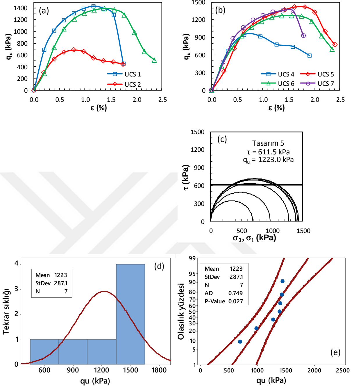
Şekil Ek 2.5. BÖ-5 numaralı kolona ait gerilme-birim deformasyon grafikleri: a) kolon üst bölgesi, b) kolon alt bölgesi ve c) Mohr daireleri, d) histogram grafiği, e) olasılık grafiği (Büyük ölçekli DKK, UCS, 28 gün)
