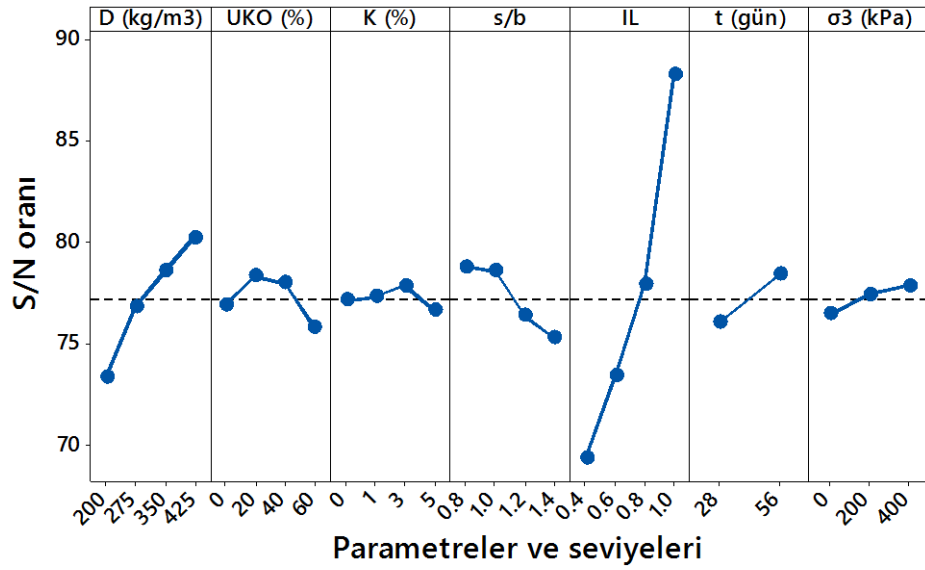
Şekil 4.112. RI için elde edilen S/N grafiği (Büyük ölçekli DKK)
