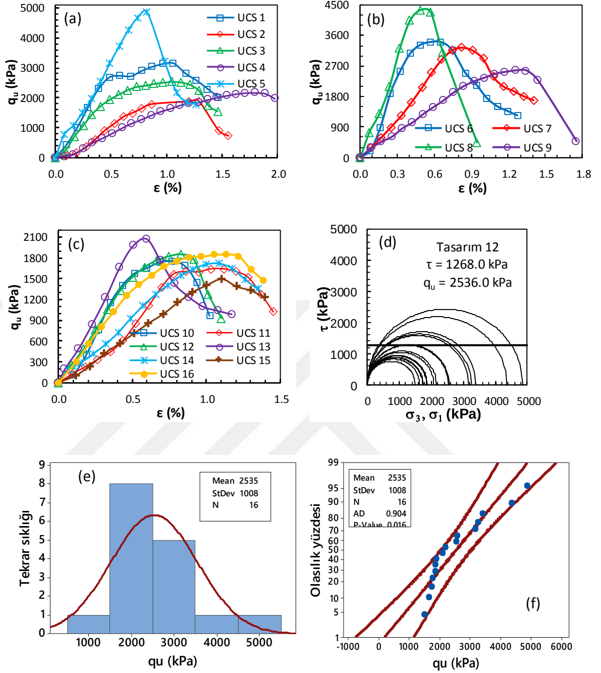
Şekil Ek 2.28. BÖ-12 numaralı kolona ait gerilme-birim deformasyon grafikleri: a) kolon üst bölgesi, b) kolon orta bölgesi, c) kolon alt bölgesi ve d) Mohr daireleri, e) histogram grafiği, f) olasılık grafiği (Büyük ölçekli DKK, UCS, 56 gün)
