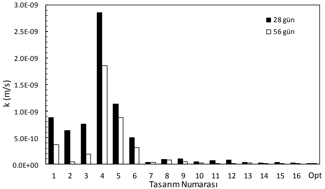
Şekil 4.46. Permeabilite deney sonuçları (Büyük ölçekli DKK)
