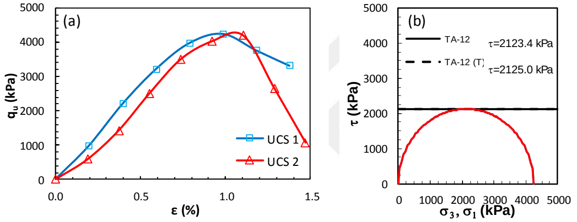
Şekil Ek 5.44. KÖ-12 numaralı tasarım: a) gerilme-birim deformasyon grafikleri ve b) Mohr daireleri (Küçük ölçekli DKK, UCS, 56 gün)
