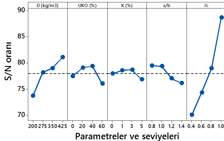
Şekil 4.22. Zemin iyileştirme derecesi için elde edilen S/N grafiği (Büyük ölçekli DKK, UCS, 56 gün)
