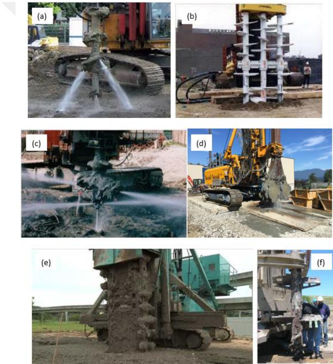
Şekil 2.9. Farklı derin karıştırma yöntemleri için kullanılan karıştırma ekipmanları: a, b) WRS ekipmanı, c) WJE ekipmanı, d) CSM ekipmanı, e) TRD ekipmanı, f) WRE ekipmanı
