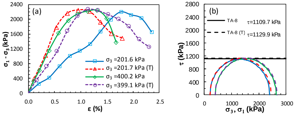
Şekil Ek 6.24. KÖ-8 numaralı tasarım: a) deviator gerilme-birim deformasyon grafikleri ve b) Mohr daireleri (Küçük ölçekli DKK, UU, 28 gün)
