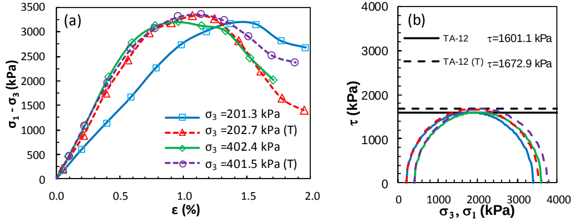
Şekil Ek 6.28. KÖ-12 numaralı tasarım: a) deviator gerilme-birim deformasyon grafikleri ve b) Mohr daireleri (Küçük ölçekli DKK, UU, 28 gün)
