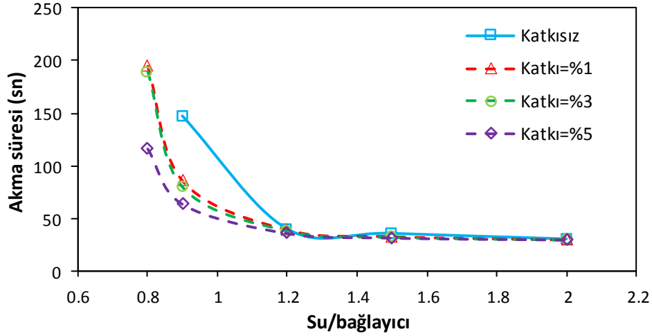
Şekil 3.46. Optima 100 katkısı ile farklı su/bağlayıcı oranlarına sahip enjeksiyonların marsh hunisi deneyi sonuçları (UKO=%60)
