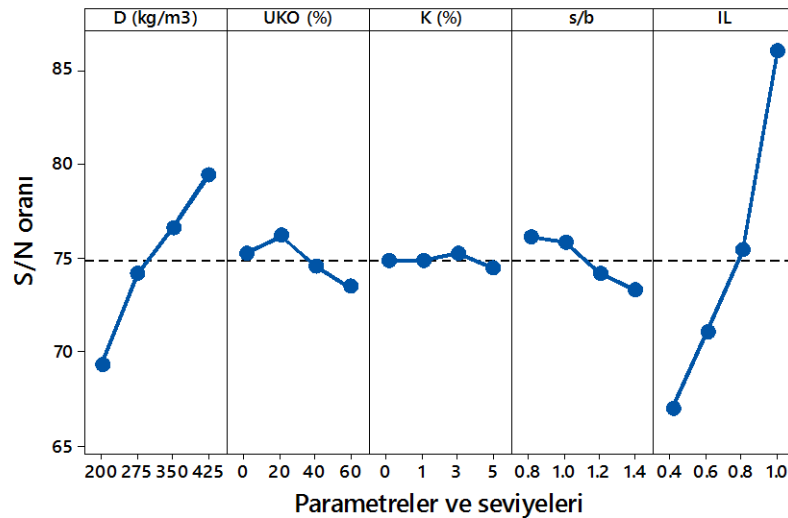
Şekil 4.20. Zemin iyileştirme derecesi için elde edilen S/N grafiği (Büyük ölçekli DKK, UCS, 28 gün)
