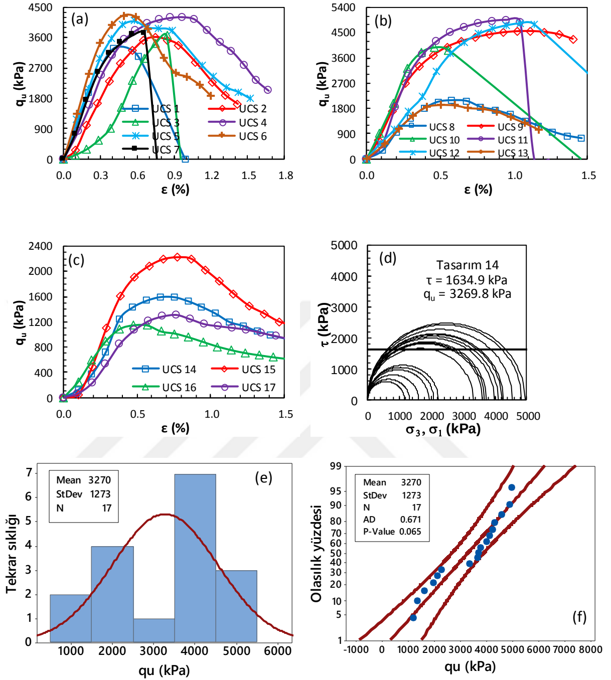
Şekil Ek 2.14. BÖ-14 numaralı kolona ait gerilme-birim deformasyon grafikleri: a) kolon üst bölgesi, b) kolon orta bölgesi, c) kolon alt bölgesi ve d) Mohr daireleri, e) histogram grafiği, f) olasılık grafiği (Büyük ölçekli DKK, UCS, 28 gün)
