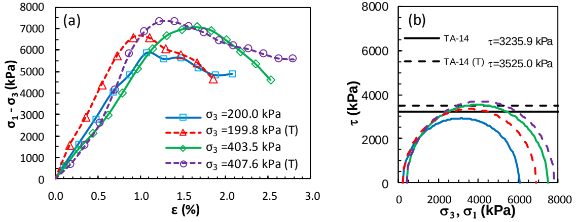
Şekil Ek 6.46. KÖ-14 numaralı tasarım: a) deviator gerilme-birim deformasyon grafikleri ve b) Mohr daireleri (Küçük ölçekli DKK, UU, 56 gün)
