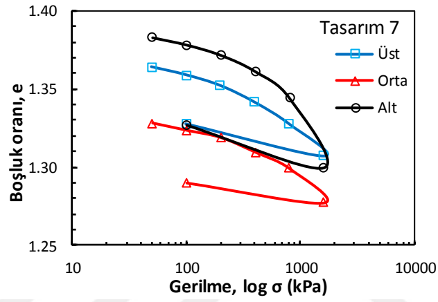
Şekil Ek 4.23. BÖ-7 numaralı kolona ait konsolidasyon deney sonucu (Büyük ölçekli DKK, 56 gün)
