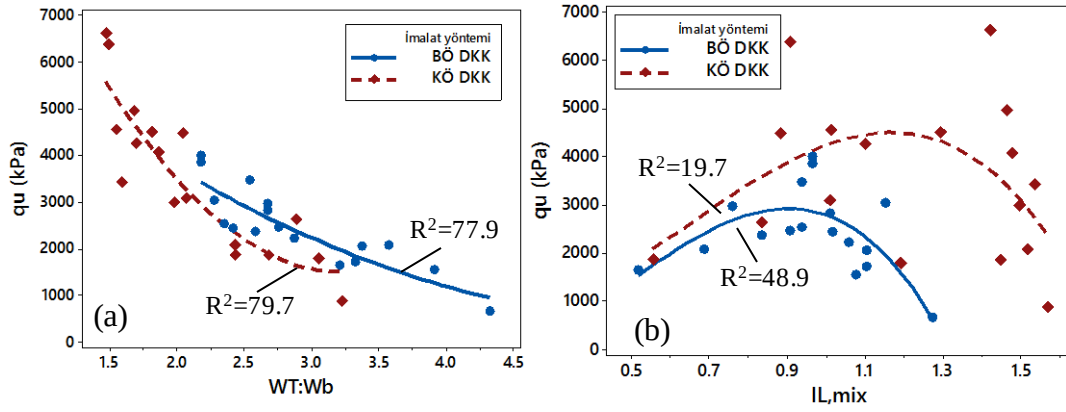
Şekil 4.97. Serbest basınç dayanımının a) W_T:W_b ve b) I_{L,mix} ile ilişkileri (Küçük ve büyük ölçekli DKK, 56 gün)
