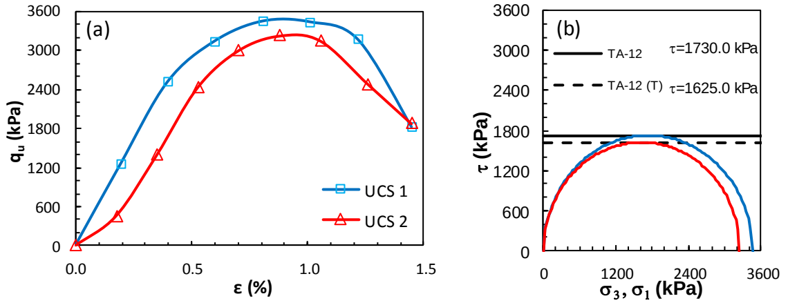
Şekil Ek 5.28. KÖ-12 numaralı tasarım: a) gerilme-birim deformasyon grafikleri ve b) Mohr daireleri (Küçük ölçekli DKK, UCS, 28 gün)
