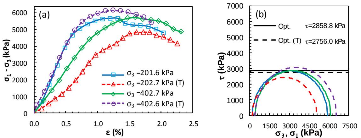
Şekil 4.93. Optimum tasarıma ait UU deney sonuçları: a) deviatör gerilme-birim boy kısalması grafikleri, b) Mohr daireleri ile kırılma zarfları (Küçük ölçekli DKK, UU, 28 gün)
