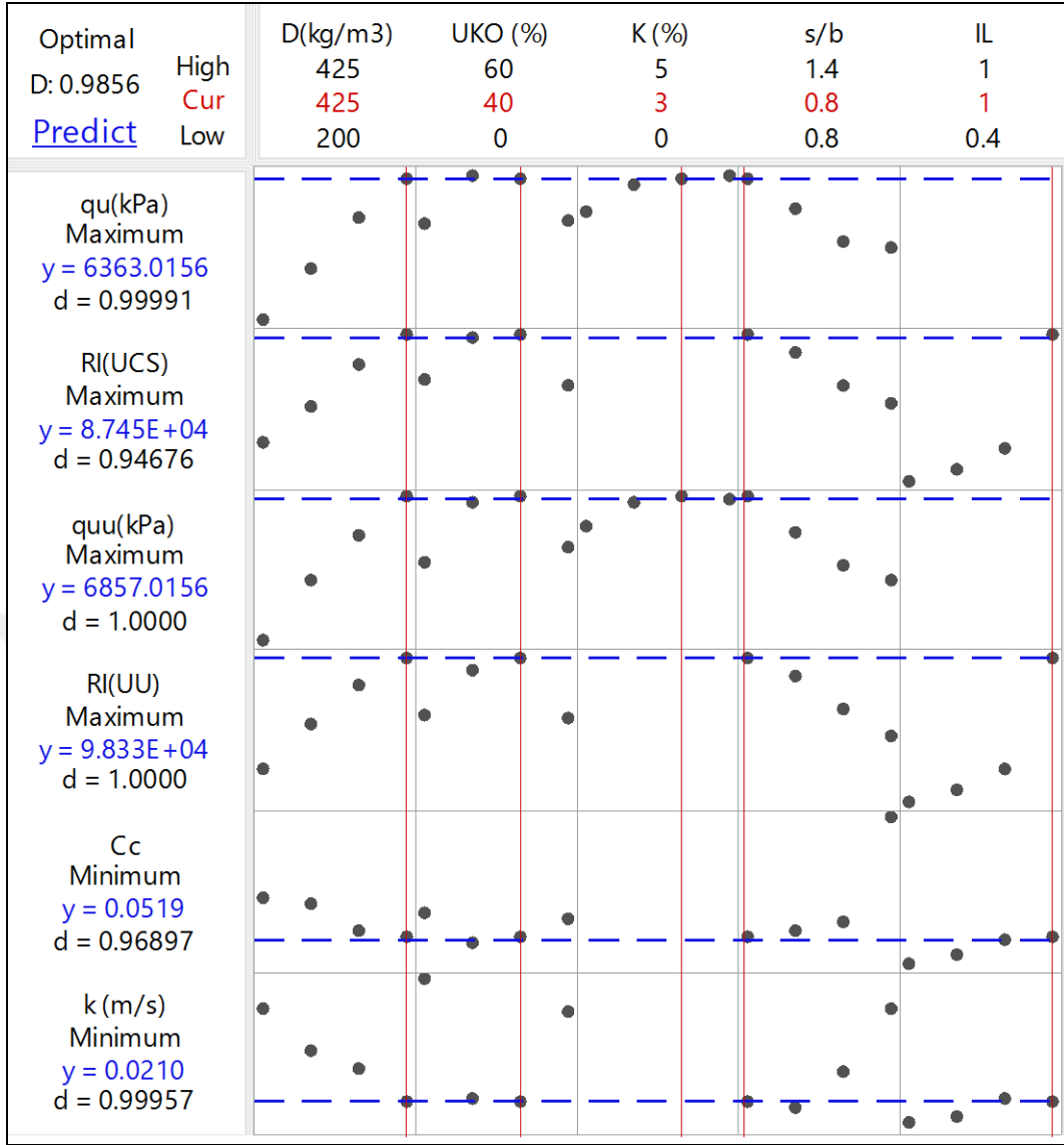
Şekil 4.88. Optimizasyon grafiği (Küçük ölçekli DKK, 56 gün) Not: k değeri 10^{-9} ile çarpılmalıdır.
