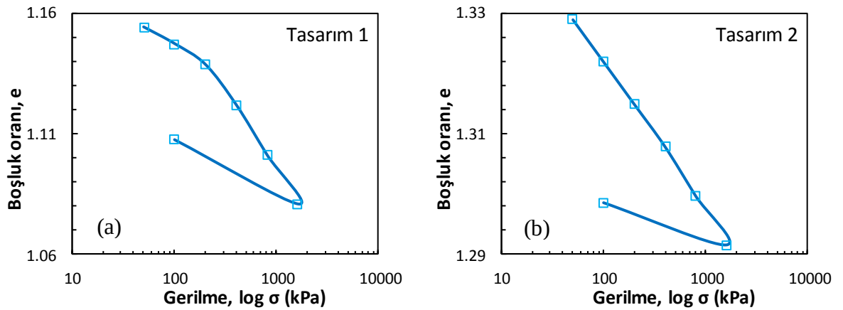
Şekil Ek 7.9. Küçük ölçekli DKK, konsolidasyon deneyi, 56 gün: a) Tasarım 1 ve b) Tasarım 2
