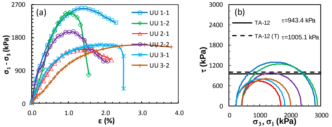
Şekil Ek 3.12. BÖ-12 numaralı kolona ait UU deney sonuçları: a) deviator gerilme-birim boy kısalması grafikleri, b) Mohr daireleri ile kırılma zarfları (Büyük ölçekli DKK, UU, 28 gün)
