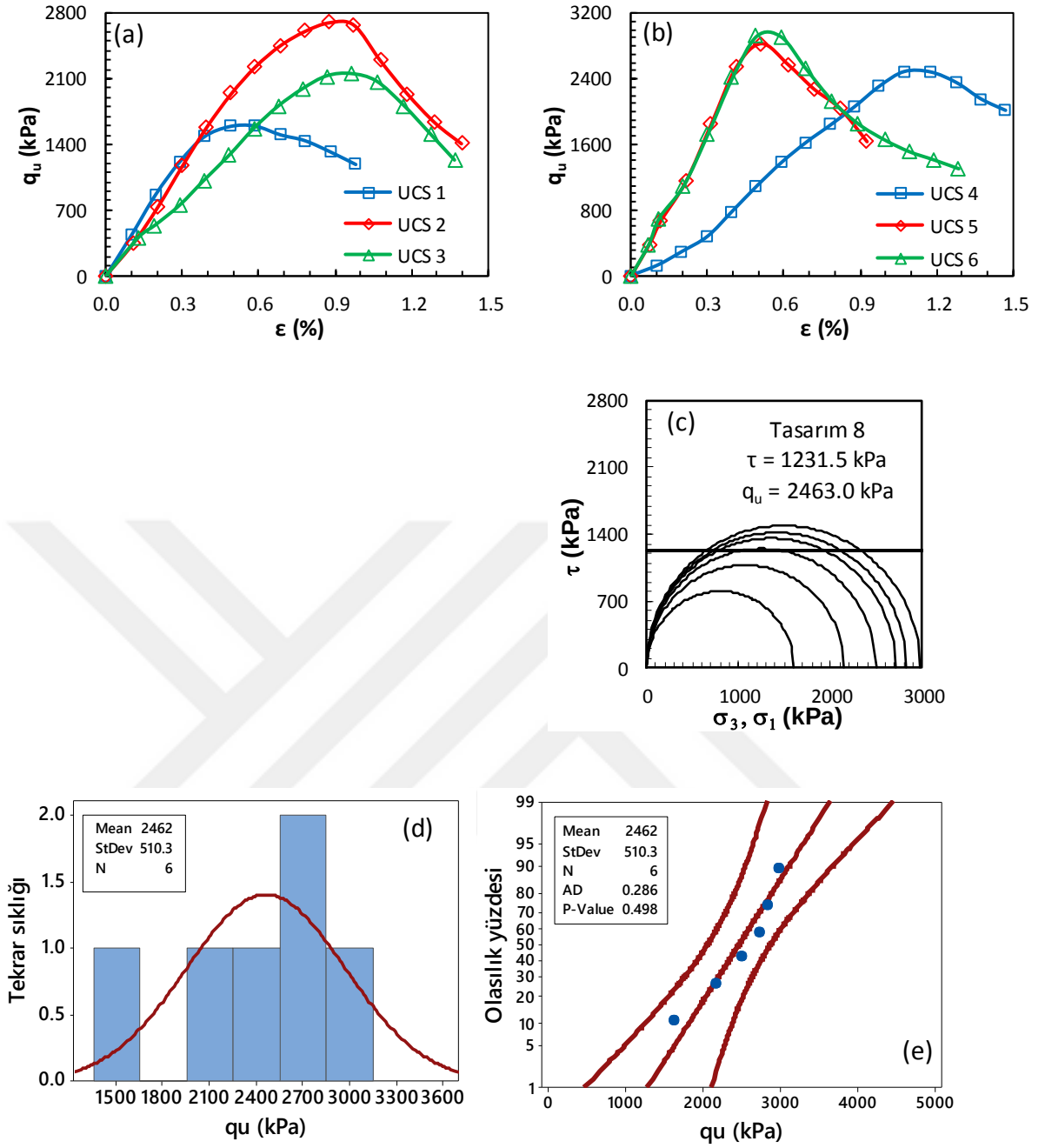
Şekil Ek 2.24. BÖ-8 numaralı kolona ait gerilme-birim deformasyon grafikleri: a) kolon üst bölgesi, b) kolon alt bölgesi ve c) Mohr daireleri, d) histogram grafiği, e) olasılık grafiği (Büyük ölçekli DKK, UCS, 56 gün)
