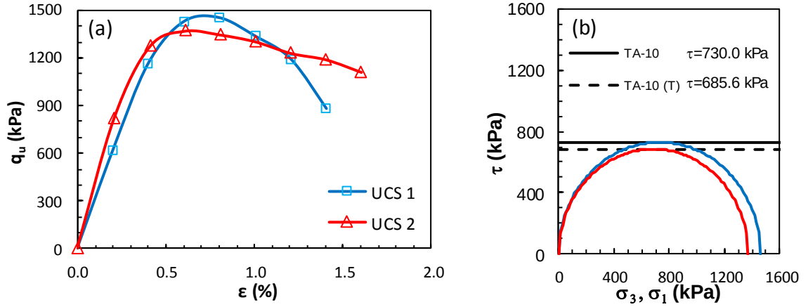
Şekil Ek 5.10. KÖ-10 numaralı tasarım: a) gerilme-birim deformasyon grafikleri ve b) Mohr daireleri (Küçük ölçekli DKK UCS, 7 gün)
