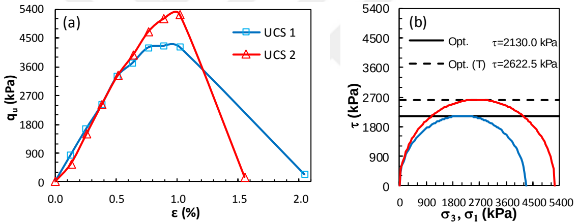
Şekil 4.91. Optimum tasarıma ait a) gerilme-birim deformasyon grafikleri ve b) Mohr daireleri (Küçük ölçekli DKK, UCS, 28 gün)
