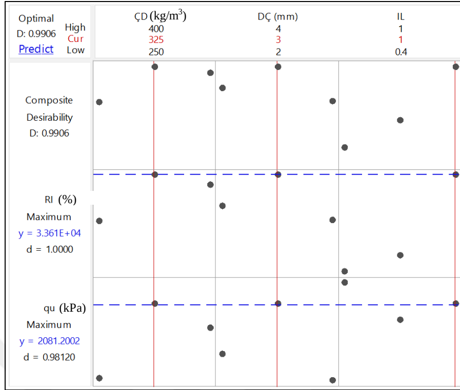
Şekil 4.15. ANOVA sonuçlarına göre elde edilen optimizasyon sonuçları (Sistem parametrelerinin araştırılması)
