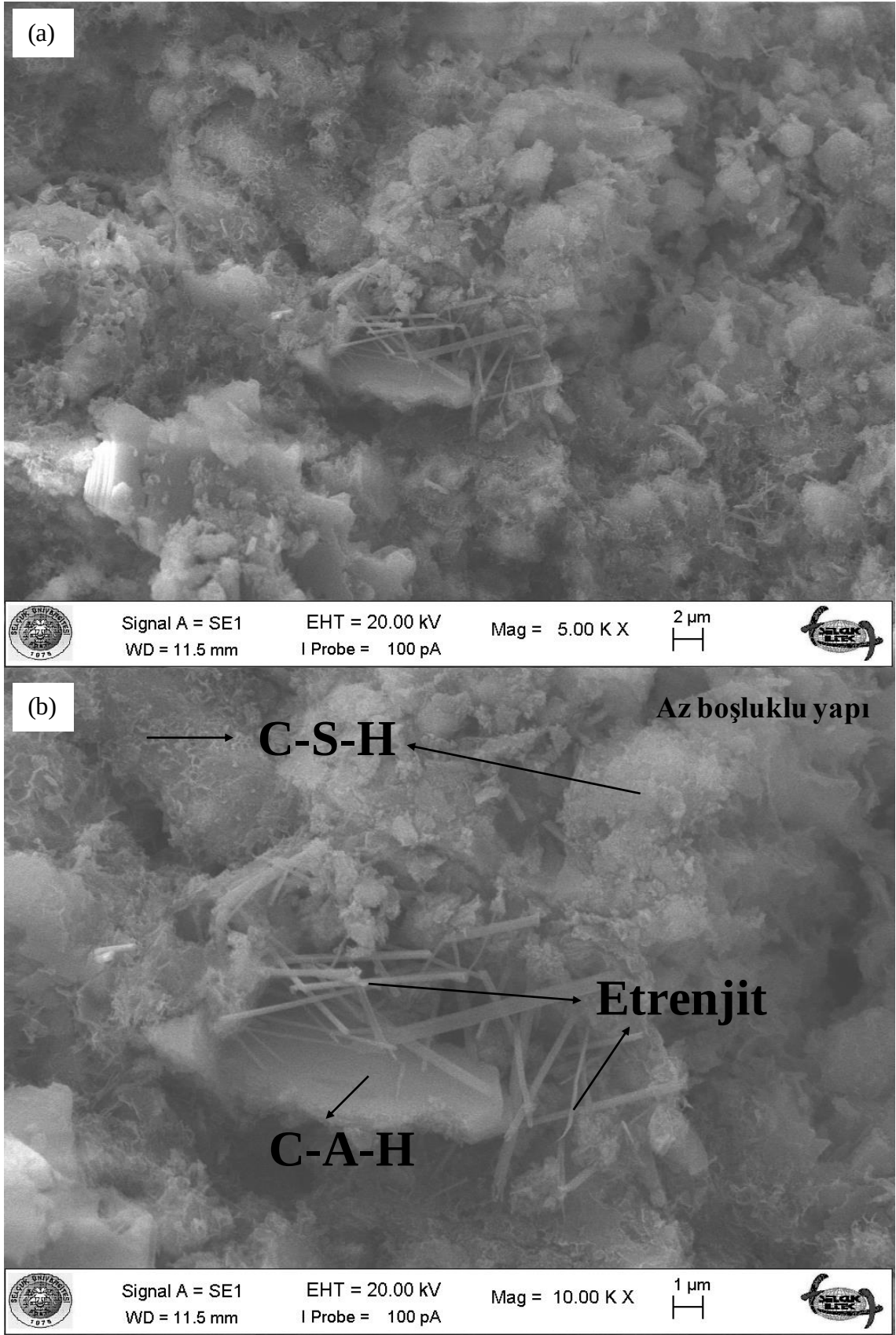
Şekil 4.138. Tasarım 14'e ait SEM görüntüleri: a) x5000, b) x10000 (Büyük ölçekli DKK, 56 gün)
