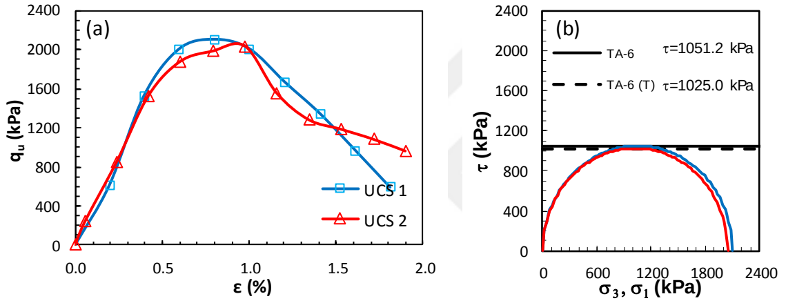
Şekil Ek 5.38. KÖ-6 numaralı tasarım: a) gerilme-birim deformasyon grafikleri ve b) Mohr daireleri (Küçük ölçekli DKK, UCS, 56 gün)
