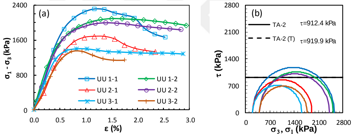
Şekil Ek 3.2. BÖ-2 numaralı kolona ait UU deney sonuçları: a) deviator gerilme-birim boy kısalması grafikleri, b) Mohr daireleri ile kırılma zarfları (Büyük ölçekli DKK, UU, 28 gün)
