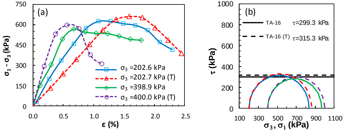
Şekil Ek 6.16. KÖ-16 numaralı tasarım: a) deviator gerilme-birim deformasyon grafikleri ve b) Mohr daireleri (Küçük ölçekli DKK, UU, 7 gün)
