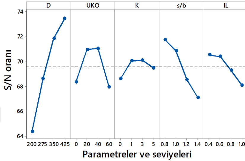
Şekil 4.53. Serbest basınç dayanımı için elde edilen S/N grafiği (Küçük ölçekli DKK, UCS, 56 gün)
