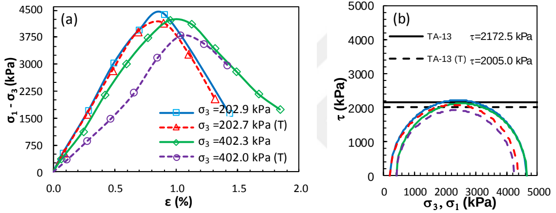
Şekil Ek 6.29. KÖ-13 numaralı tasarım: a) deviator gerilme-birim deformasyon grafikleri ve b) Mohr daireleri (Küçük ölçekli DKK, UU, 28 gün)
