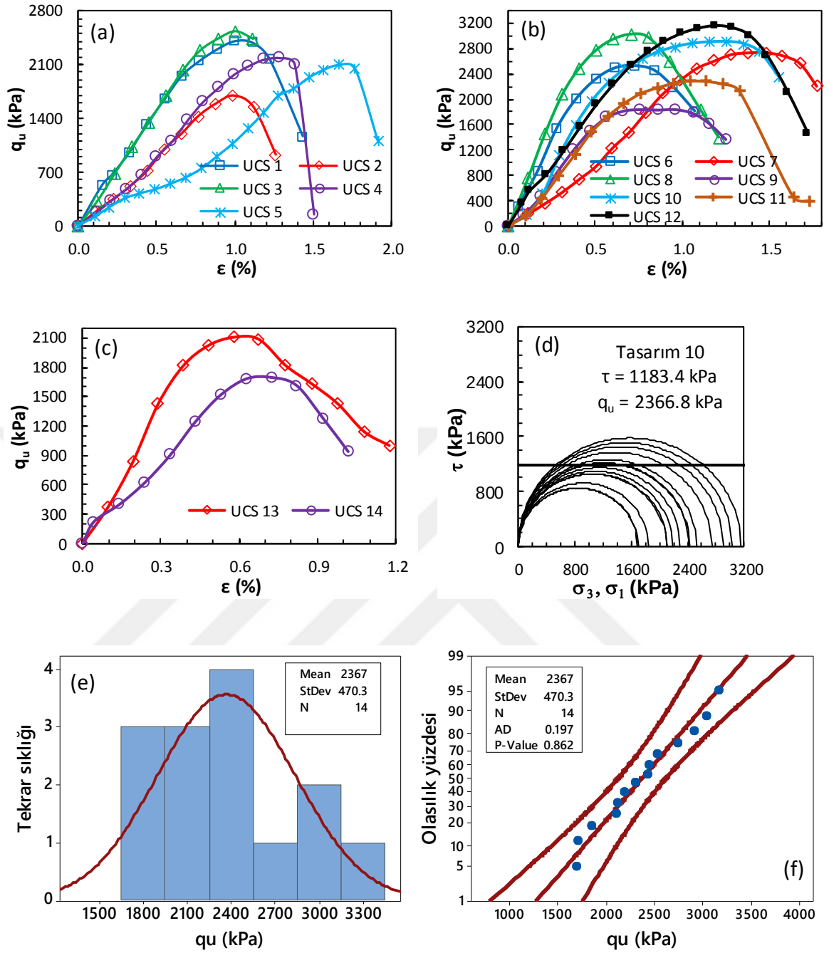
Şekil Ek 2.26. BÖ-10 numaralı kolona ait gerilme-birim deformasyon grafikleri: a) kolon üst bölgesi, b) kolon orta bölgesi, c) kolon alt bölgesi ve d) Mohr daireleri, e) histogram grafiği, f) olasılık grafiği (Büyük ölçekli DKK, UCS, 56 gün)
