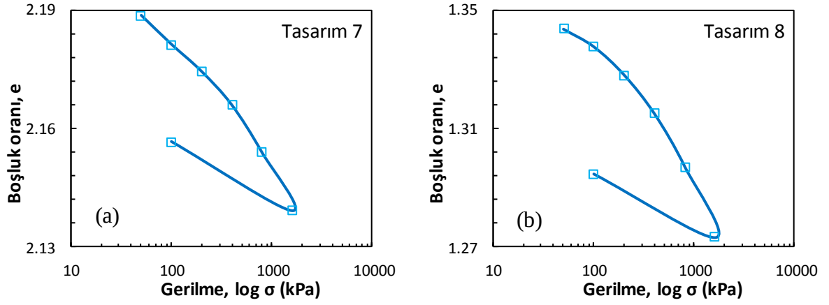
Şekil Ek 7.4. Küçük ölçekli DKK, konsolidasyon deneyi, 28 gün: a) Tasarım 7 ve b) Tasarım 8
