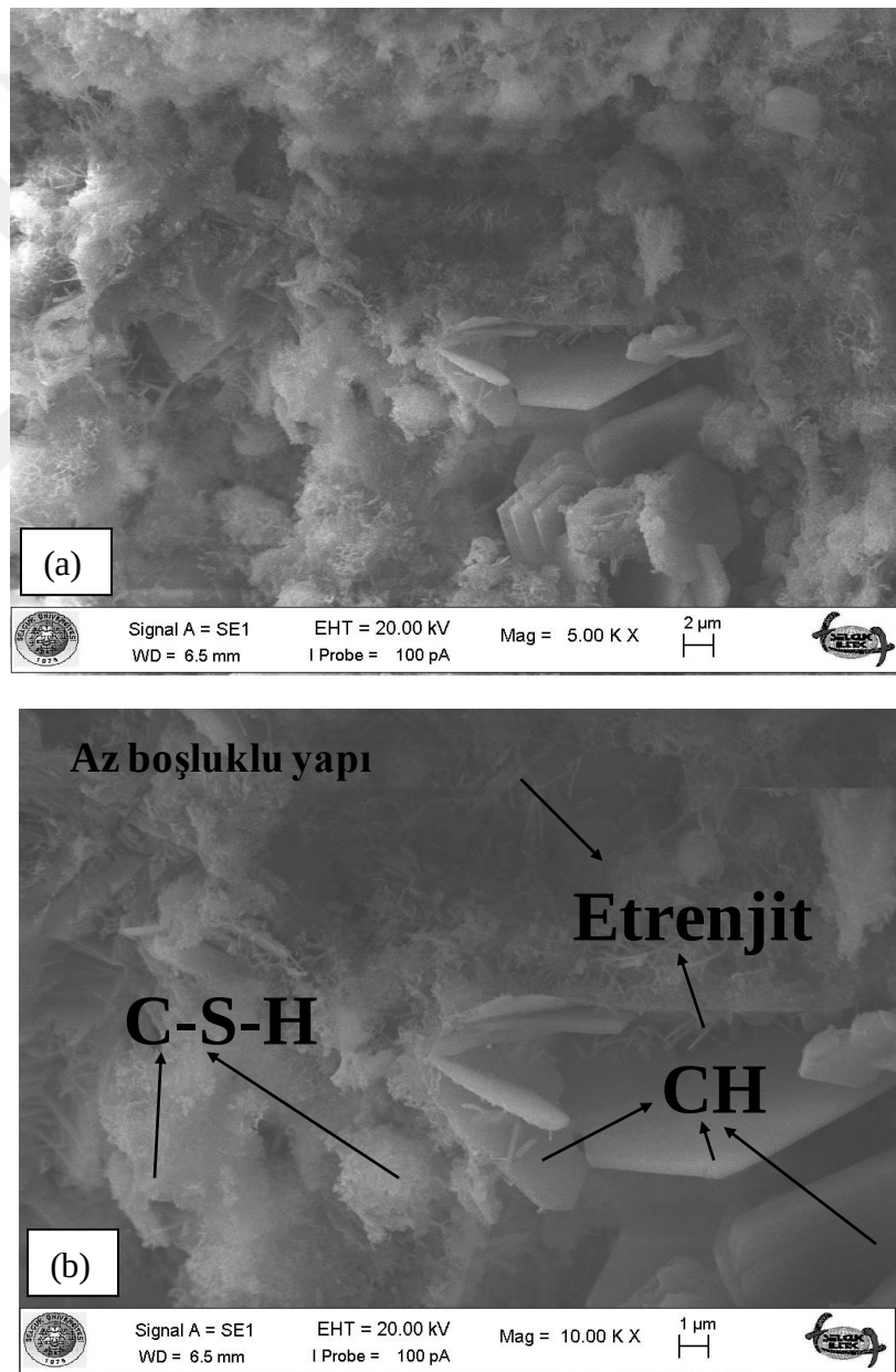
Şekil 4.125. Tasarım 14'e ait SEM görüntüleri: a) x5000, b) x10000 (Küçük ölçekli DKK, 28 gün)
