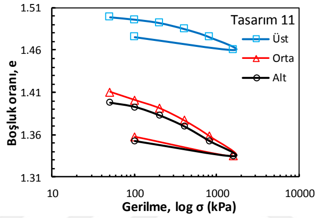
Şekil Ek 4.11. BÖ-11 numaralı kolona ait konsolidasyon deney sonucu (Büyük ölçekli DKK, 28 gün)
