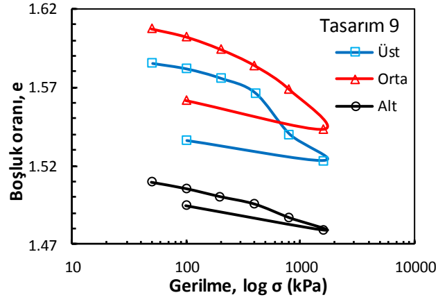
Şekil Ek 4.25. BÖ-9 numaralı kolona ait konsolidasyon deney sonucu (Büyük ölçekli DKK, 56 gün)
