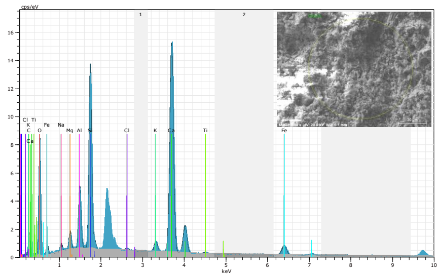
Şekil 4.131. Tasarım 14'e ait EDX analizi sonucu (Küçük ölçekli DKK, 28 gün)
