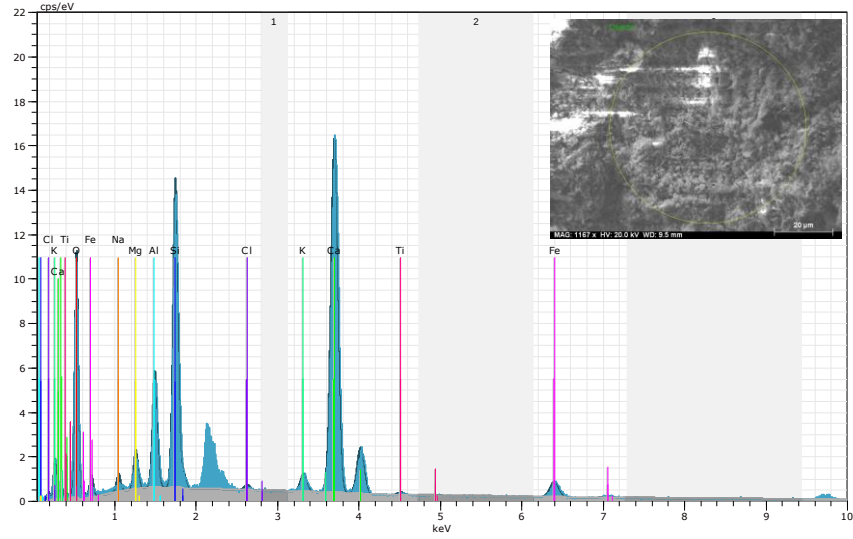
Şekil 4.132. Tasarım 14'e ait EDX analizi sonucu (Küçük ölçekli DKK, 56 gün)
