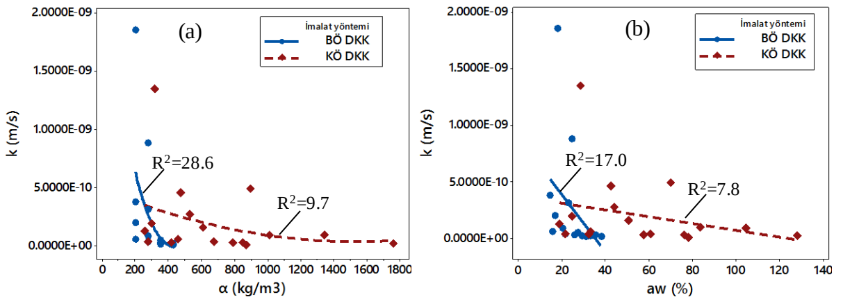
Şekil 4.102. Permeabilite katsayısının a) \alpha ve b) a_w ile ilişkileri (Küçük ve büyük ölçekli DKK, 56 gün)
