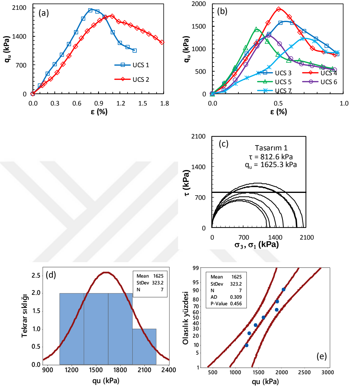
Şekil Ek 2.17. BÖ-1 numaralı kolona ait gerilme-birim deformasyon grafikleri: a) kolon üst bölgesi, b) kolon alt bölgesi ve c) Mohr daireleri, d) histogram grafiği, e) olasılık grafiği (Büyük ölçekli DKK, UCS, 56 gün)
