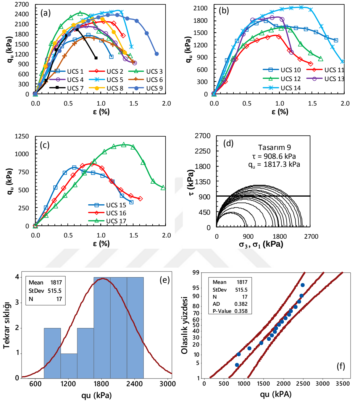
Şekil Ek 2.9. BÖ-9 numaralı kolona ait gerilme-birim deformasyon grafikleri: a) kolon üst bölgesi, b) kolon orta bölgesi, c) kolon alt bölgesi ve d) Mohr daireleri, e) histogram grafiği, f) olasılık grafiği (Büyük ölçekli DKK, UCS, 28 gün)
