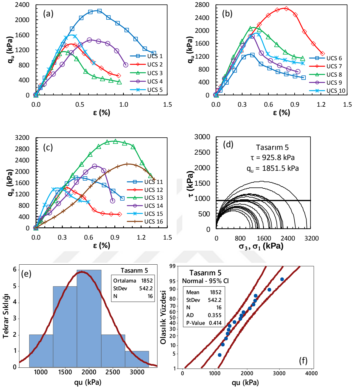
Şekil Ek 1.5. SP-5 numaralı kolona ait gerilme-birim deformasyon grafikleri: a) kolon alt bölgesi, b) kolon orta bölgesi, c) kolon üst bölgesi ve d) Mohr daireleri, e) histogram grafiği, f) olasılık grafiği (Sistem parametreleri, UCS, 28 gün)
