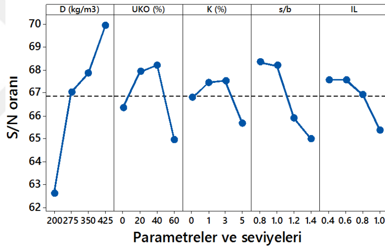
Şekil 4.21. Kolon dayanımı için elde edilen S/N grafiği (Büyük ölçekli DKK, UCS, 56 gün)
