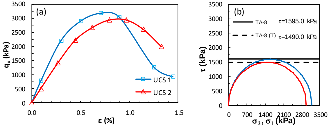
Şekil Ek 5.40. KÖ-8 numaralı tasarım: a) gerilme-birim deformasyon grafikleri ve b) Mohr daireleri (Küçük ölçekli DKK, UCS, 56 gün)
