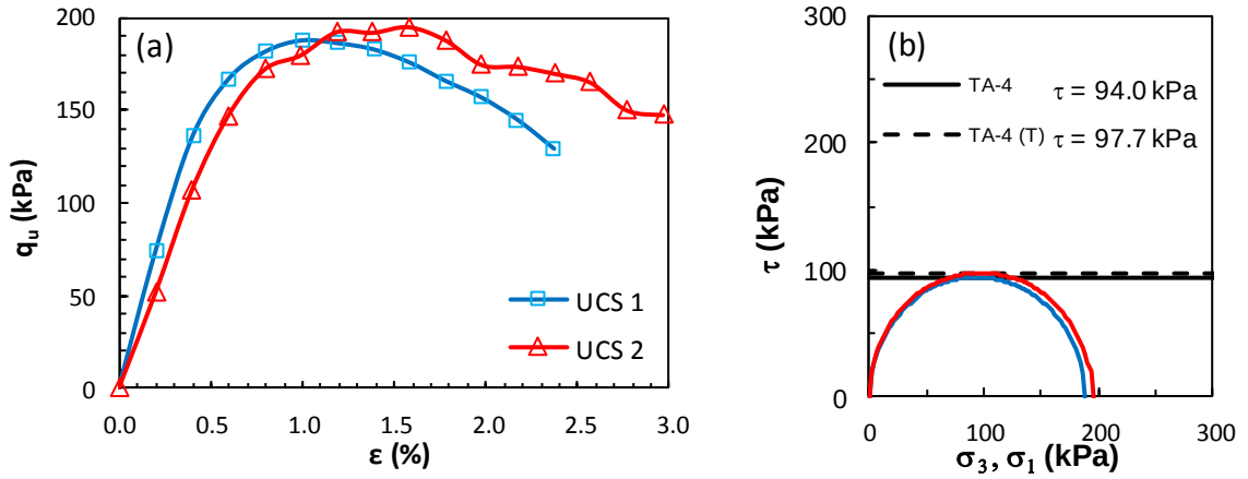
Şekil Ek 5.4. KÖ-4 numaralı tasarım: a) gerilme-birim deformasyon grafikleri ve b) Mohr daireleri (Küçük ölçekli DKK, UCS, 7 gün)
