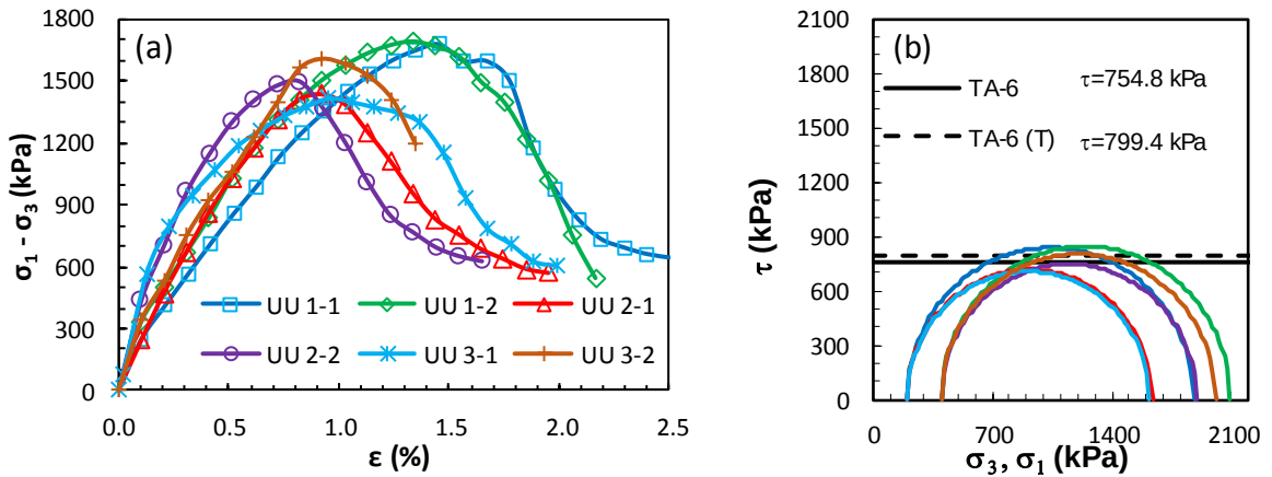
Şekil Ek 3.6. BÖ-6 numaralı kolona ait UU deney sonuçları: a) deviator gerilme-birim boy kısalması grafikleri, b) Mohr daireleri ile kırılma zarfları (Büyük ölçekli DKK, UU, 28 gün)
