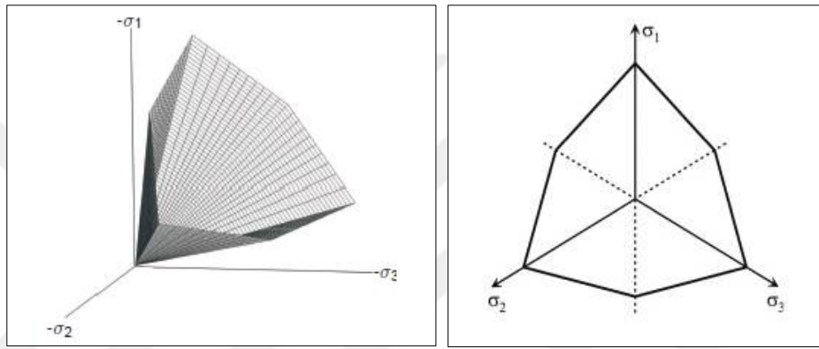
Şekil 3.11. Asal gerilme uzayında Mohr- Coulomb akma yüzeyleri( c=0 ) (PLAXİS).
