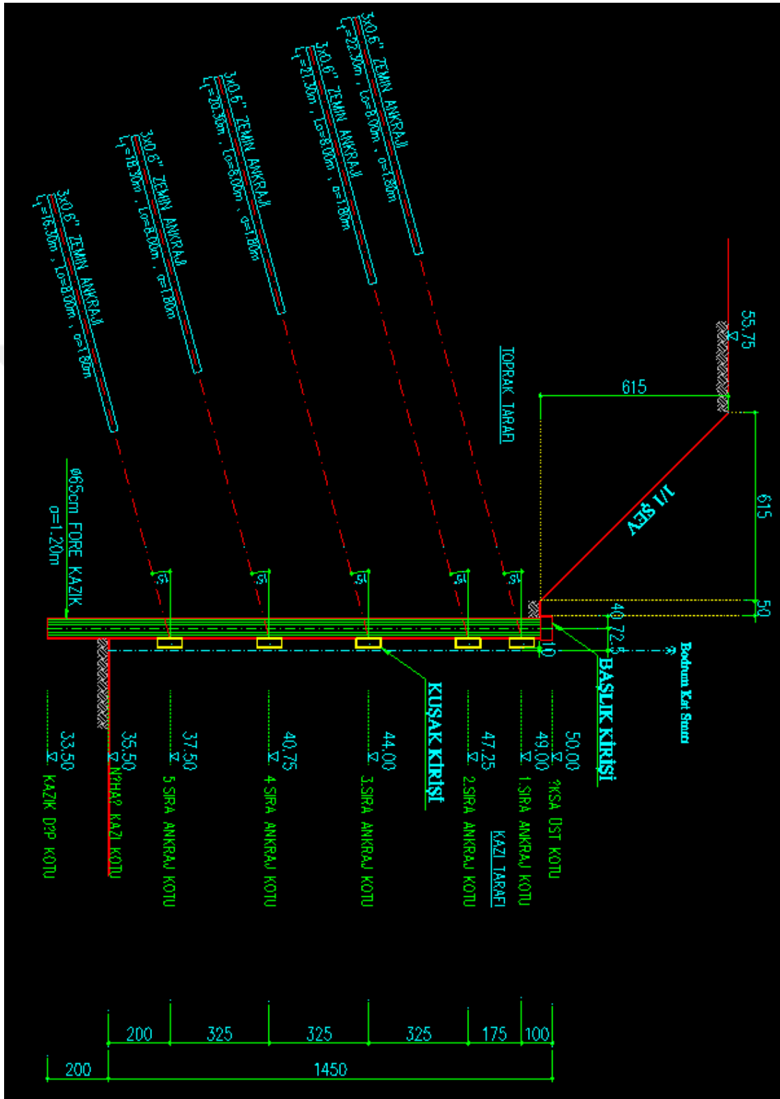
Ek-6: Uygulama-3 İksa Kesiti
