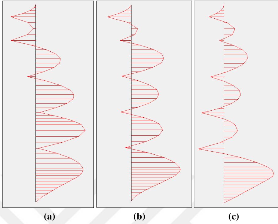
Şekil 4.22. MC(a), HS(b), HS_ss(c) moment diyagramları.
