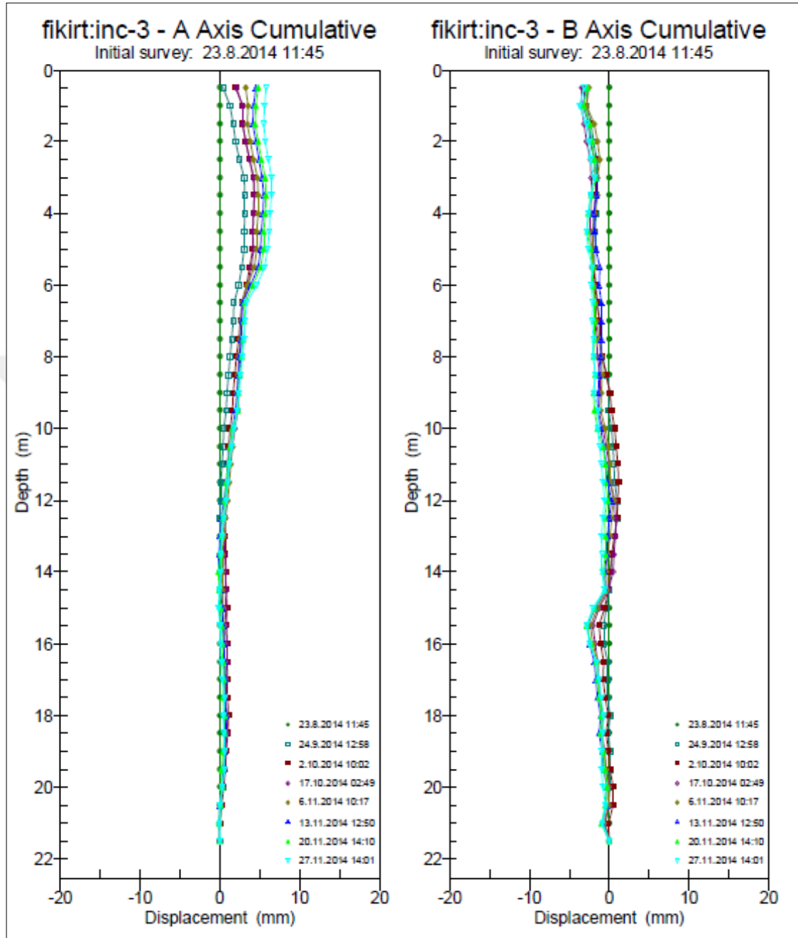
Ek-3: Uygulama-3 İnklinometre Okumaları
