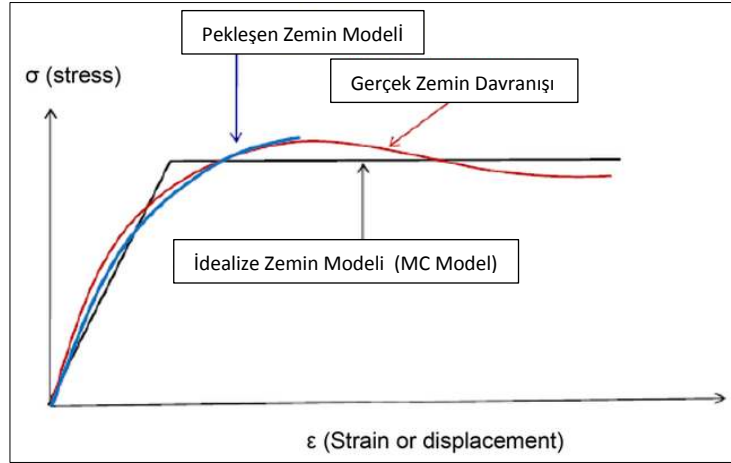
Şekil 3.12. Gerçek zemin ve model davranışları.
