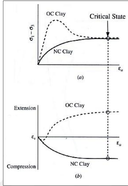
Şekil 3.14. OC(a) ve NC(b) kil davranışı (Bartlett, 2010).
