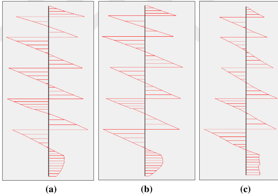
Şekil 4.23. MC(a), HS(b), HS_ss(c) kesme kuvveti diyagramları.
