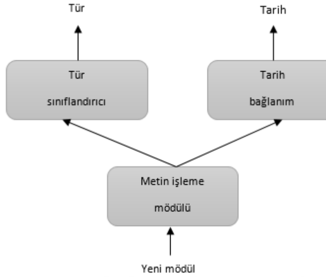
Şekil 3.14. Çoklu çıktı (ya da çok başlı) model
