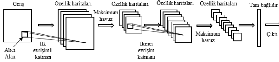
Şekil 2.5. İki evrişimli katmana sahip basit bir CNN mimarisi
