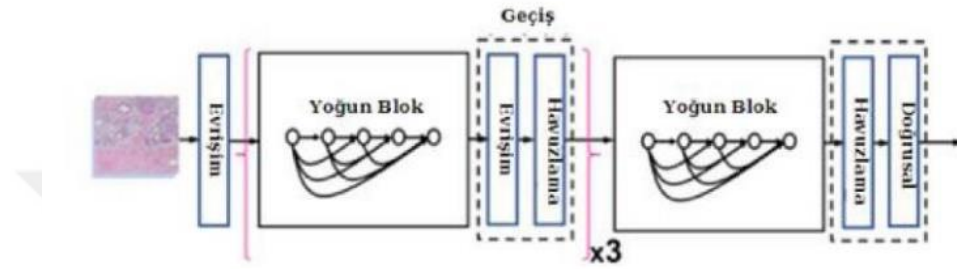
Şekil 3.7. DenseNet mimarisi (Li ve ark., 2020).
