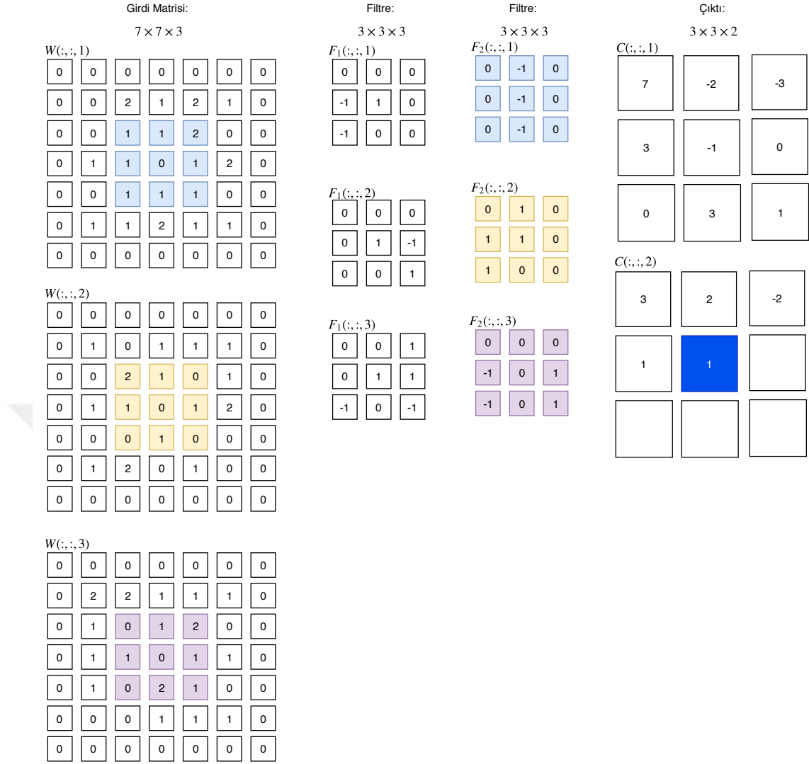
Şekil 2.27. Evrişim işlemi örneği, adım 3
