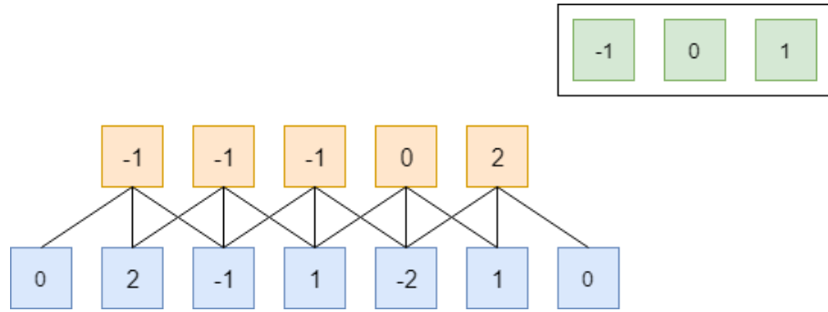
Şekil 2.22. Çıktı boyutu hesaplama örneği, kaydırma=1, sıfır ekleme=1
