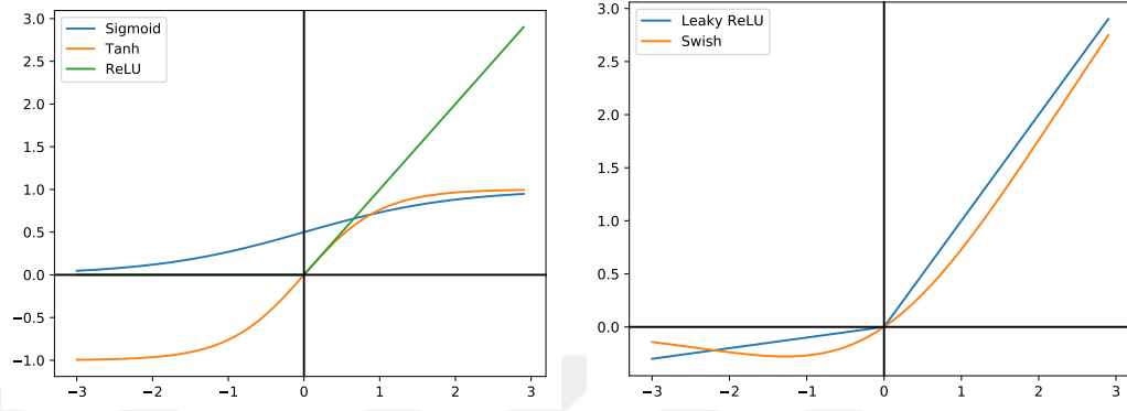
Şekil 2.4. Aktivasyon fonksiyonları (Kızrak, 2019)
