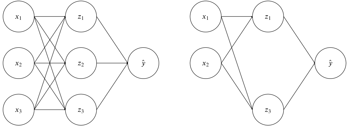
řekil 2.18. Seyreltme yntemi
