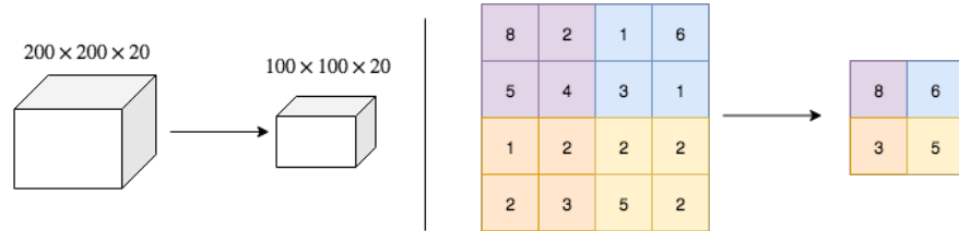
Şekil 2.28. Maksimum bölütleme (Max-Pooling)
