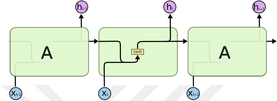
Şekil 3.5. RNN ağ yapısı [52]
