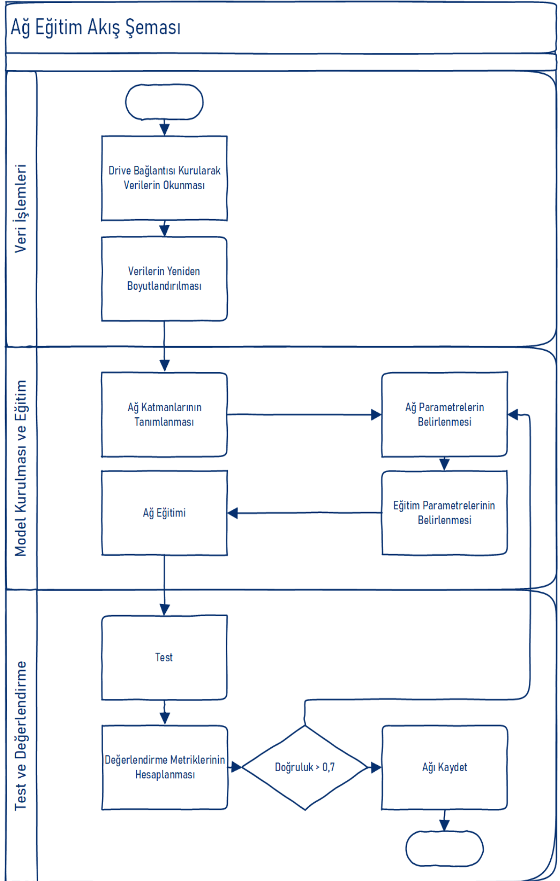
Şekil 4.1. Ağ eğitim akış şeması
