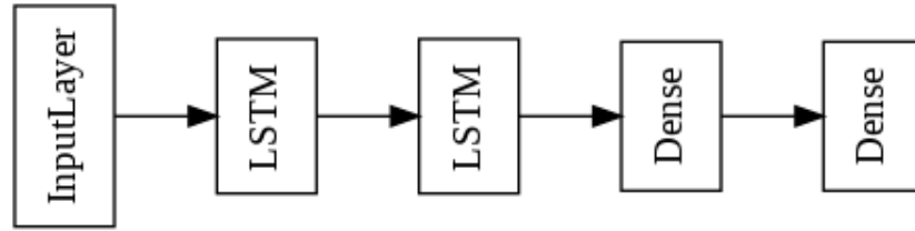
Şekil 4.4. Geliştirilen LSTM modelinin ağ katmanları
