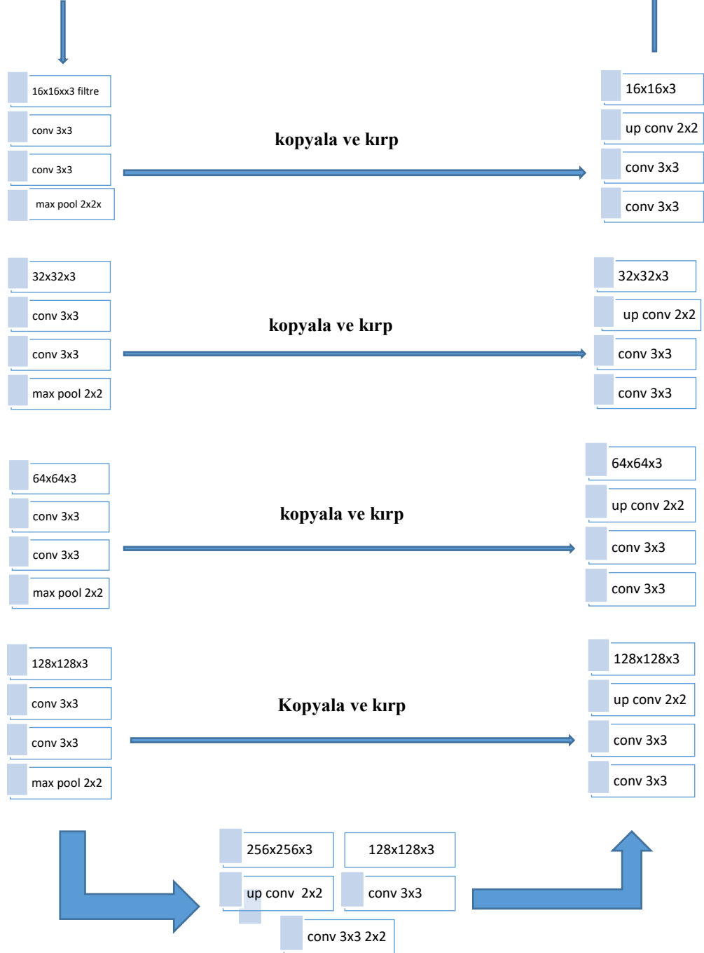
Şekil 3.9. U-Net modelinin akış şeması
