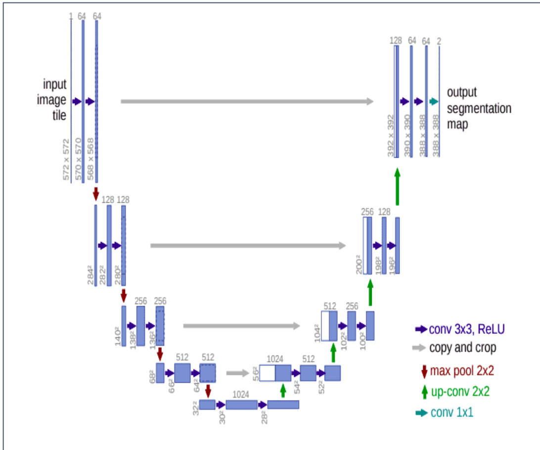
Şekil 1.17. U-Net mimarisi
