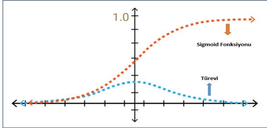
Şekil 1.8. Sigmoid fonksiyonu grafiği
