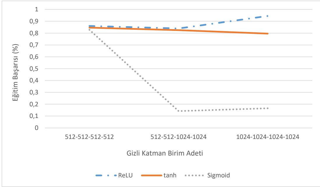
Şekil 4.6. Aktivasyon fonksiyonlarının eğitim başarıları
