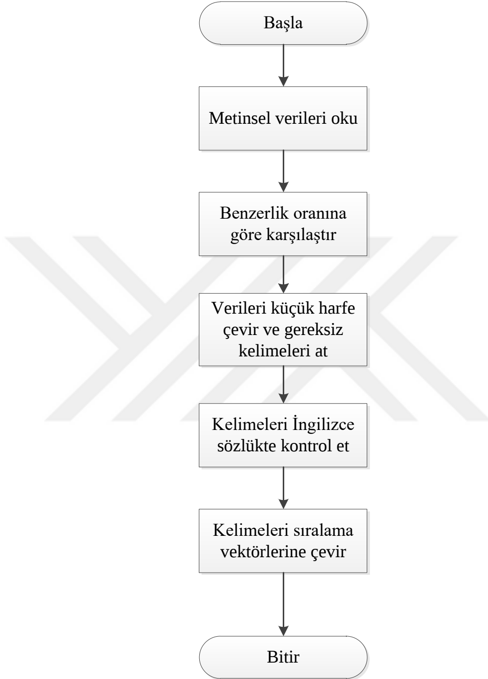
Şekil 4.3. LSTM için veri ön işleme
