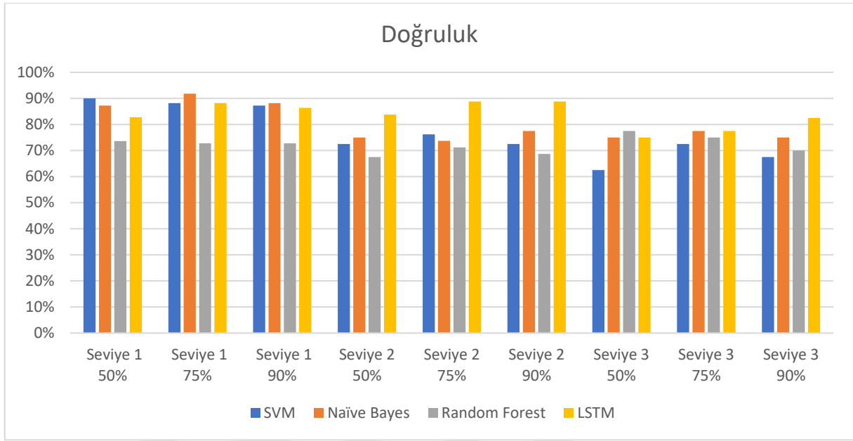
Şekil 6.1. Sınıflandırma yöntemleri için doğruluk oranları
