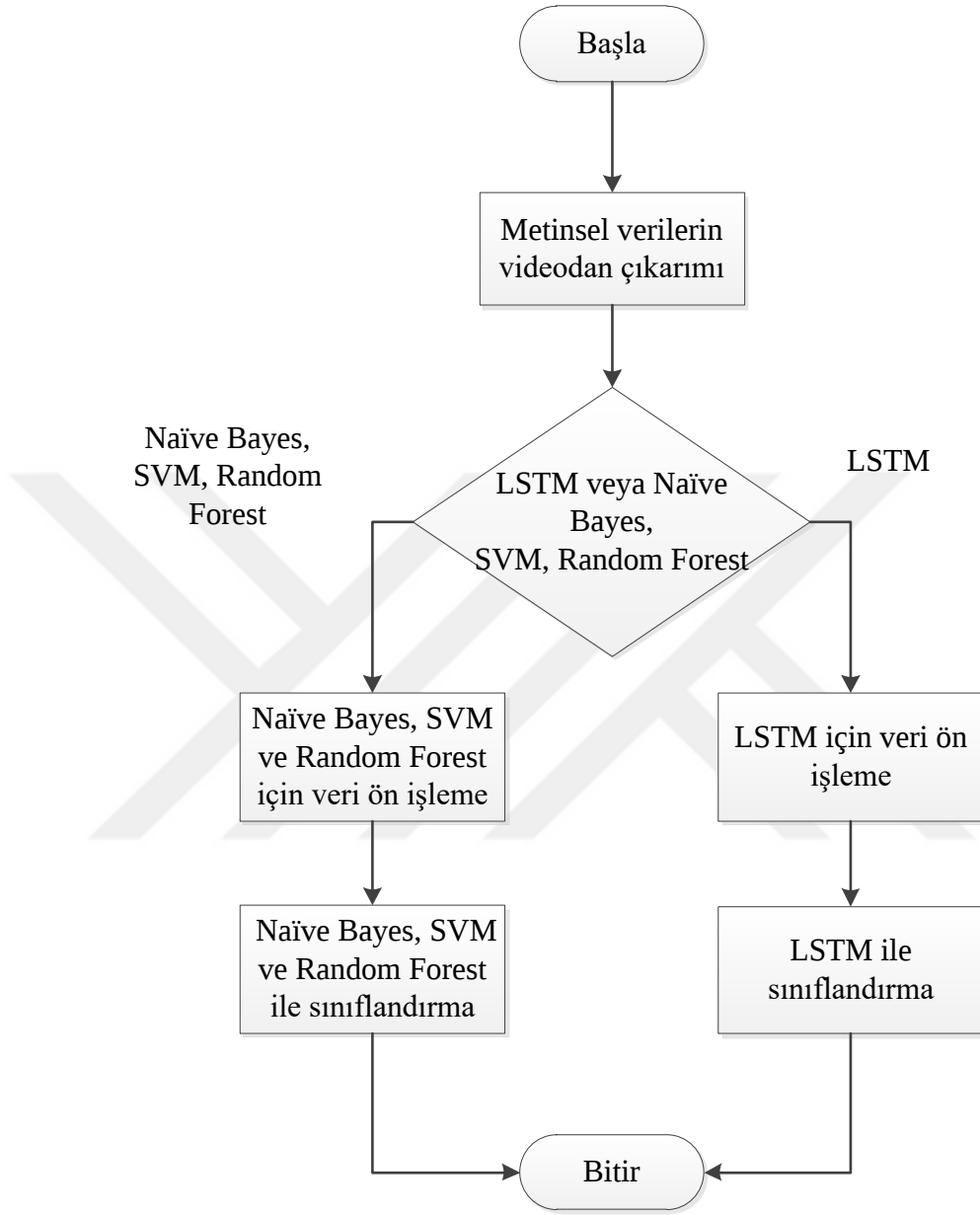
Şekil 4.1. Genel Mimari Akış Şeması
