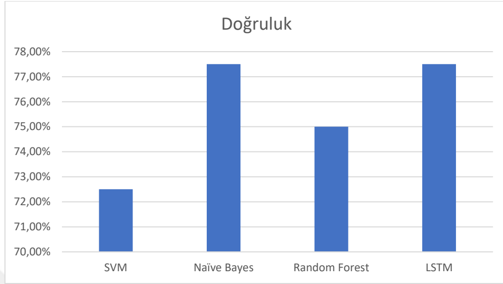
Şekil 5.22. Seviye 3 veri kümesinde %75 benzerlik oranı için sınıflandırma sonuçları
