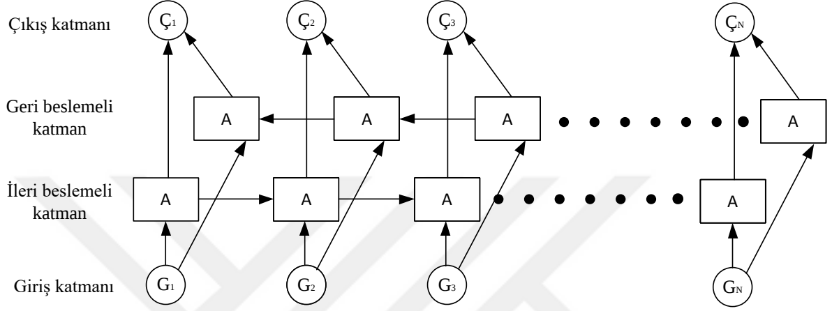
Şekil 3.5. Bidirectional LSTM
