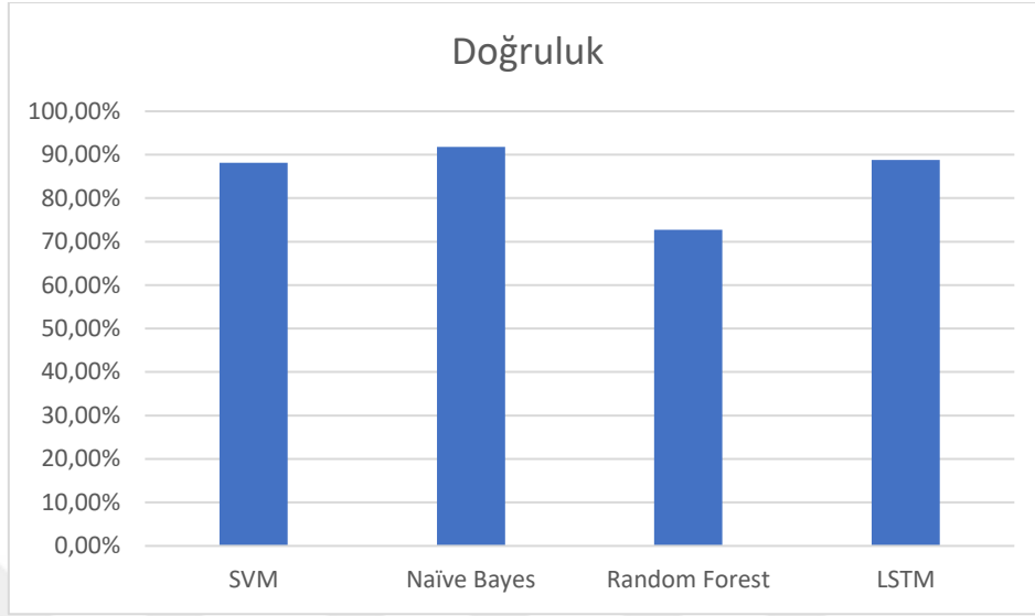
Şekil 5.16. Seviye 1 veri kümesinde %75 benzerlik oranı için sınıflandırma sonuçları
