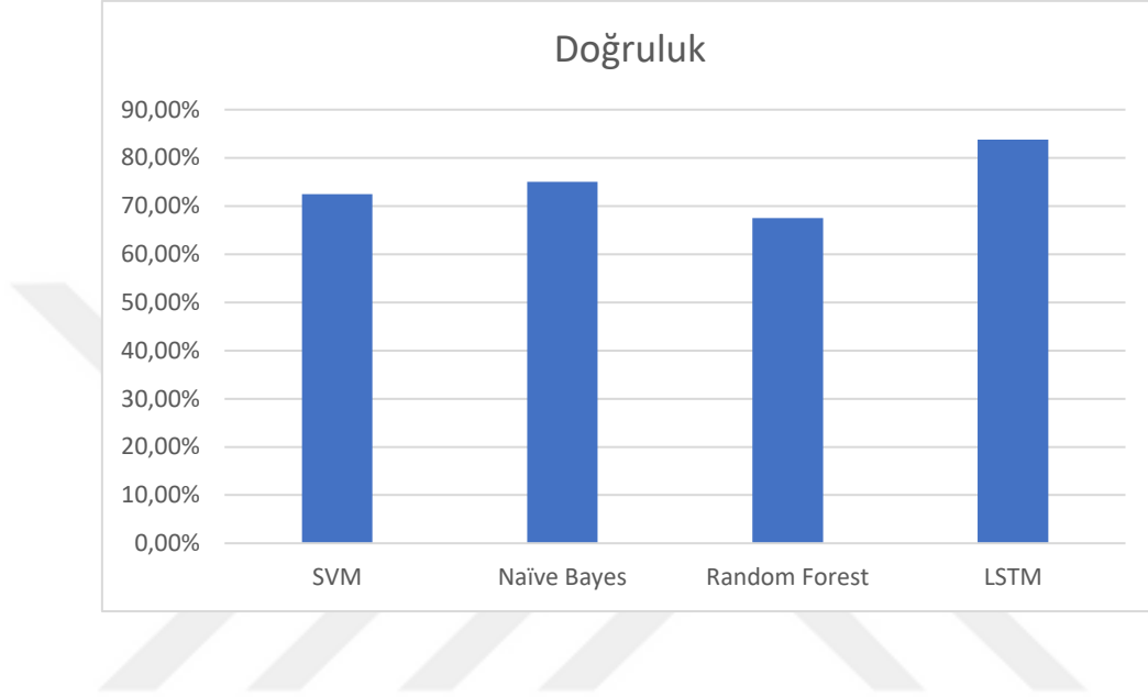
Şekil 5.18. Seviye 2 veri kümesinde %50 benzerlik oranı için sınıflandırma sonuçları
