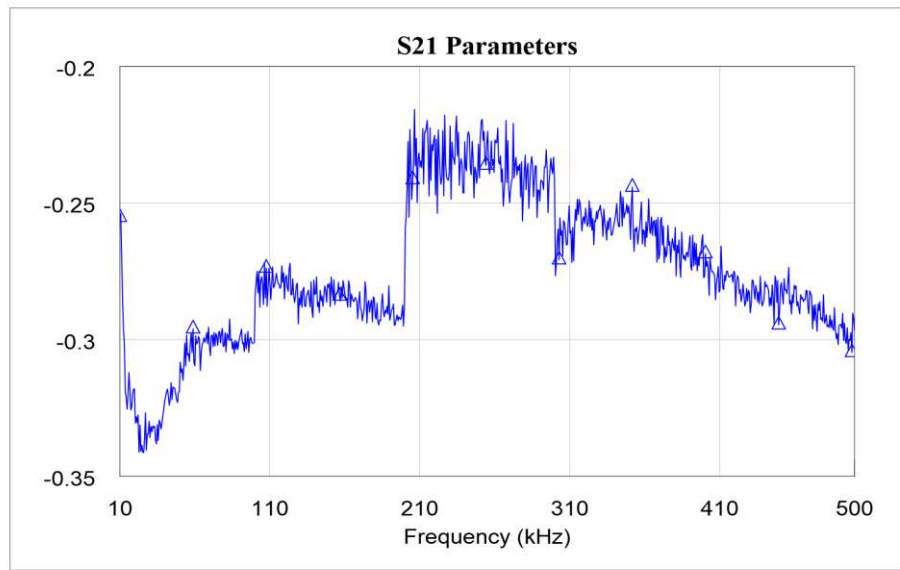
Figure 15 S21 Parameters
