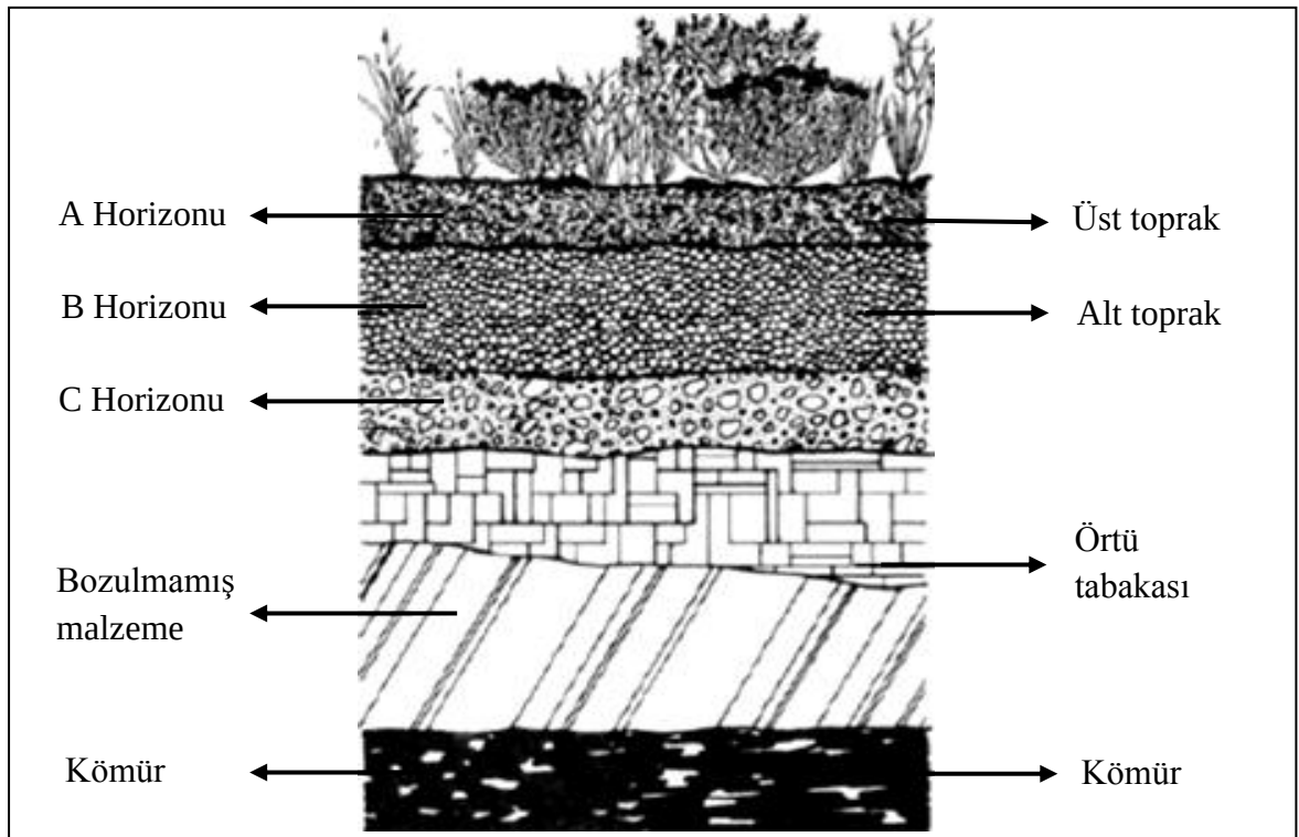
Şekil 2: Bitki örtüsü, üst-alt toprak ve kömürün bulunduğu alan (Karakurt, 2006’dan değiştirilerek).
