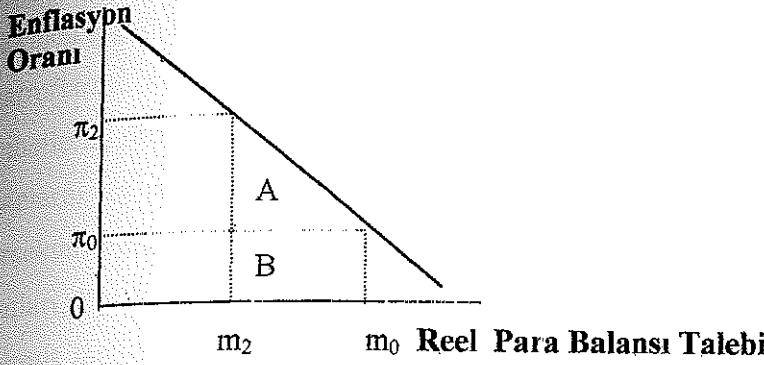
Şekil 1.4: Refah Kaybı
