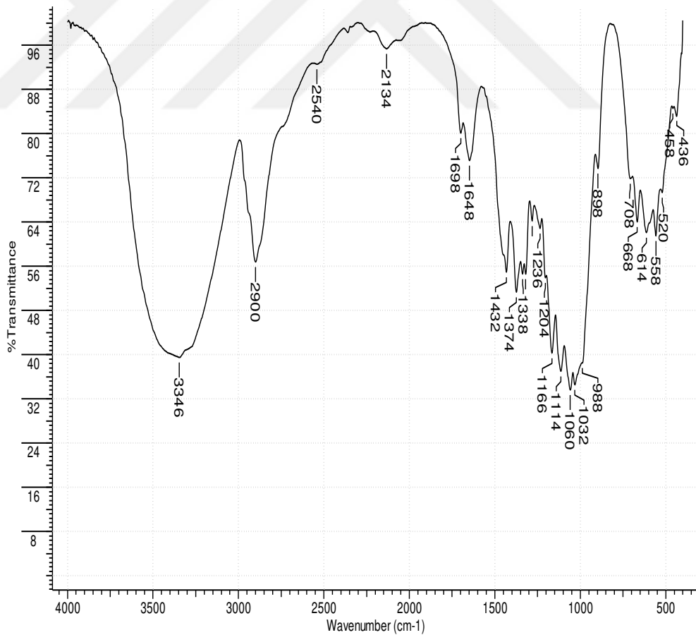
Şekil 5.1. Mikrokristalin selüloza ait FTIR sonucu
