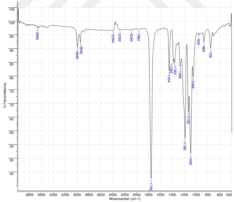
Şekil 5.5. PLA'ya ait FTIR sonucu
