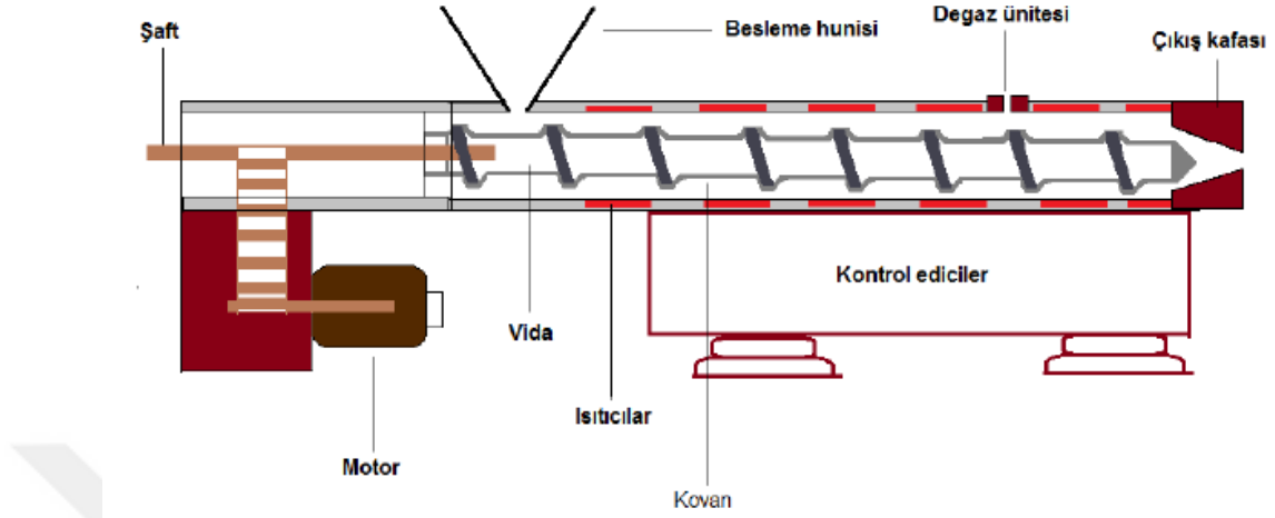
Şekil 2.9. Tek vidalı ekstrüder[14].
