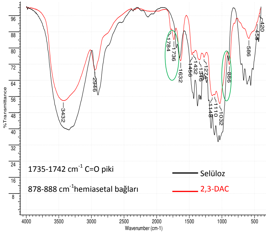
Şekil 5.3. Mikrokrystalin selüloz ve 2,3-DAC FTIR sonuçları
