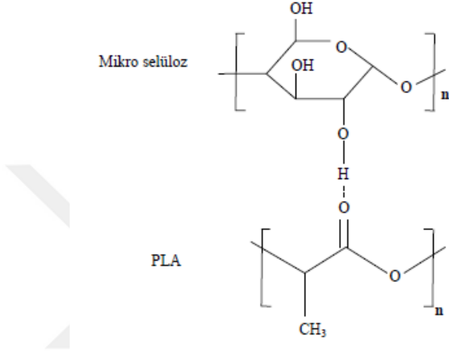
Şekil 6.1. PLA-Selüloz blend yapısı
