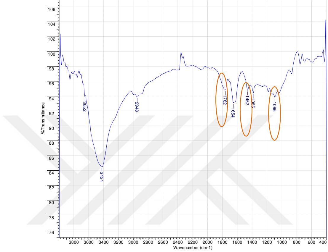
Şekil 5.7. 2,3-DAC/PLA/PEG FTIR sonucu
